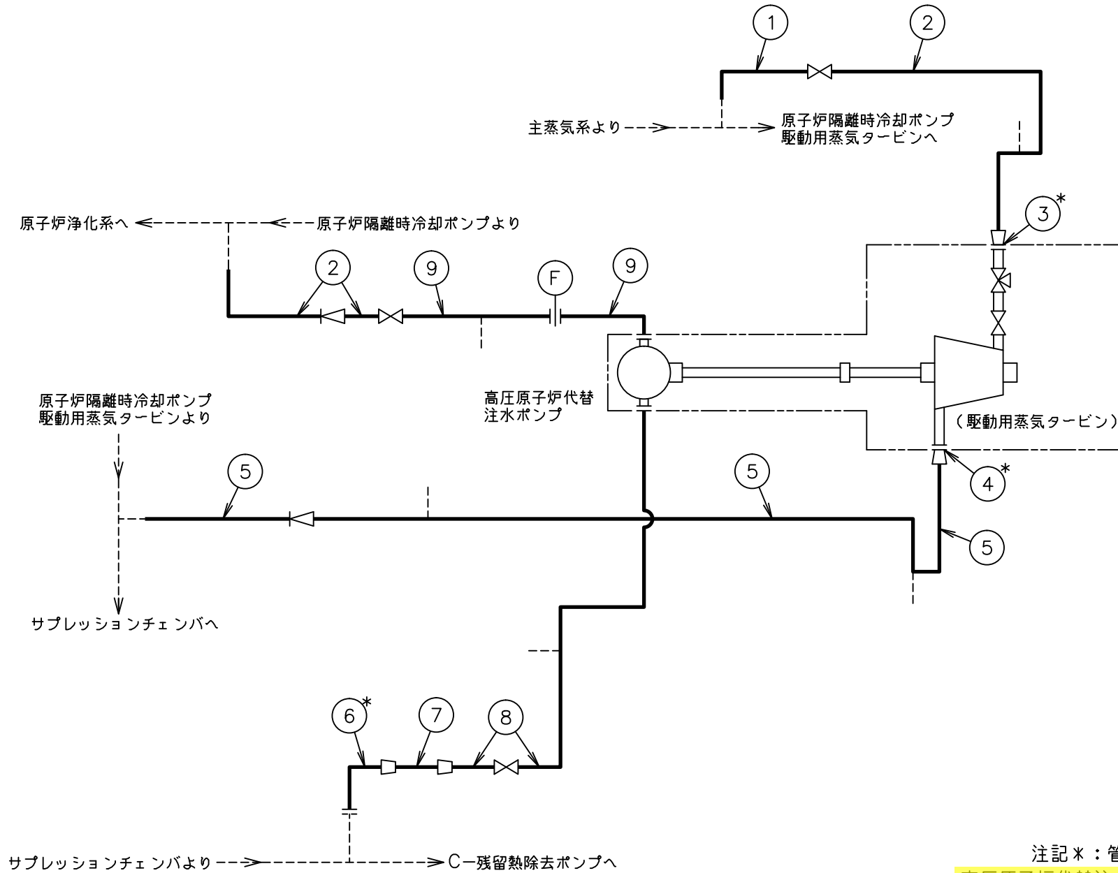
高圧原子炉代替注水系概略系統図
