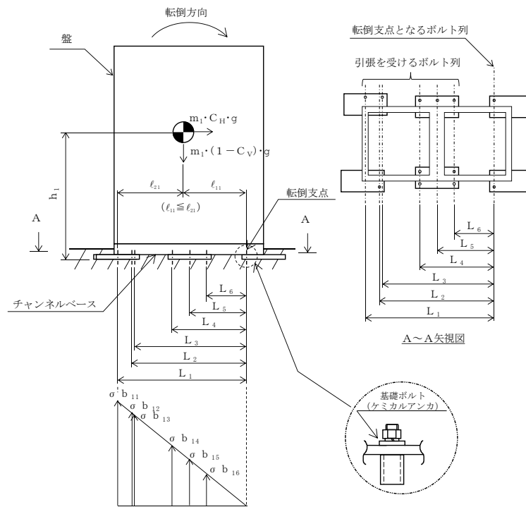
図5-1(5) 計算モデル
