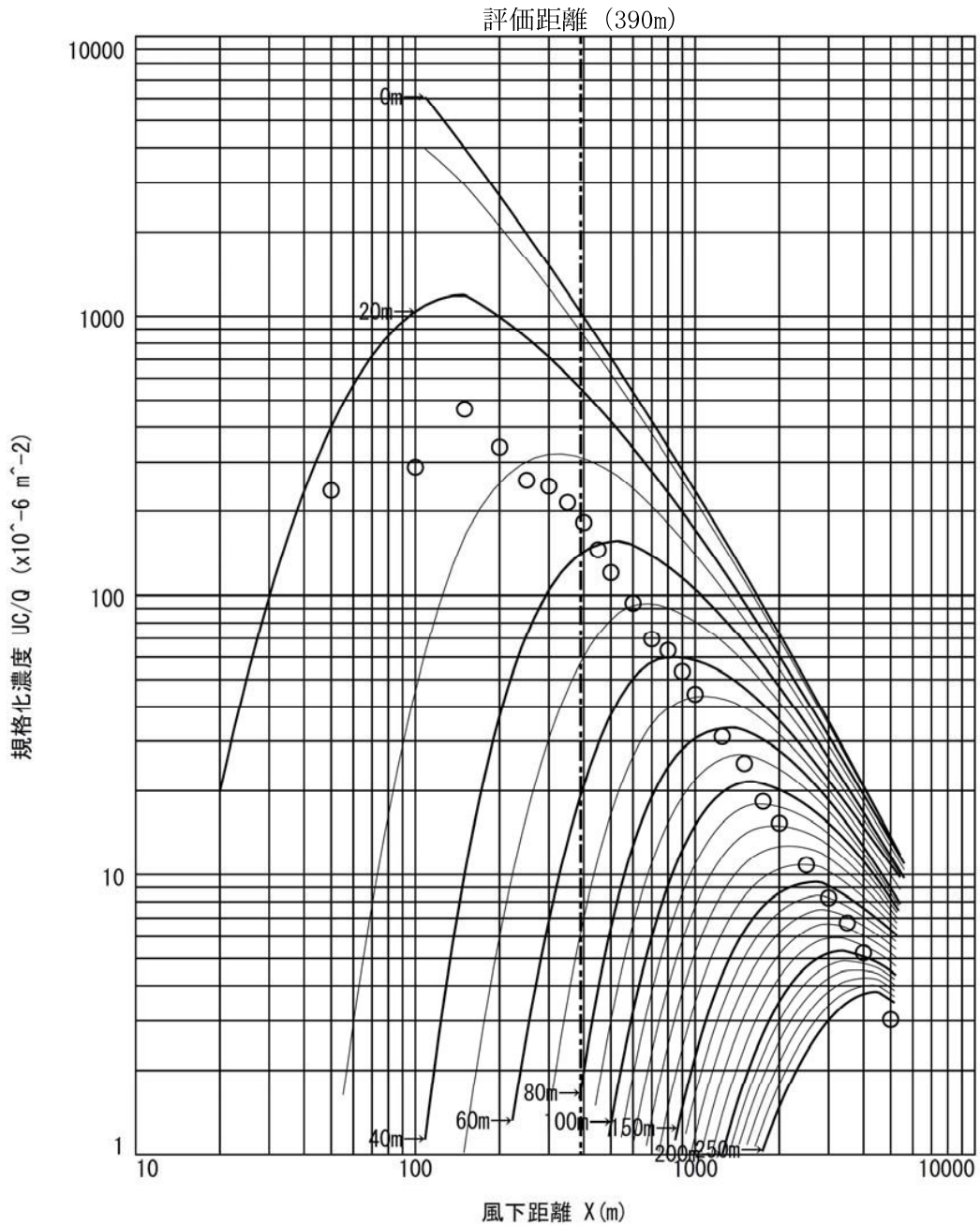
图 5.3-2 地表煙軸濃度分布图 (風向: ENE、排出源: 4号排気筒、事故時)
