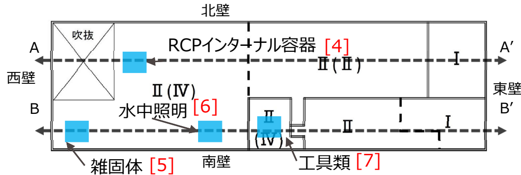
図 地上1階の評価対象壁
