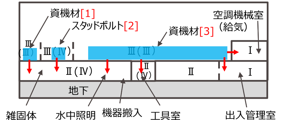
図 地上2階の評価対象壁
