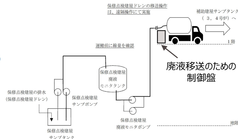
図 廃液の運搬容器への移送
