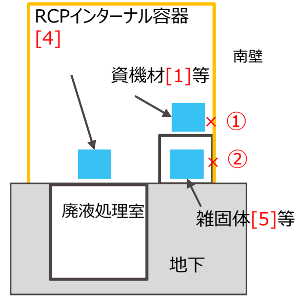
図 立面図 (C-C'断面)
