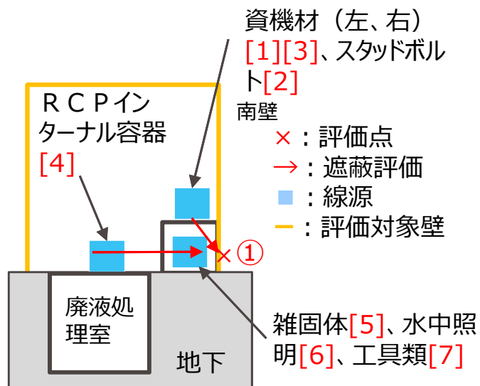
図 評価点②（南壁）評価イメージ（C-C'断面）
