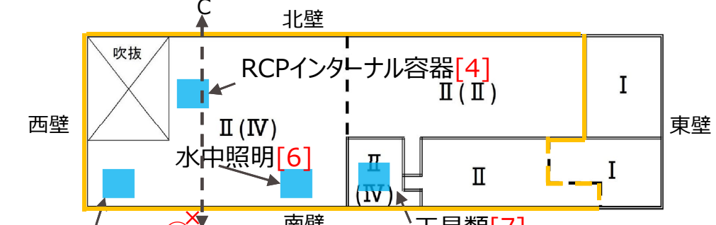
図 地上1階の評価対象壁
