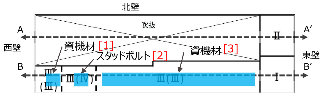
図 地上2階の評価対象壁
