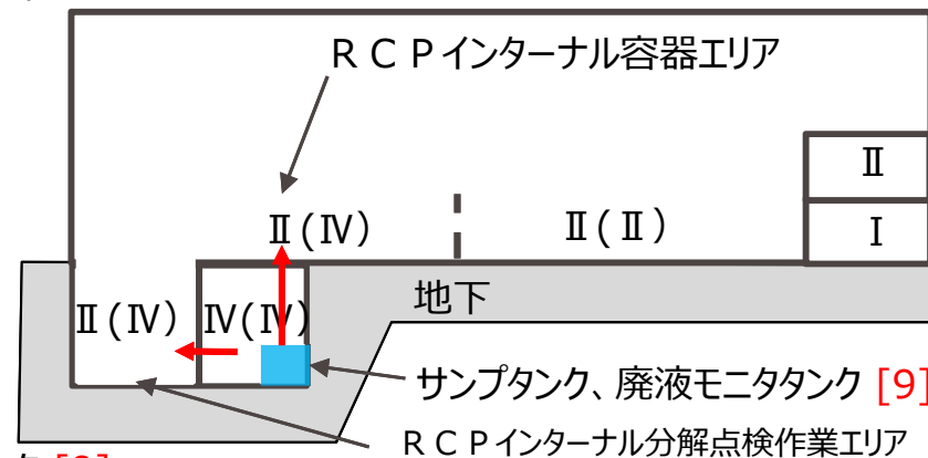
図 立面図 (A-A'断面)
