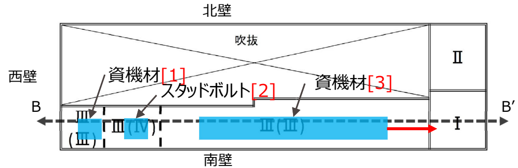
図 地上2階の評価対象壁
