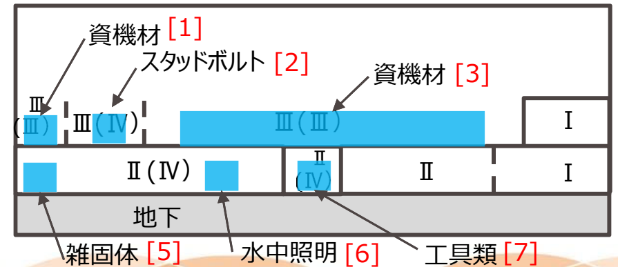
図 立面図 (B-B'断面)
