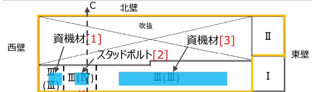
図 地上2階の評価対象壁
