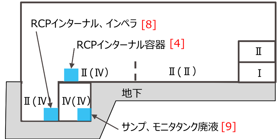
図 立面図 (A-A'断面)
