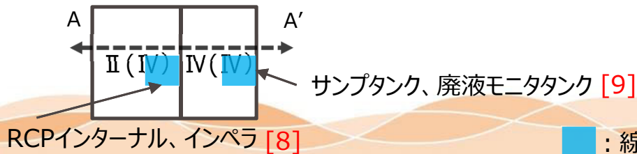
図 地階 評価対象壁
