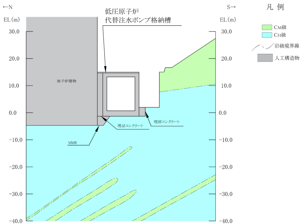
図 3-3 低圧原子炉代替注水ポンプ格納槽 評価対象断面図 (B-B断面)
