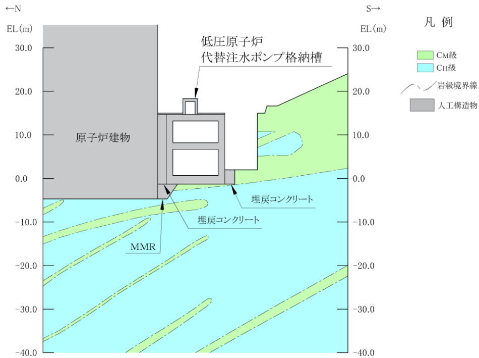
図 3-2 低圧原子炉代替注水ポンプ格納槽 評価対象断面図 (A-A断面)
