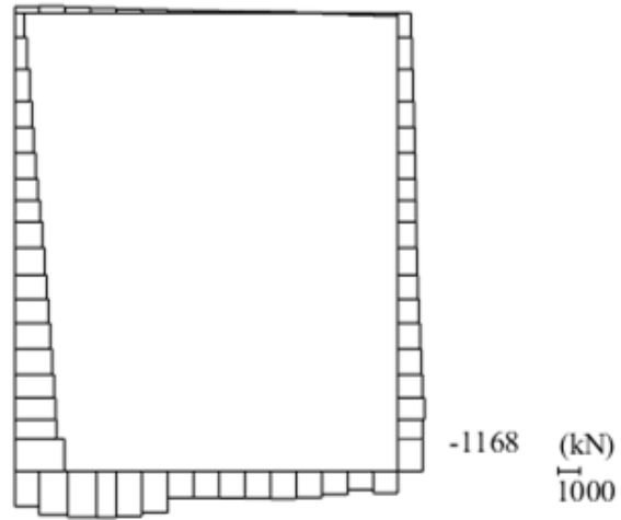
数値：評価位置における断面力 (b) 軸力 (kN) (+ : 引張, - : 圧縮)
