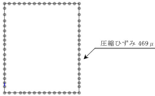
図 3-5 曲げ・軸力系の破壊に対する照査におけるひずみ（コンクリート）の時刻歴波形（B-B断面，解析ケース③，S s -N1（++））
