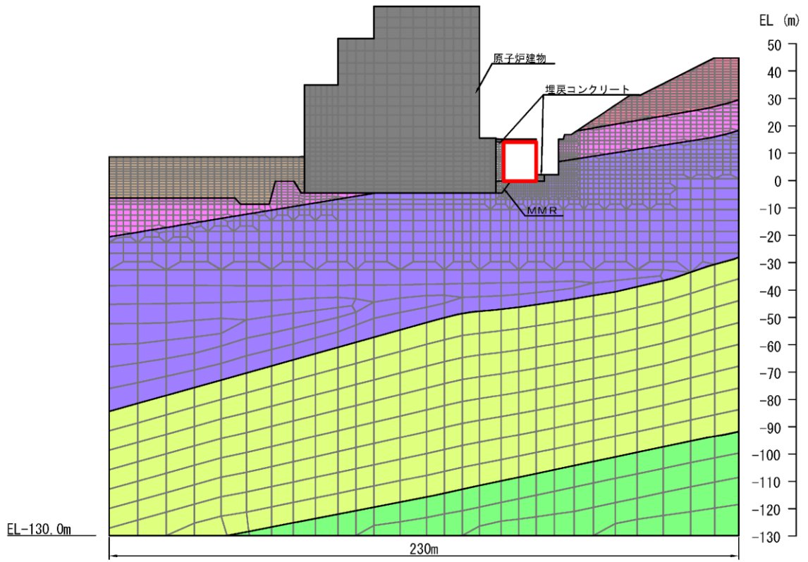
(全体図)
