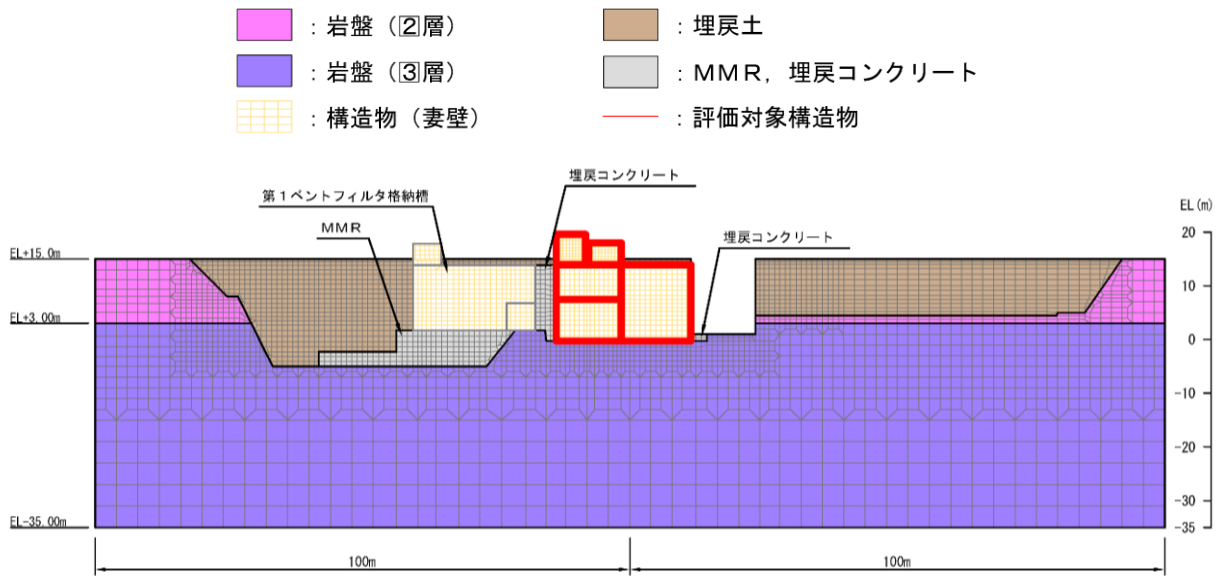
(全体図)
