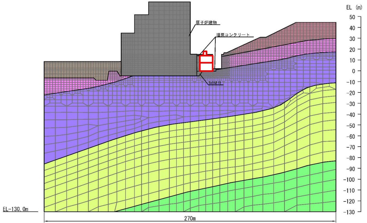
(全体図)
