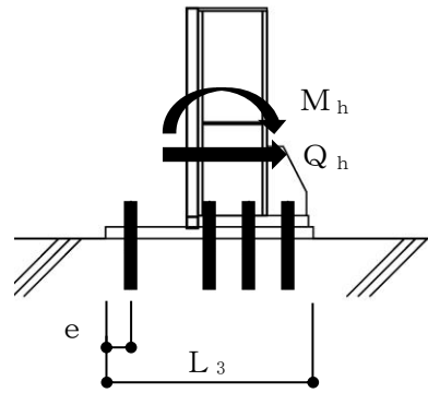
図 4-4 地震時のアンカーボルトに生じる力の断面概念図
