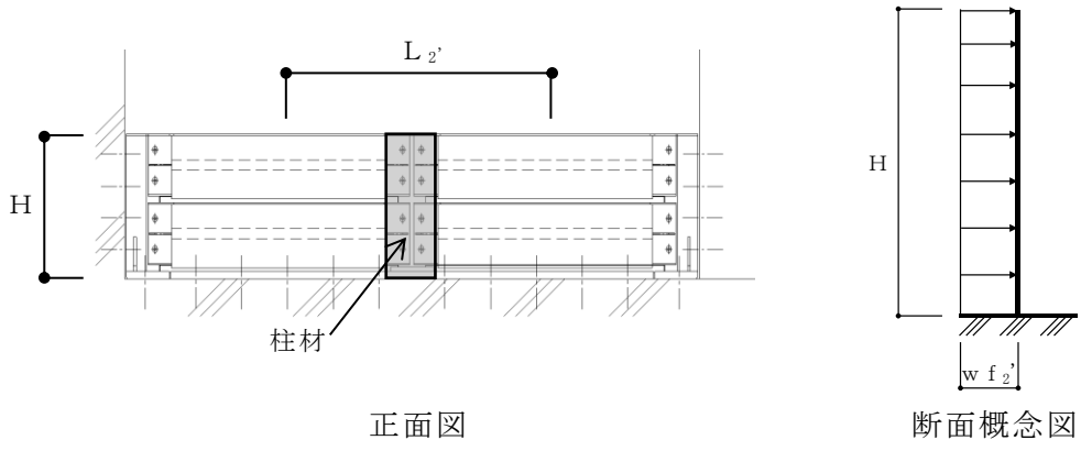
図 4-3 地震時の柱材に生じる力の断面概念図
