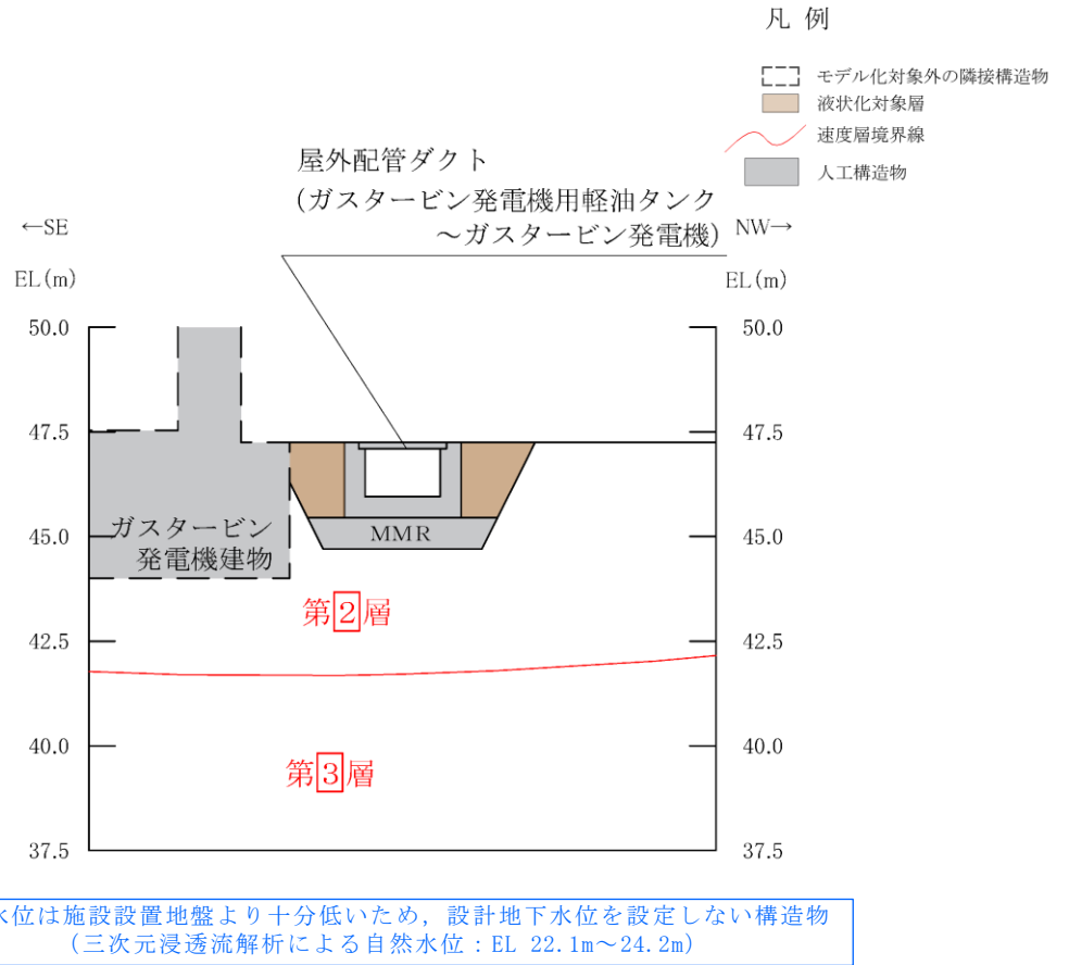
図 3-2 屋外配管ダクト (ガスタービン発電機用軽油タンク～ガスタービン発電機) 評価対象断面図 (A-A 断面位置)
