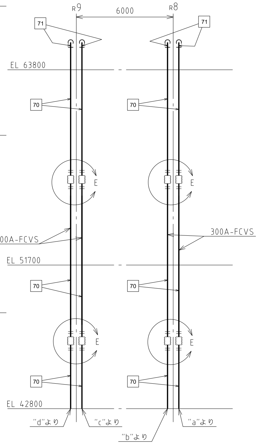
B~B矢视图
