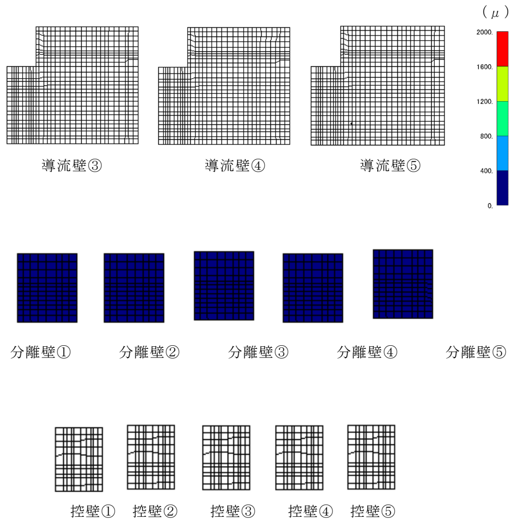
図 4-6 (2) 曲げ・軸力系の破壊に対する照査値最大時のひずみ分布図 (主筋ひずみ) (中床版, 解析ケース②, S_s - D (-+) )
