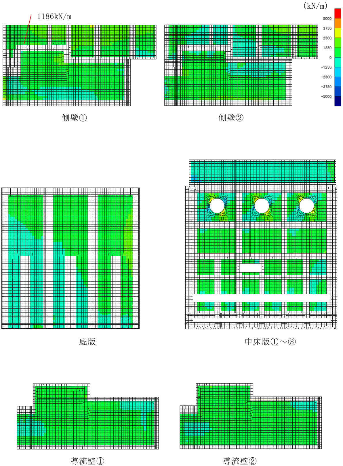
図 4-10 (1) せん断破壊に対する照査値最大時の断面力分布図
