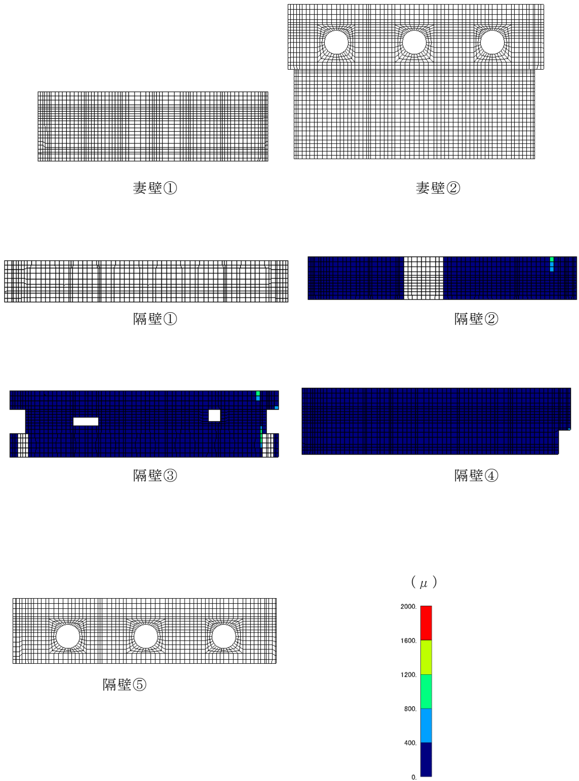
図 4-6 (3) 曲げ・軸力系の破壊に対する照査値最大時のひずみ分布図 (主筋ひずみ) (中床版, 解析ケース②, S s -D (-+))
