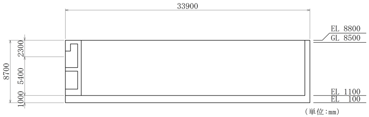
图 2-5 取水槽断面图 (C-C 断面)
