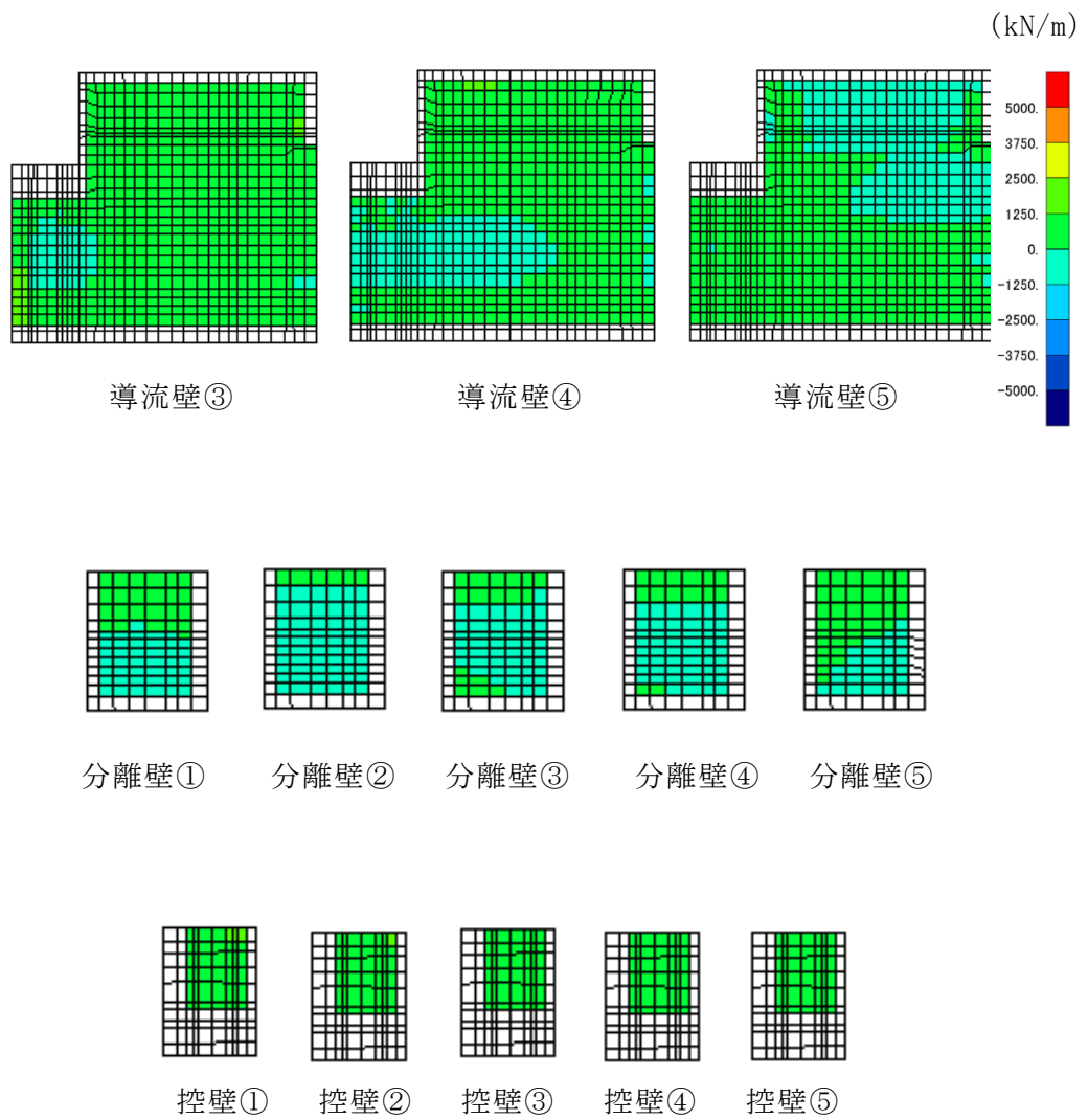
図 4-10 (2) せん断破壊に対する照査値最大時の断面力分布図
