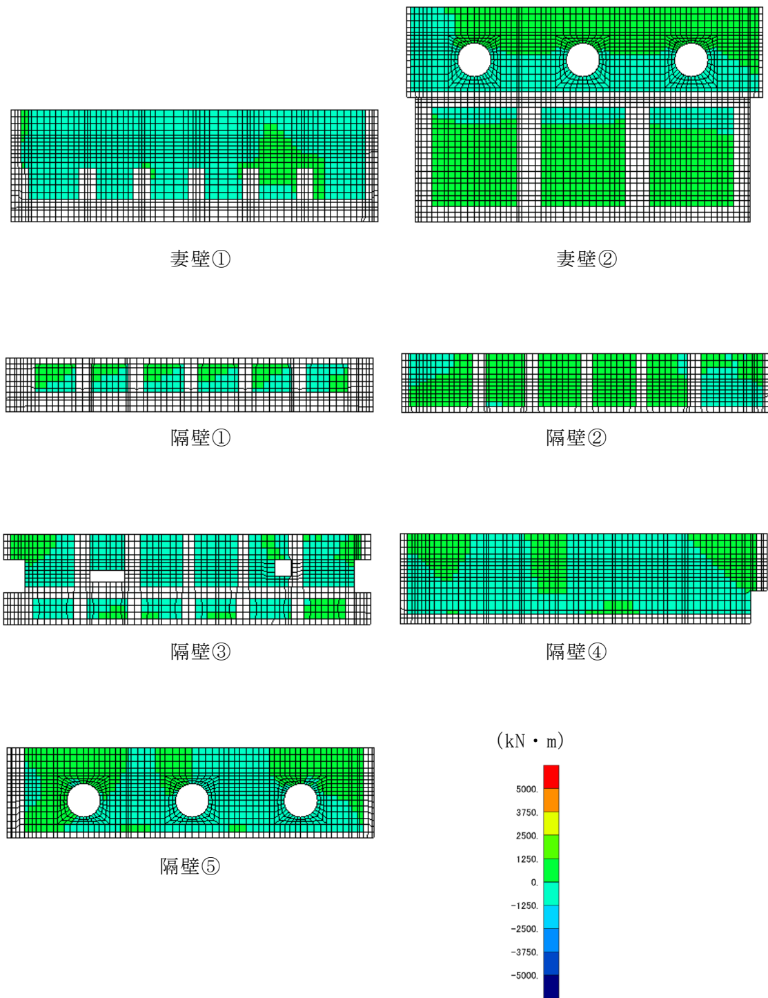
図 4-8 (3) せん断破壊に対する照査値最大時の断面力分布図
