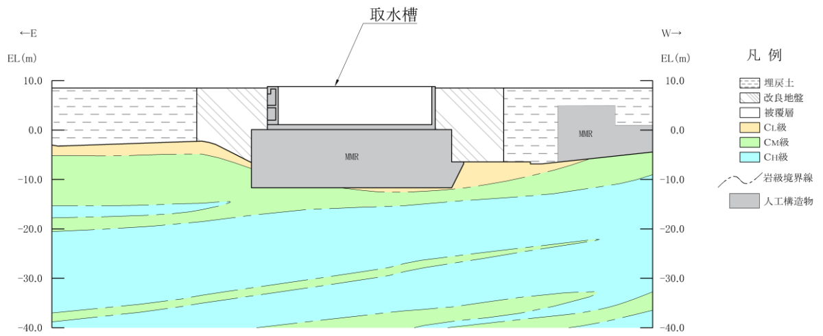
図 3-4 取水槽 地震時荷重算出用地質断面図 (C-C断面位置)
