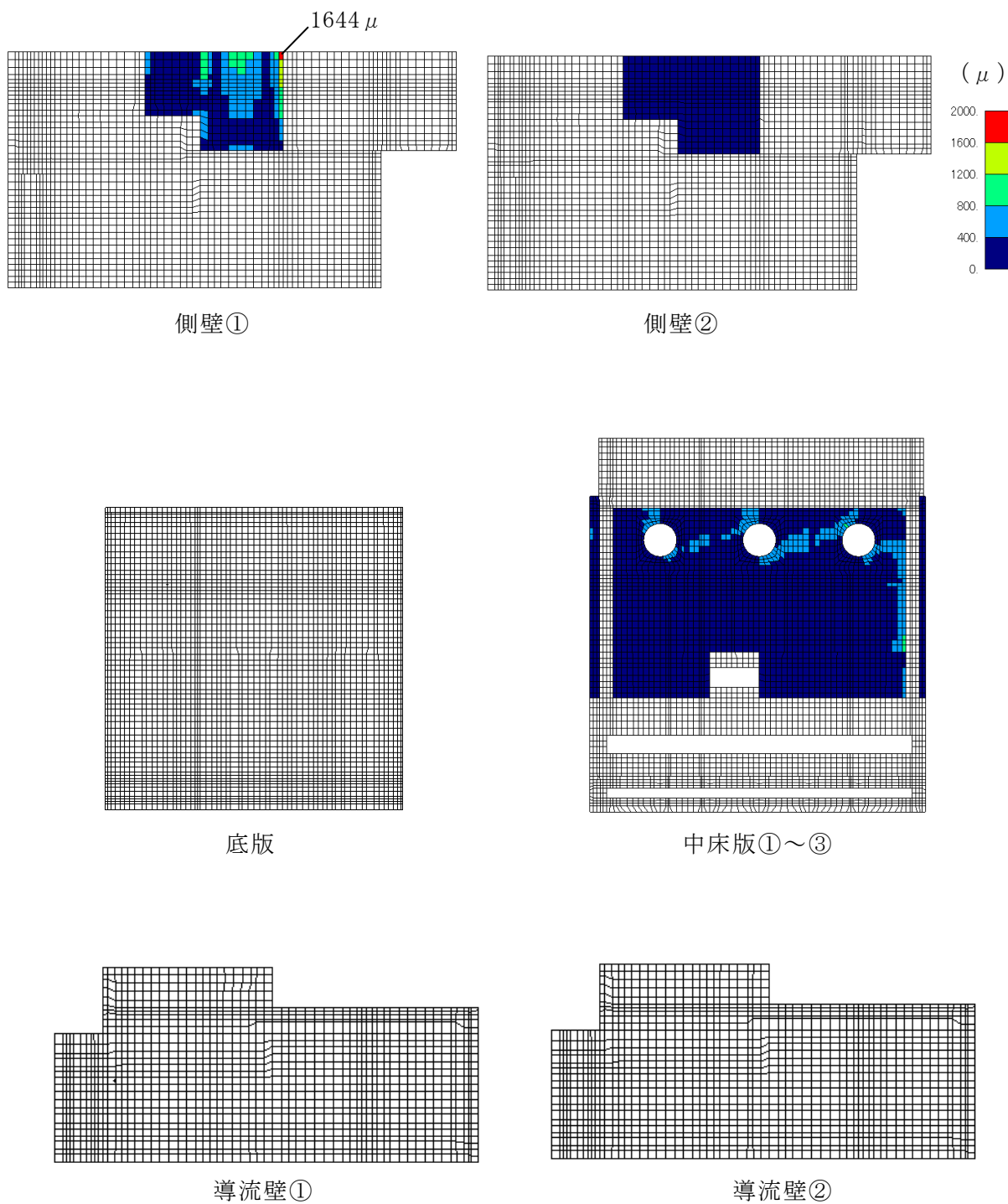
図 4-5 (1) 曲げ・軸力系の破壊に対する照査値最大時のひずみ分布図 (コンクリートの圧縮ひずみ) (側壁, 解析ケース④, S_s - D (-+) )
