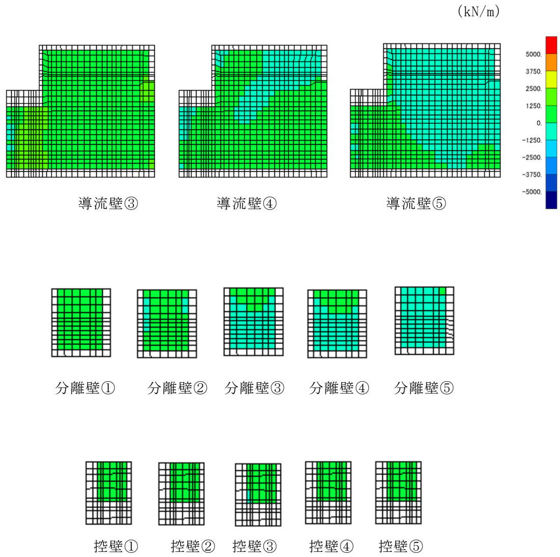
図 4-9 (2) せん断破壊に対する照査値最大時の断面力分布図
