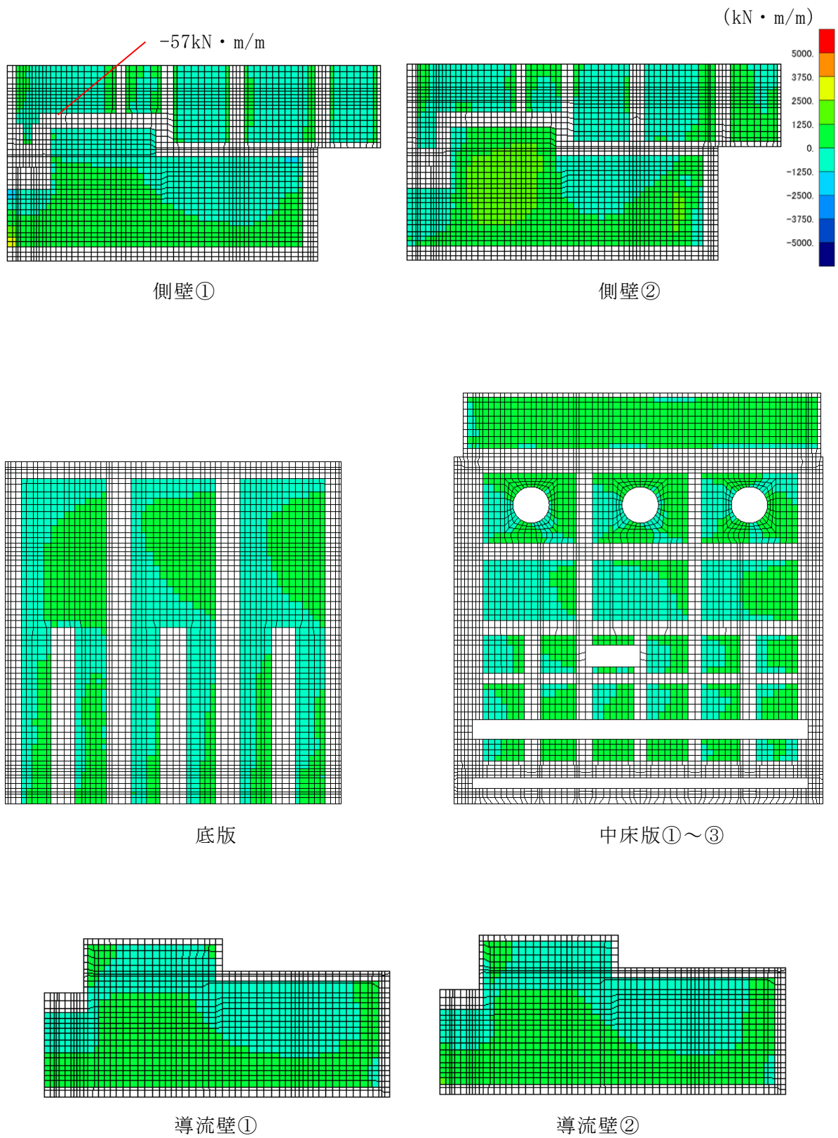
図 4-8 (1) せん断破壊に対する照査値最大時の断面力分布図
