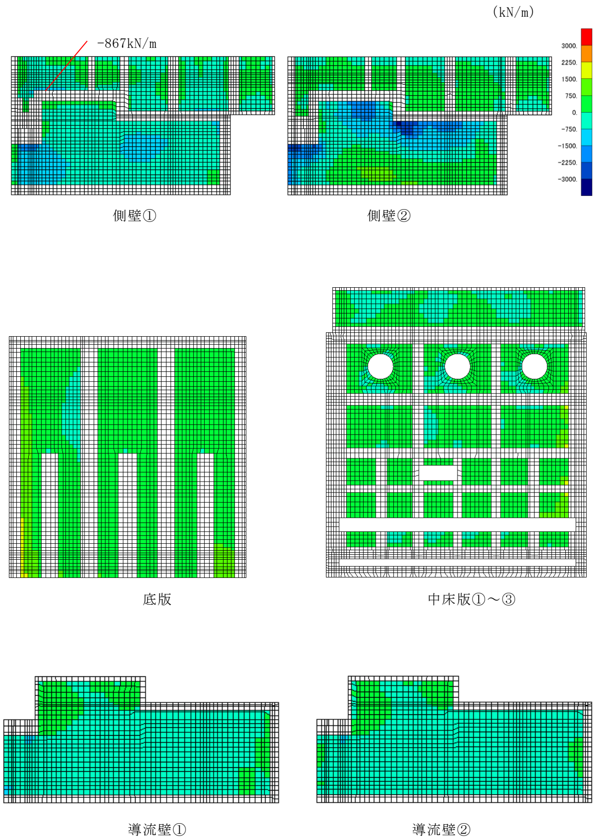
図 4-11 (1) せん断破壊に対する照査値最大時の断面力分布図
