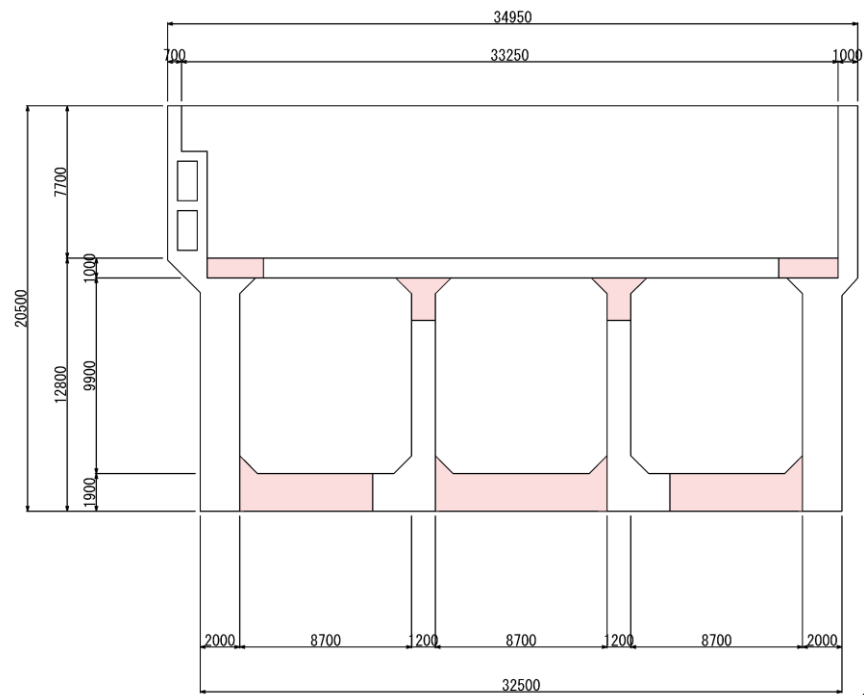
図 2-14 せん断補強計画図 (B-B断面)
