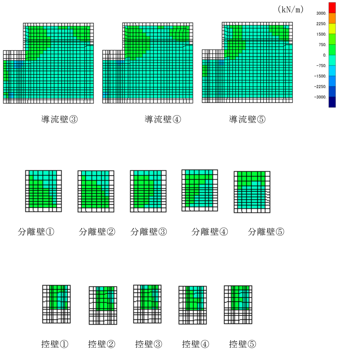
図 4-11 (2) せん断破壊に対する照査値最大時の断面力分布図
