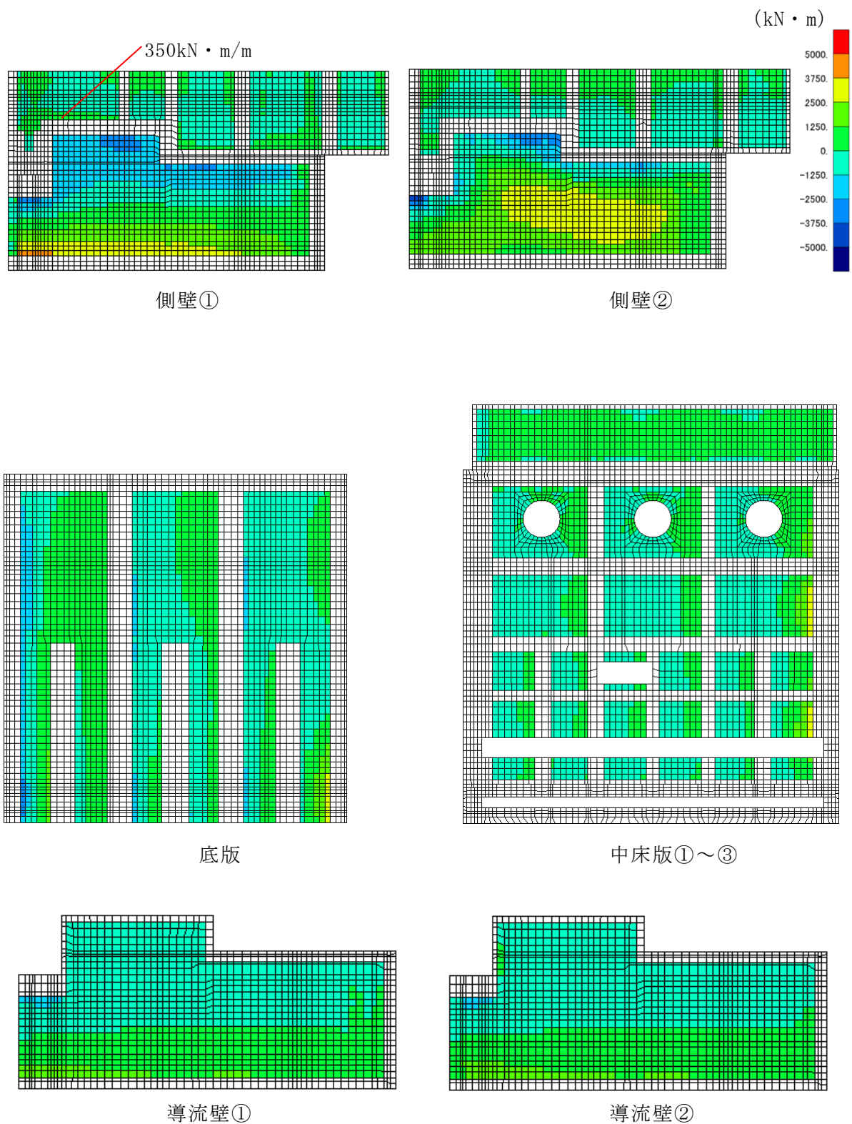
図 4-7 (1) せん断破壊に対する照査値最大時の断面力分布図
