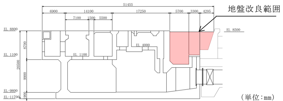
(D - D 断面)
