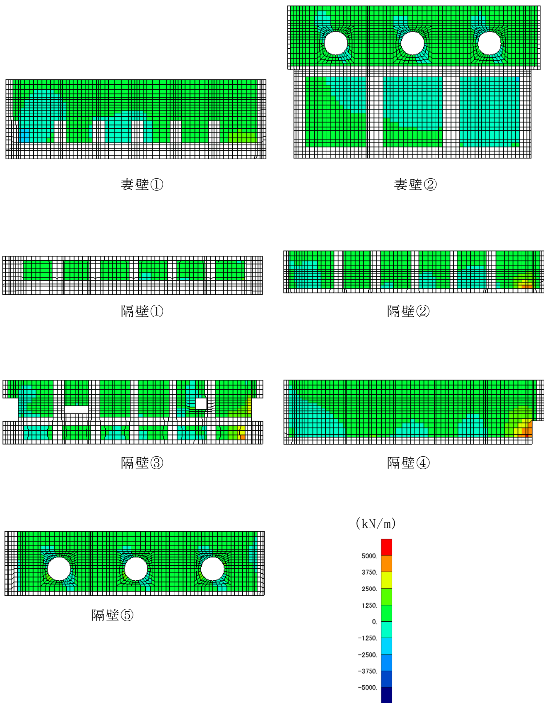
図 4-10 (3) せん断破壊に対する照査値最大時の断面力分布図
