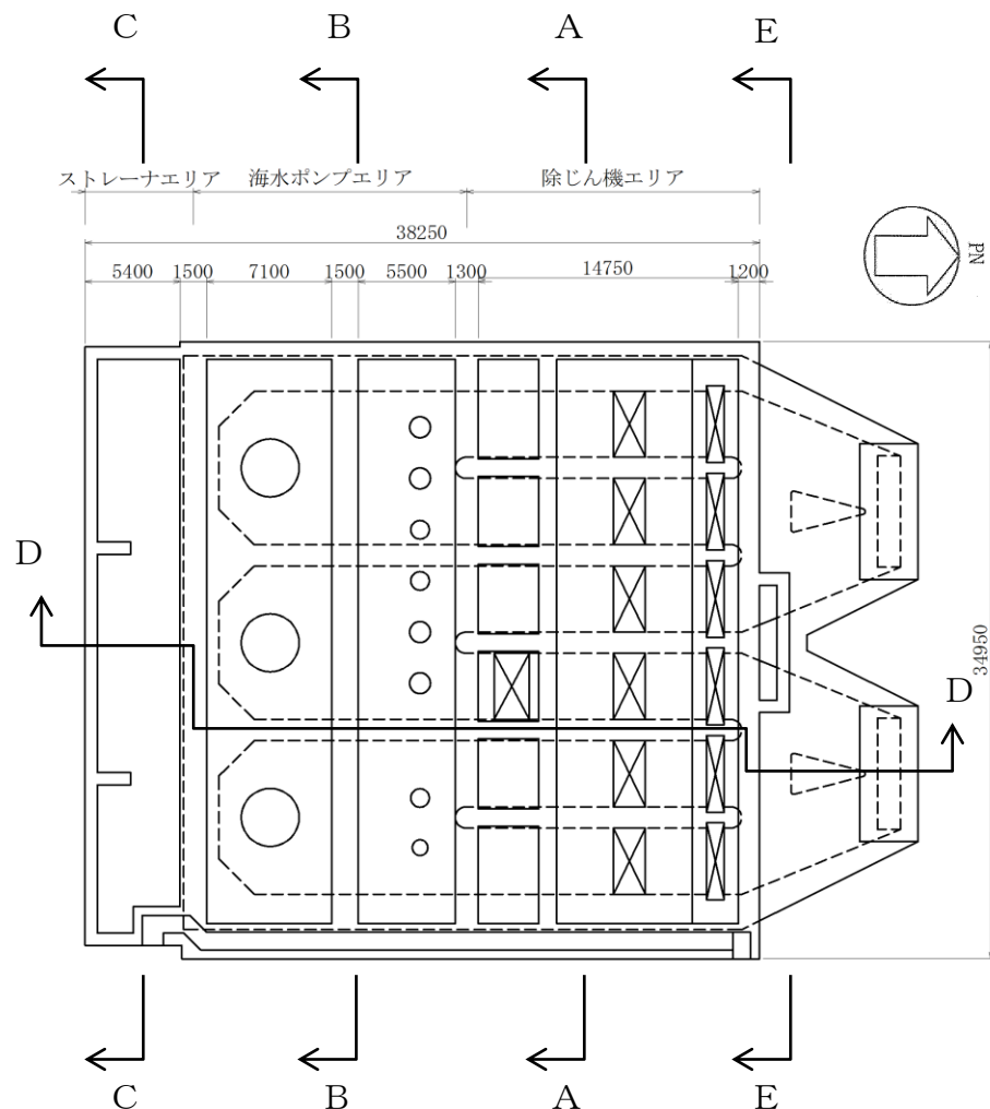
図 3-1 取水槽の地震時荷重算出断面位置図
