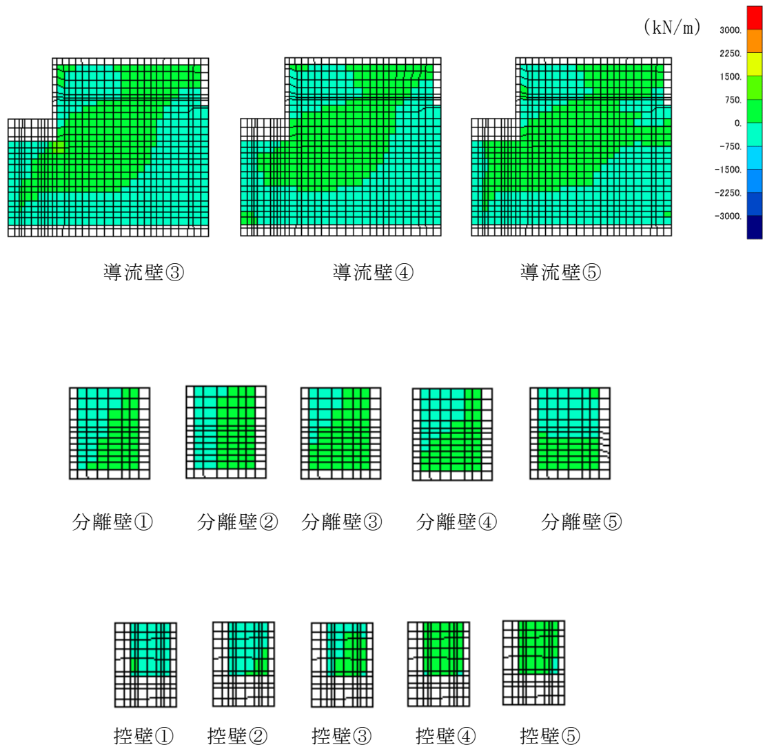
図 4-12 (2) せん断破壊に対する照査値最大時の断面力分布図
