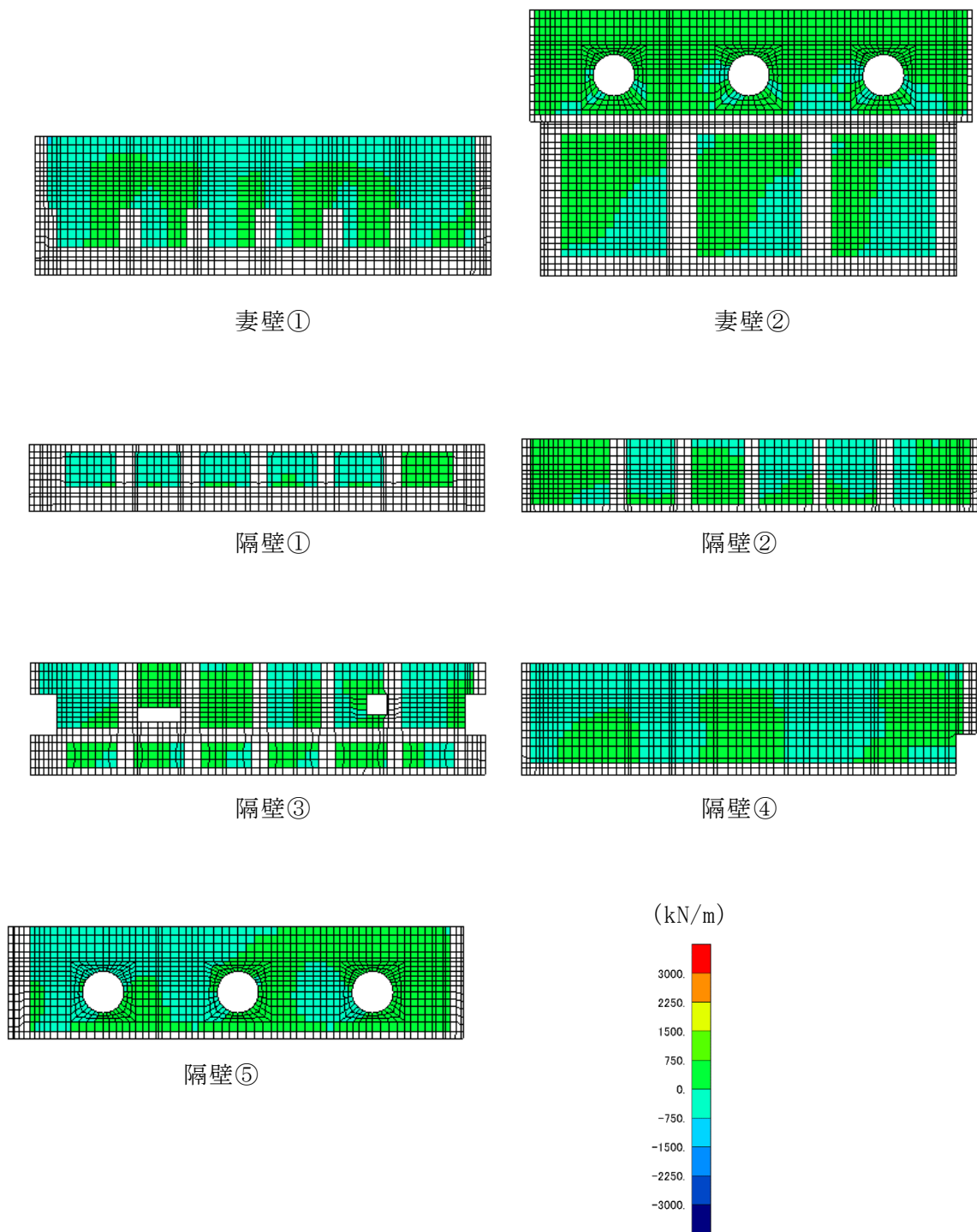
図 4-11 (3) せん断破壊に対する照査値最大時の断面力分布図
