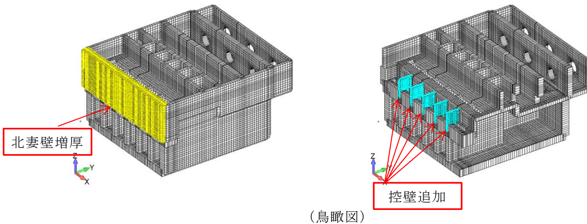
図 2-12 取水槽妻壁補強概要図
