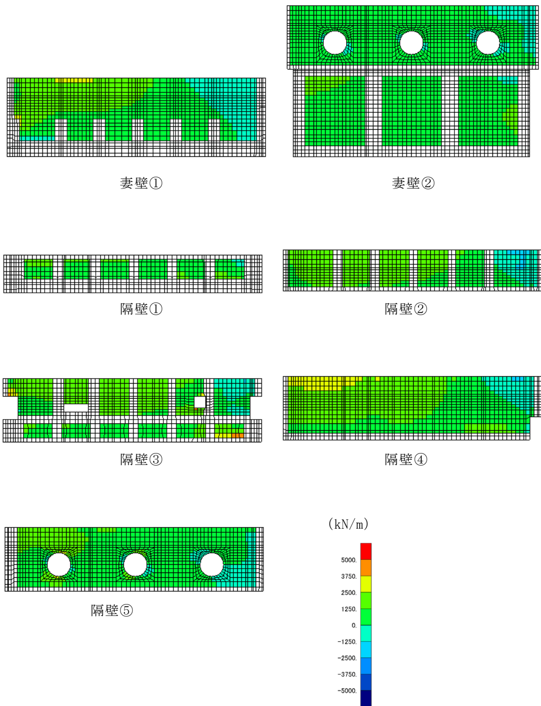
図 4-9 (3) せん断破壊に対する照査値最大時の断面力分布図
