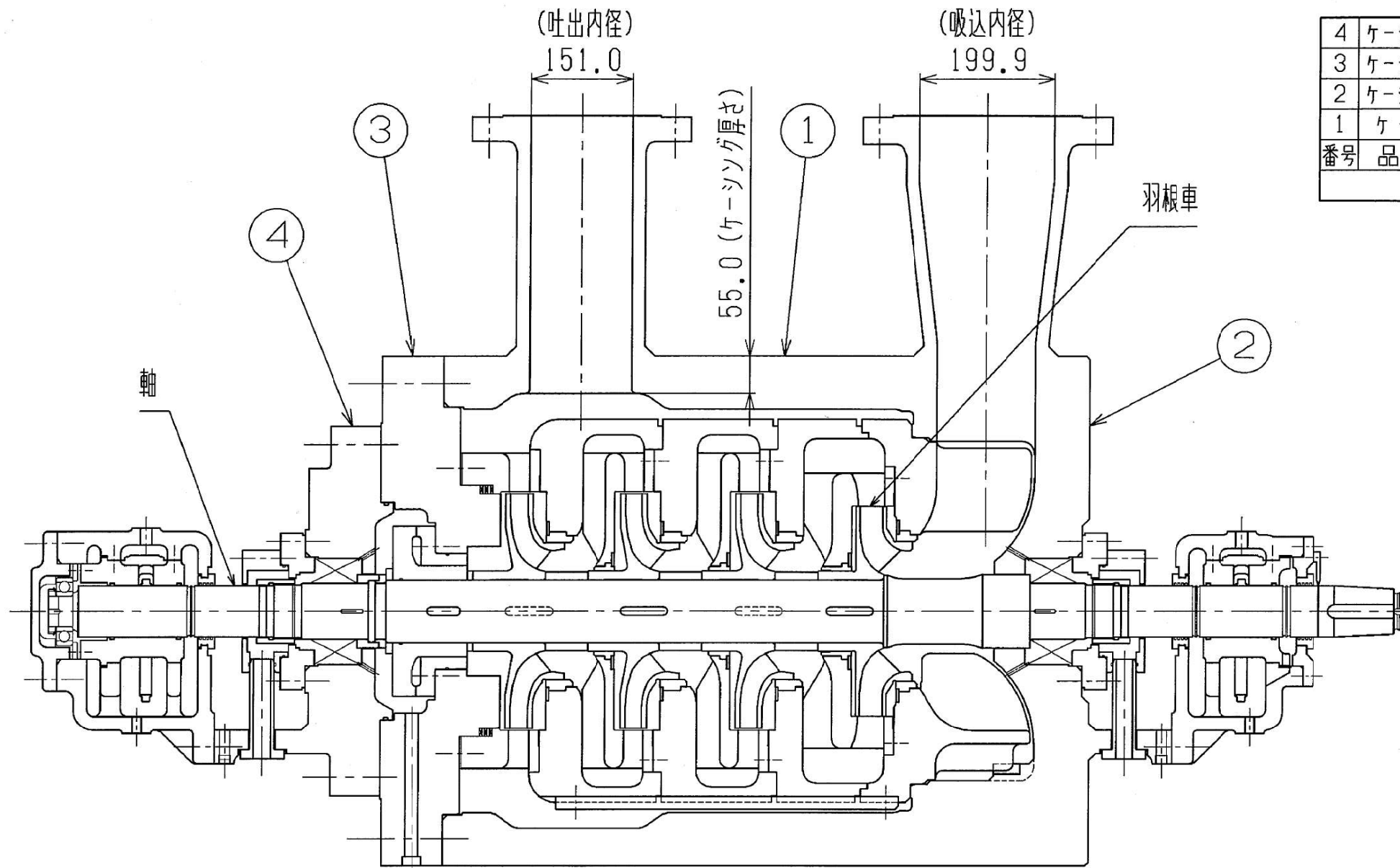
A~A断面図
