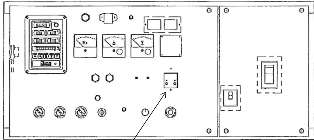
漏電継電器
