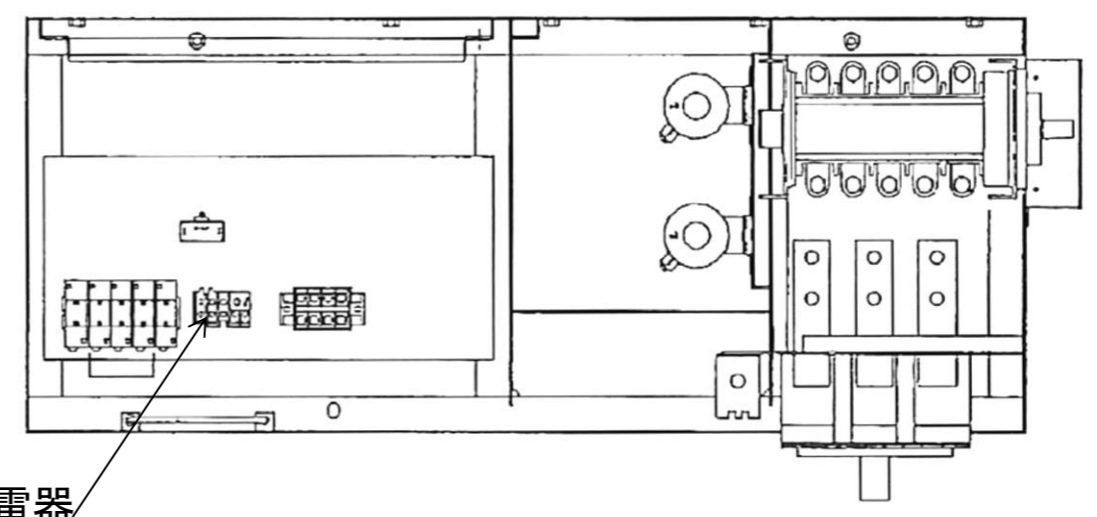
A~A矢視図
