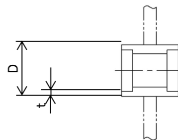
タイプ-1 (管台外径(燃料移送ポンプ吸込, 燃料油取出口))
