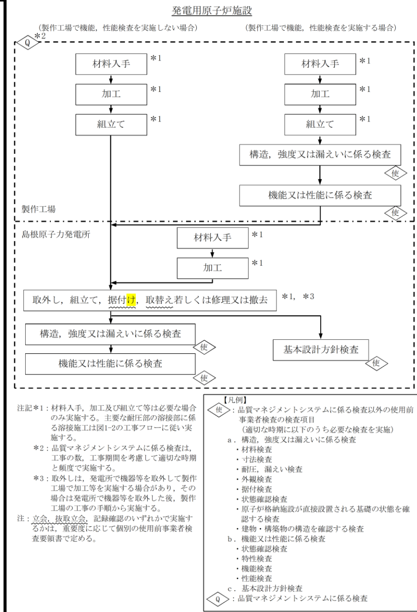
図1-1 工事の手順と使用前事業者検査のフロー (燃料体を除く)
