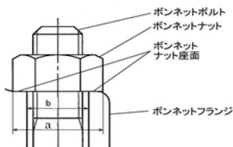
別図3-2 ボンネットナット座面
