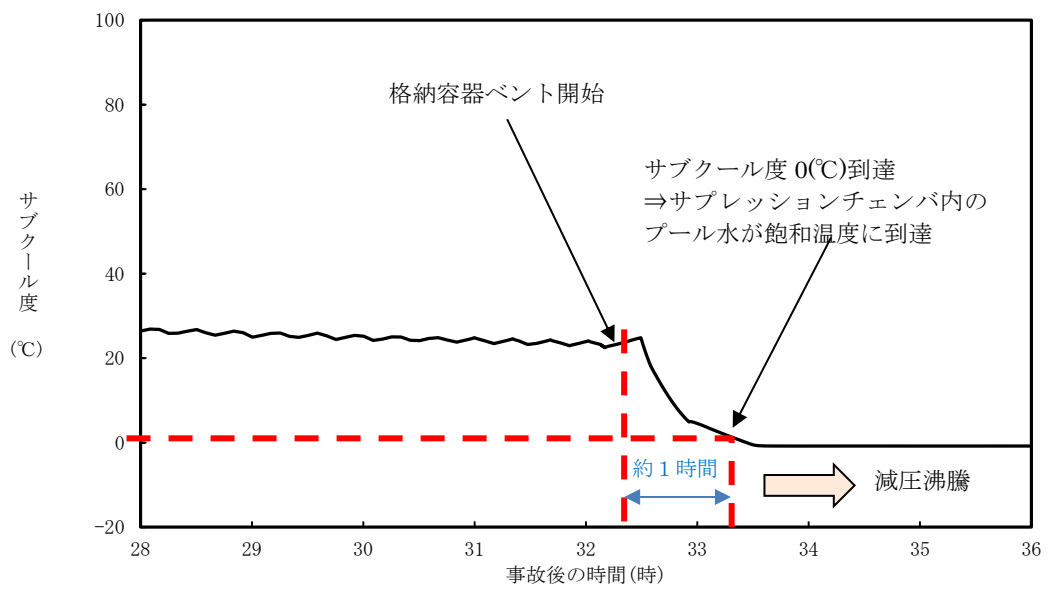
図 5-2 サプレッションプール水のサブクール度
