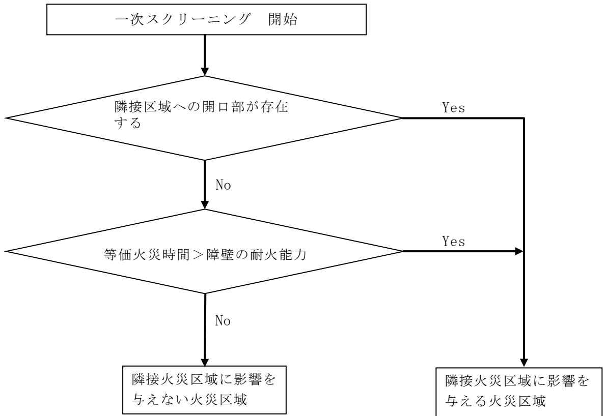
図 7-1 一次スクリーニング：火災伝播評価手順の概要フロー
