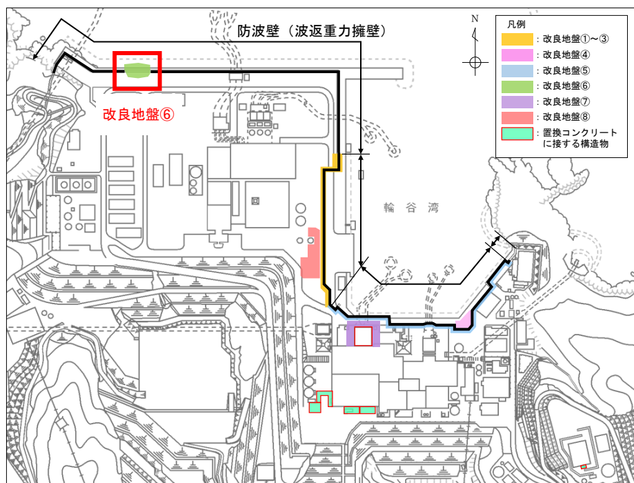
図 6.1.1-1 改良地盤を設置する施設の平面配置図
