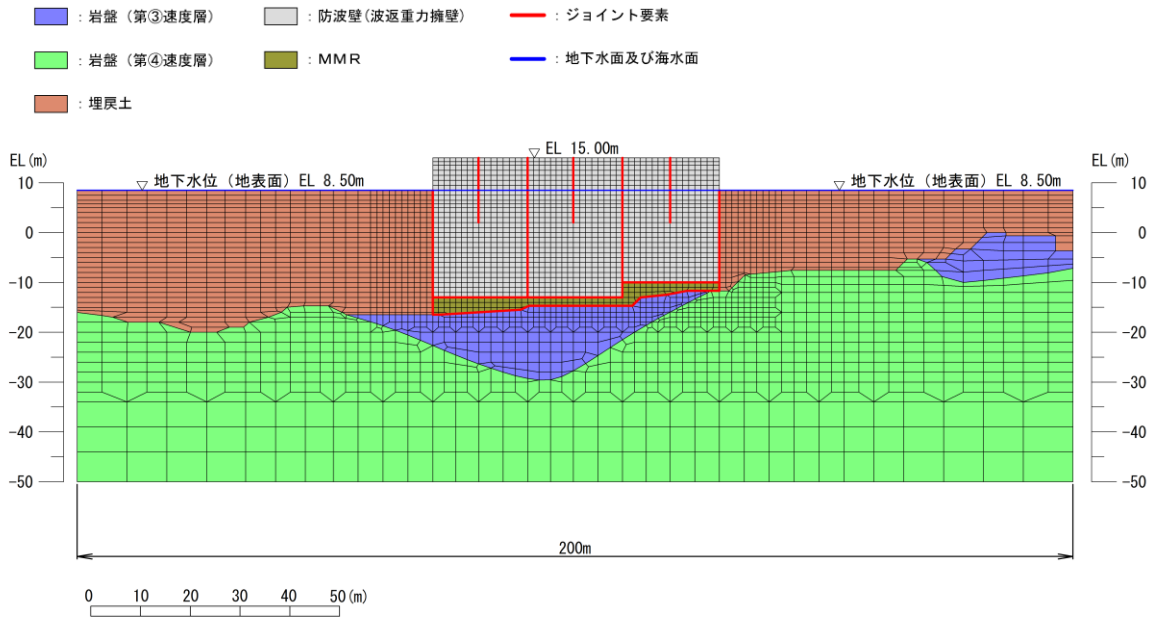
図 4.1.7-10 地震応答解析モデル (⑦-⑦断面)
