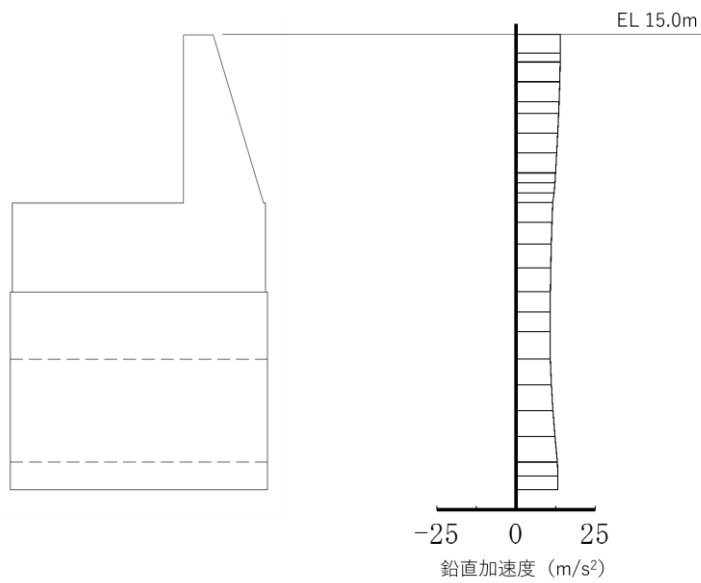
鉛直加速度
