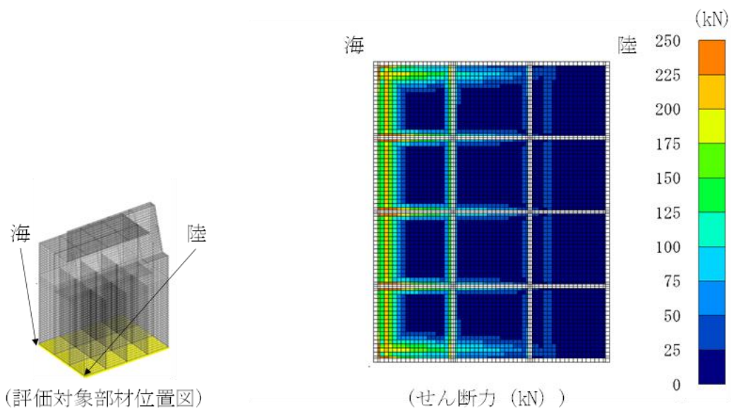
図 5.2.6-1(2) コンクリートのせん断破壊 (面外) に対する照査に用いる断面力図 (④-④断面, S_s - N1 (- +) , 評価対象部材: 底版) 解析ケース②: 地盤物性のばらつきを考慮した解析ケース (平均値+ 1\sigma )
