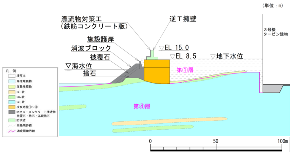
図 3.5.2-7 地質断面図 (⑤-⑤断面)
