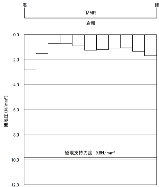
図 4.2.11-2(2) 支持地盤の接地圧分布図 (③-③断面, 岩盤) ( S_s - N1 (- +) )
