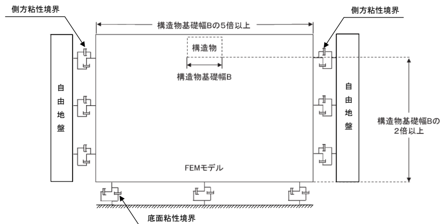
図 4.1.7-14 地震応答解析における境界条件の概念図
