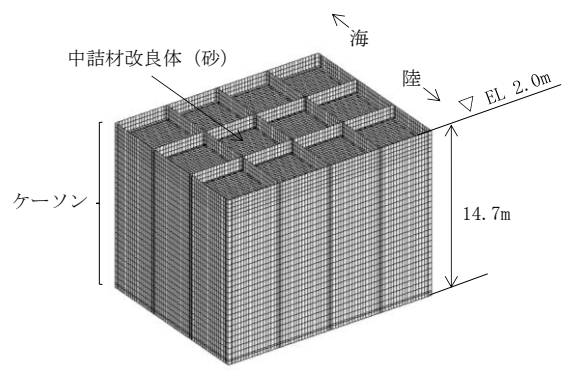
ケーソンのモデル図 (陸側) *
