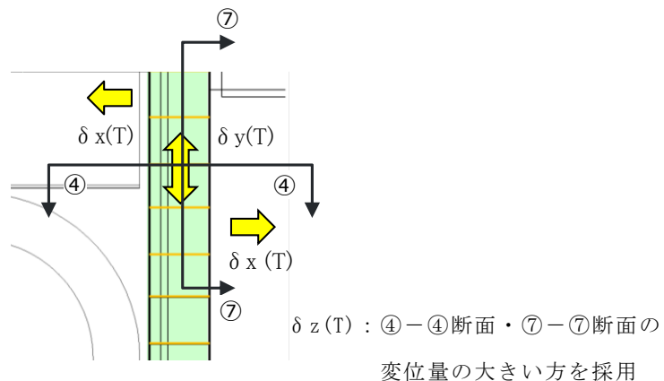
図 4.1.8-6 地震時の変位量の概念図
