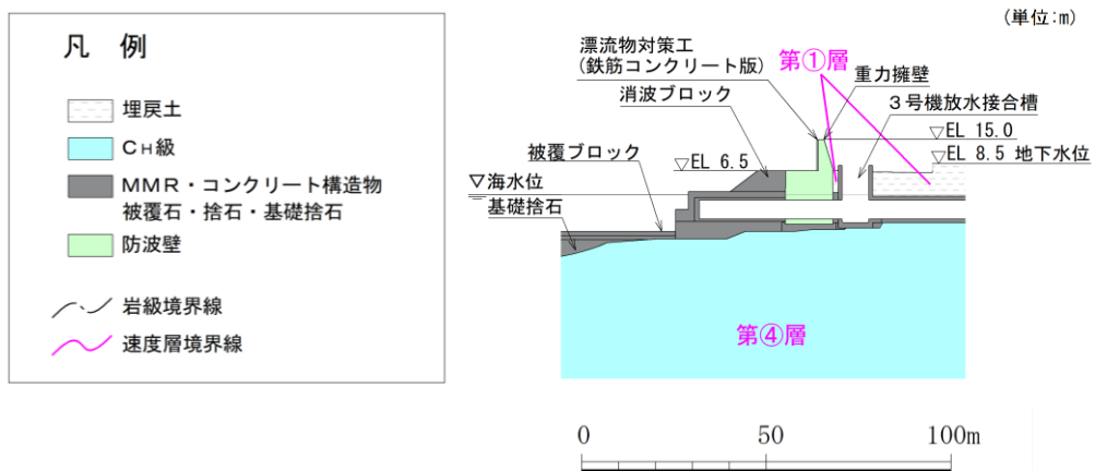
図 4.1.7-5 地質断面図 (③-③断面)
