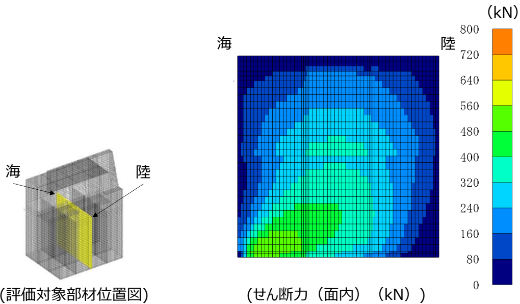
図 5.2.7-1(2) コンクリートのせん断破壊（面内）に対する照査に用いる断面力図 (④－④断面, S_s - N1(-+) , 解析ケース②, 評価対象部材：隔壁④) 解析ケース②：地盤物性のばらつきを考慮した解析ケース（平均値+ 1\sigma ）
