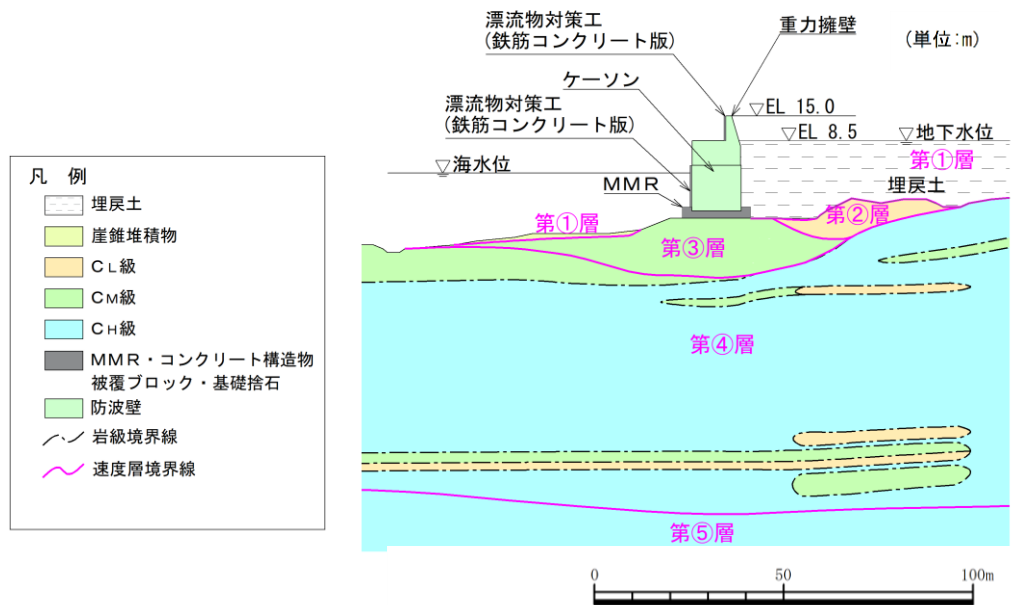
図 4.1.7-7 地質断面図 (④-④断面)
