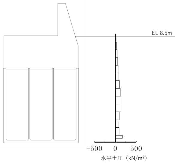
水平土圧
