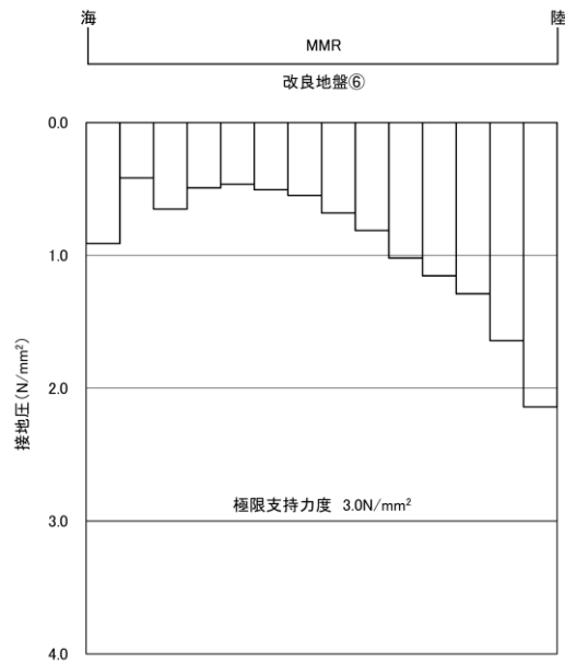
図 4.2.11-1(2) 支持地盤の接地圧分布図 (②-②断面, 改良地盤⑥) (S s - D (++) )
