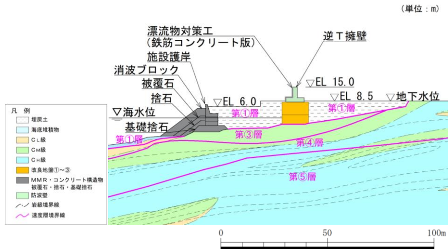
図 3.5.2-3 地質断面図 (①-①断面)
