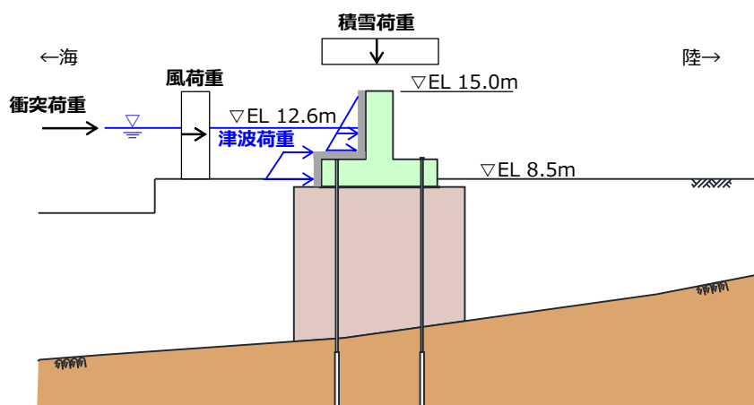
図 3.3.2-1 防波壁（逆 T 擁壁）の荷重作用図
