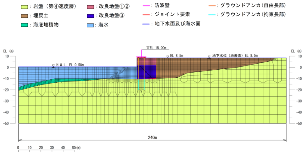
図 5.6.2-1 ⑤-⑤断面における施設護岸等が損傷した場合の解析モデル
