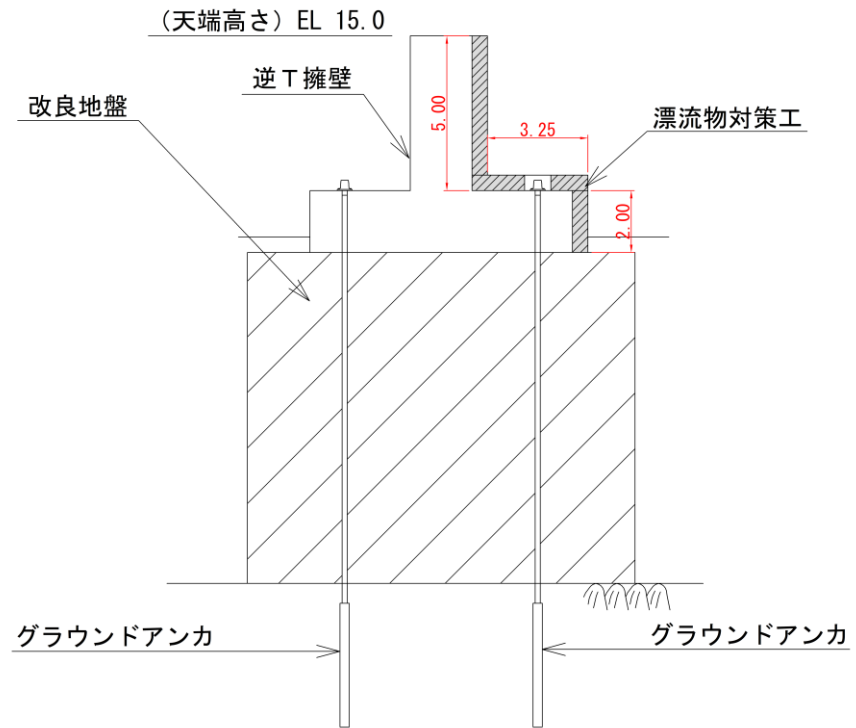
図 5.2.2-1 漂流物対策工 (0.5m 幅) 設置図
