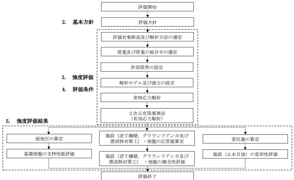
図 2.3-1 防波壁（逆 T 擁壁）の強度評価の検討フロー
