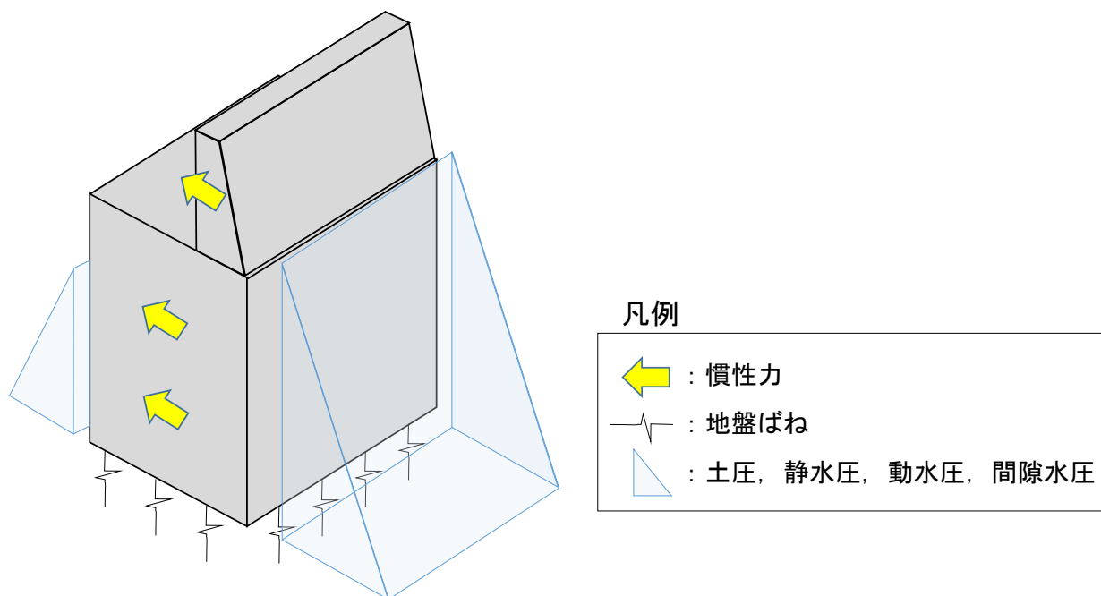
図 5.1.3-1(1) 3次元構造解析への入力イメージ
