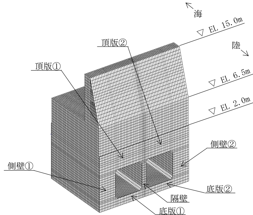
図 5.2.4-2 評価対象部材位置図 (③-③断面)
