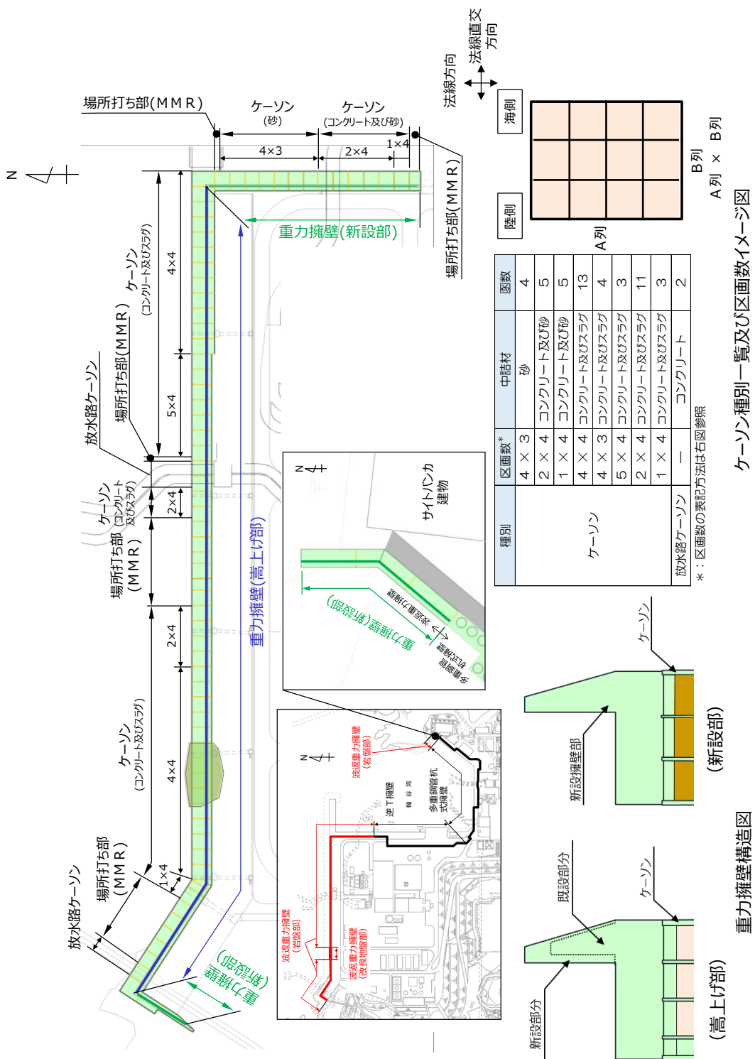
図 3.1-11 防波壁（波返重力擁壁）における重力擁壁及びケーンの構造種別
