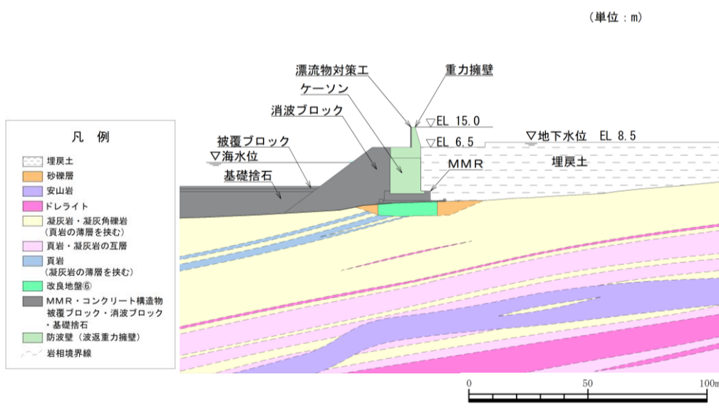
図 6.1.1-2 改良地盤⑥の配置図（②-②断面）
