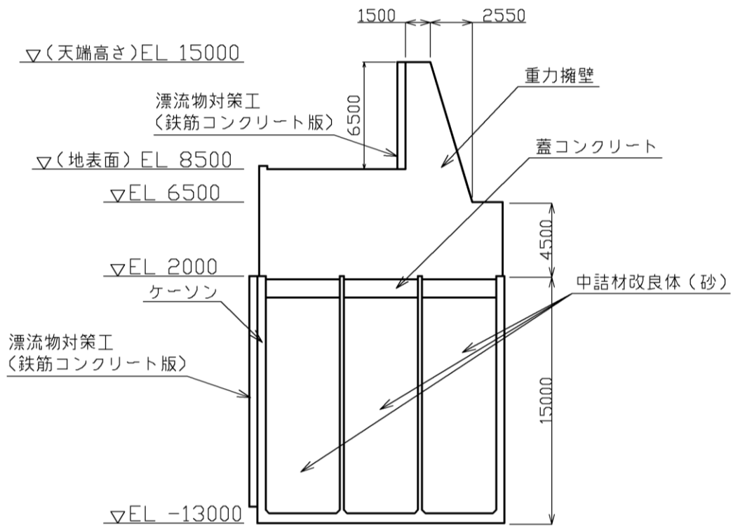
(断面図)
