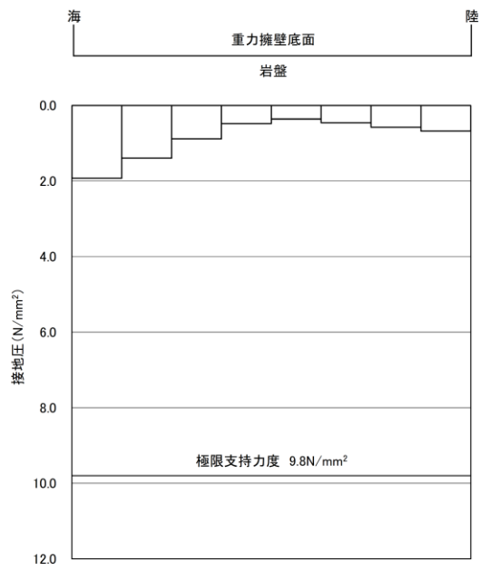
図 4.2.11-4 支持地盤の接地圧分布図 (⑤-⑤断面, 岩盤) (S s -N2 (EW) (-+)) 解析ケース①: 基本ケース
