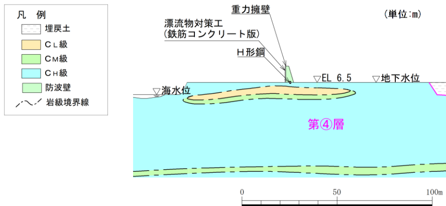
図 3.1-8 防波壁（波返重力擁壁）の横断面図（⑥-⑥断面）
