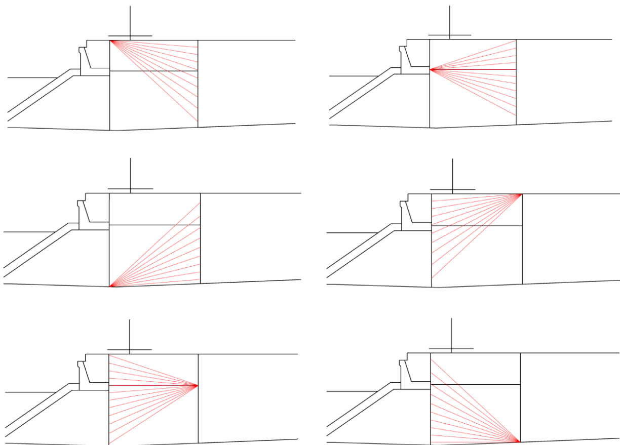
図 3.5.3-5(3) 改良地盤の想定すべり線 (⑤-⑤断面)
