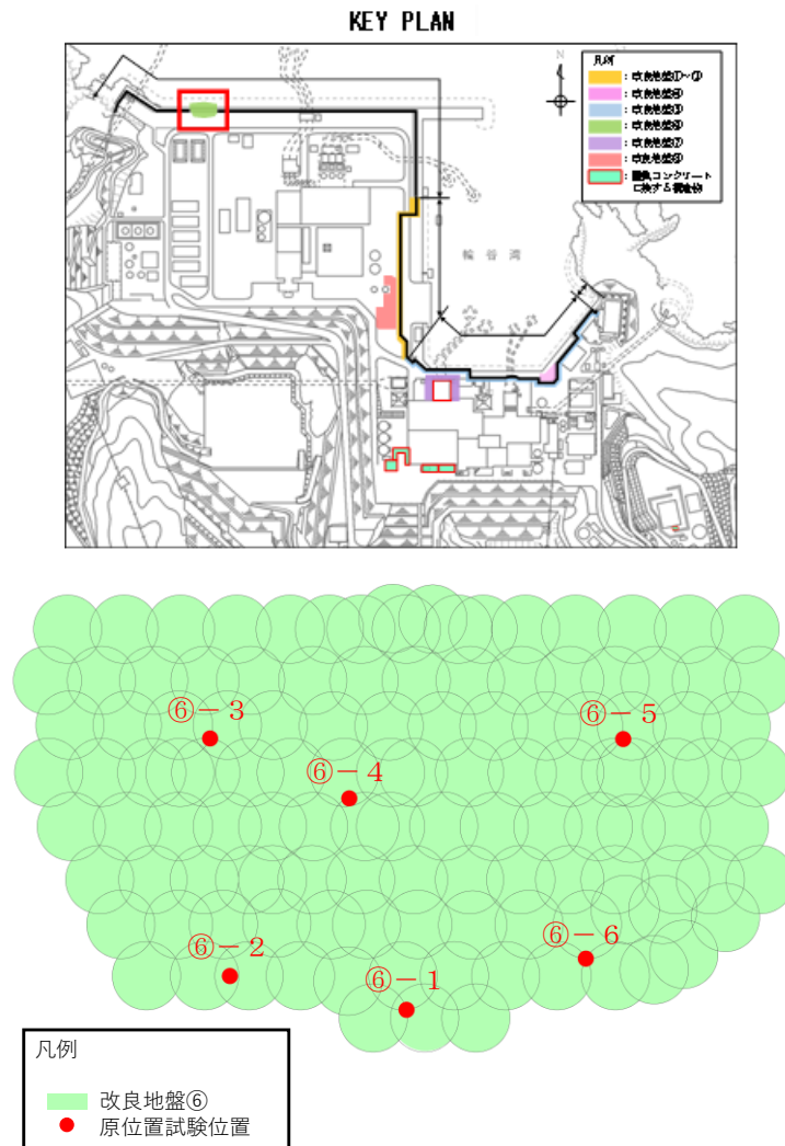
図 6.1.1-4 改良地盤⑥の原位置試験位置図
