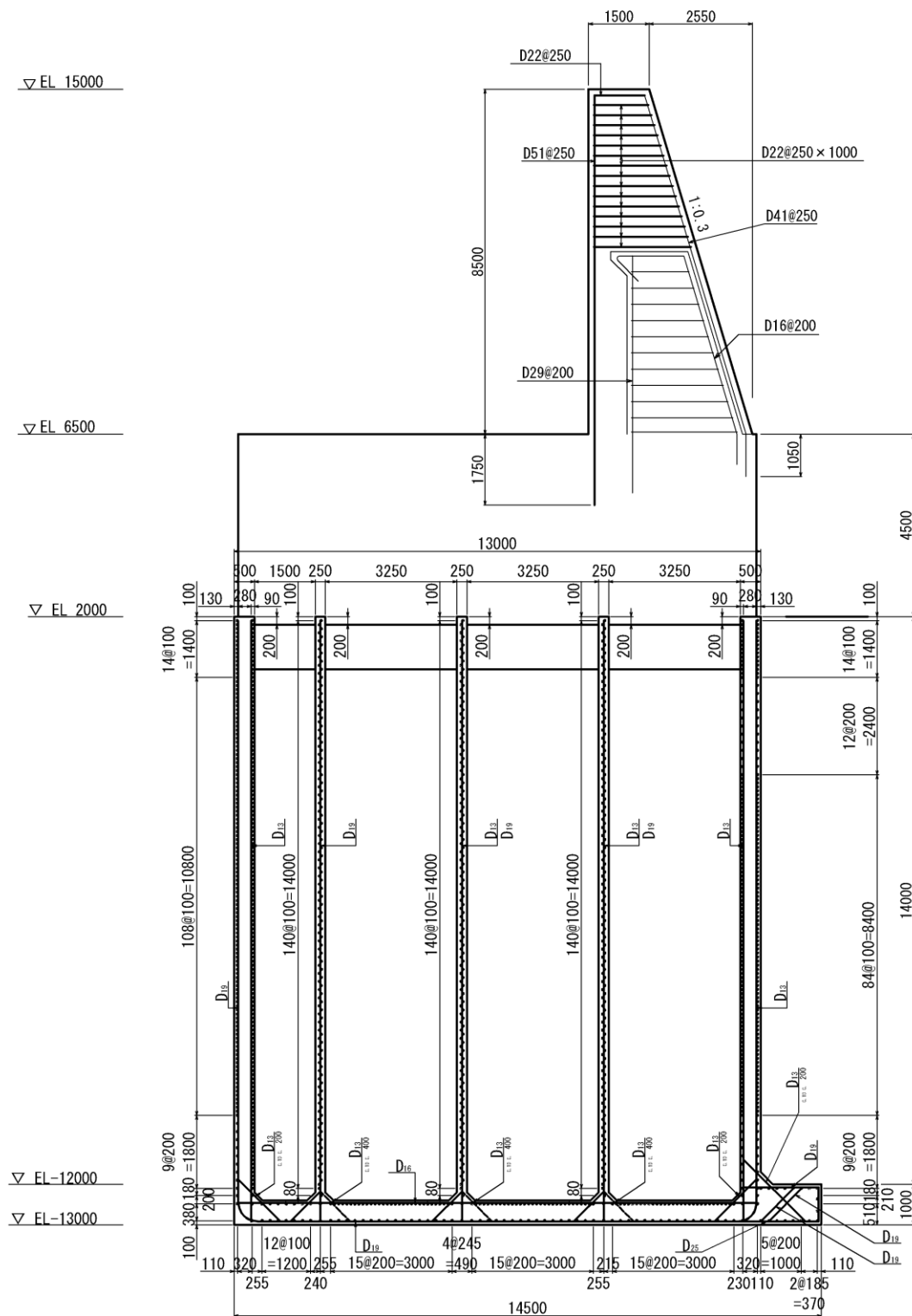
図 3.1-10(1) 防波壁（波返重力擁壁）の重力擁壁及びゲートソンの概略配筋図 (②-②断面)
