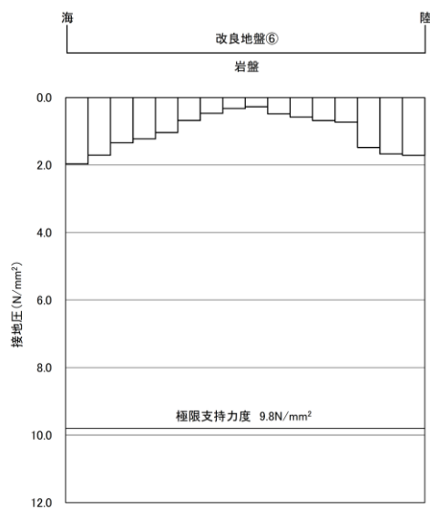
図 4.2.11-1(3) 支持地盤の接地圧分布図 (②-②断面, 岩盤) (S s - D (--) )
