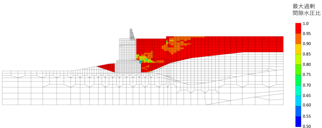
図 4.2.4-1(3) ②-②断面の過剰間隙水圧比最大値分布 (解析ケース①, S_s - D(-+) )
