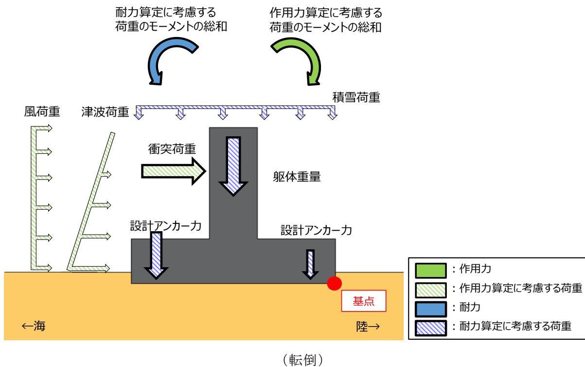
図 5.2.2-2 逆T擁壁に作用する荷重イメージ
