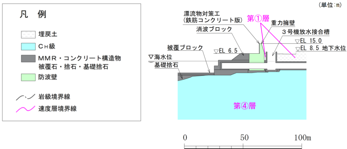
図 3.1-5 防波壁 (波返重力擁壁) の横断面図 (③-③断面)
