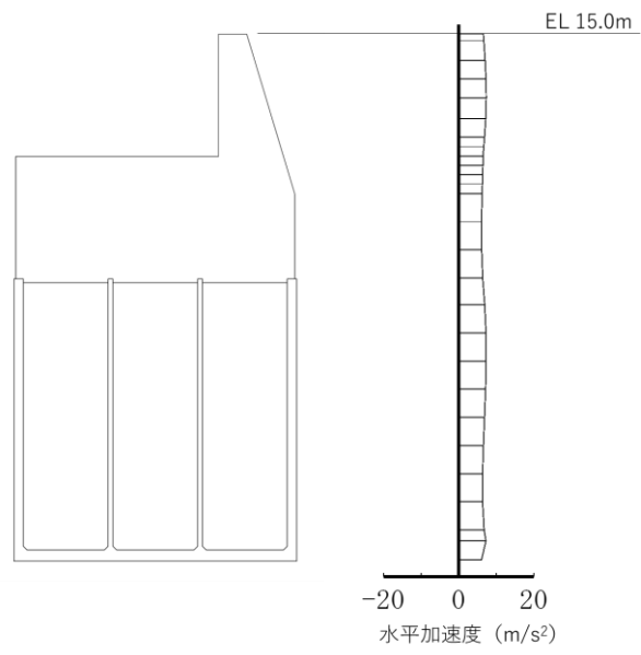
水平加速度
