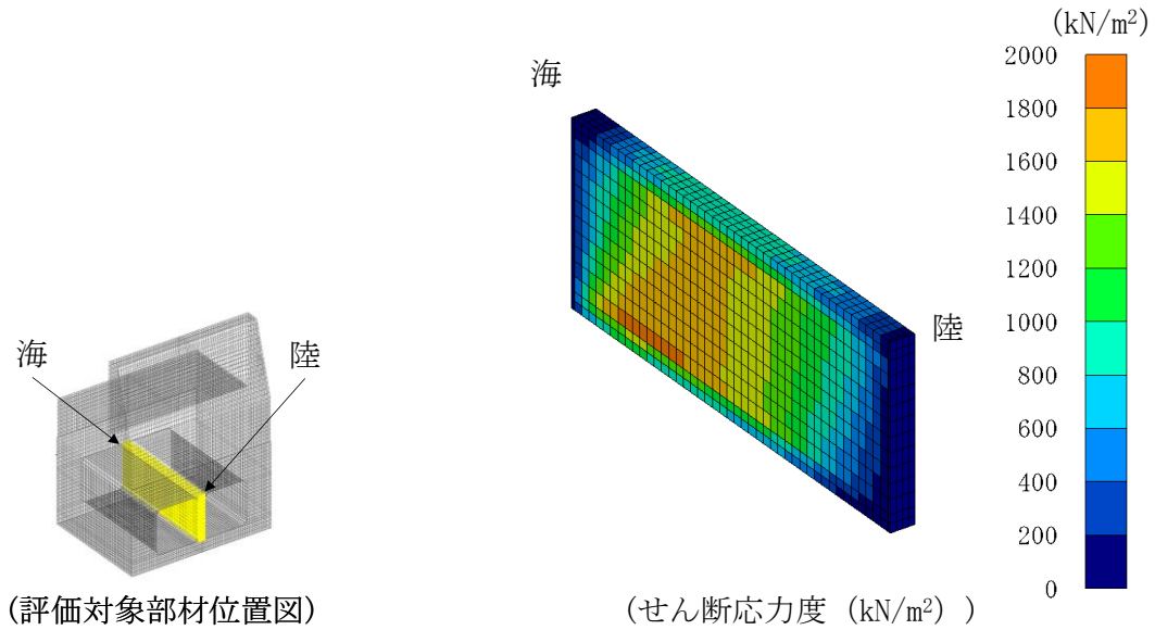
図 5.2.11-1 コンクリートのせん断破壊（面内）に対する照査に用いる断面力分布
