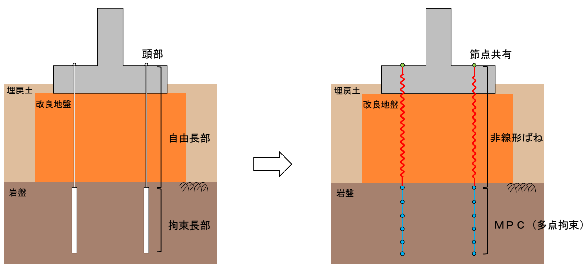
図 3.5.2-14 モデル化概念図
