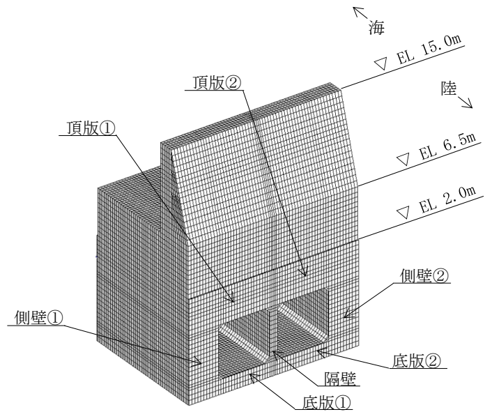
図 5.2.1-1(2) 放水路ケースンの構造部材 (③-③断面)
