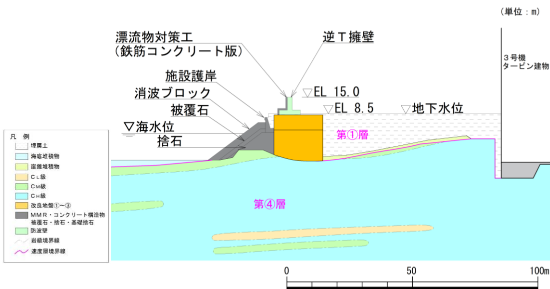
図 3.2.1-8 防波壁（逆T擁壁）の横断面図（⑤-⑤断面）
