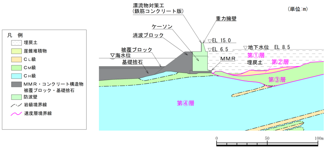
図 3.1-3 防波壁（波返重力擁壁）の横断面図（①-①断面）
