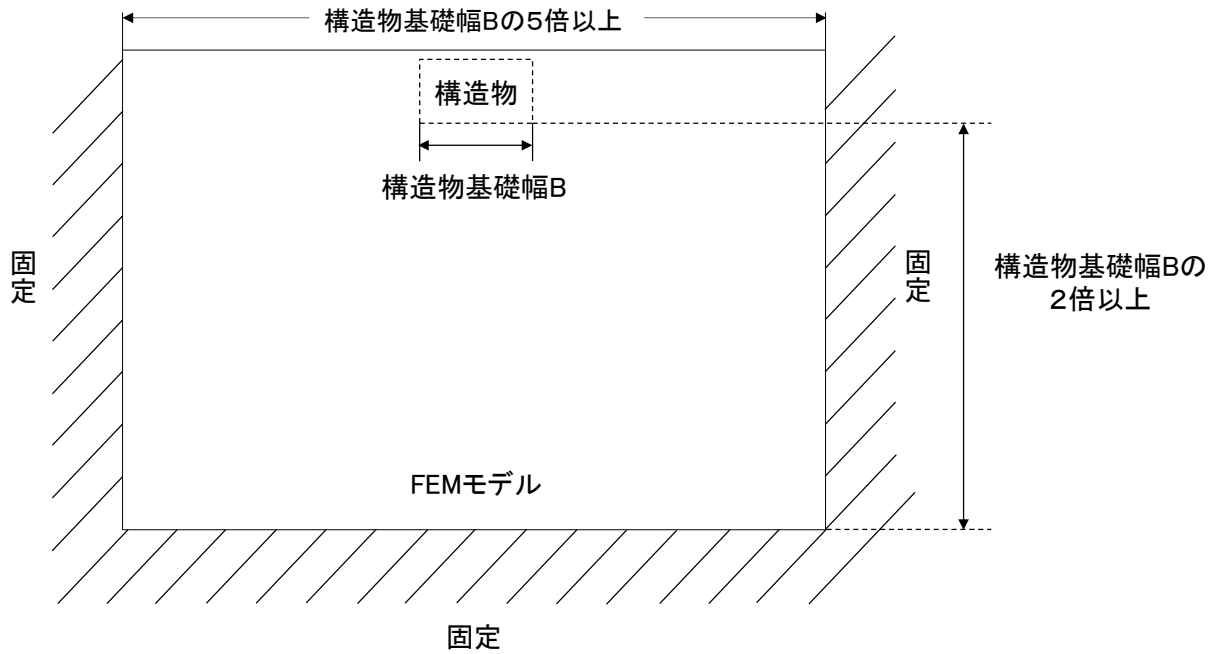
図 3.5.2-9 津波時の2次元有限要素法における境界条件の概念図
