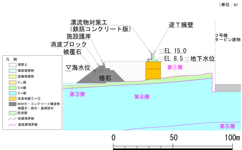
図 3.5.2-5 地質断面図 (④-④断面)
