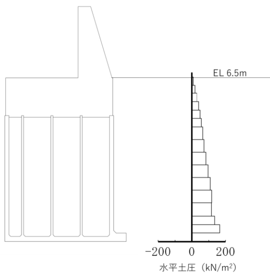
水平土圧
