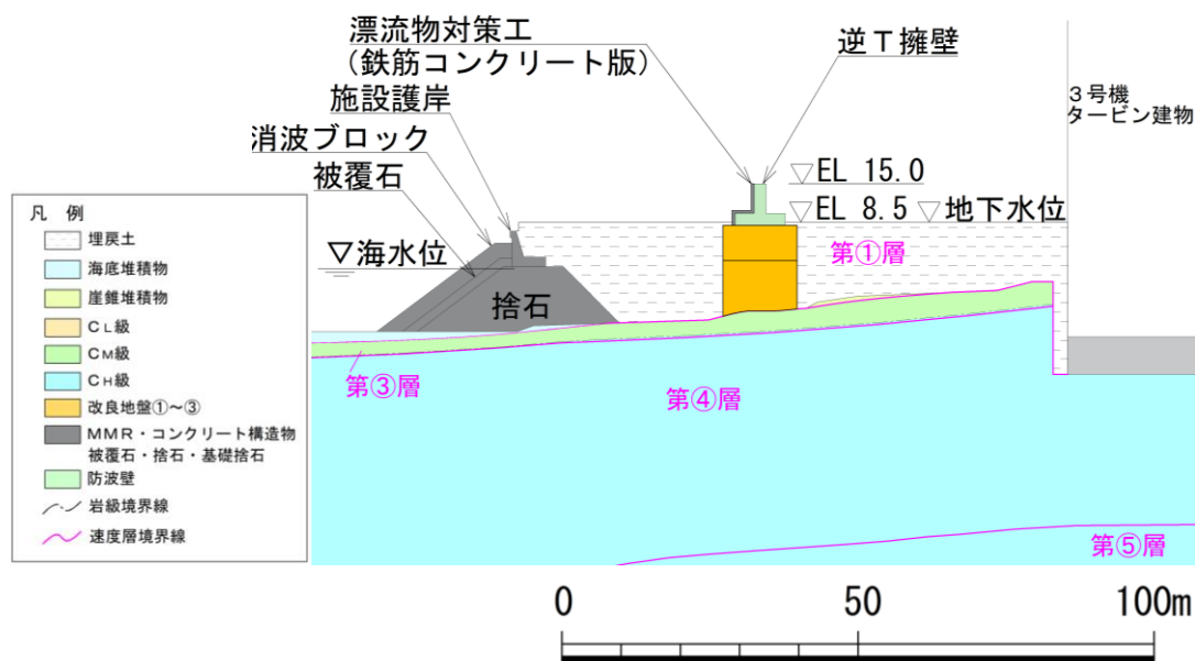
図 3.2.1-7 防波壁（逆T擁壁）の横断面図（④-④断面）
