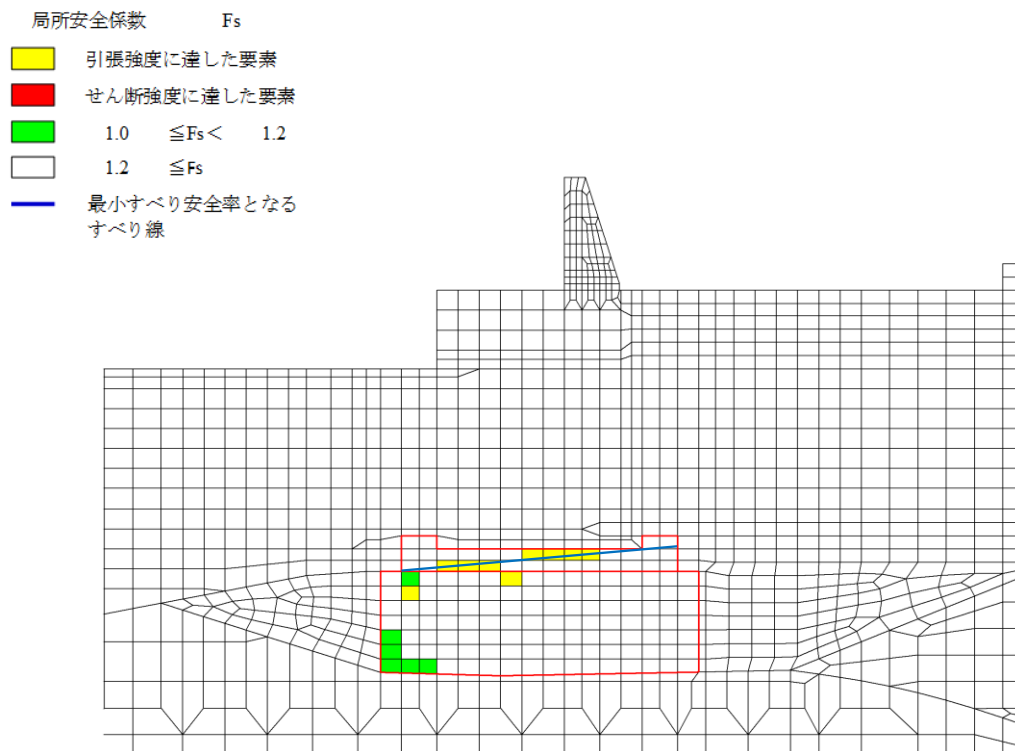
図 4.2.8-1(1) MMR の最小すべり安全率時刻におけるすべり線及び局所安全係数分布図
