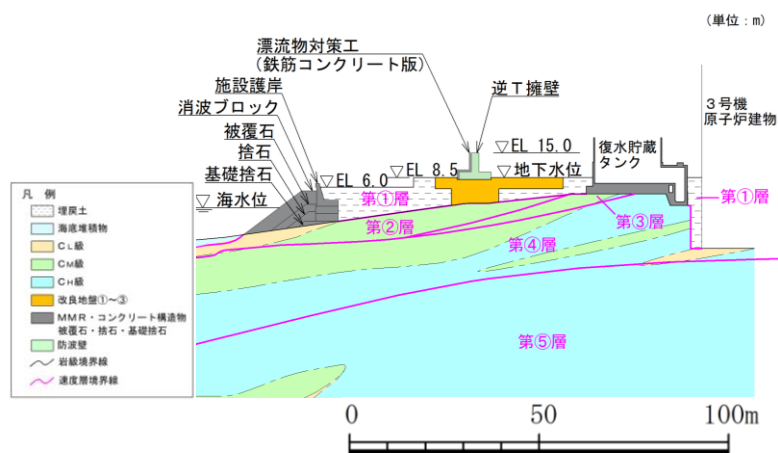
図 3.2.1-6 防波壁 (逆T擁壁) の横断面図 (③-③断面)
