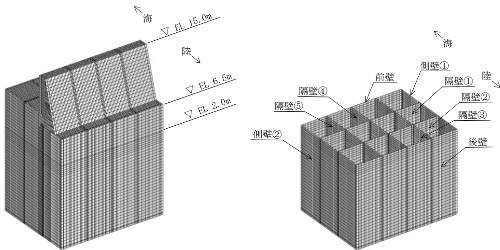
図 5.2.1-1(3) ケースンの構造部材 (④-④断面)
