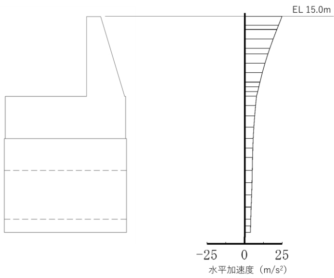
水平加速度
