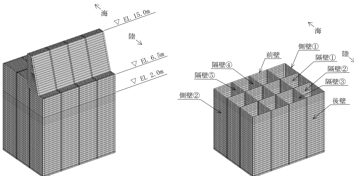
図 5.2.4-1(2) 評価対象部材位置図 (④-④断面)
