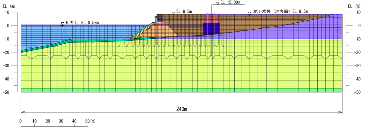
図 3.5.2-4 解析モデル (④-④断面)
