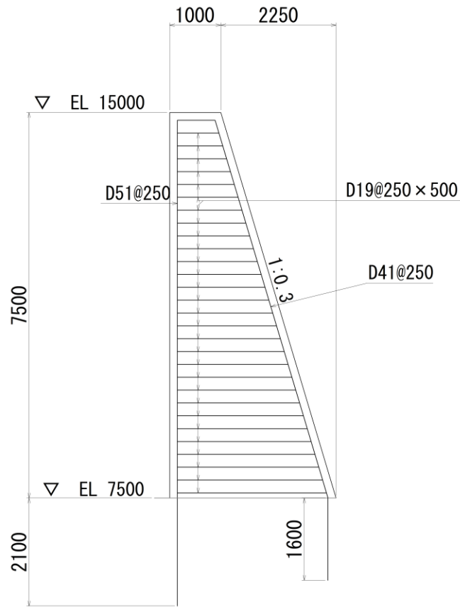
図 3.1-10(5) 防波壁（波返重力擁壁）の重力擁壁の概略配筋図（⑤-⑤断面）
