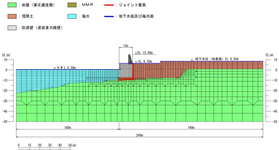
図 4.1.7-4 地震応答解析モデル (③-③断面)
