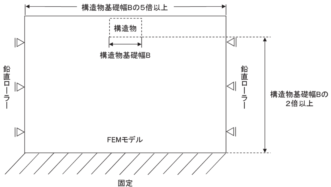
図 3.5.2-8 常時応力解析における境界条件の概念図
