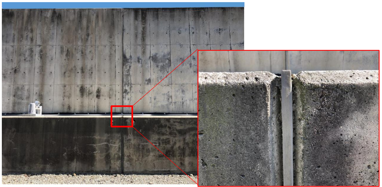
図 2.2-5 目地材写真（樹脂発泡体目地材，厚さ 20mm）
