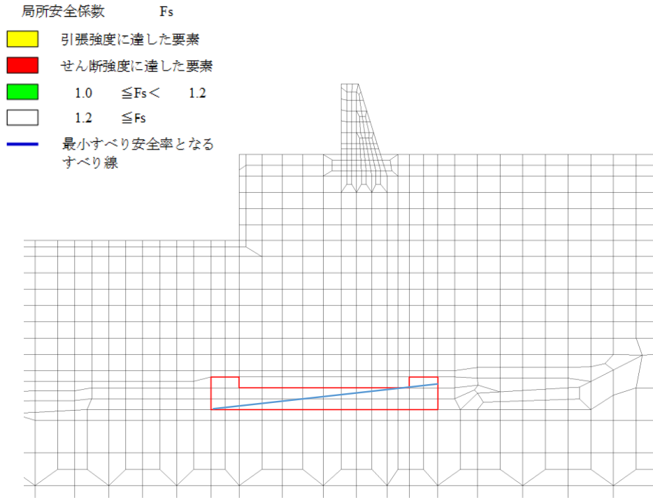
図 4.2.8-1(3) MMR の最小すべり安全率時刻におけるすべり線及び局所安全係数 分布図
