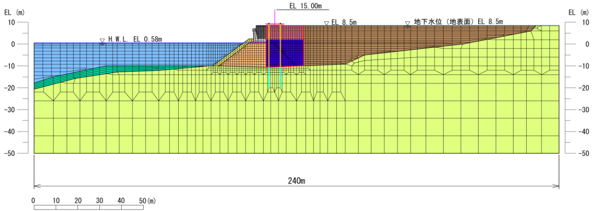
図 3.5.2-6 解析モデル (⑤-⑤断面)
