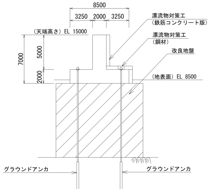
図 2.2-4 防波壁 (逆 T 擁壁) の構造図 (断面図)
