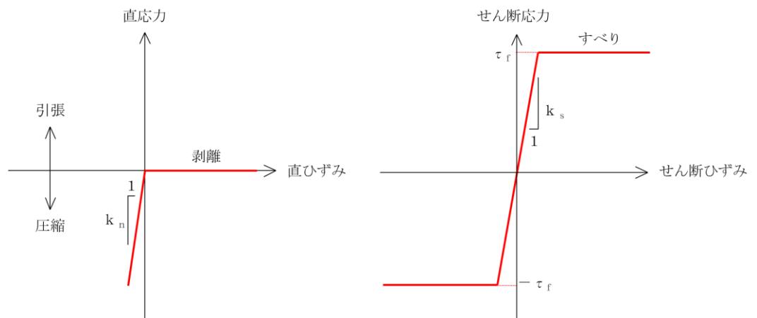
図 3.5.2-23 ジョイント要素の力学特性
