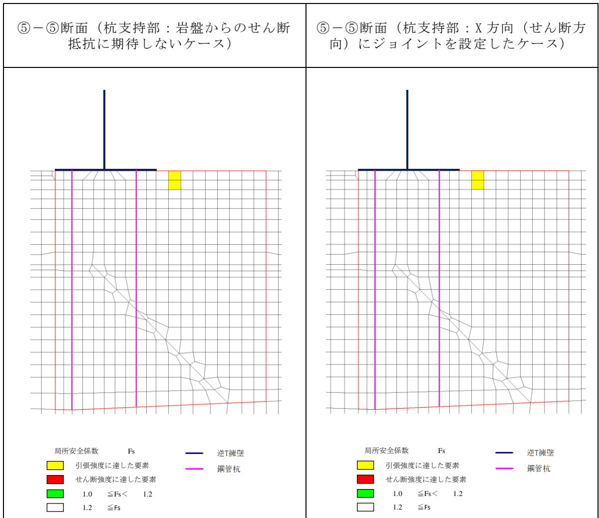
図 6.1.2-1 鋼管杭をモデル化した改良地盤の局所安全係数分布
