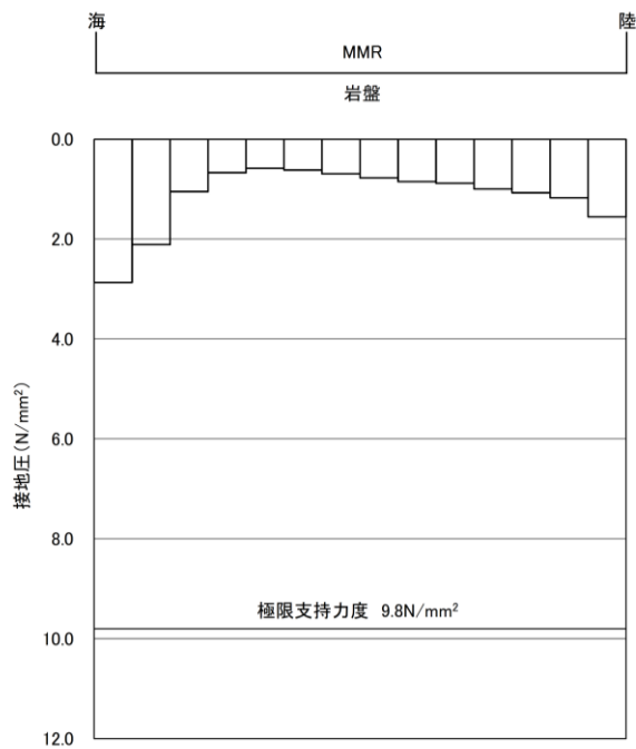
図 4.2.11-3(2) 支持地盤の接地圧分布図 (④-④断面, 岩盤) ( S_s - D(-) )
