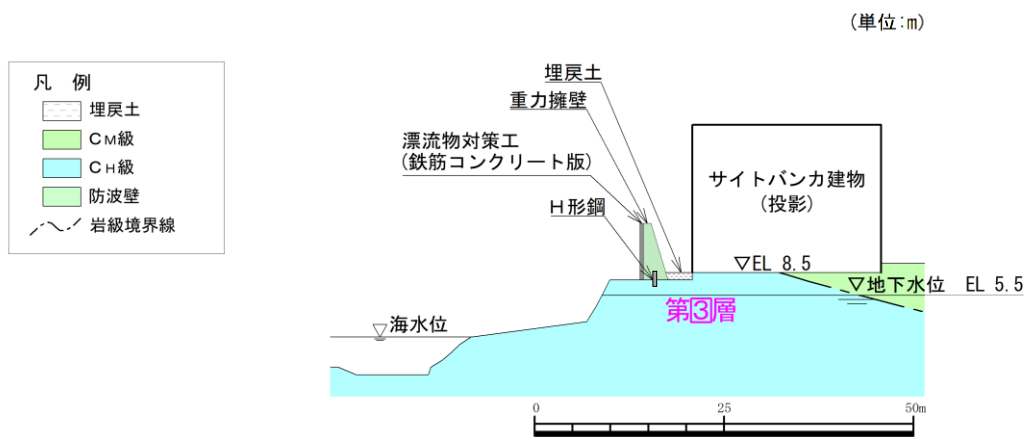
図 4.1.7-9 地質断面図 (⑤-⑤断面)
