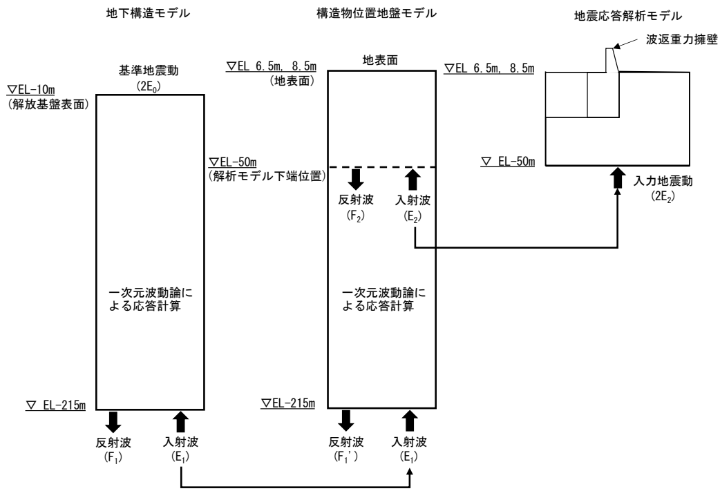
図 4.1.6-1 入力地震動算定の概念図
