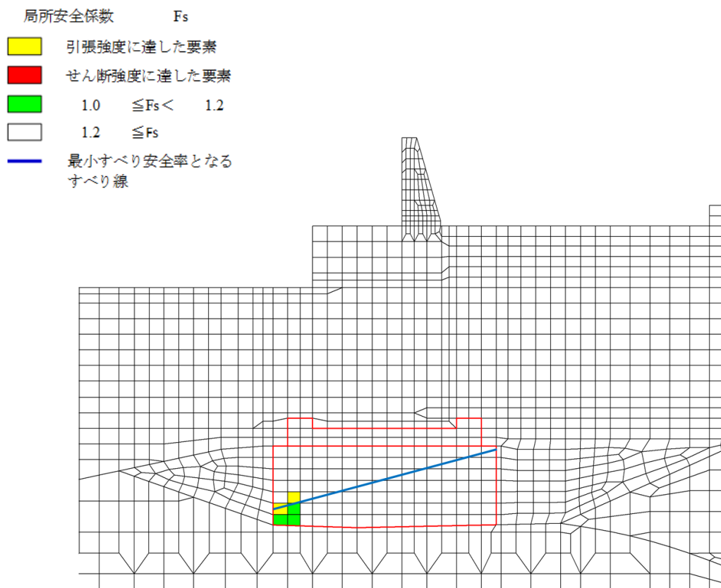
図 4.2.9-1 改良地盤⑥の最小すべり安全率時刻におけるすべり線 及び局所安全係数分布 (②-②断面, S s - D (---), t = 10.26 s, 解析ケース①)
