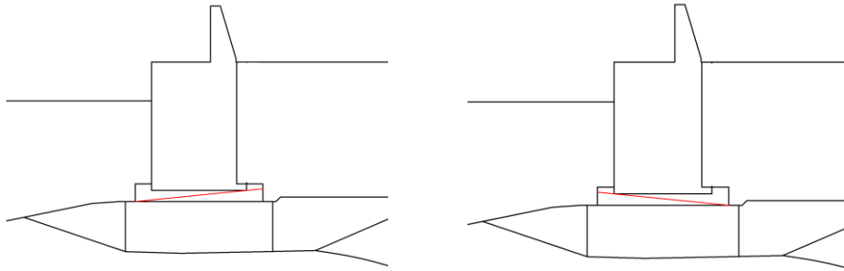
図 4.1.8-4(1) MMR の想定すべり線 (②-②断面)
