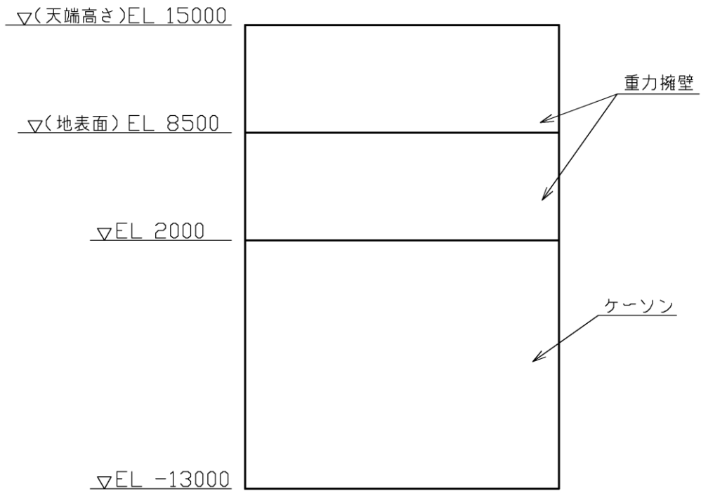
(正面図)
