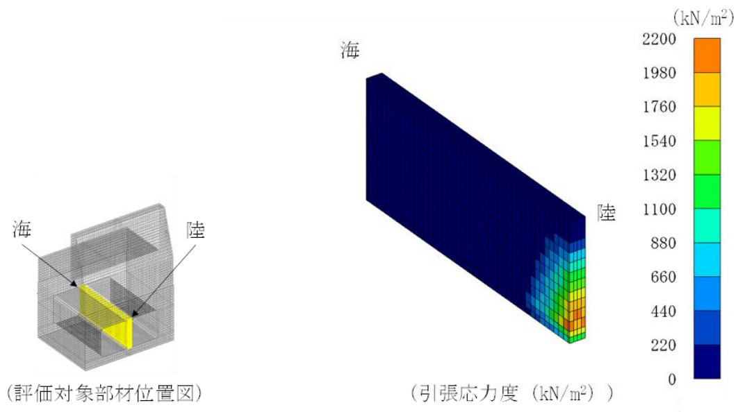
図 5.2.9-1 コンクリートの引張破壊に対する照査に用いる断面力図 （③-③断面， S_s - N1(-+) ，評価対象部材：隔壁） 解析ケース①：基本ケース
