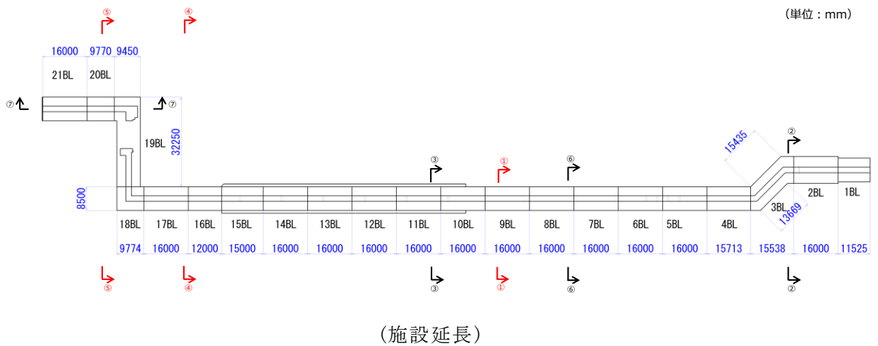
図 3.2.1-2 防波壁（逆T擁壁）の施設延長
