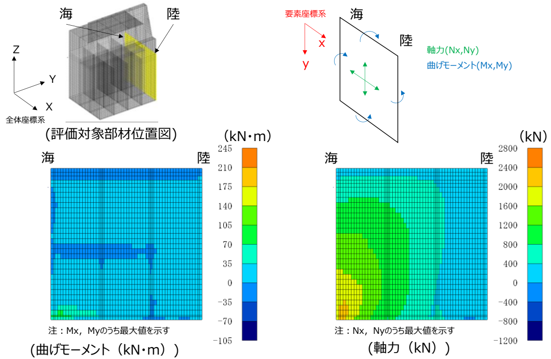
図 5.2.5-1(2) コンクリートの曲げ圧縮応力に対する照査に用いる断面力図
