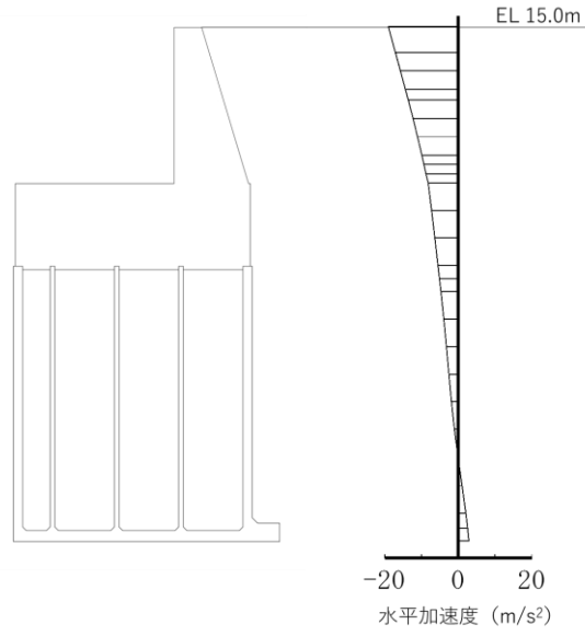
水平加速度
