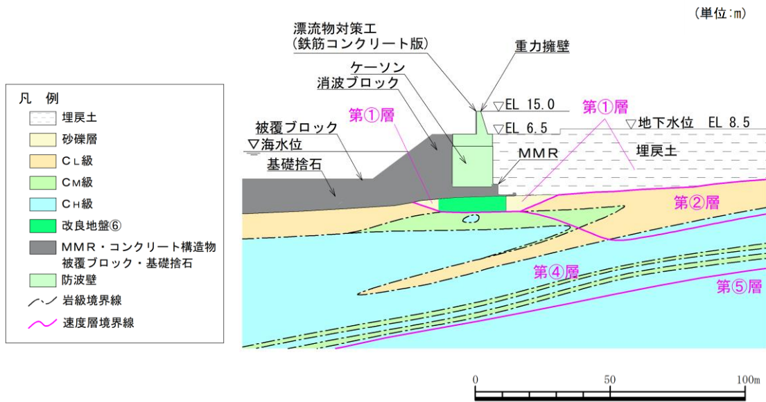
図 3.1-4 防波壁（波返重力擁壁）の横断面図（②-②断面）
