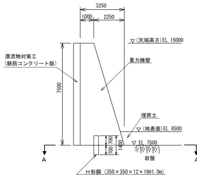
(断面図)
