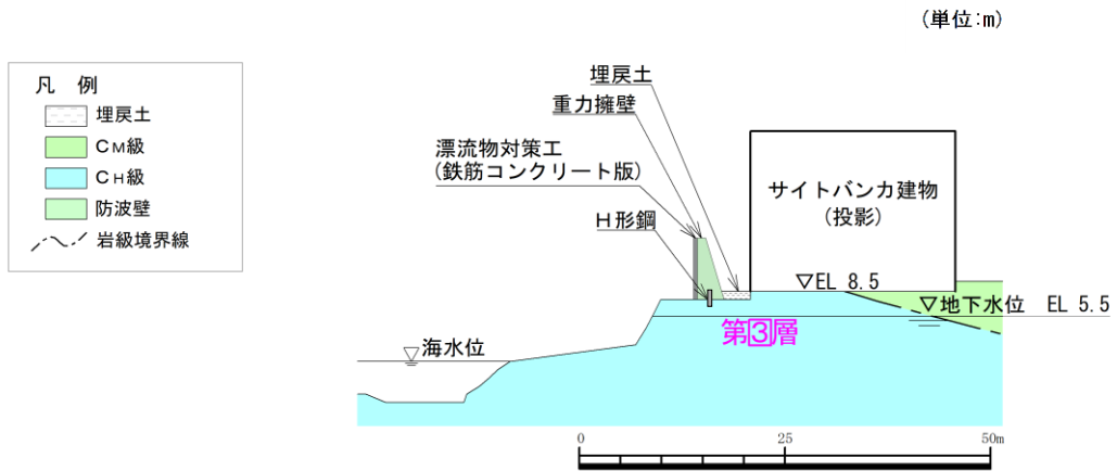
図 3.1-7 防波壁（波返重力擁壁）の横断面図（⑤-⑤断面）
