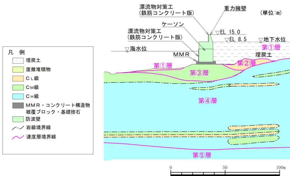
図 3.1-6 防波壁 (波返重力擁壁) の横断面図 (④-④断面)
