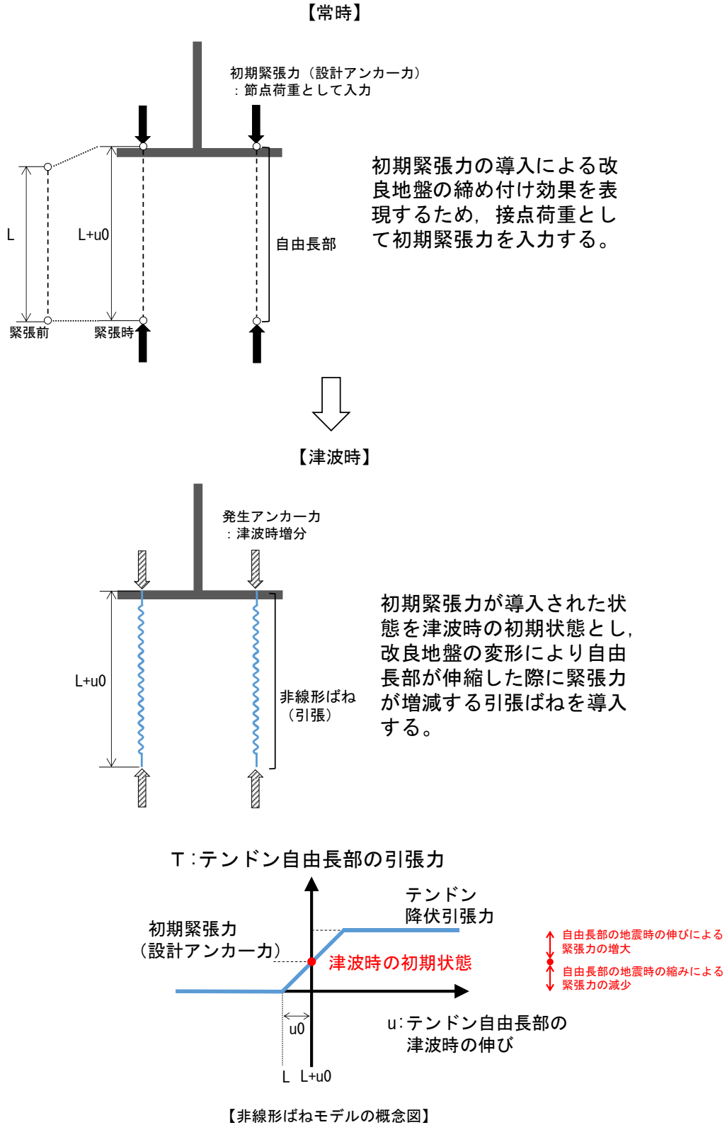
図 3.5.2-15 モデル化したグラウンドアンカの緊張力
