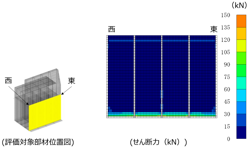
図 5.2.6-1(1) コンクリートのせん断破壊 (面外) に対する照査に用いる断面力図 (②-②断面, S_s - N1 (+ +) , 評価対象部材: 後壁) 解析ケース②: 地盤物性のばらつきを考慮した解析ケース (平均値+ 1\sigma )
