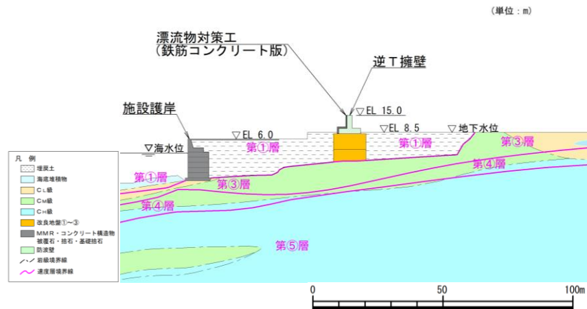
図 3.2.1-9 防波壁（逆 T 擁壁）の横断面図（⑥-⑥断面）
