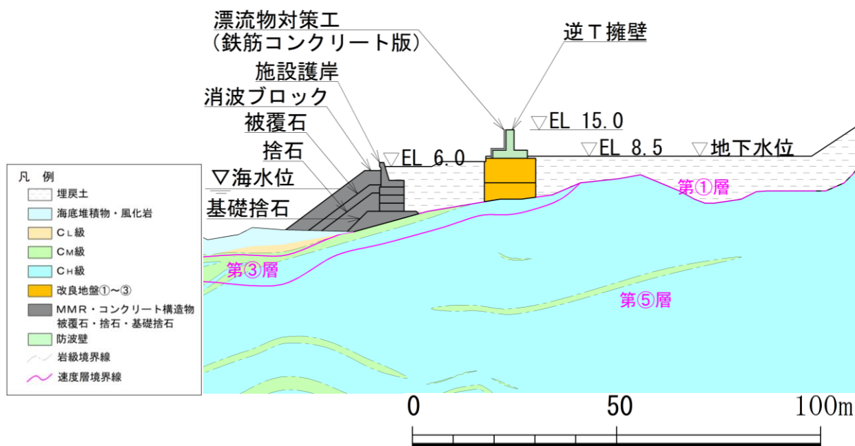
図 3.2.1-5 防波壁 (逆T擁壁) の横断面図 (②-②断面)
