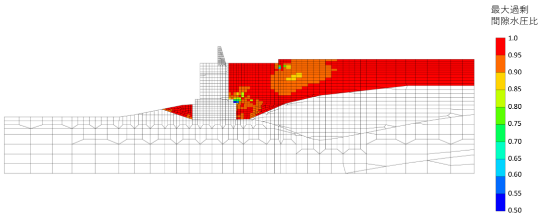
図 4.2.4-1(2) ②-②断面の過剰間隙水圧比最大値分布 (解析ケース②, S_s - D(++) )
