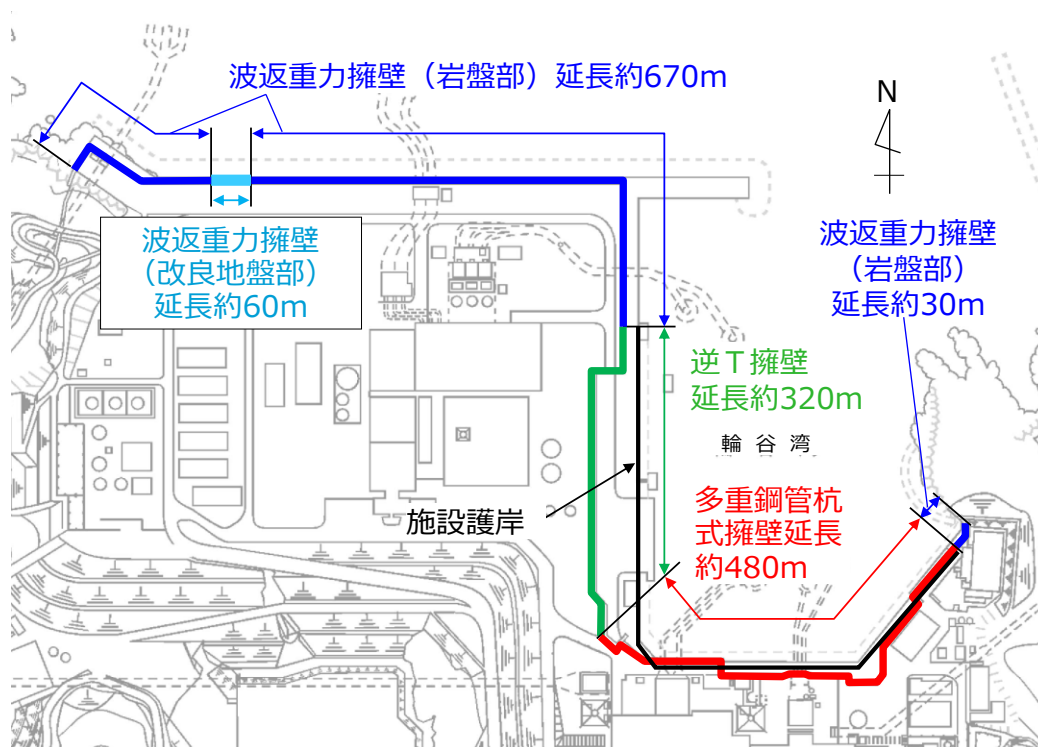
図 5.6.1-1 防波壁と施設護岸の配置（全体平面図）
