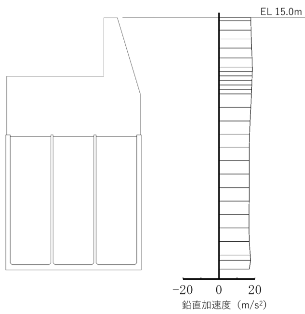
鉛直加速度
