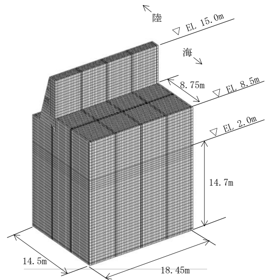
モデル全体図 (海側)
