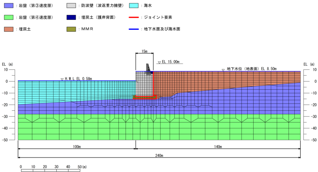
図 4.1.7-6 地震応答解析モデル (④-④断面)
