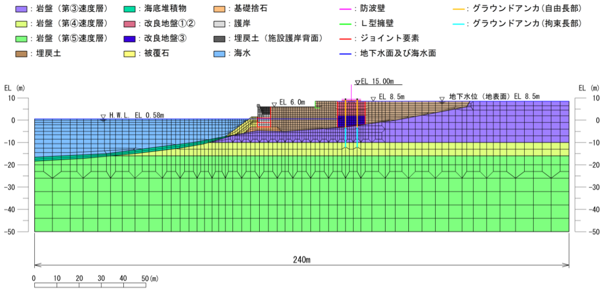
図 3.5.2-2 解析モデル (①-①断面)
