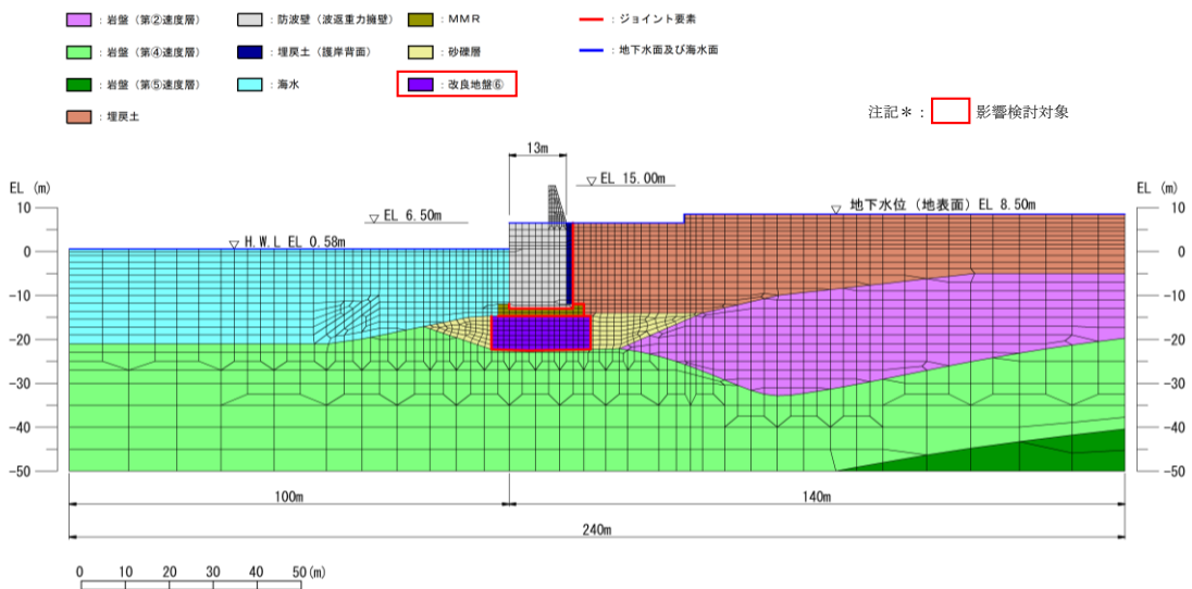
図 6.1.2-1 地震応答解析モデル（②-②断面）
