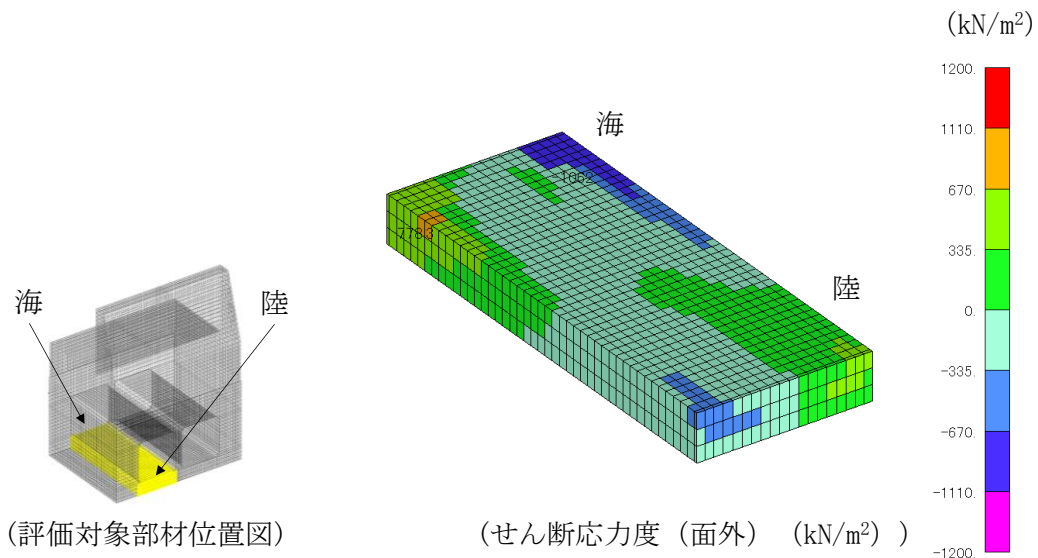
図 5.2.10-1 コンクリートのせん断破壊（面外）に対する照査に用いる断面力分布 （③－③断面， S_s - N_1 (-+) ，評価対象部材：底版①） 解析ケース③：地盤物性のばらつきを考慮した解析ケース（平均値 -1\sigma ）
