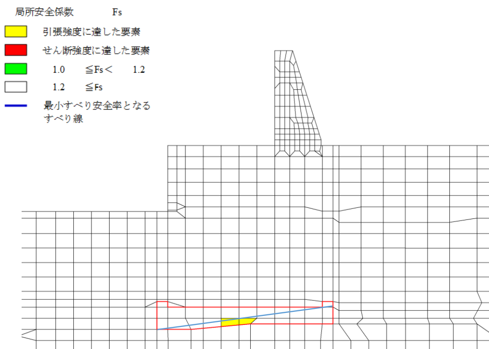
図 4.2.8-1(2) MMR の最小すべり安全率時刻におけるすべり線及び局所安全係数分布図
