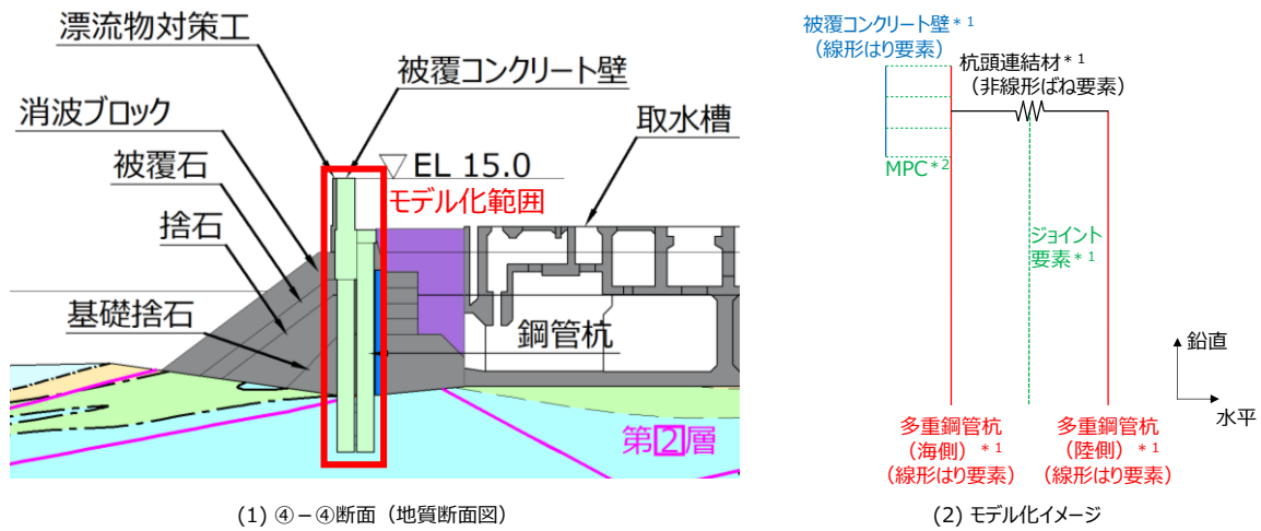
(1) ④-④断面 (地質断面図)
