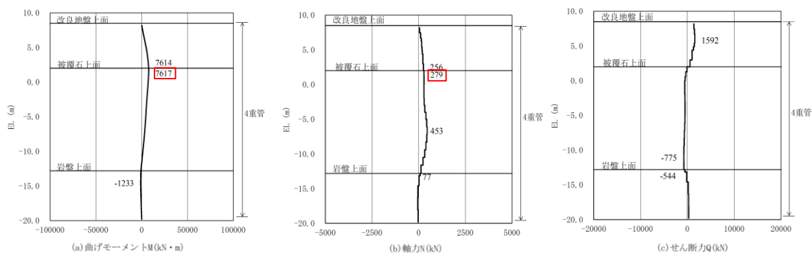
図 2.2.2-8 鋼管杭の曲げ・軸力系の破壊に対する照査における断面力図
