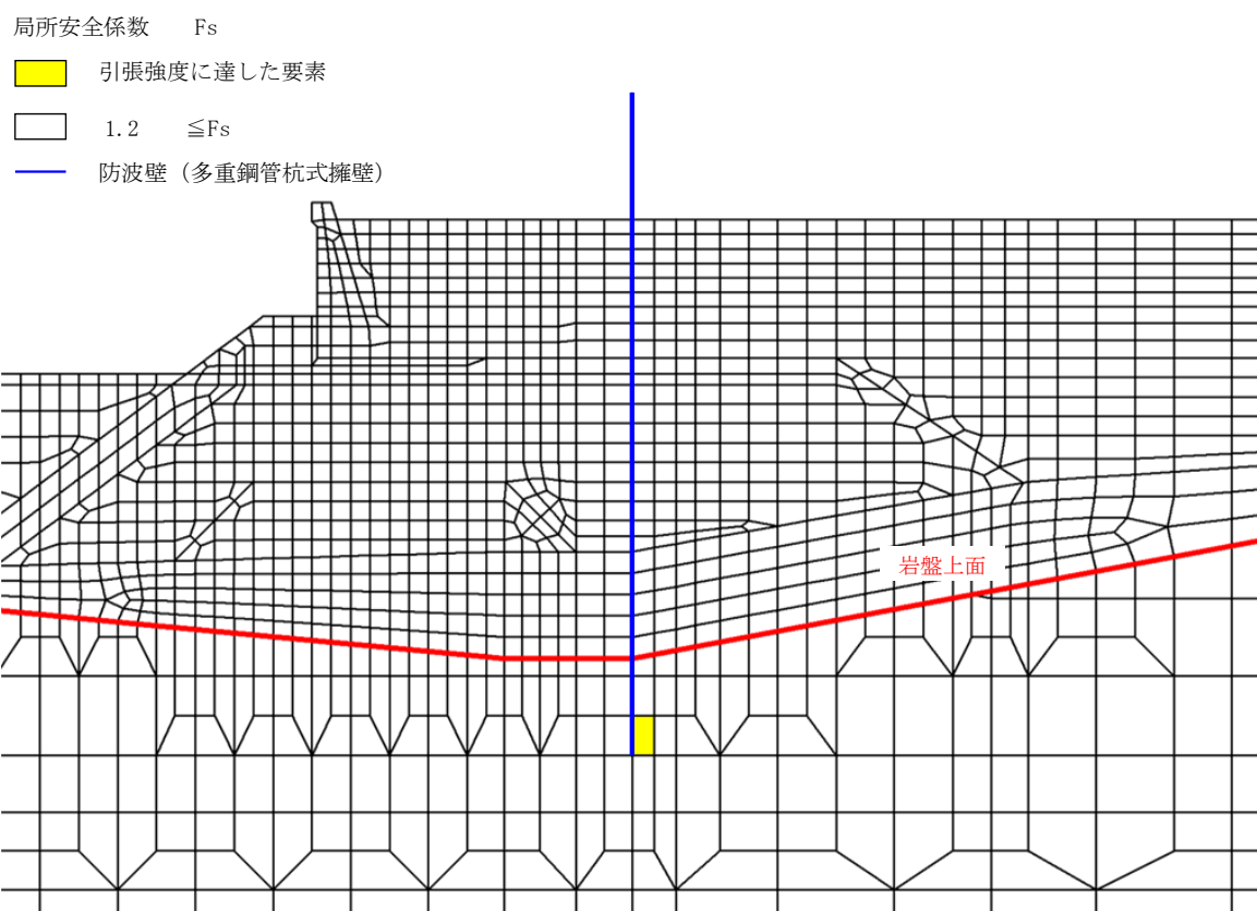
図 4.3.1-3 鋼管杭周辺岩盤の局所安全係数分布図 (②-②断面)
