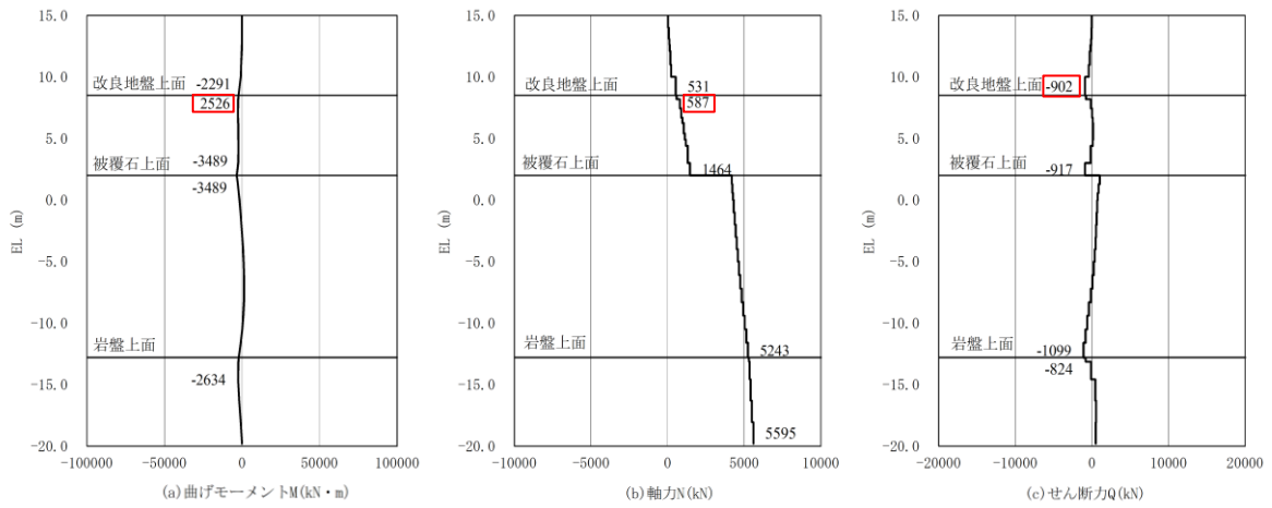
(㊦-㊦断面, 海側杭)
