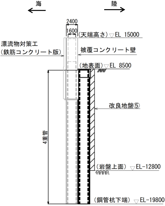
（断面図）
