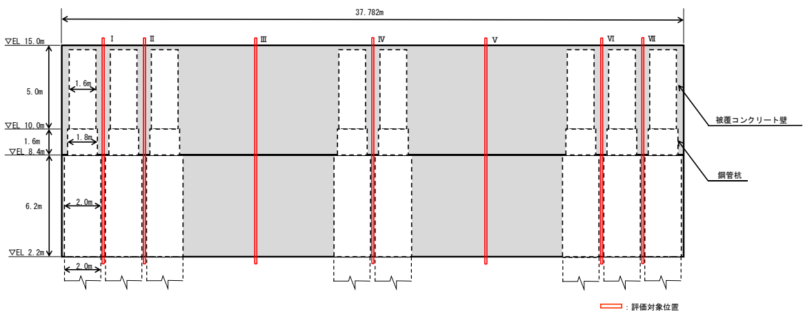
(④-④断面)
