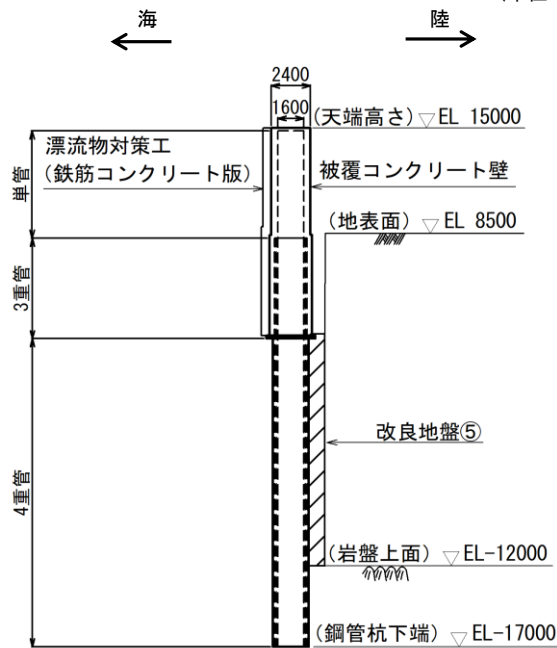
(断面図)
