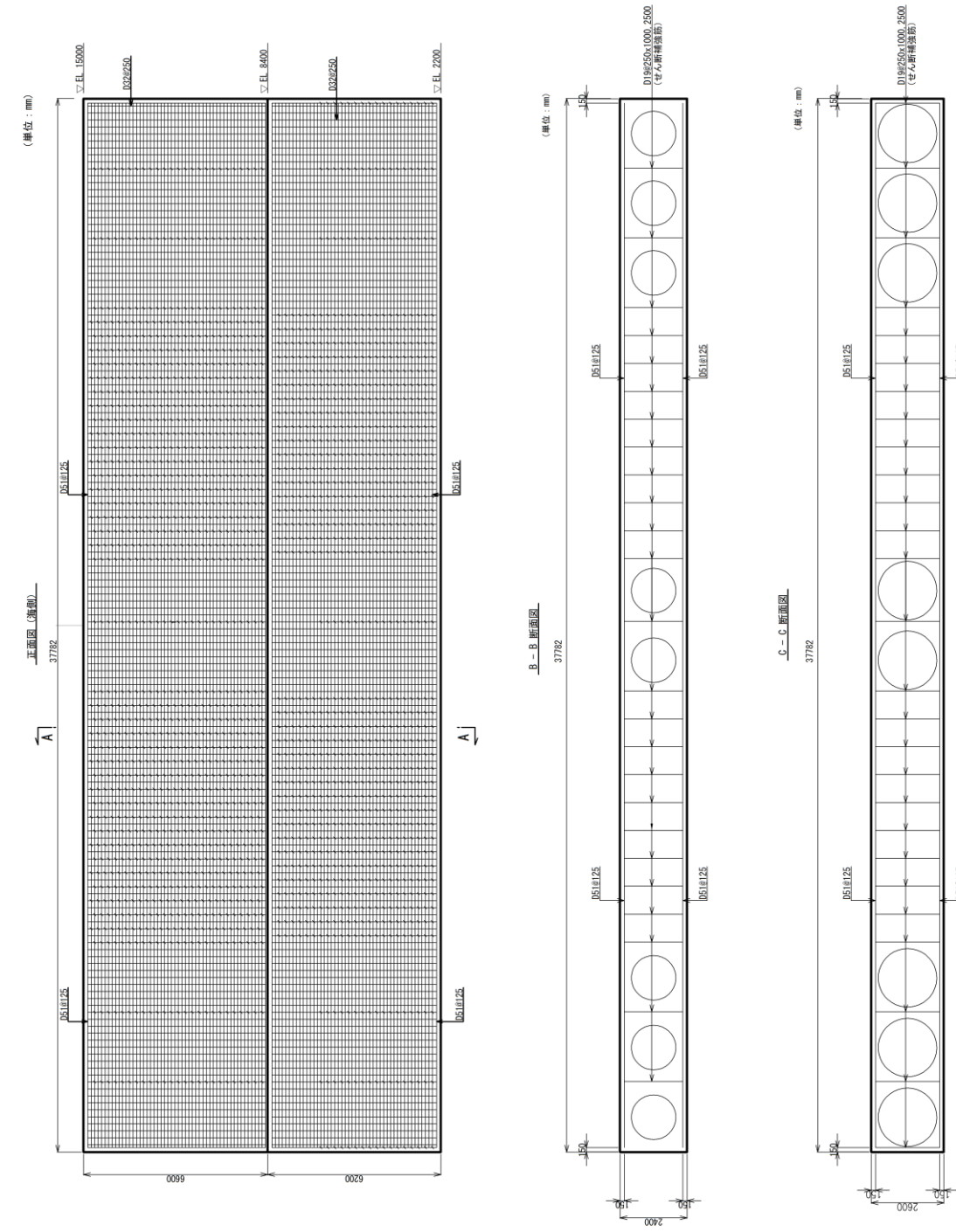
図 3.2.1-15 防波壁 (多重鋼管杭式擁壁) の被覆コンクリート壁の概略配筋図 (④-④断面)
