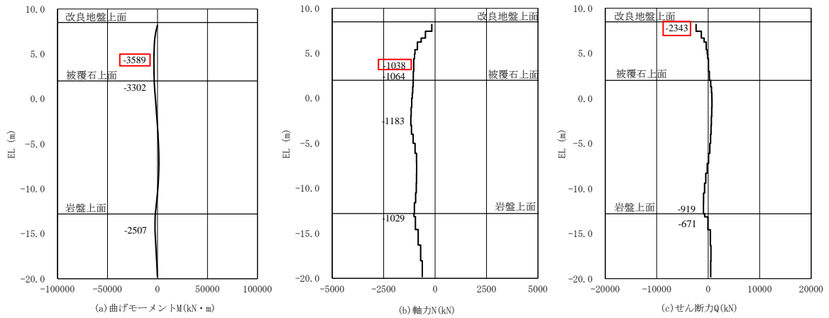
(㊦-㊦断面, 陸側杭)
