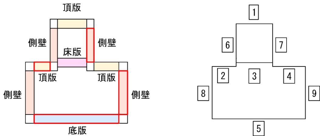
(B-B断面)
