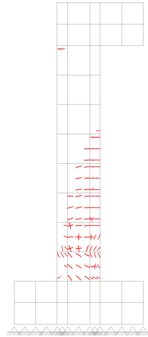
187 ステップ 斜めひび割れ進行時
