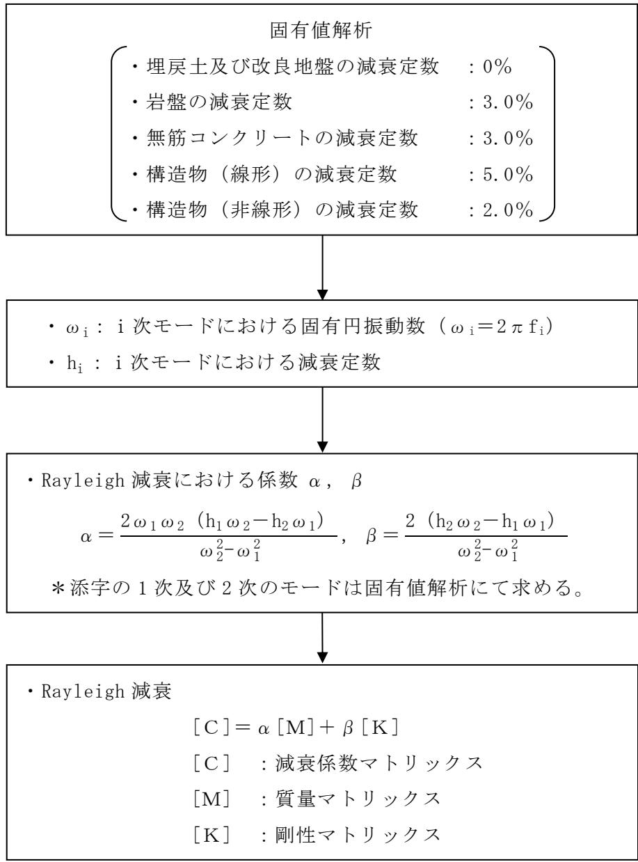
図 3-24 Rayleigh 減衰の設定フロー
