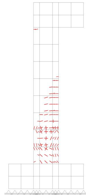
193 ステップ 破壊
