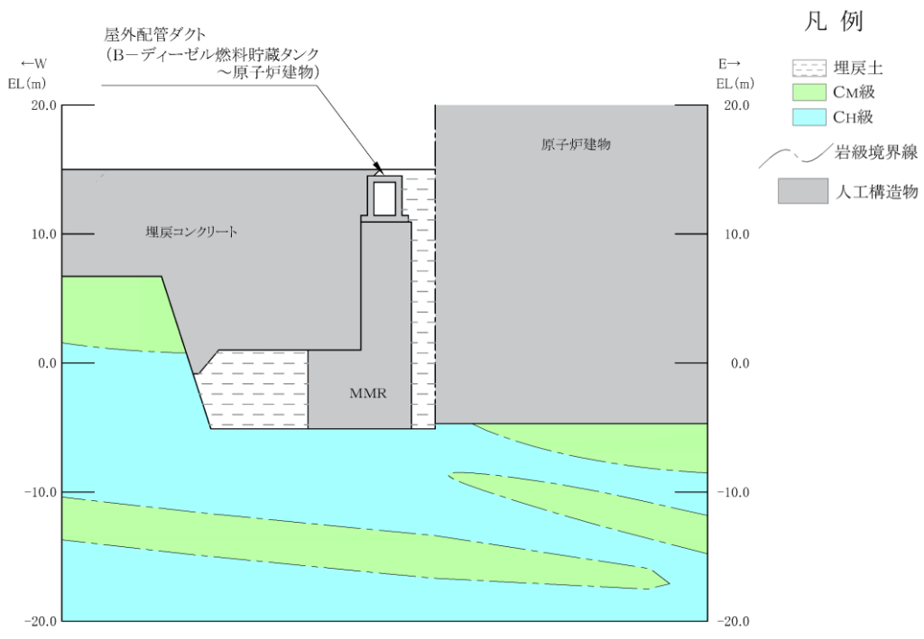
(岩級図)
