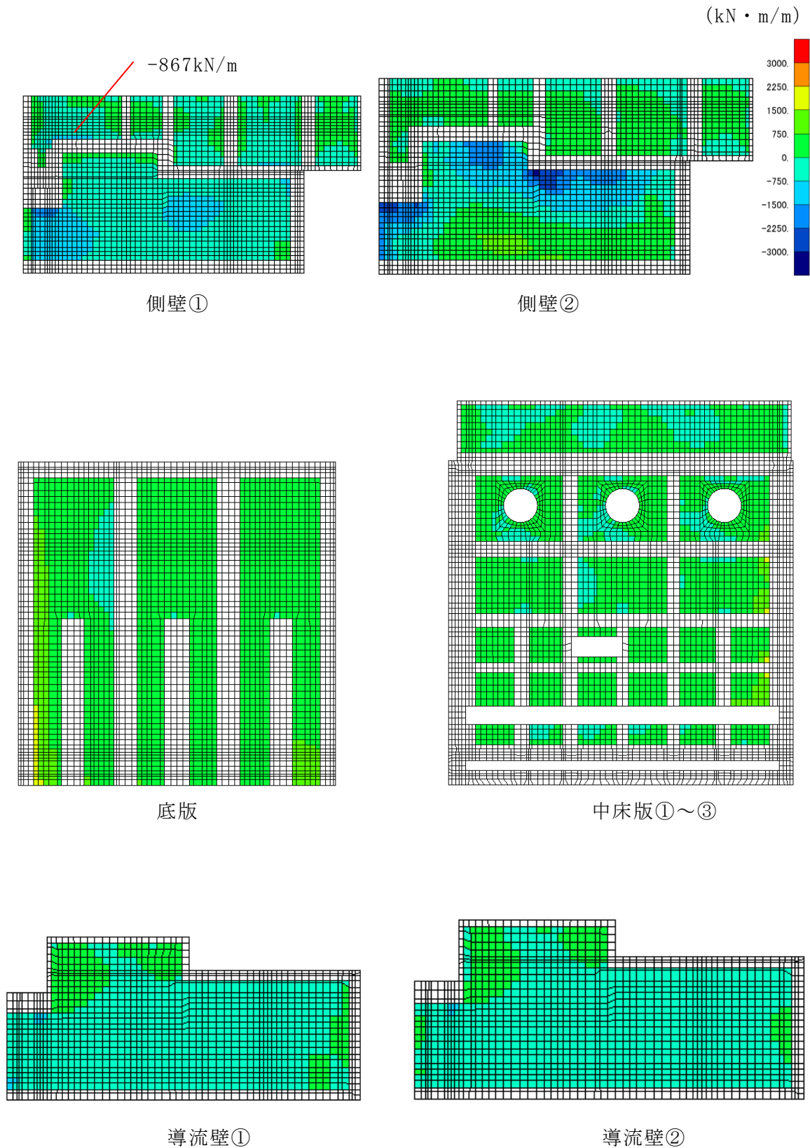
図 6-50 せん断破壊に対する照査値最大時の断面力分布図 (せん断力 (kN/m) : Q_x ) (側壁, 解析ケース②, S_s - D (-+) )
