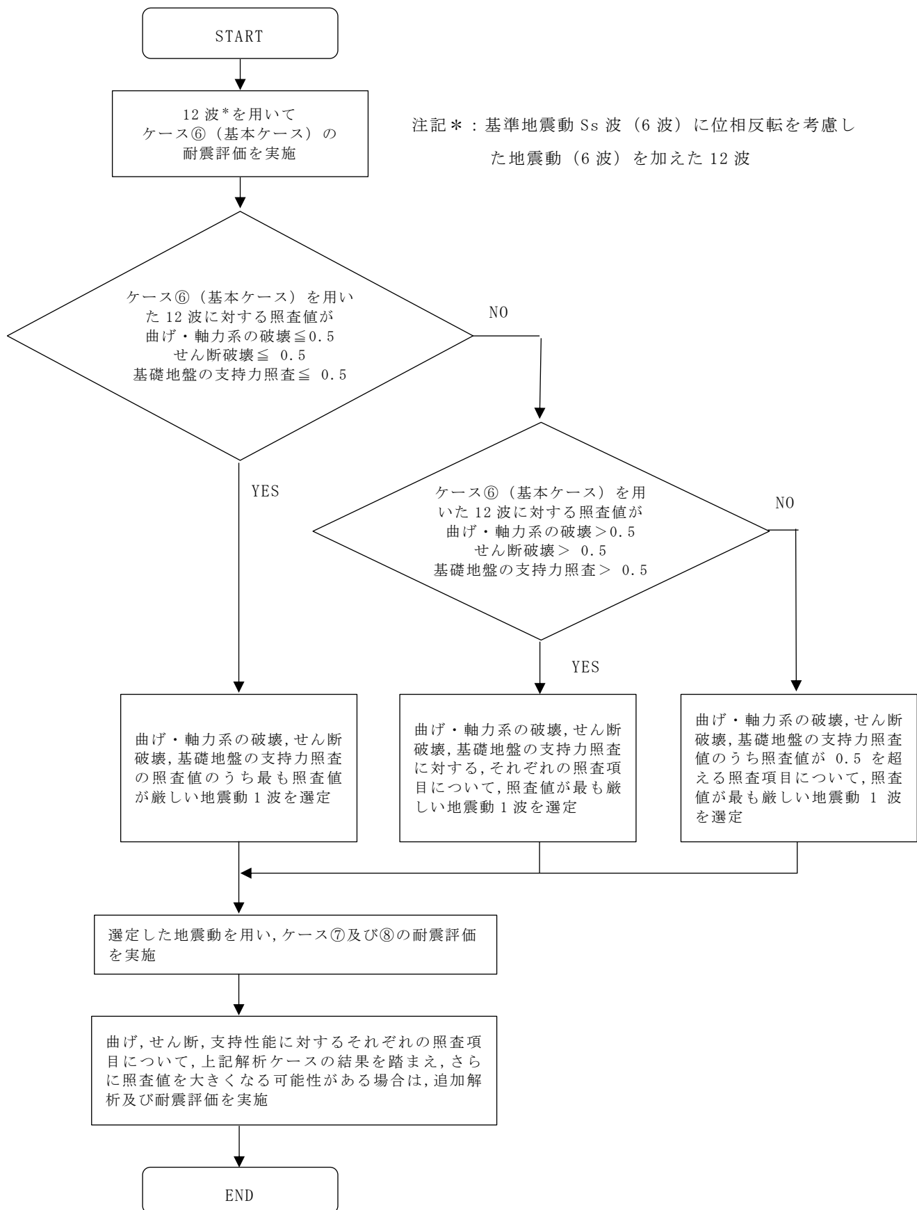
図 3-65 追加解析を実施する地震動の選定フロー（D-D 断面の例）
