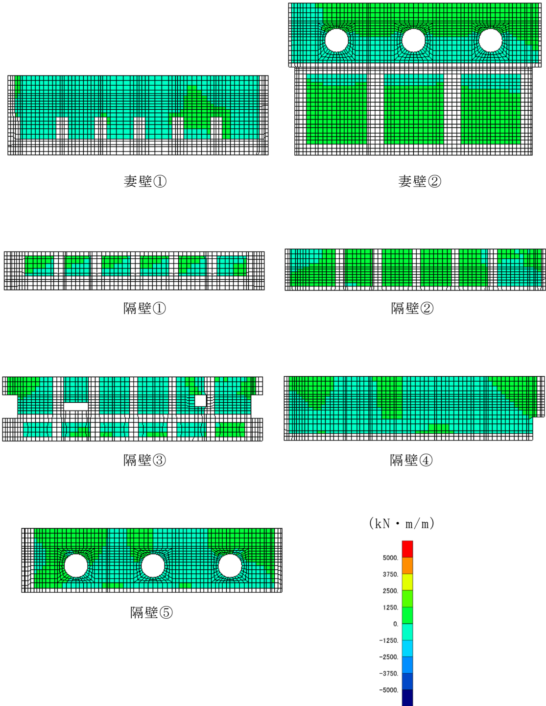
図 6-43 せん断破壊に対する照査値最大時の断面力分布図
