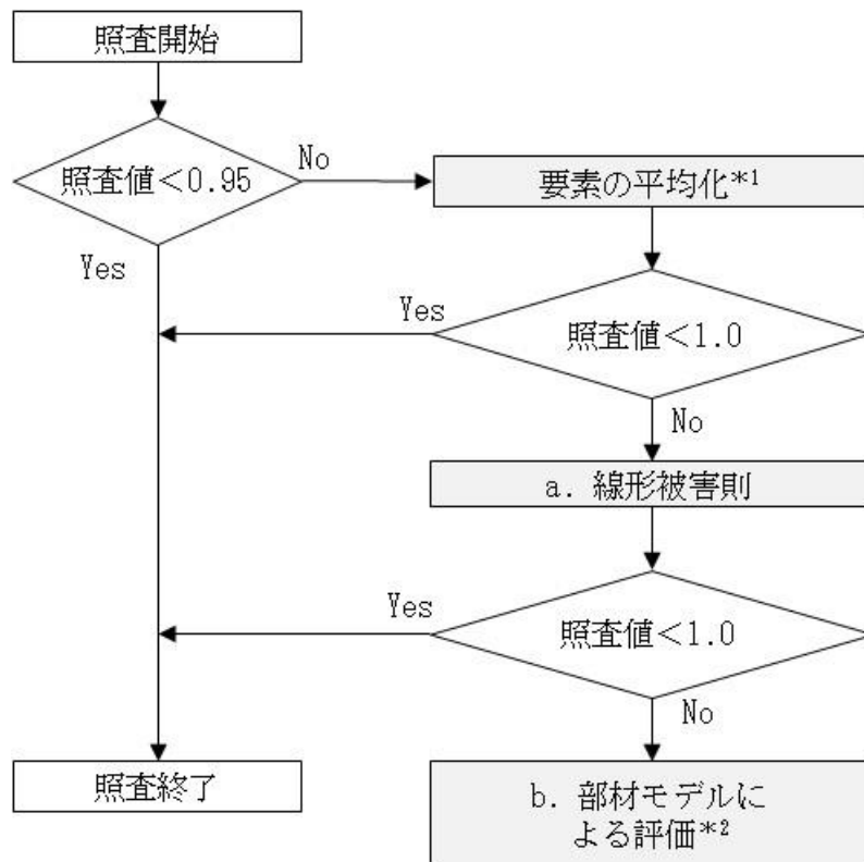
図 5-68 セン断破壊による照査フロー (PHb 設置なし)
