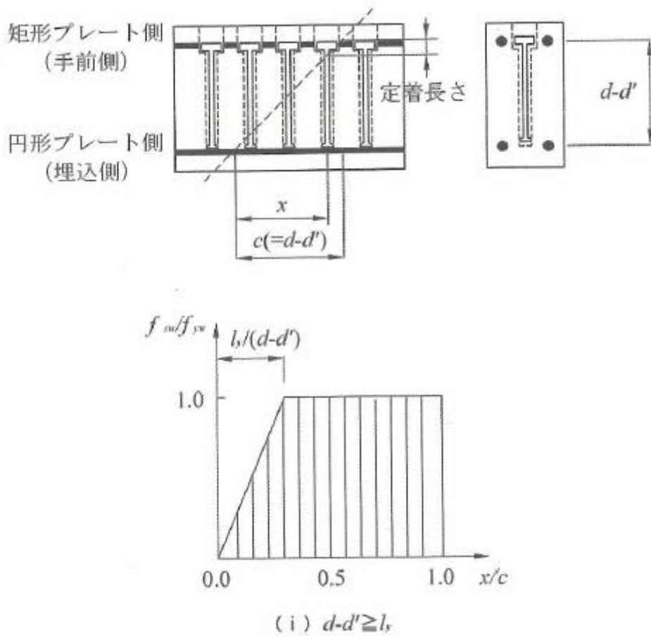
図 5-60 ポストヘッドバー (PHb) の有効率算定の概念図
