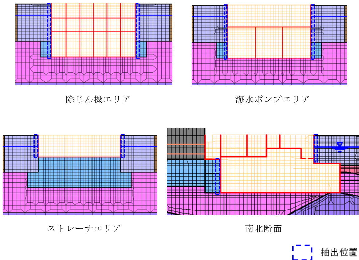
図4-24 地震時土圧・水圧及び周面せん断力の抽出位置
