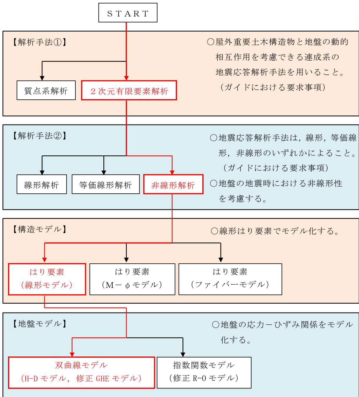
図 3-2 地震応答解析の選定フロー
