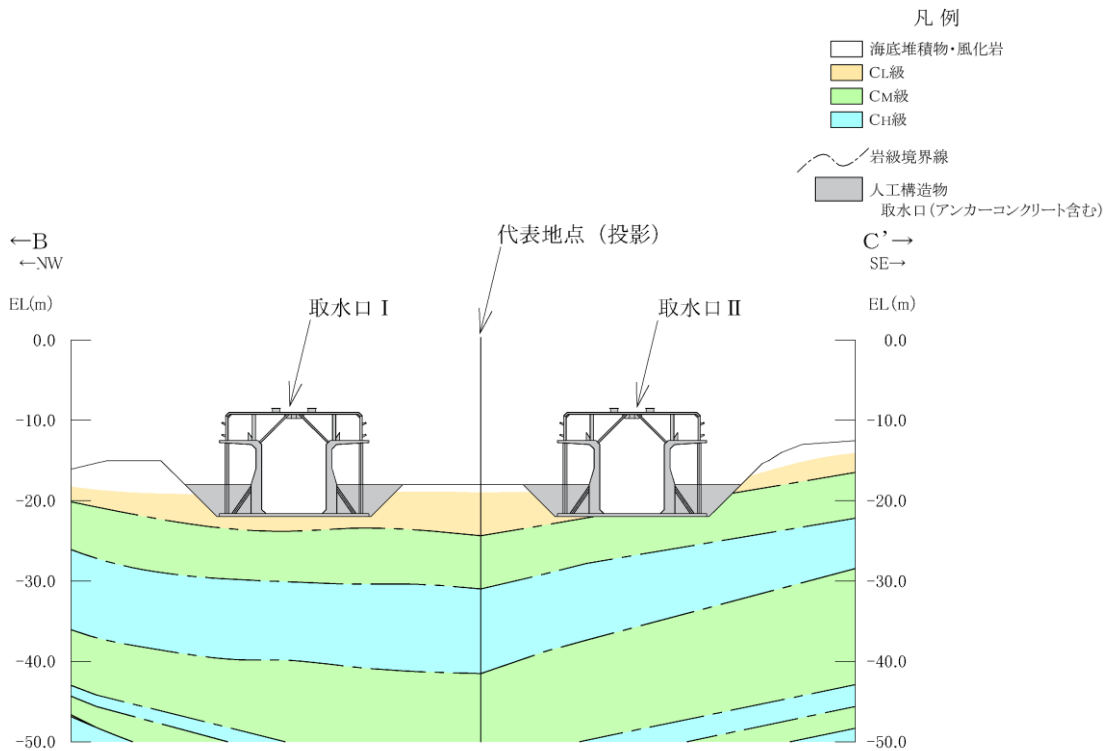
(岩級図)
