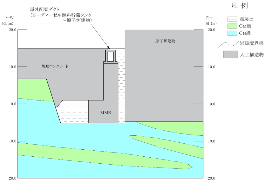
(岩級図)
