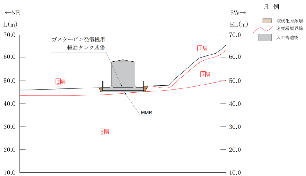
(速度層図)
