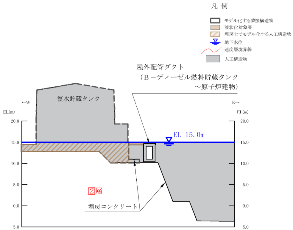
(速度層図)
