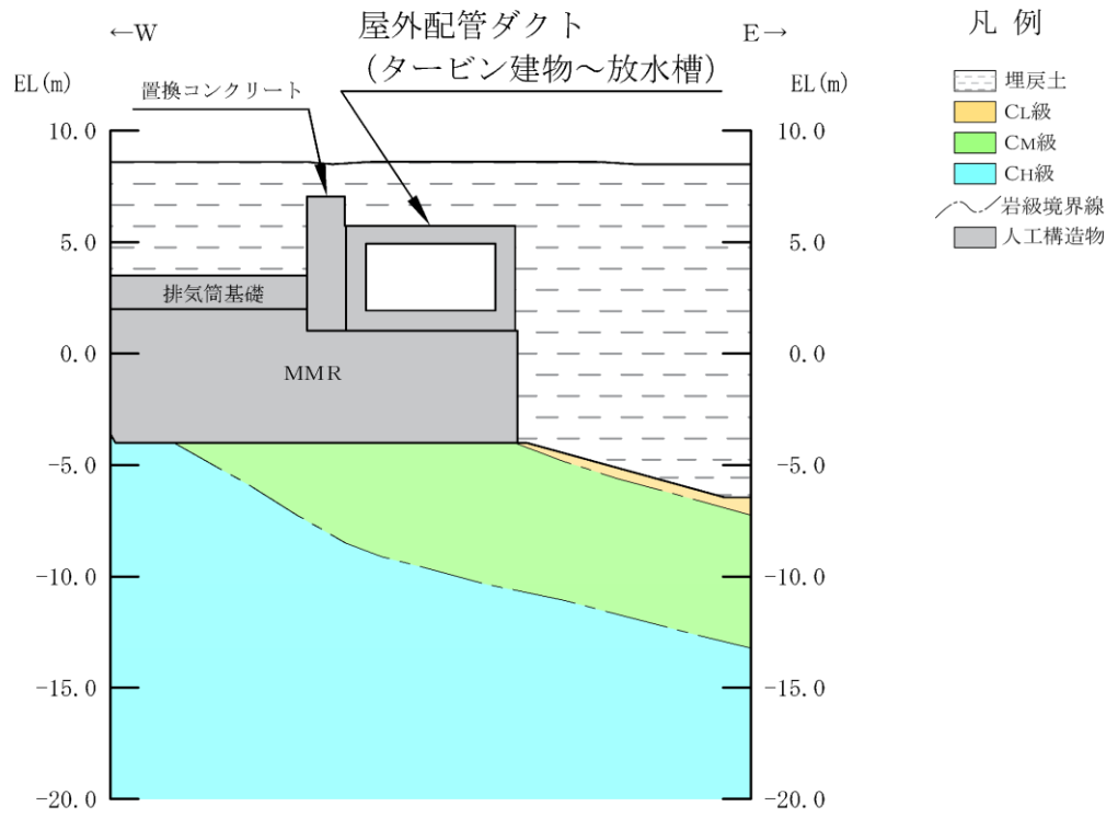
(岩級図)
