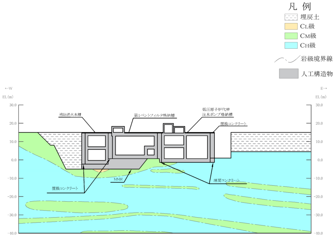
(岩級図)
