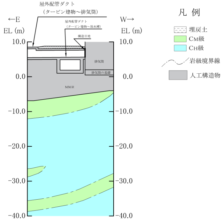
(岩級図)
