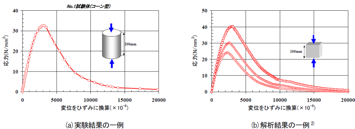
図6.3-3 コンクリートの圧縮ひずみが1.0% (10000 \mu ) 時点における残留応力 (「土木学会マニュアル2005」)
