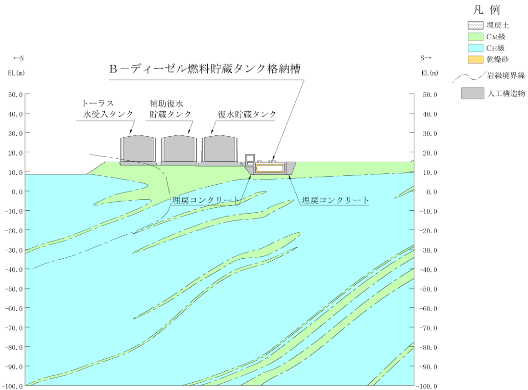
(岩級図)
