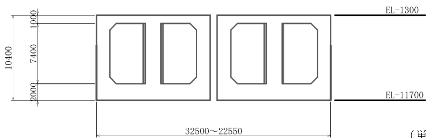
図 4.4-3(5) 取水槽 断面図(E-E断面)
