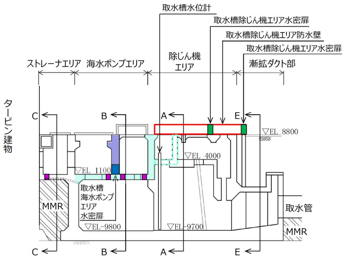
縦断図
