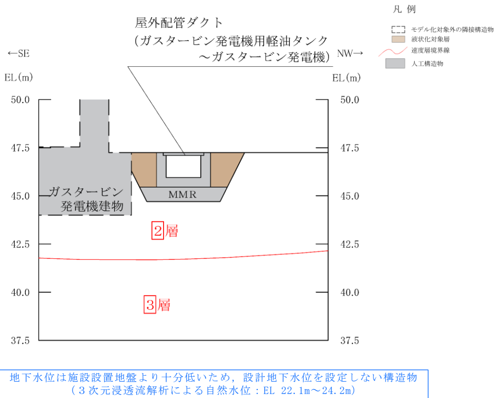
図 4.3-2(4) 屋外配管ダクト (ガスタービン発電機用軽油タンク～ガスタービン 発電機)【A-A断面位置】 地質断面図 (①全応力解析)
