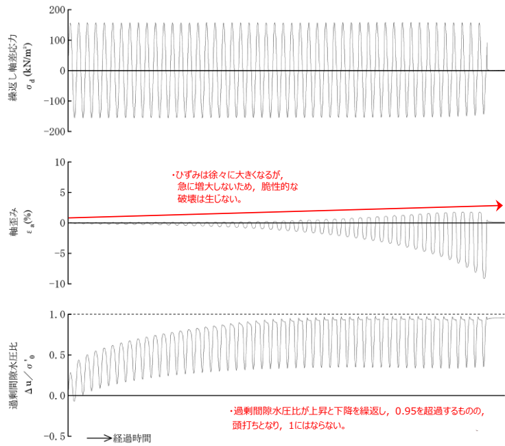
図 2-25 液状化強度試験結果 (E-7 : S7-16-1) (砂礫層)
