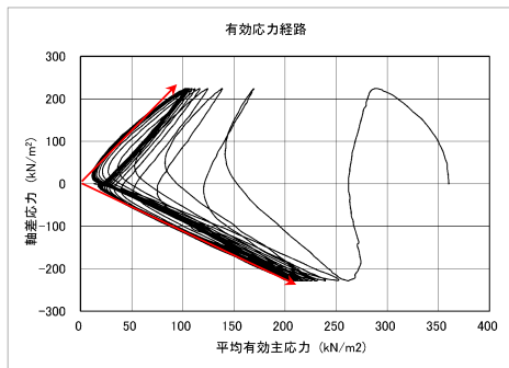
図 2-32 液状化強度試験結果 (E-8 : S8-24-1) (砂礫層)
