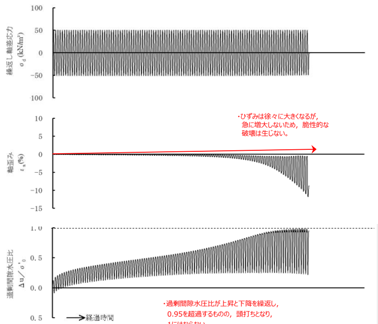
図 2-46 液状化強度試験結果 (E-1)
