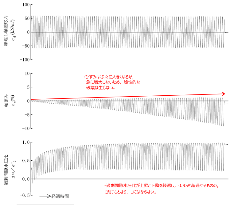
図 2-23 液状化強度試験結果 (E-7 : S7-3-4) (埋戻土)
