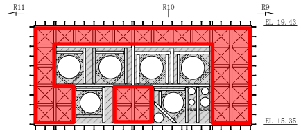
(a) MSトンネルBOP No. 1
