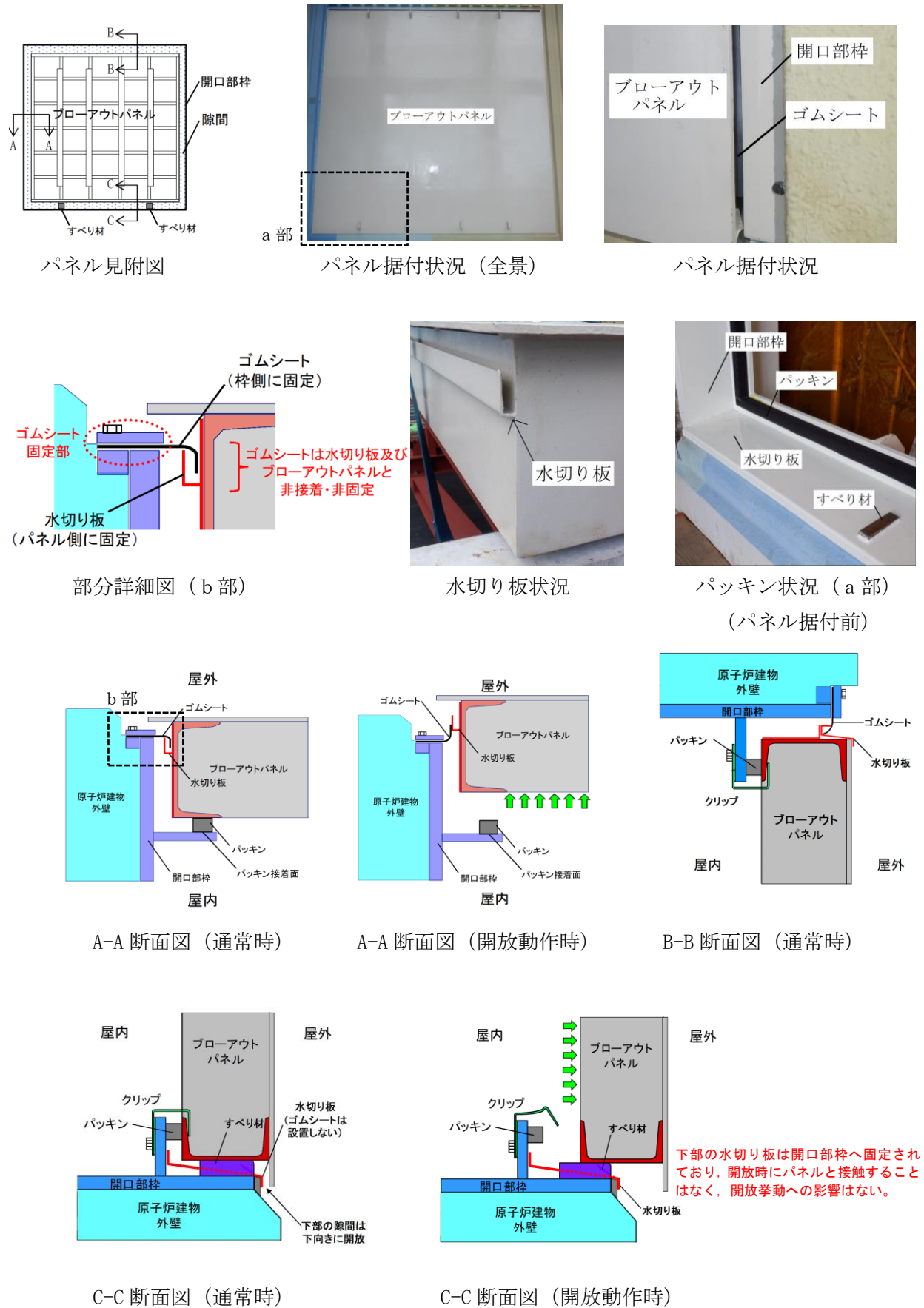
図 3-1(1) 水切り板，ゴムシート及びパッキンの設置状況概要
