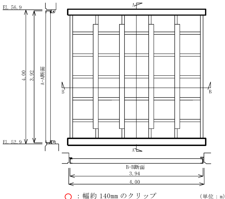
図4-4 クリップ取付け位置図（立面図）
