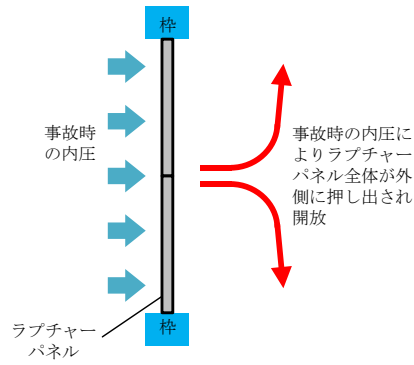
図 6-1 MS トンネル室 BOP の構造と作動原理
