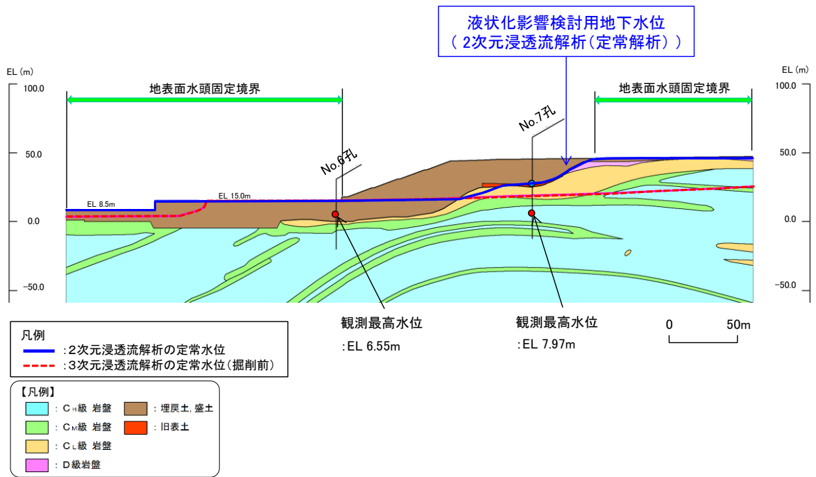
図 2.9.5-4 浸透流解析による地下水位の設定 (掘削形状等反映前)
