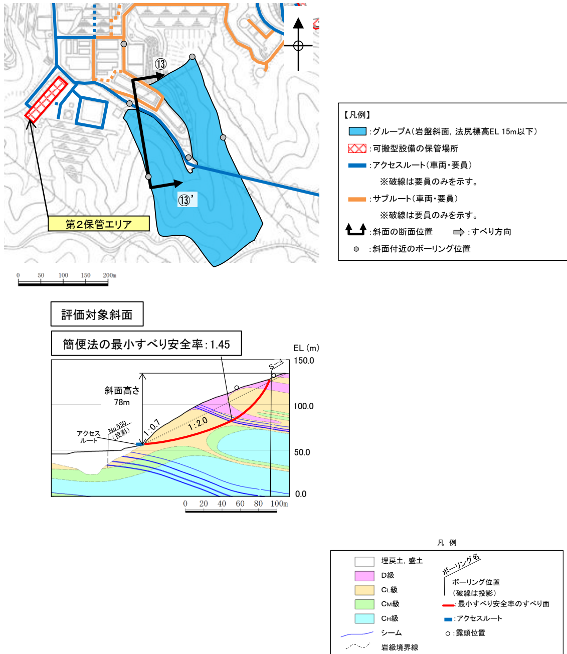
図 10 ⑬-⑬' 断面の比較結果
