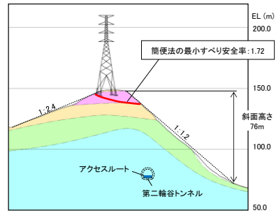
B-B' 断面
