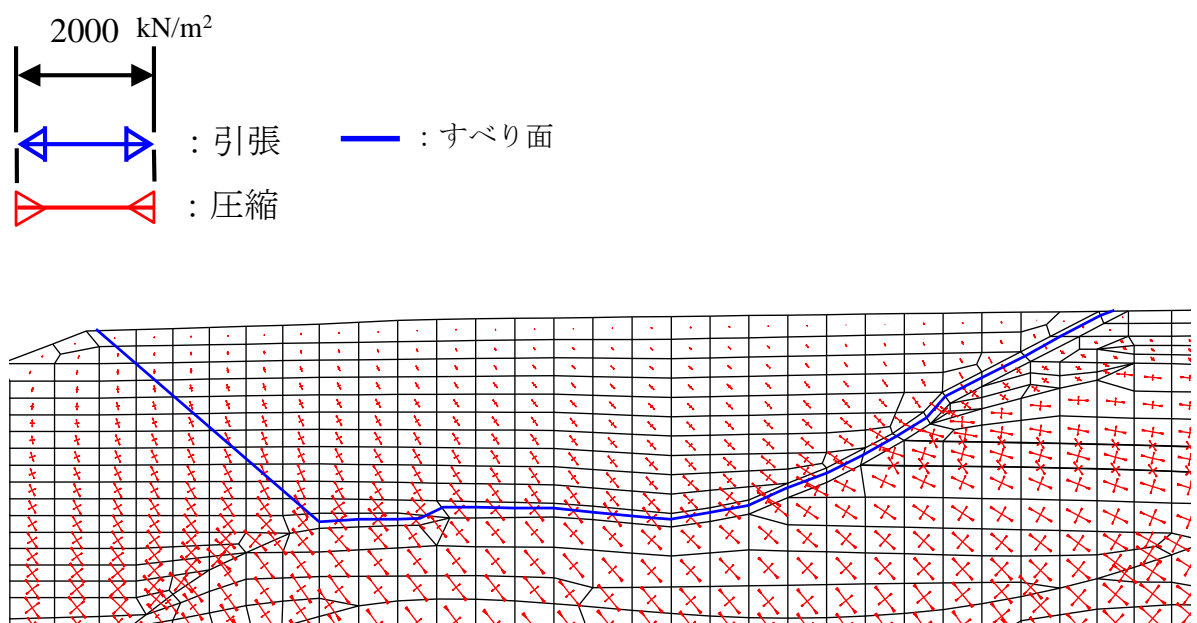
図 2.9.8-2 主応力図 (2号機南側盛土斜面 (⑧-⑧' 断面)) (S s -N1 (++) , t = 7.71)
