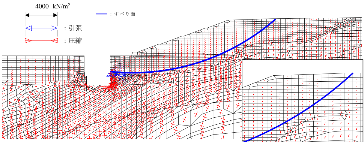
図 2.9.8-3 主応力図（2号機南側盛土斜面（⑧-⑧'断面）） （掘削後（有効応力解析）， S_s - D (-+) ， t = 10.61 ）
