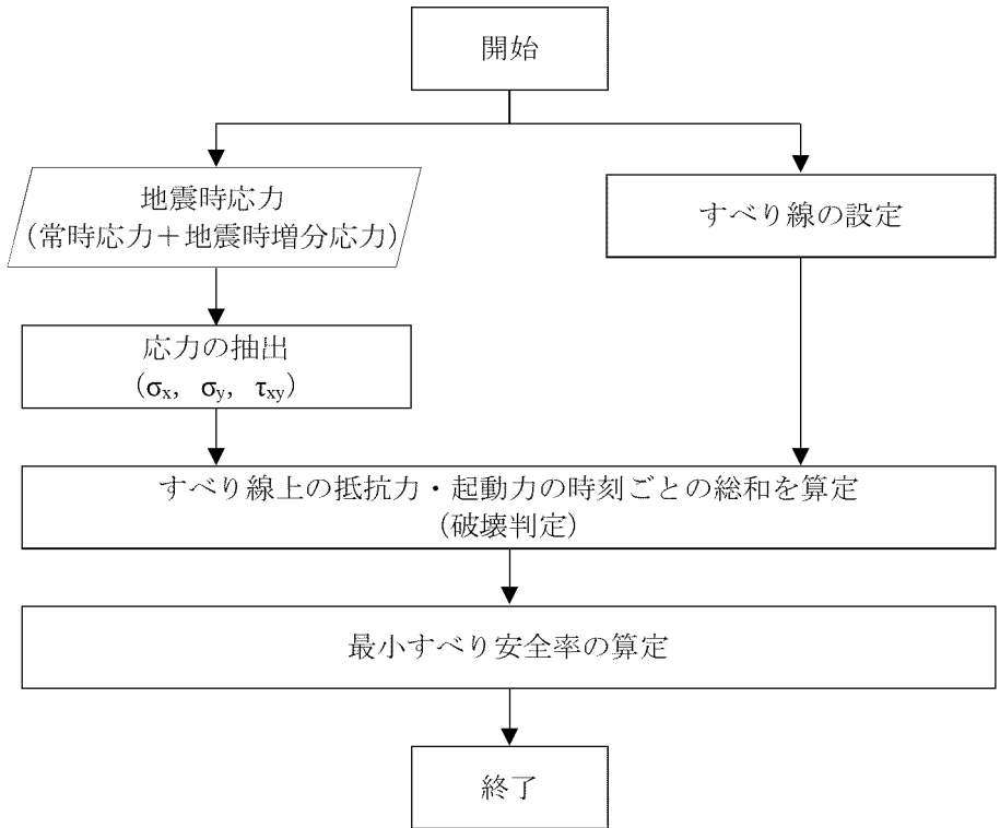
図1 解析フローチャート
