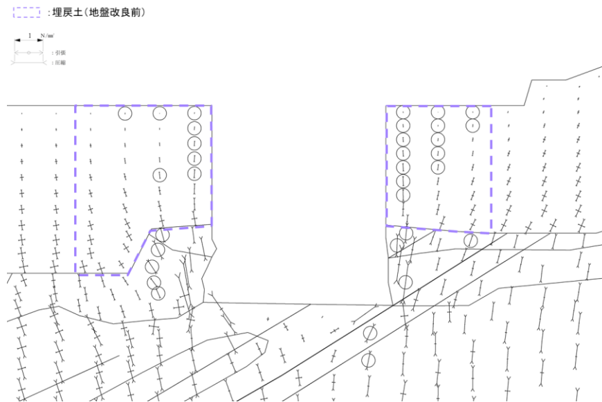
図 2.9.5-9 主応力図 (解析ケース② : ステップ A⇒B の 2 ステップ)
