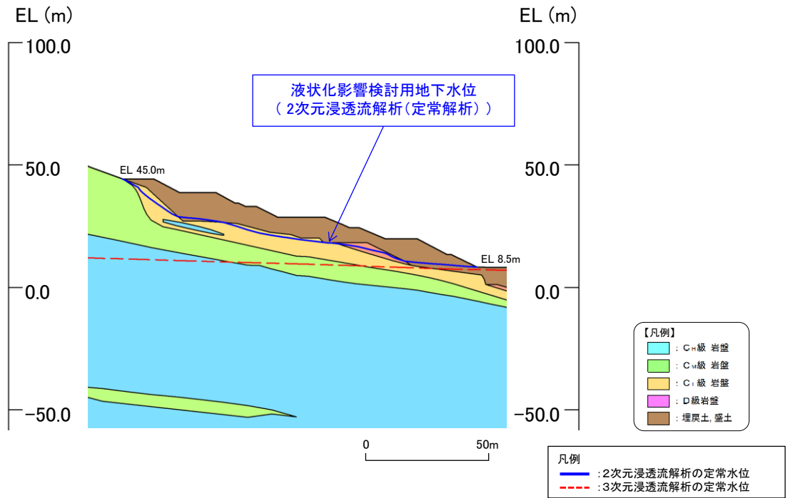
図 2.8.2.1-4 2次元浸透流解析結果
