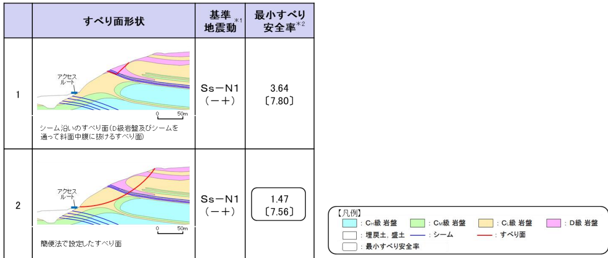
図 2.8.3.3-1 すべり安定性評価結果
