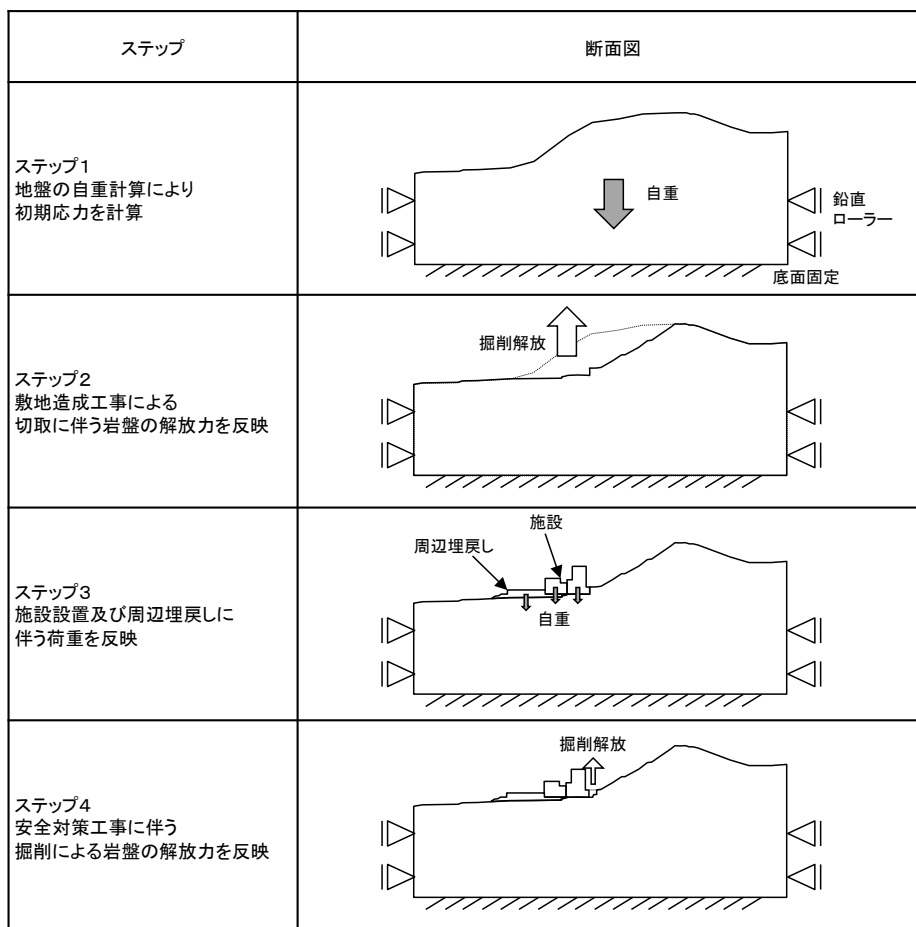
図 2.9.4-2 常時応力解析のステップ図
