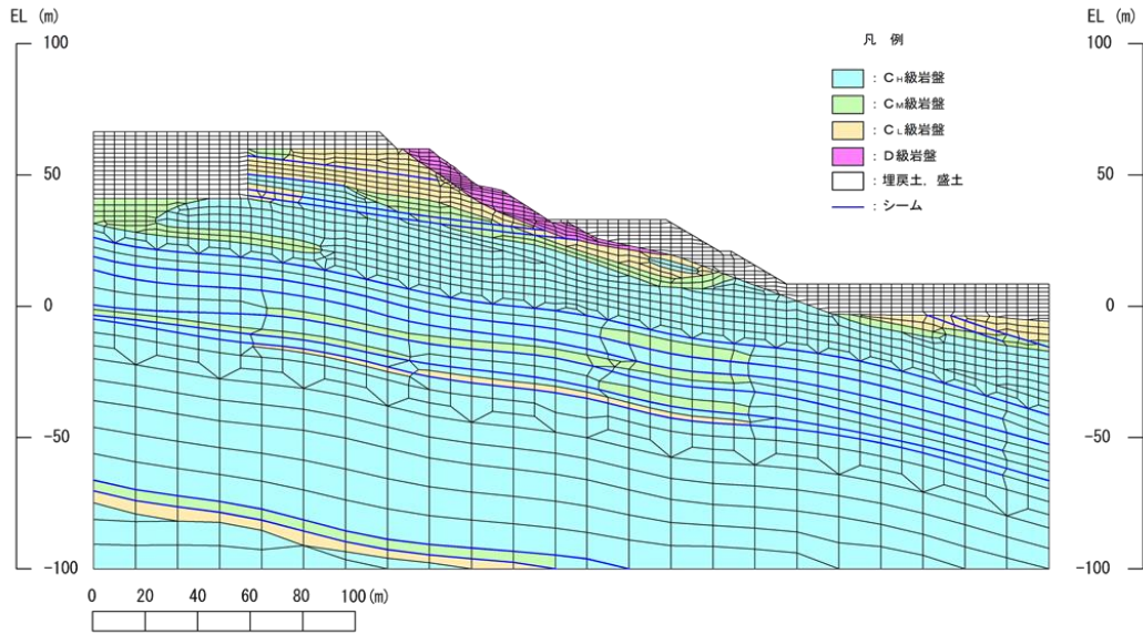
図 2.8.2.2-3 解析モデル図
