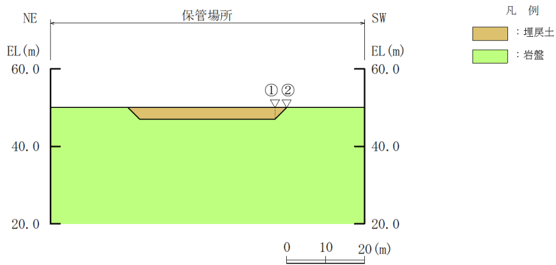
断面図
