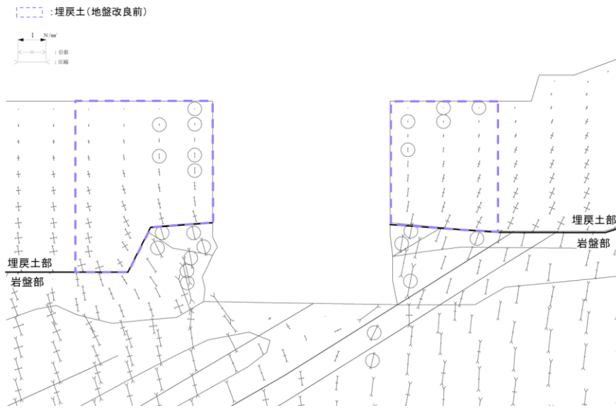
図 2.9.5-8 主応力図 (解析ケース① : ステップ B のみの 1 ステップ)
