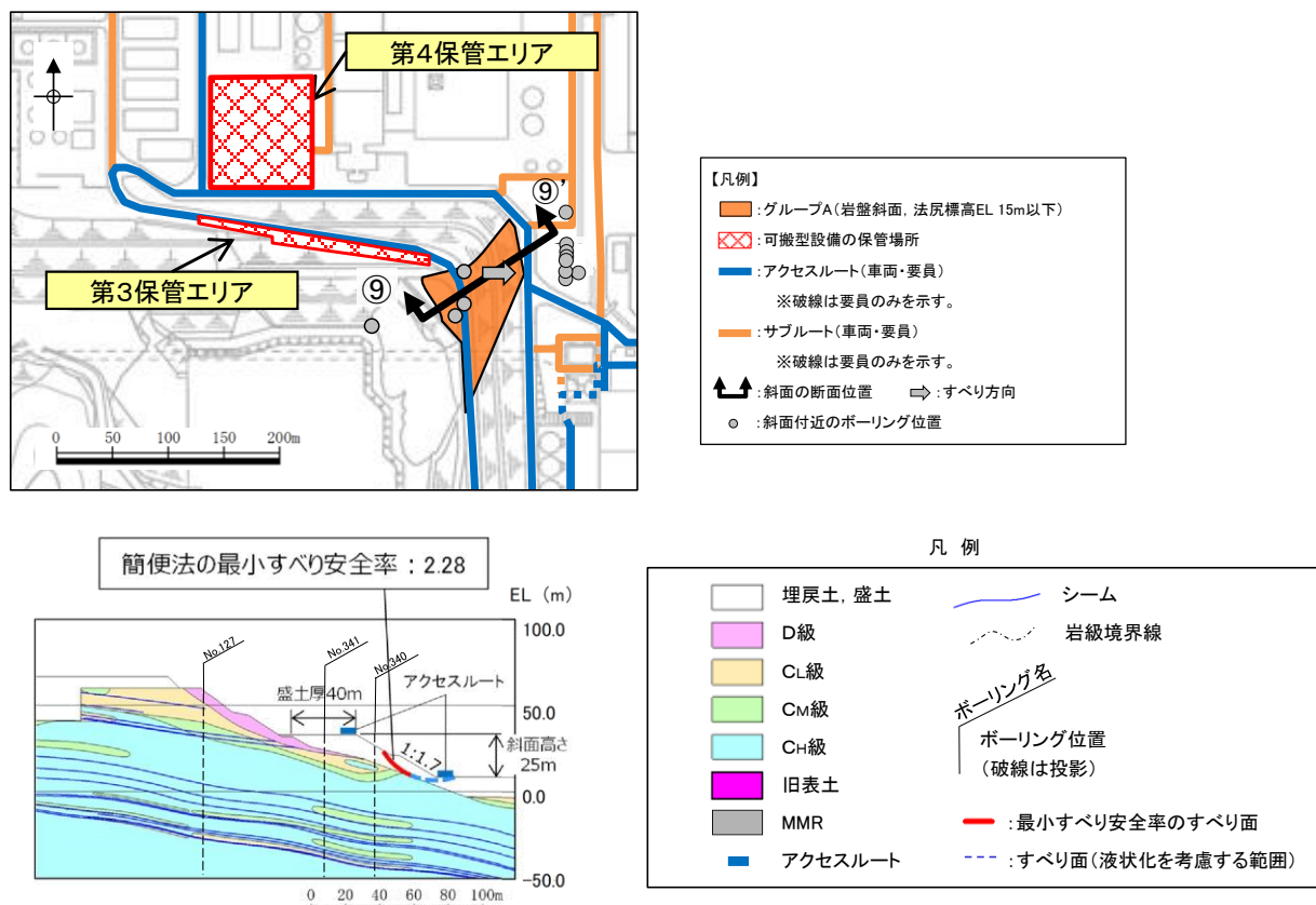
図 6 ⑨-⑨' 断面の比較結果
