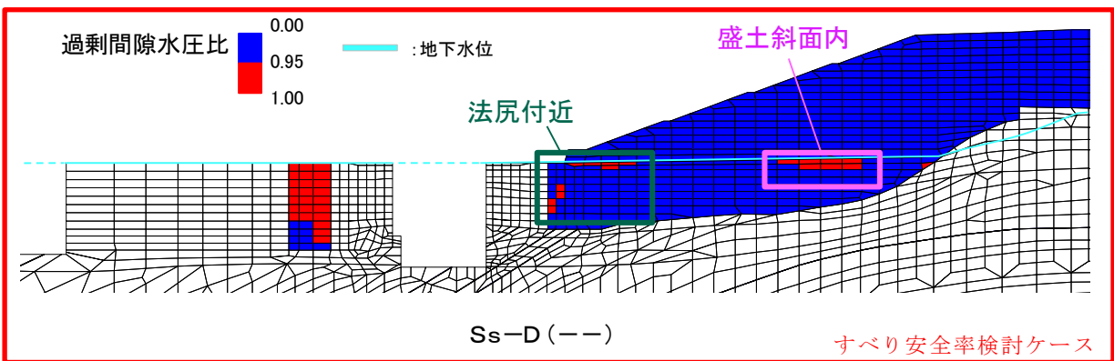
図 2.9.8-8 S s - D の各地震動方向における過剰間隙水圧比分布図 (全時刻最大)
