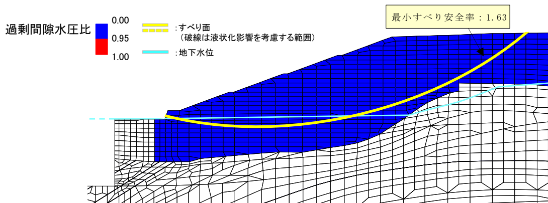
図 2.9.8-11 液状化範囲を通るすべり面の最小すべり安全率 (S s - D (---) , t=15.03s)
