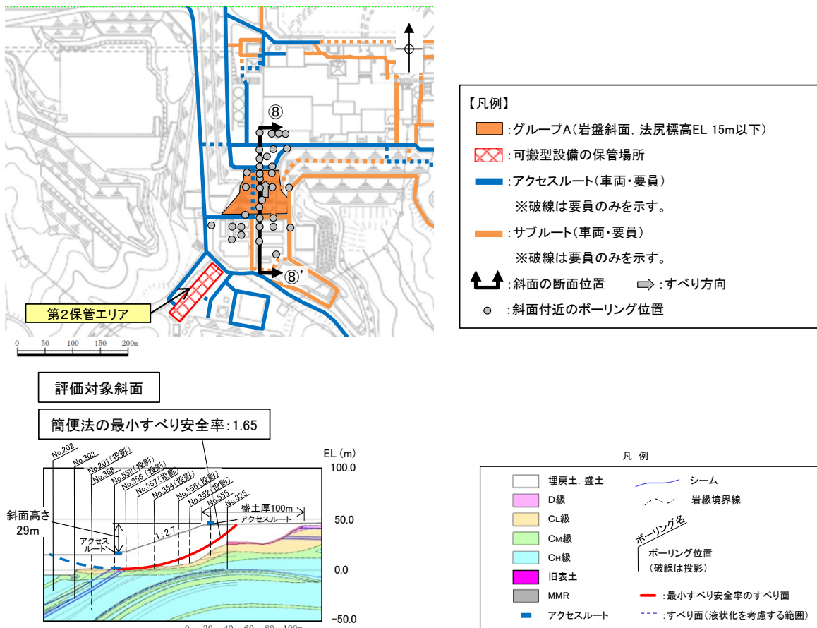
図5 ⑧-⑧'断面の比較結果
