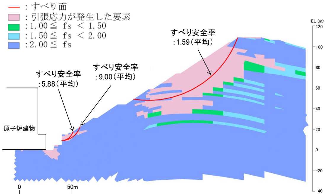
図 2.9.7-1 局所安全係数分布図（2号機南側切取斜面（④-④'断面）） （S s -D（-+）, t=19.15）
