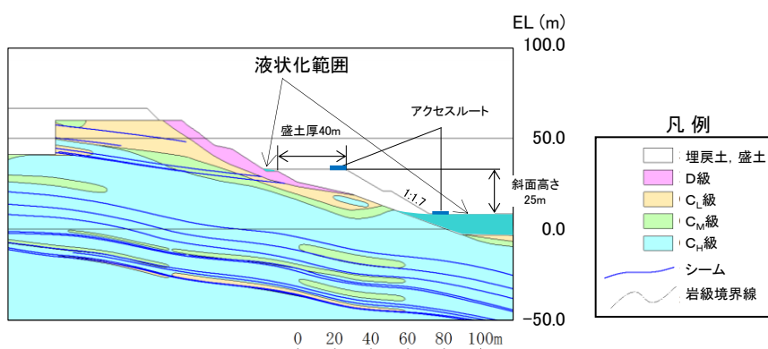
⑨-⑨' 断面
