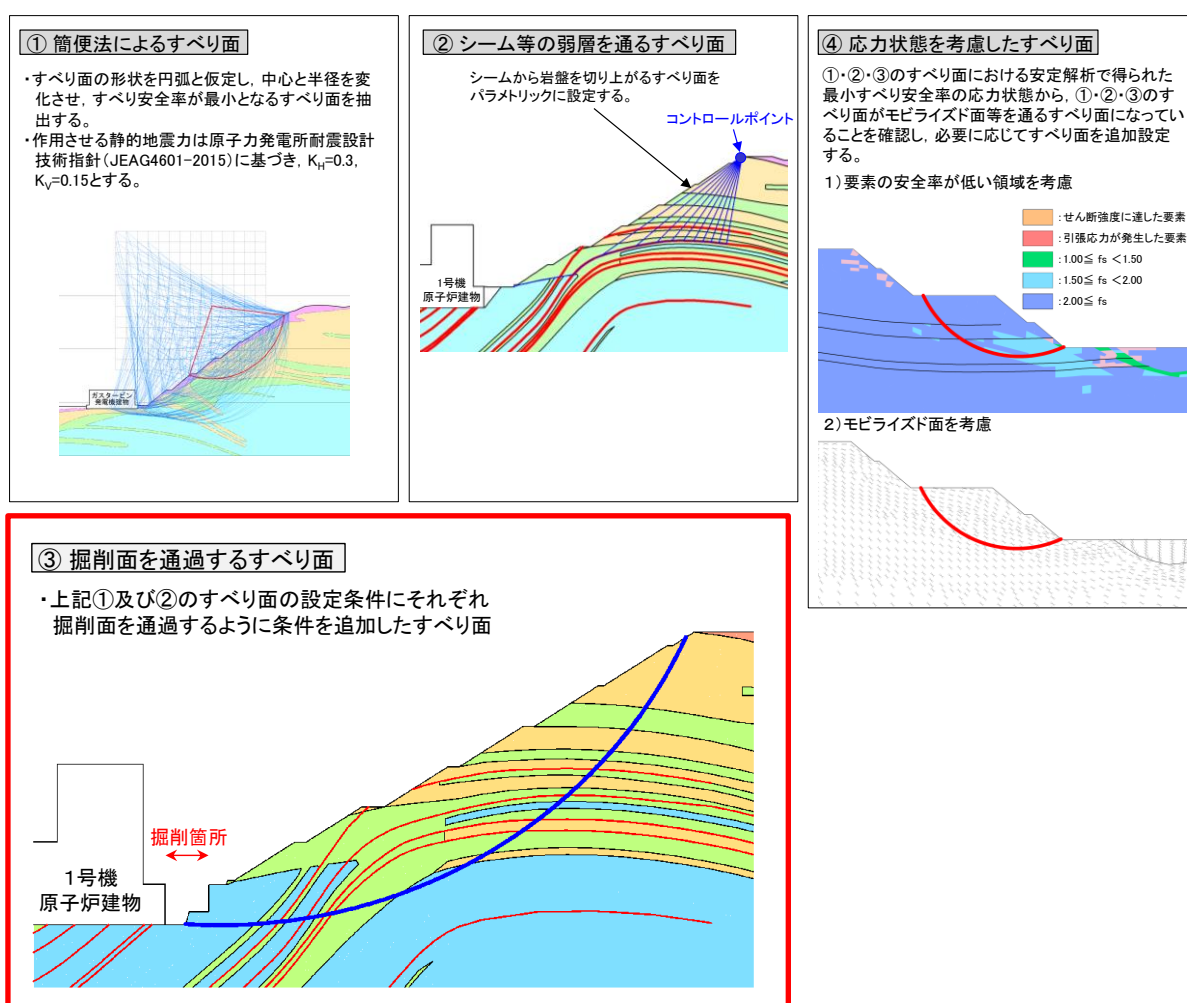
図 2.9.6-1 想定すべり面の設定方法（赤枠追加）
