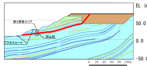
【B21・22シーム、法尻近傍のC 0 級岩盤及び B23・24シームを通過して法尻に抜けるすべり面】
