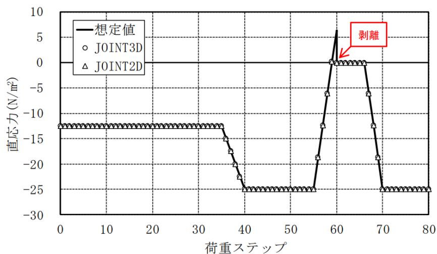
(a) 直応力
