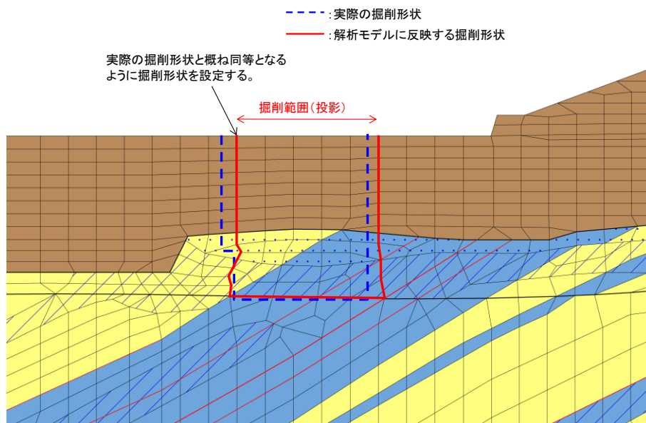
図 2.9.5-7 掘削形状の反映方法
