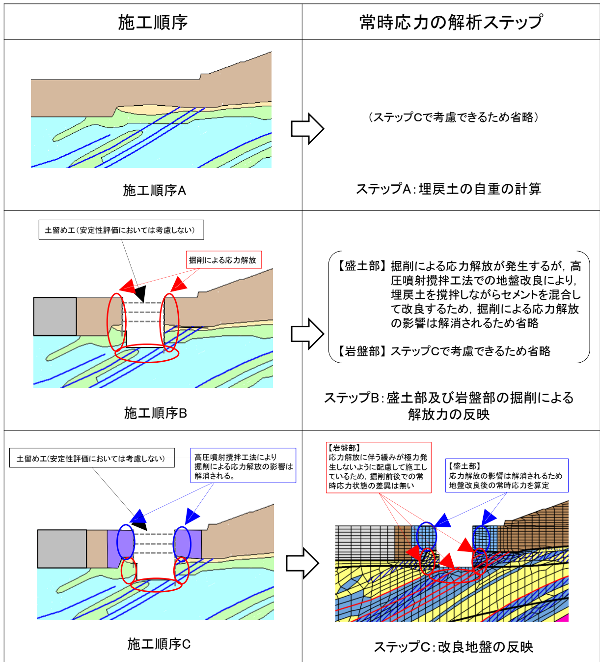
図 2.9.5-6 施工状況及び常時応力解析のモデル (2号機南側盛土斜面 掘削箇所近傍)
