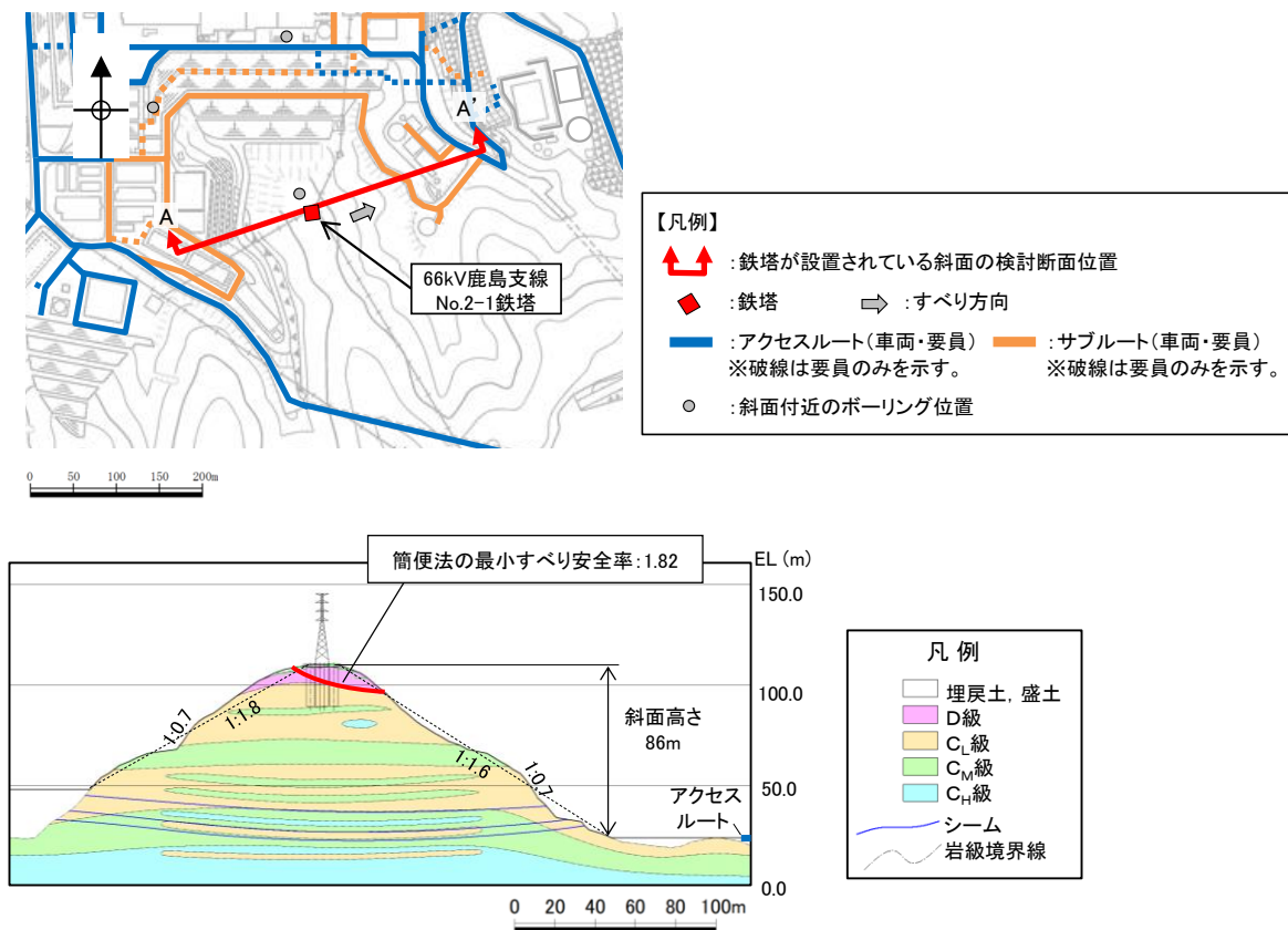
図 13 A-A' 断面の比較結果
