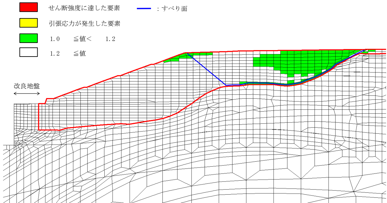
図 2.9.8-1 局所安全係数分布図 (2号機南側盛土斜面 (⑧-⑧' 断面))
