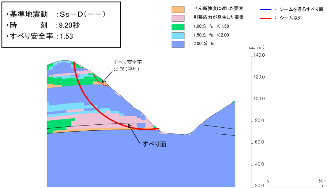
図 2.8.3.4-2 局所安全係数分布図
