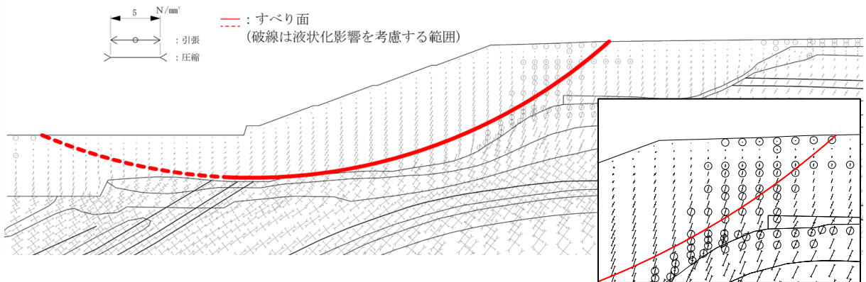
図 2.9.8-4 主応力図（2号機南側盛土斜面（⑧-⑧'断面）） （掘削前（2.6.3.2, 全応力解析）， S_s - D (-+) ， t = 13.15 ）
