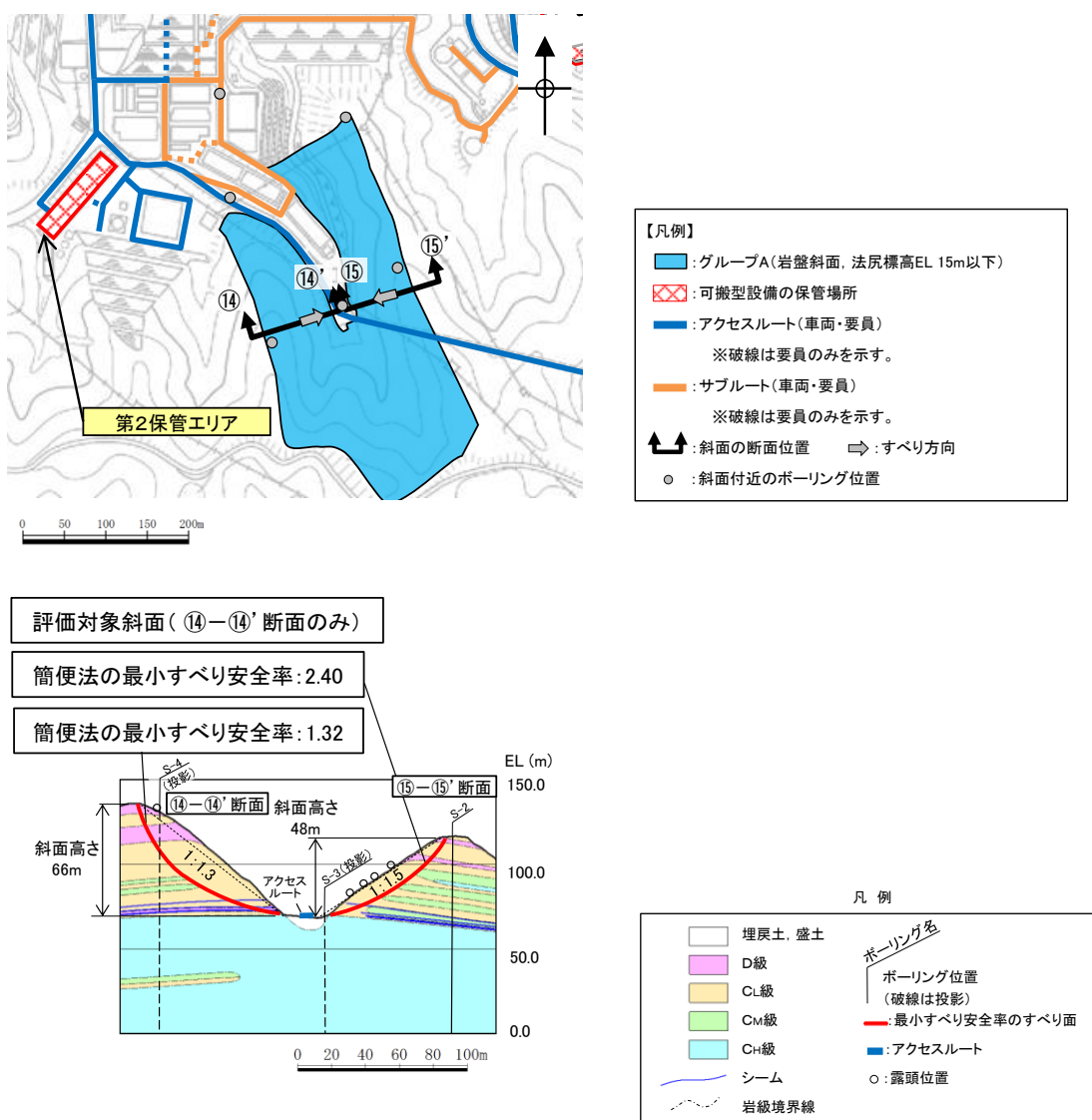
図 11 ⑭-⑭' 断面及び⑮-⑮' 断面の比較結果
