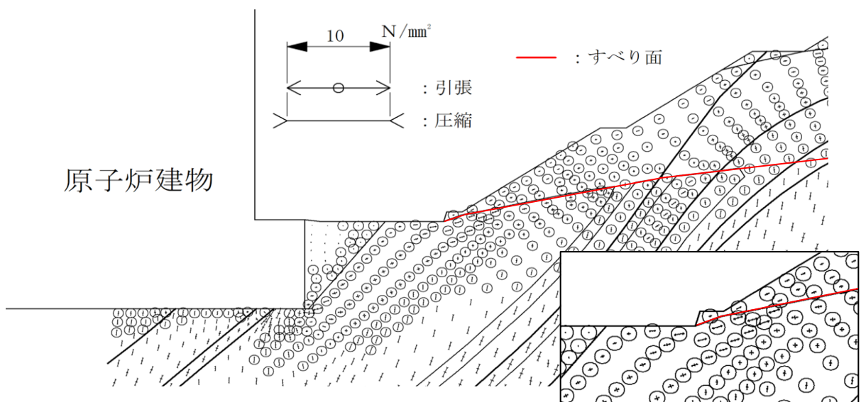
図 2.9.7-4 主応力図（2号機南側切取斜面（④-④'断面）） （掘削前（2.6.3.1，全応力解析），S s - N 1（-+），t = 7.45）
