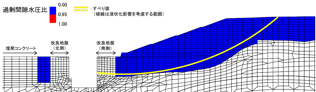
図 2.9.8-5 過剰間隙水圧比分布図（2号機南側盛土斜面（⑧-⑧'断面）） （掘削後（有効応力解析）， S_s - D(-+) ， t = 10.61 ）
