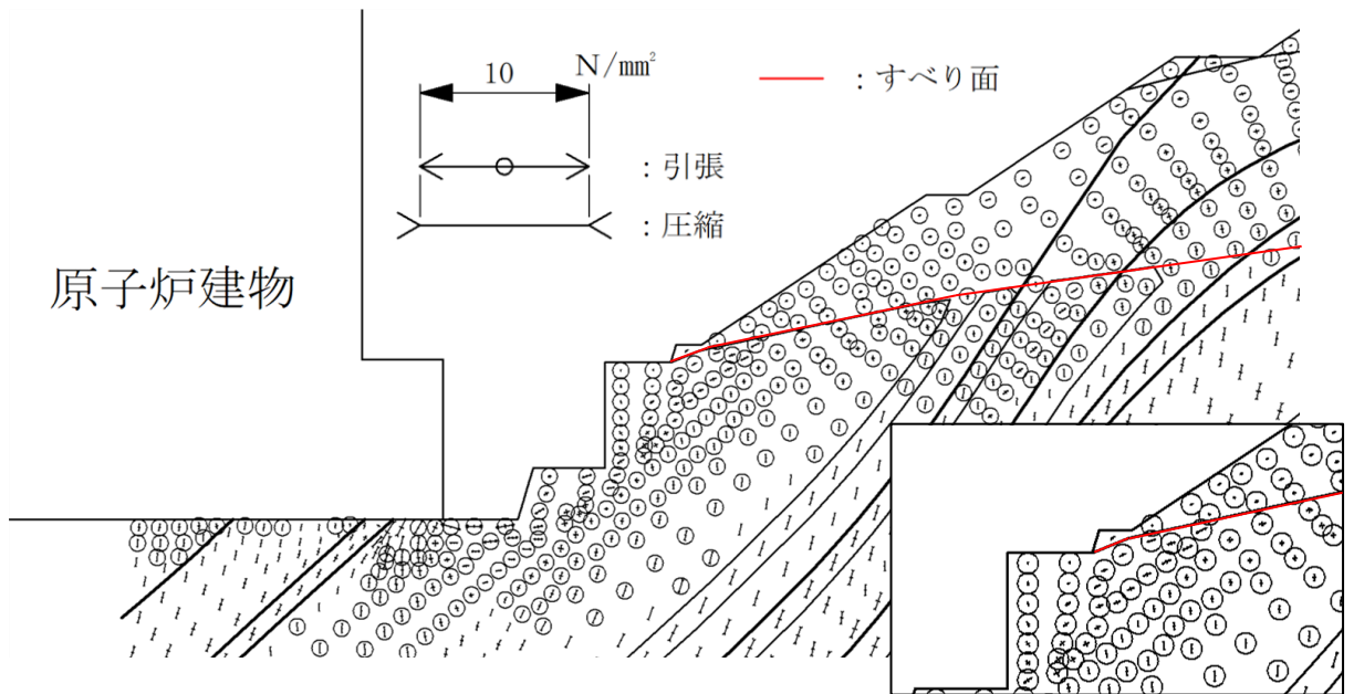
図 2.9.7-3 主応力図（2号機南側切取斜面（④-④'断面）） （掘削後（全応力解析），S s - N 1（-+），t = 7.45）
