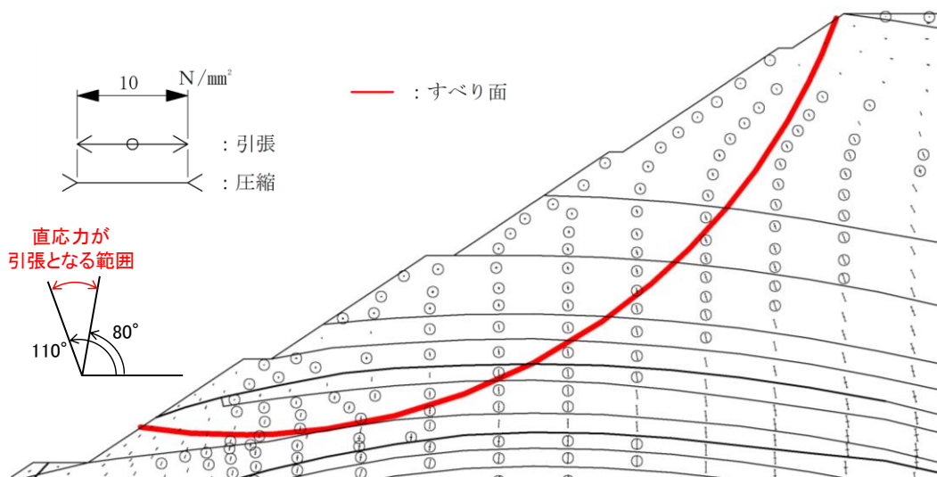
図 2.9.7-2 主応力図 (2号機南側切取斜面 (④-④' 断面)) (S s - D (-+), t = 19.15)
