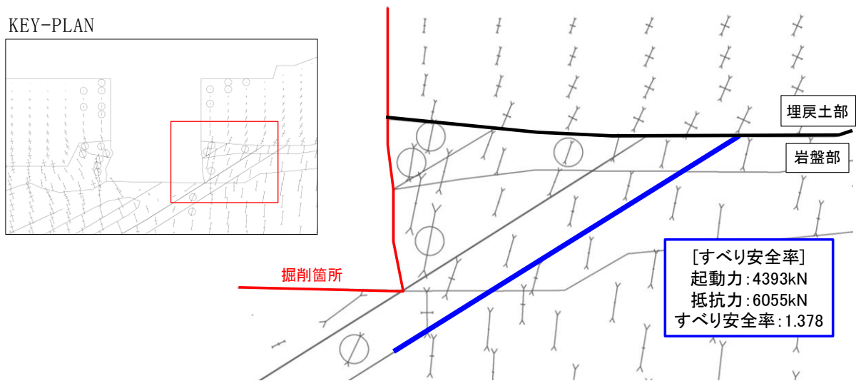
図 2.9.5-10 掘削箇所近傍を通るシームにおけるすべり安全率 (解析ケース①：ステップBのみの1ステップ)
