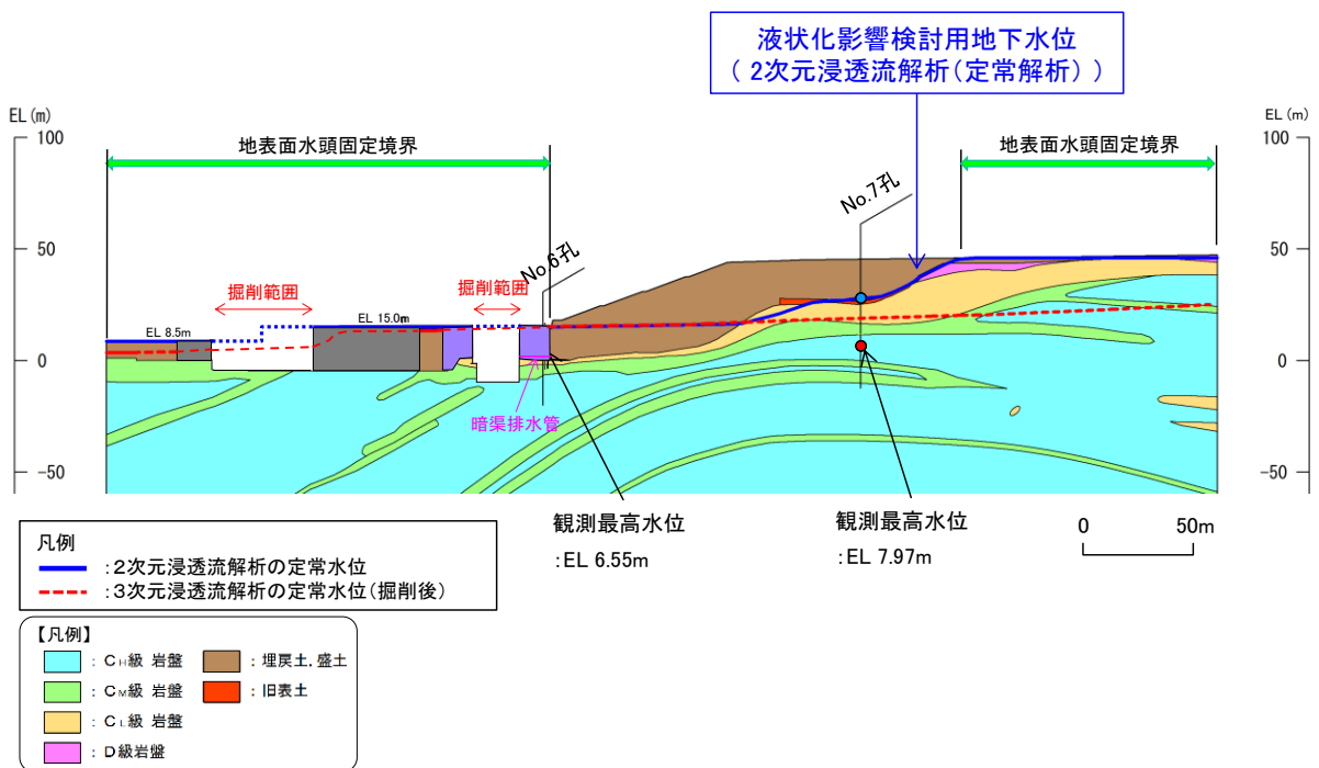
図 2.9.5-5 浸透流解析による地下水位の設定 (掘削形状等反映後)
