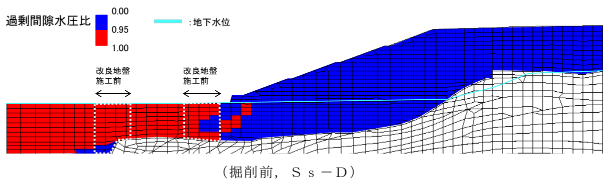
図 2.9.8-7 液状化範囲の比較
