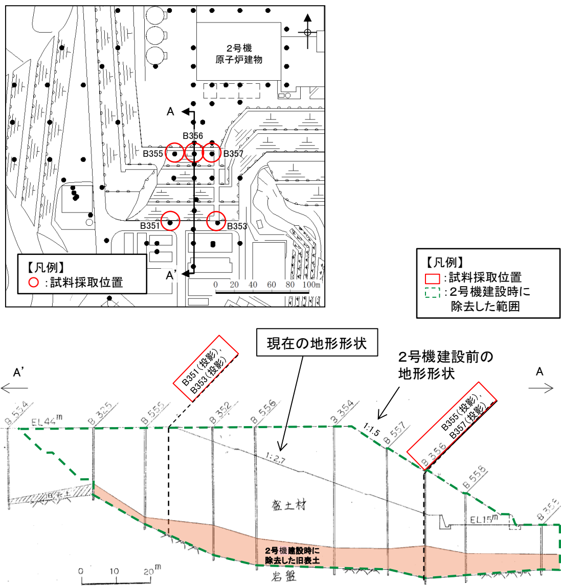
図2 試料採取位置図 (旧表土)
