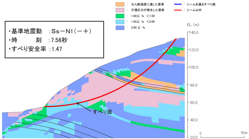
図 2.8.3.3-2 局所安全係数分布図
