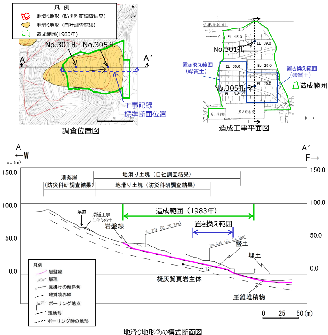
図 2.8.2.1-2 地滑り地形②の模式断面図
