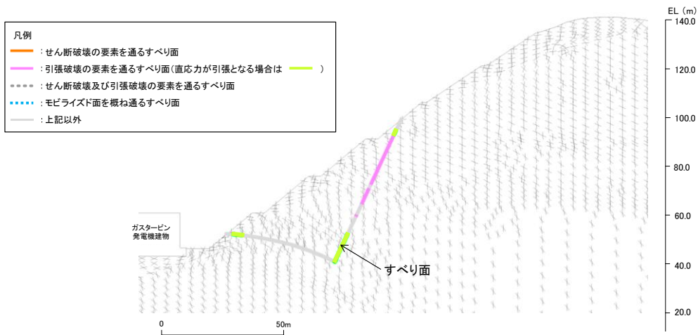
図 2.8.3.2-4 モビライズド面
