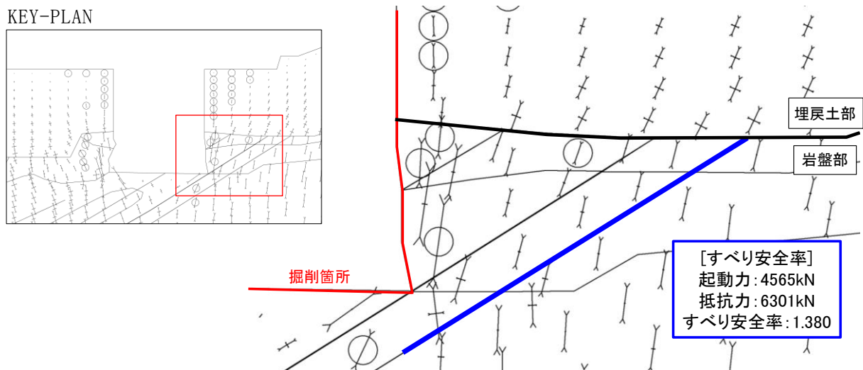
図 2.9.5-11 掘削箇所近傍を通るシームにおけるすべり安全率 (解析ケース②：ステップA⇒Bの2ステップ)
