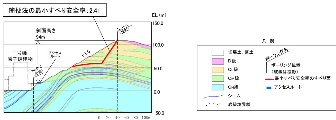
図2 ④-④'断面の比較結果
