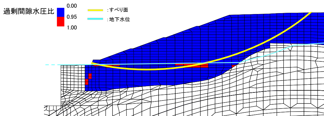
図 2.9.8-10 液状化により安全率が厳しくなると考えられるすべり面 (S s - D (---) における過剰間隙水圧比分布 (全時刻最大))
