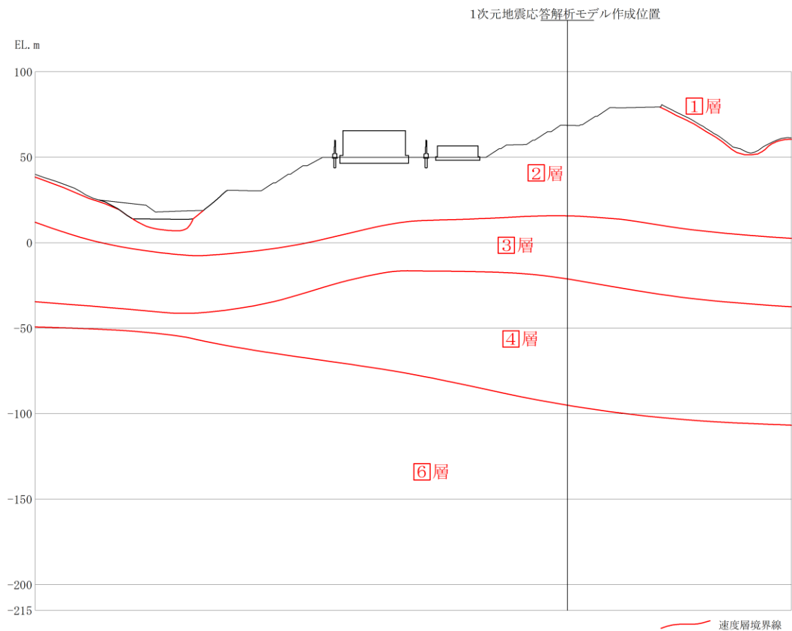
図 1.4.10-7 1次元地震応答解析モデルの作成位置（速度層区分図に追記）
