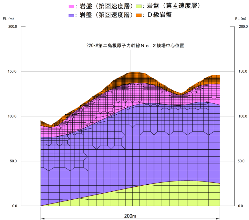
図 1. 1. 10-26 地盤の地震応答解析モデル図 (220kV 第二島根原子力幹線 No. 2 鉄塔) (東西方向)
