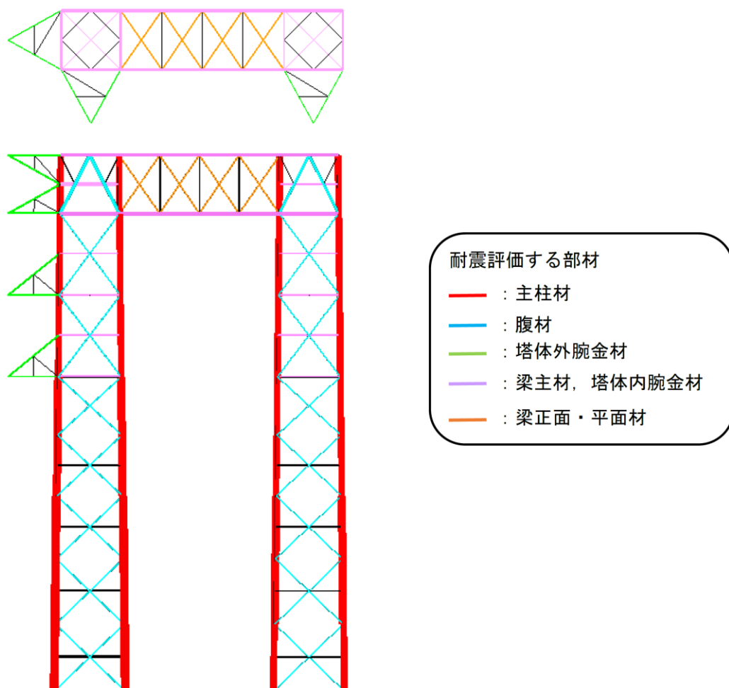
図 1.3.4-1 第 2-66kV 開閉所屋外鉄構部材名称図
