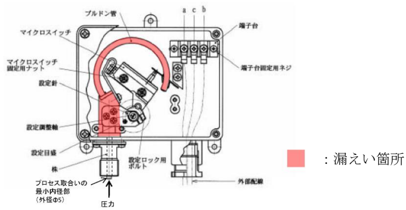
別図 5-1 計器内部構造図 (例)
