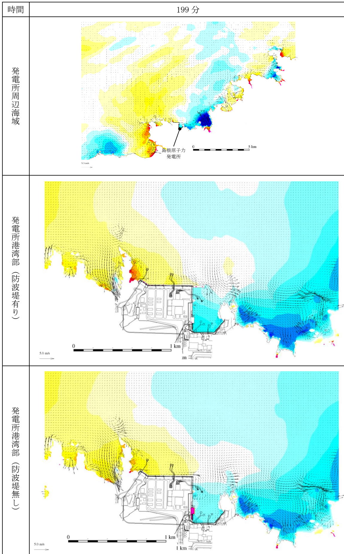
図 1-199 基準津波 1 の水位変動・流向ベクトル
