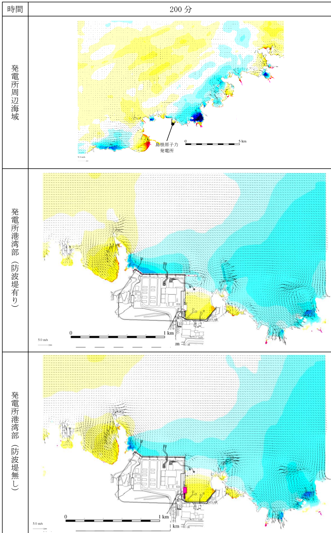
図 1-201 基準津波 1 の水位変動・流向ベクトル
