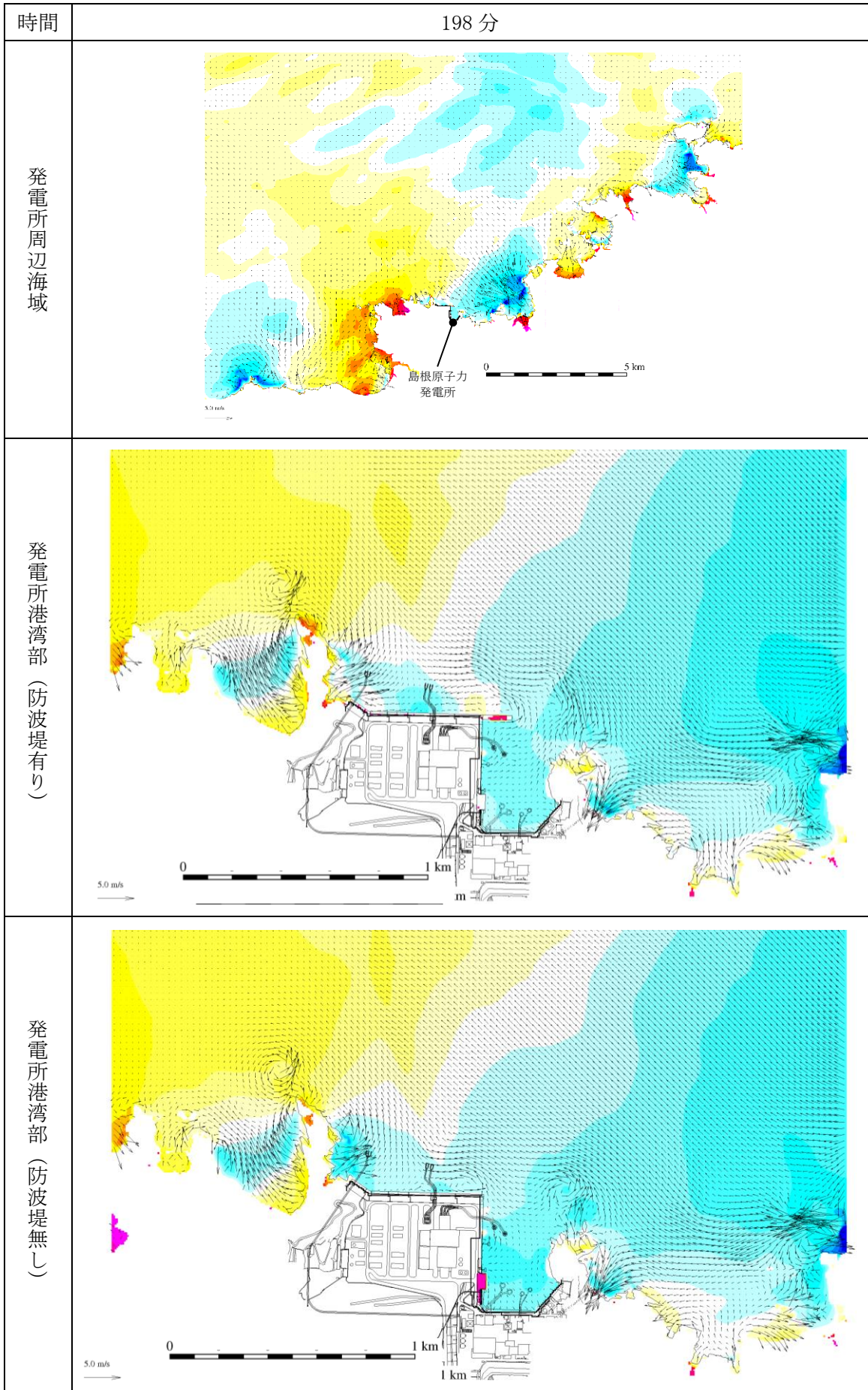
図 1-197 基準津波 1 の水位変動・流向ベクトル
