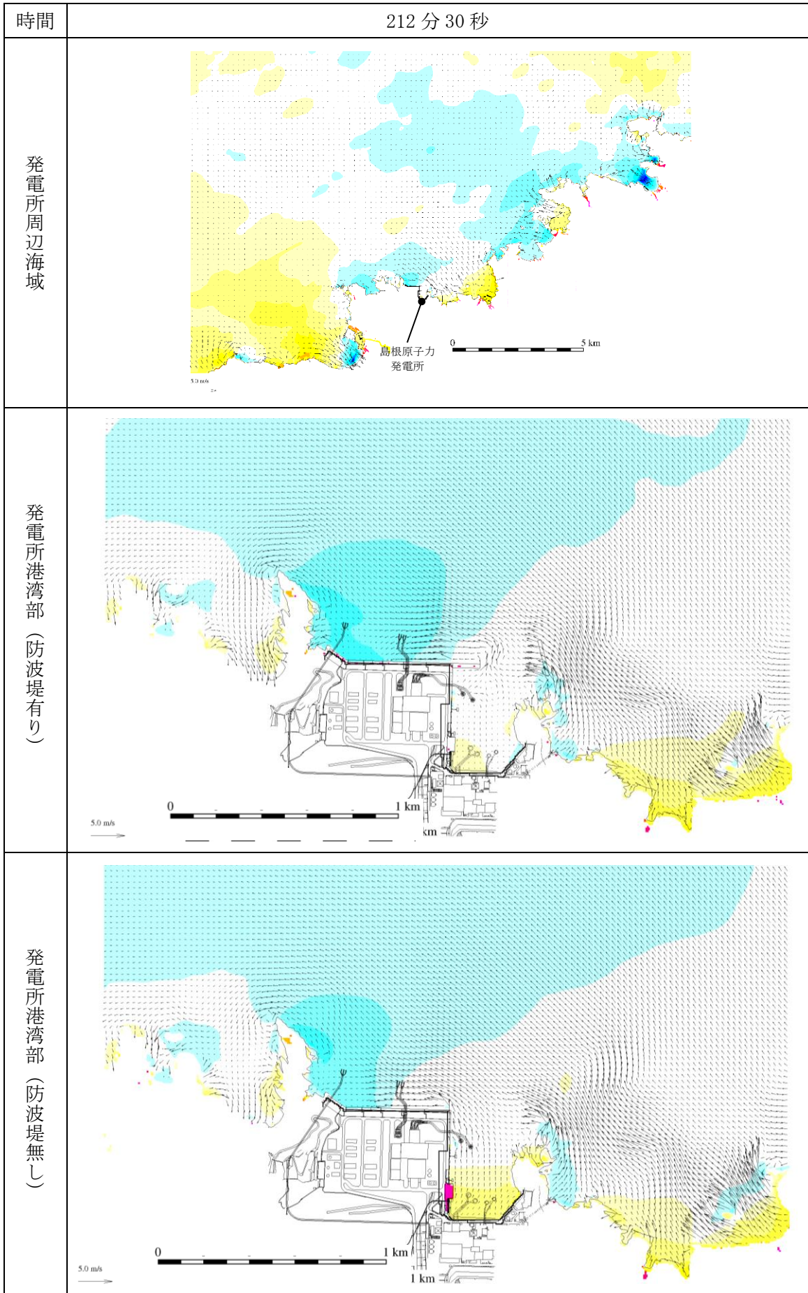
図 1-226 基準津波 1 の水位変動・流向ベクトル
