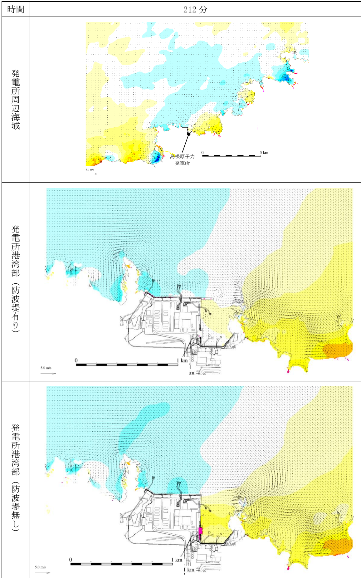
図 1-225 基準津波 1 の水位変動・流向ベクトル
