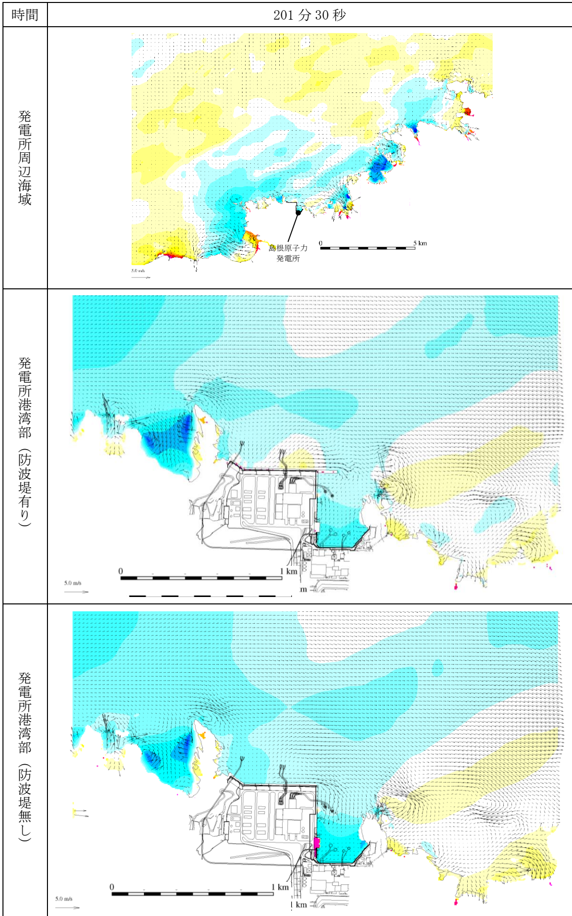
図 1-204 基準津波 1 の水位変動・流向ベクトル
