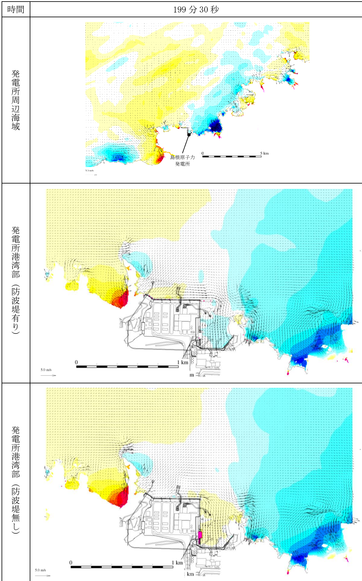
図 1-200 基準津波 1 の水位変動・流向ベクトル
