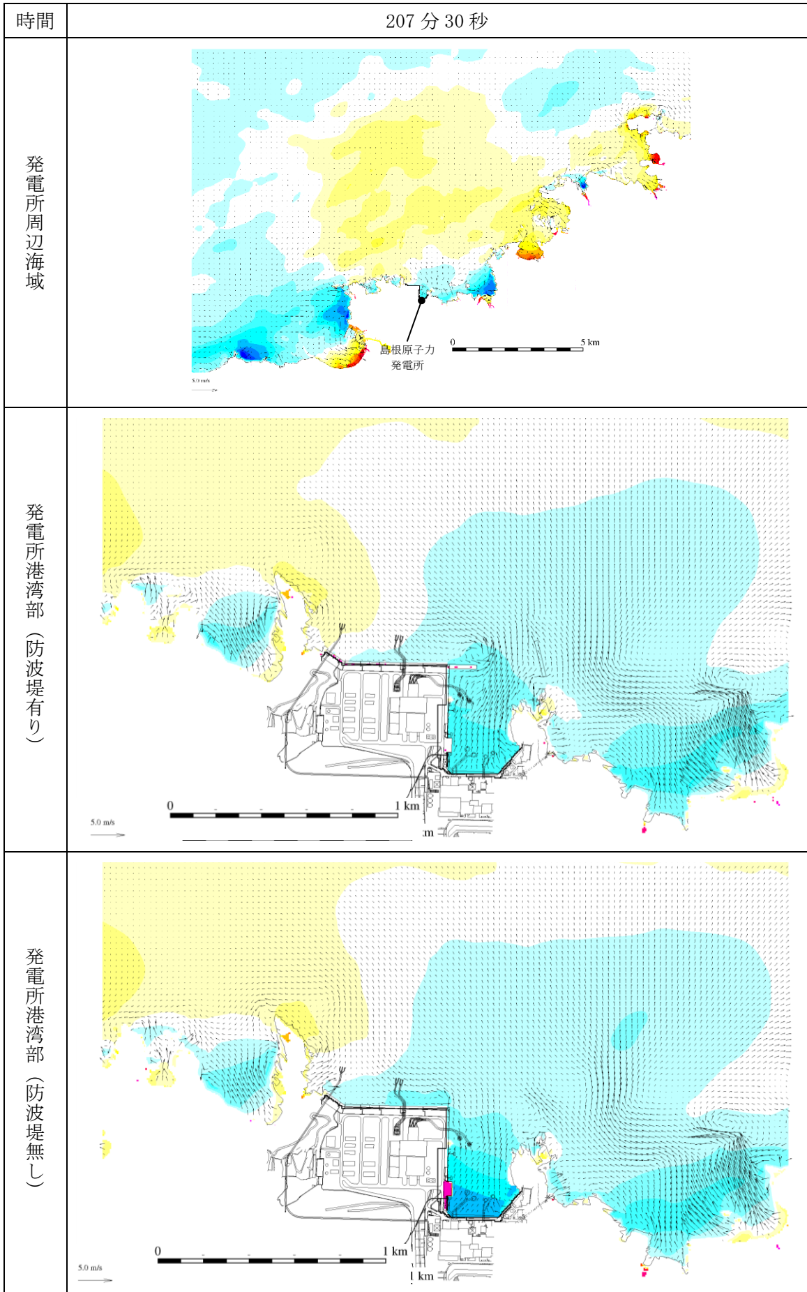
図 1-216 基準津波 1 の水位変動・流向ベクトル
