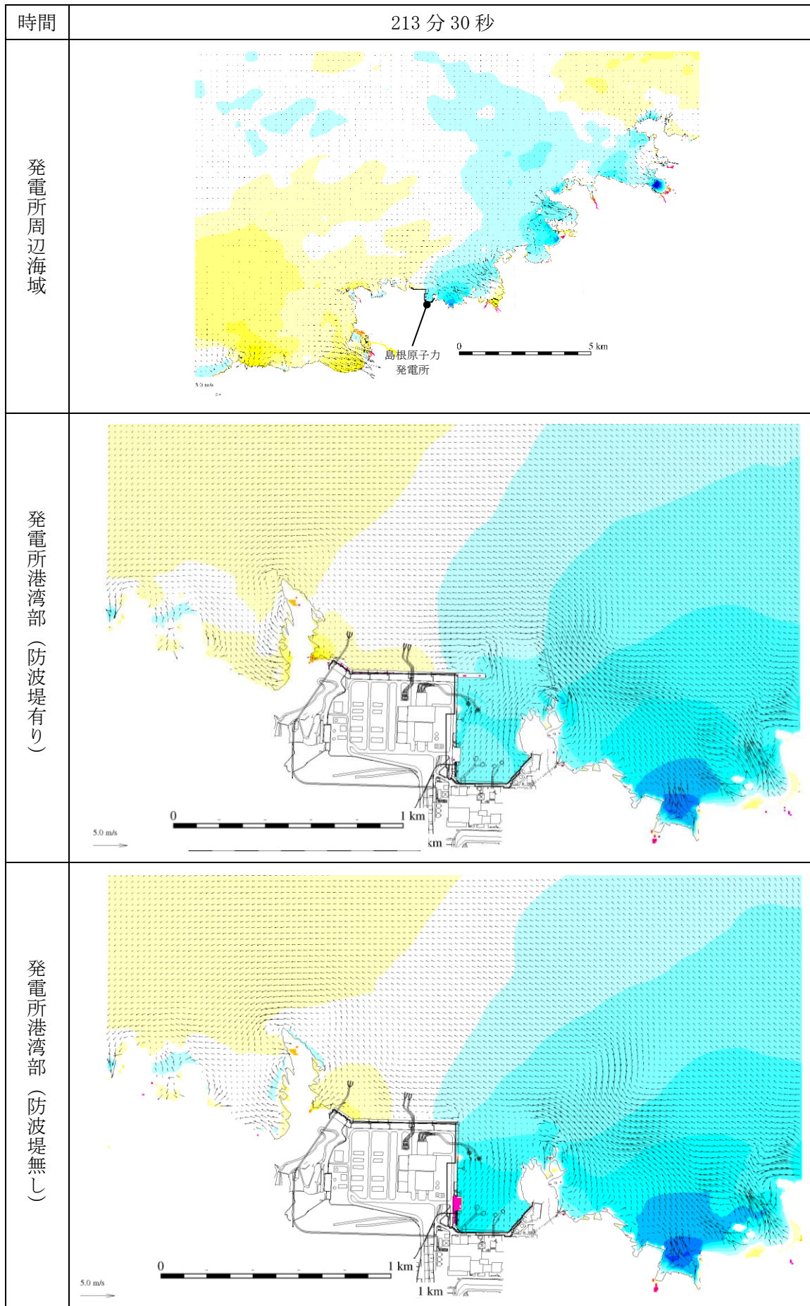
図 1-228 基準津波 1 の水位変動・流向ベクトル
