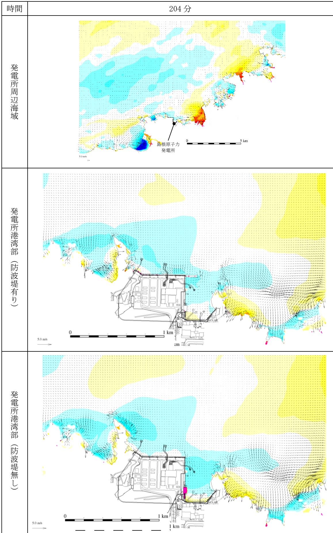
図 1-209 基準津波 1 の水位変動・流向ベクトル
