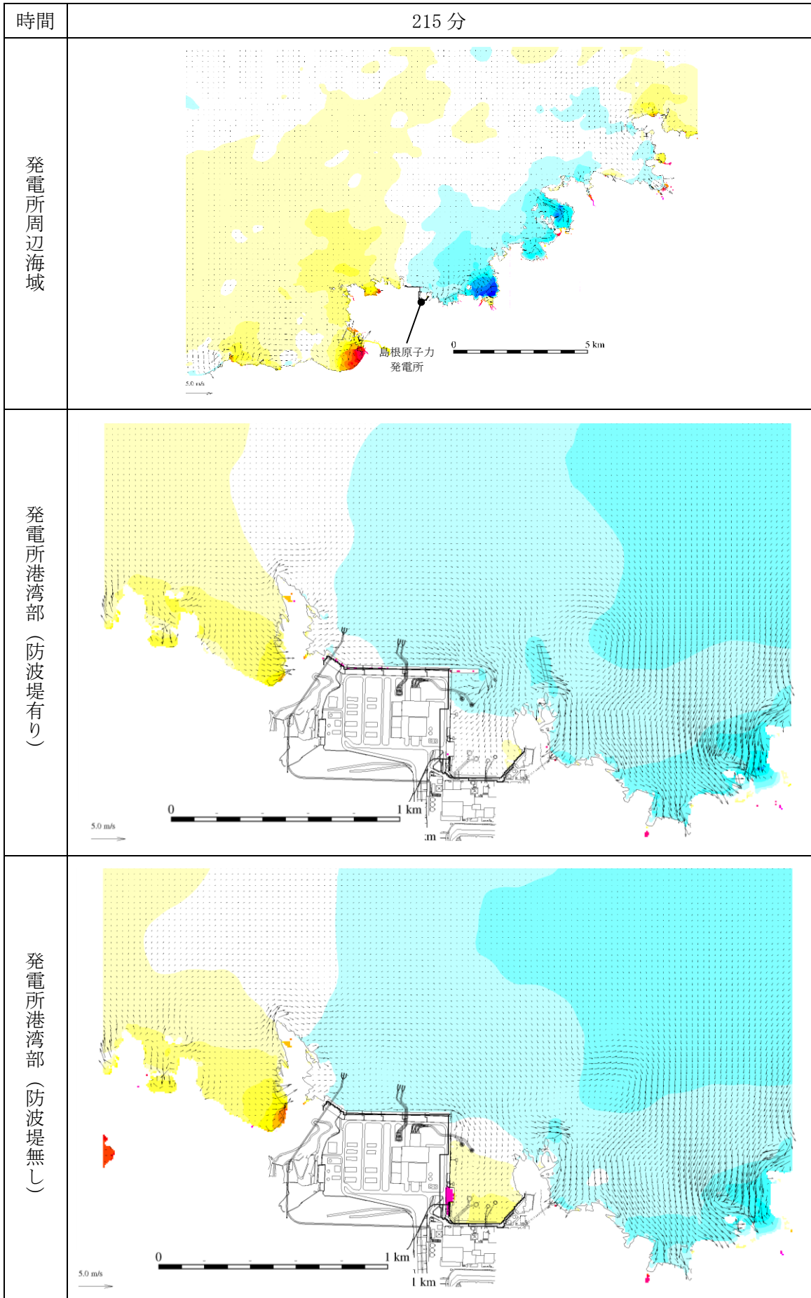
図 1-231 基準津波 1 の水位変動・流向ベクトル
