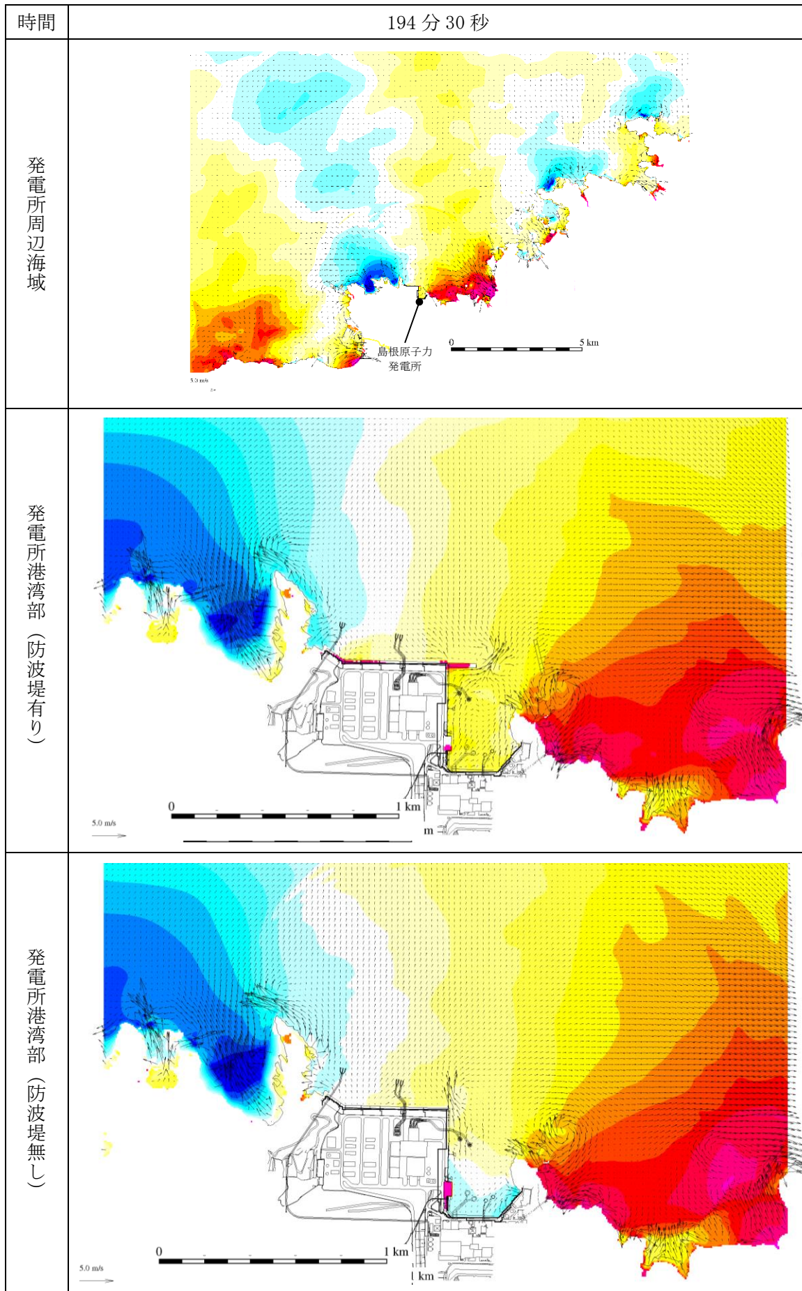
図 1-190 基準津波 1 の水位変動・流向ベクトル
