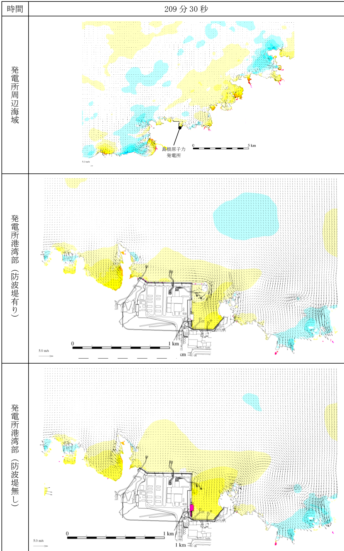
図 1-220 基準津波 1 の水位変動・流向ベクトル
