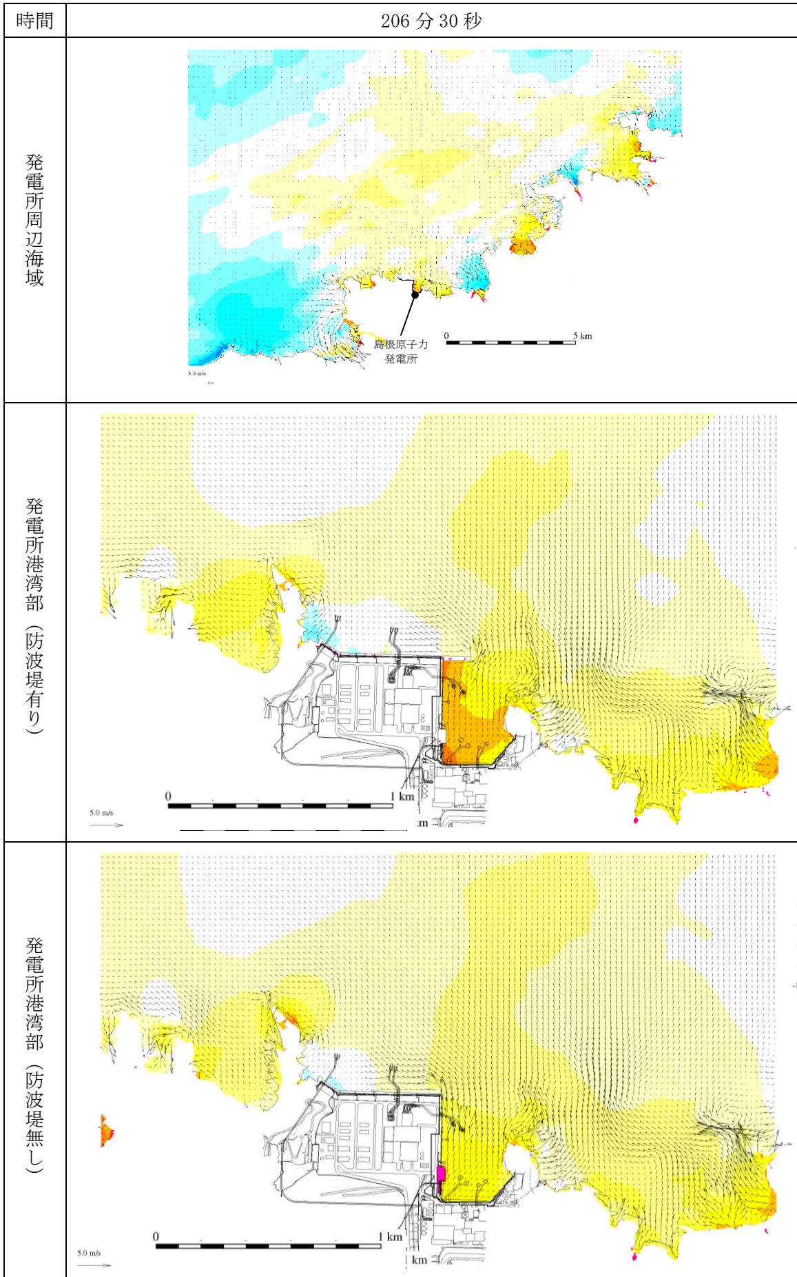
図 1-214 基準津波 1 の水位変動・流向ベクトル
