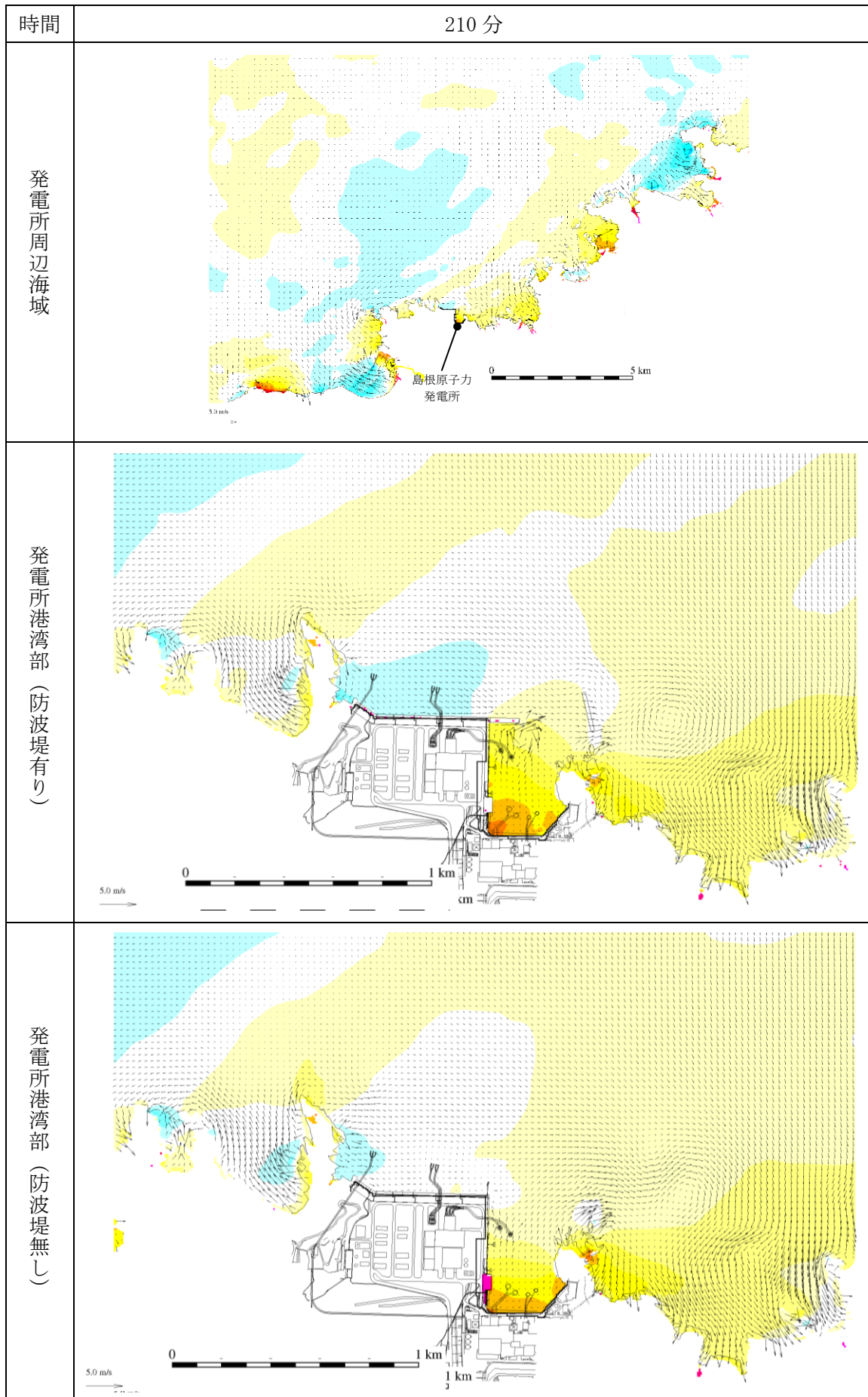
図 1-221 基準津波 1 の水位変動・流向ベクトル
