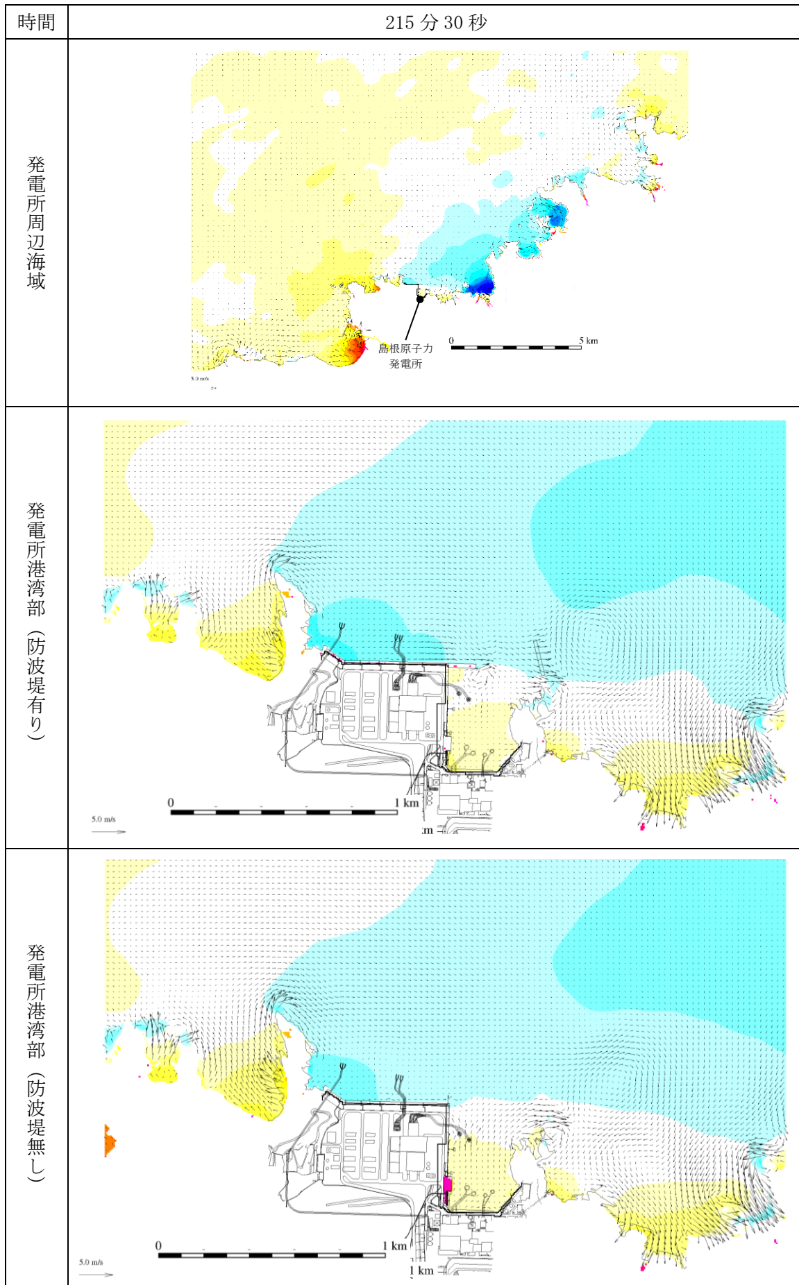
図 1-232 基準津波 1 の水位変動・流向ベクトル
