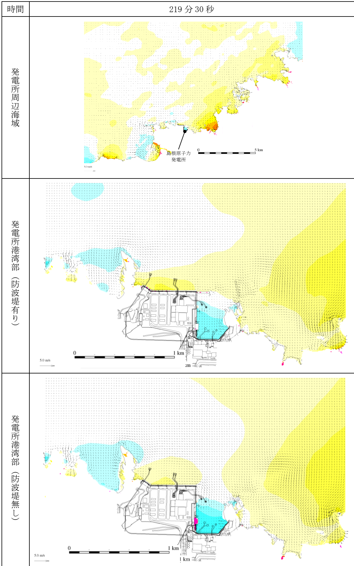
図 1-240 基準津波 1 の水位変動・流向ベクトル
