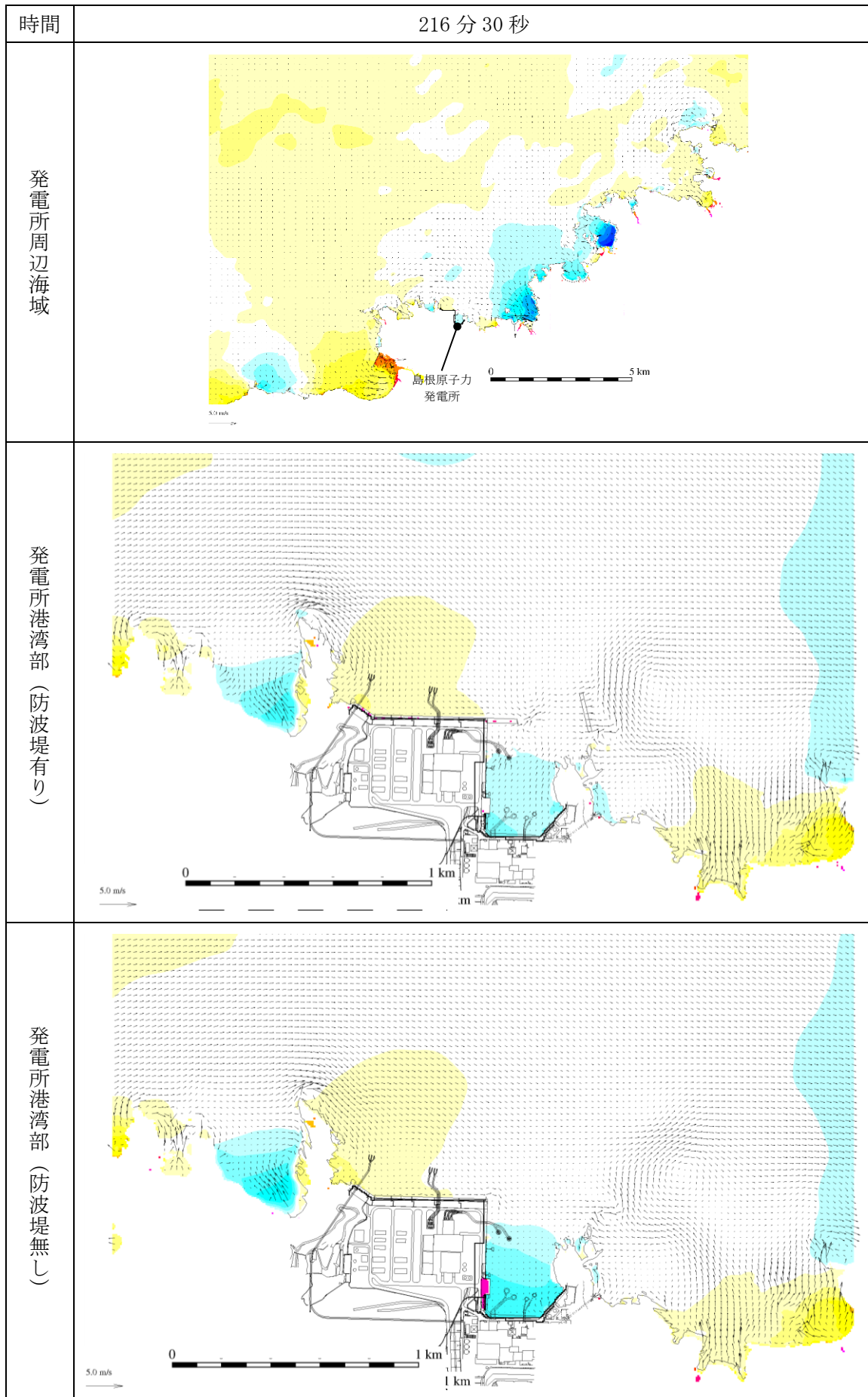
図 1-234 基準津波 1 の水位変動・流向ベクトル
