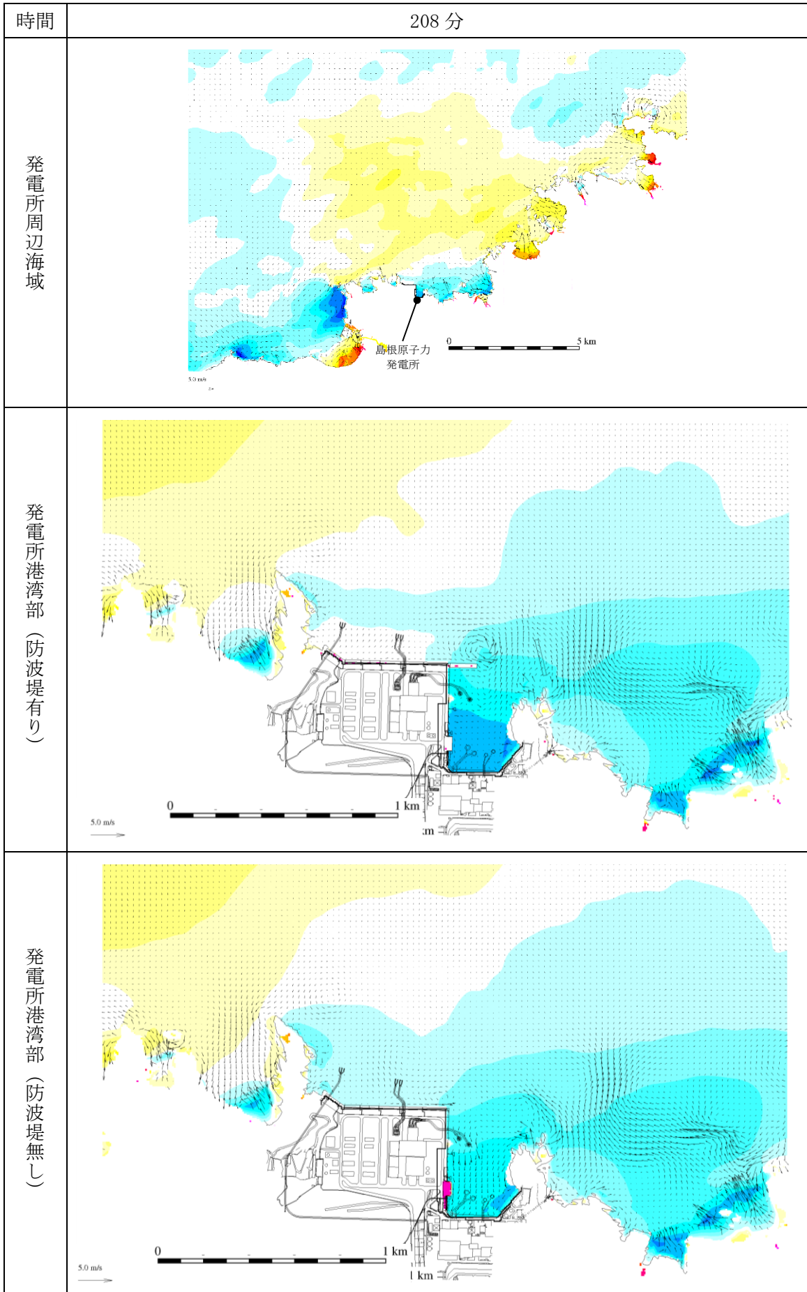
図 1-217 基準津波 1 の水位変動・流向ベクトル
