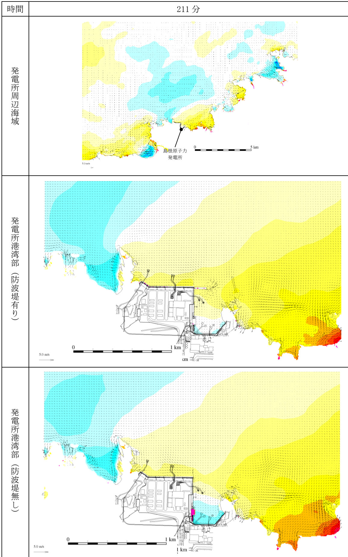
図 1-223 基準津波 1 の水位変動・流向ベクトル
