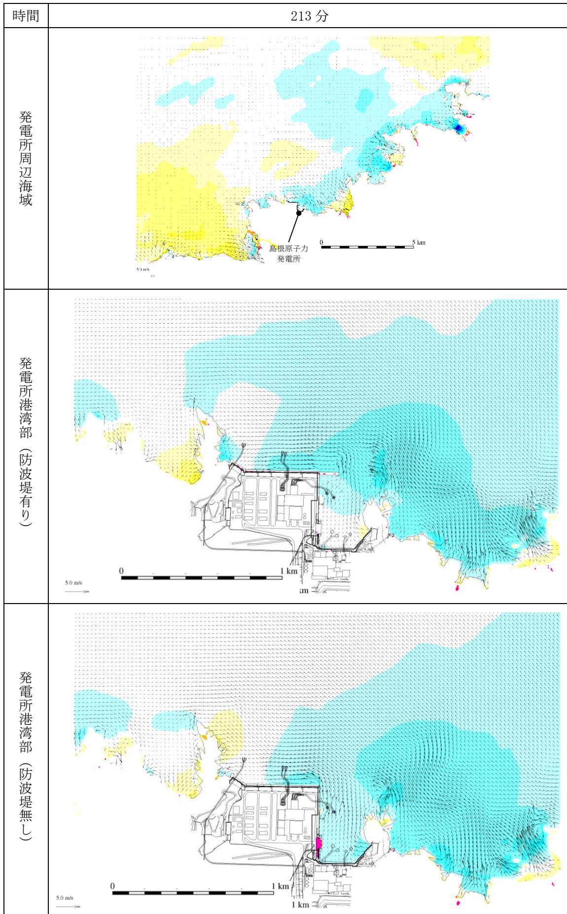
図 1-227 基準津波 1 の水位変動・流向ベクトル
