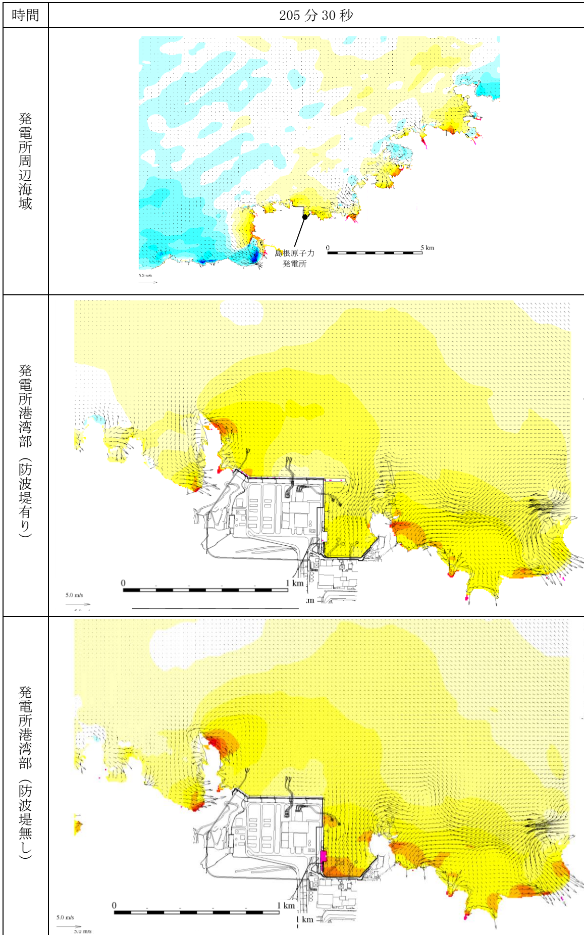
図 1-212 基準津波 1 の水位変動・流向ベクトル
