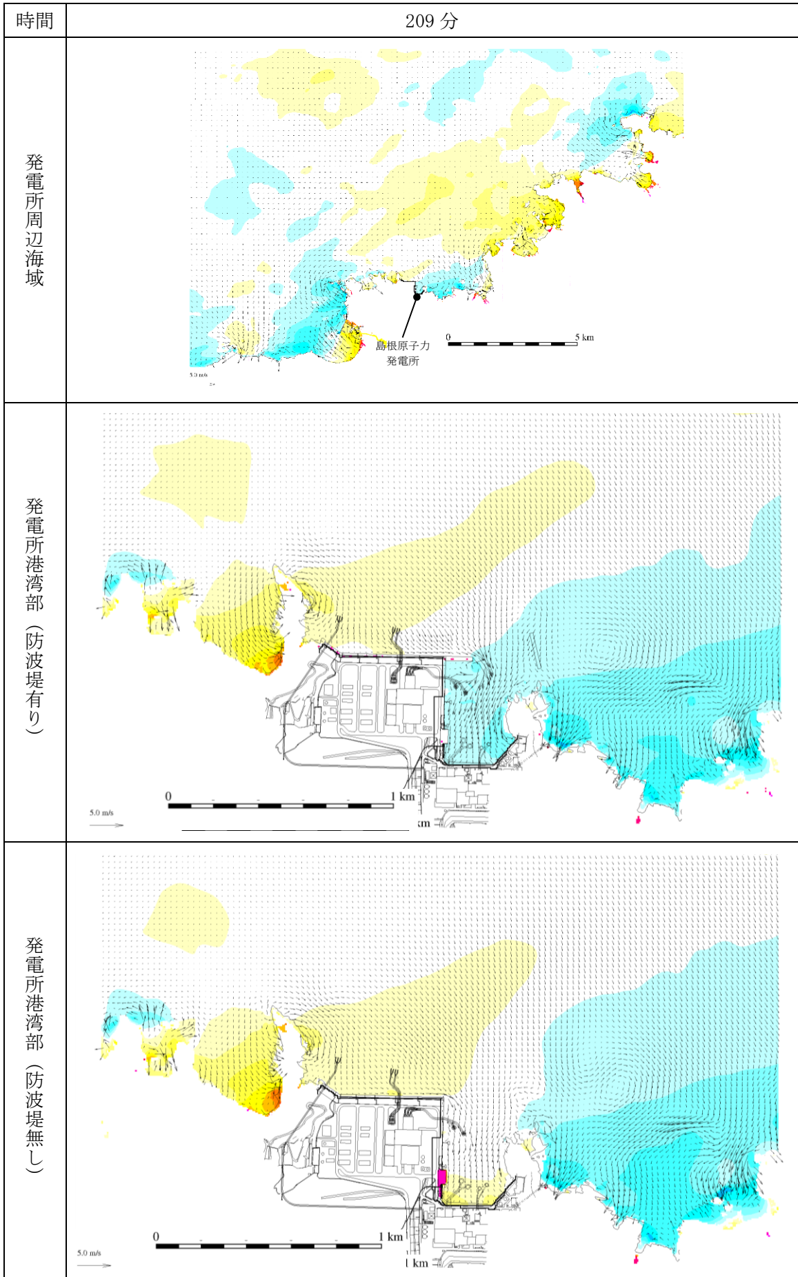
図 1-219 基準津波 1 の水位変動・流向ベクトル
