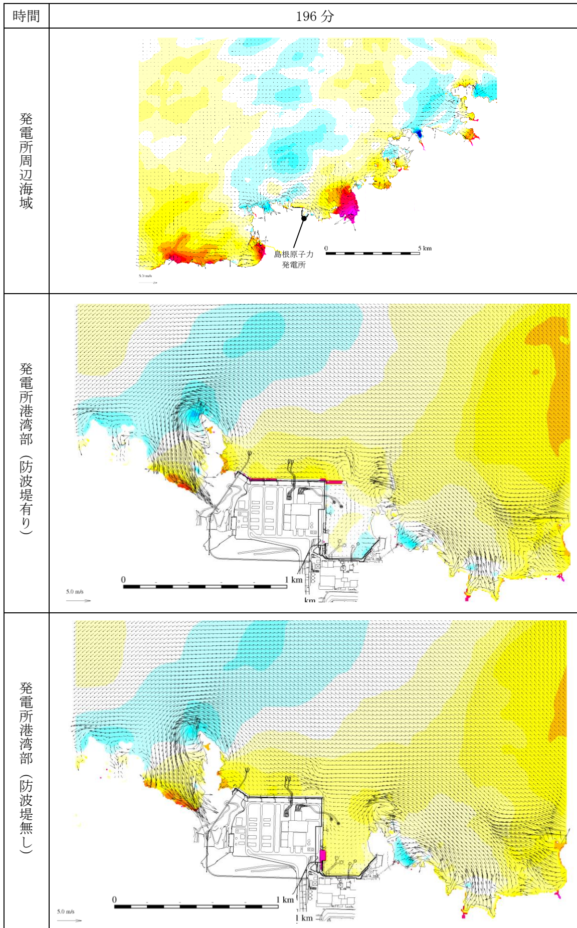
図 1-193 基準津波 1 の水位変動・流向ベクトル
