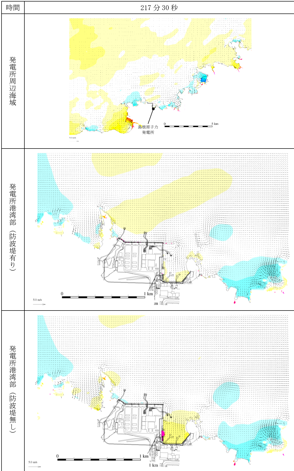
図 1-236 基準津波 1 の水位変動・流向ベクトル
