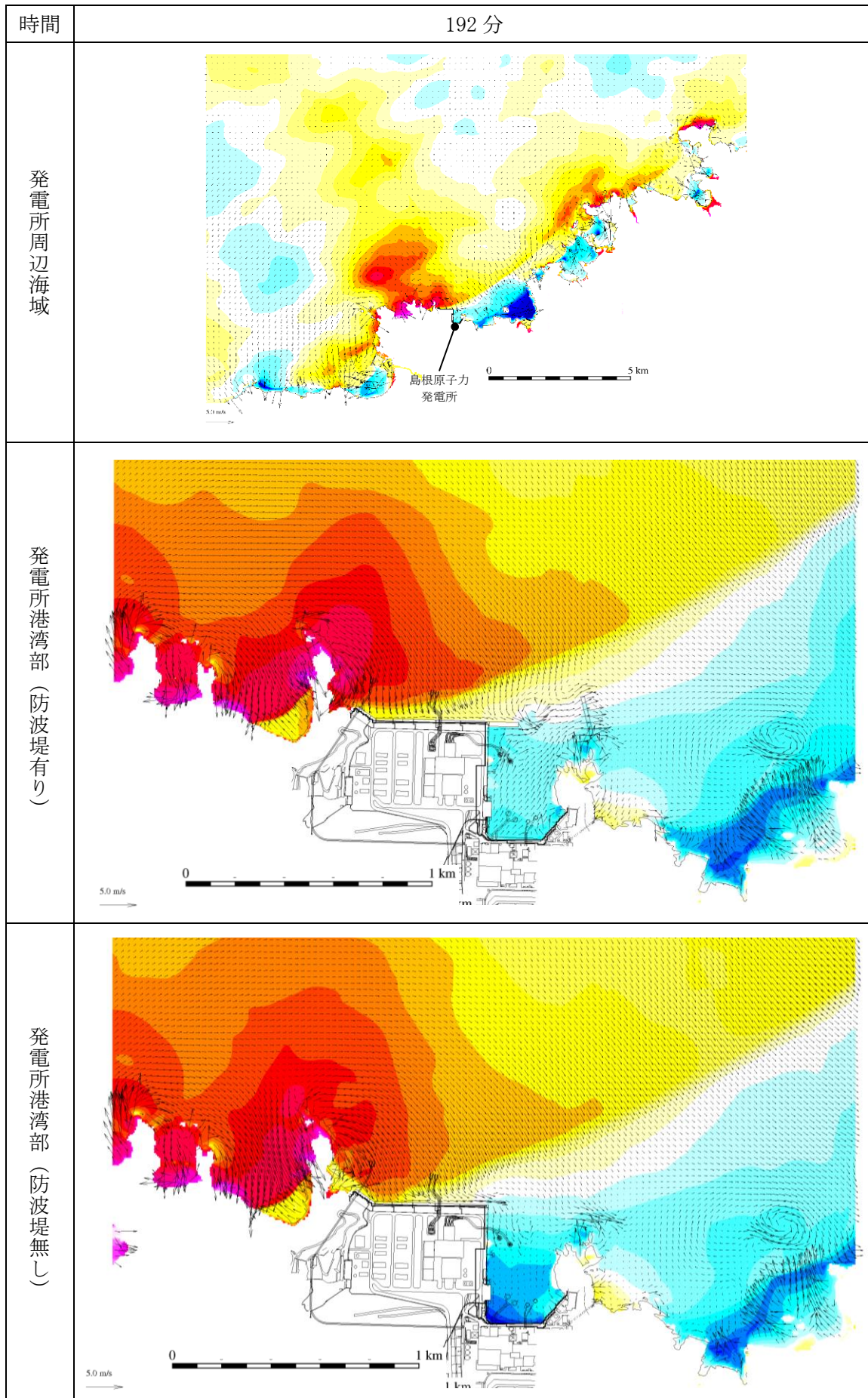
図 1-185 基準津波 1 の水位変動・流向ベクトル
