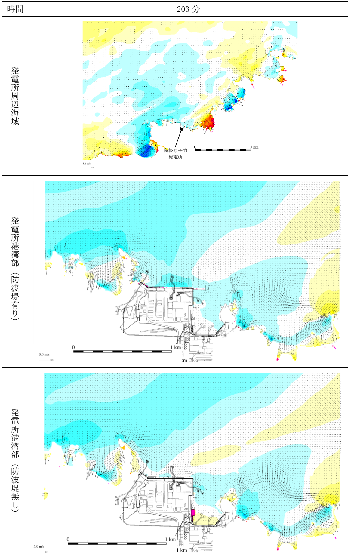
図 1-207 基準津波 1 の水位変動・流向ベクトル
