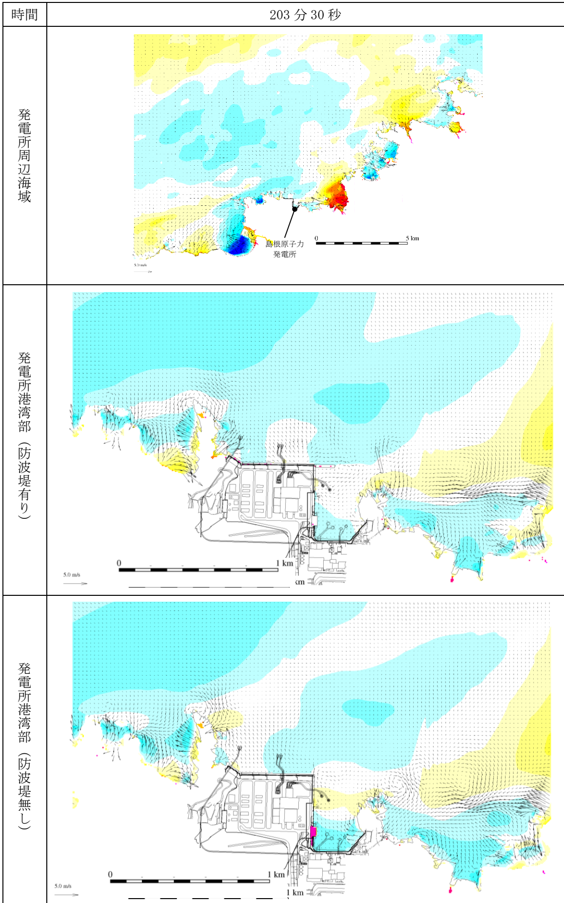
図 1-208 基準津波 1 の水位変動・流向ベクトル
