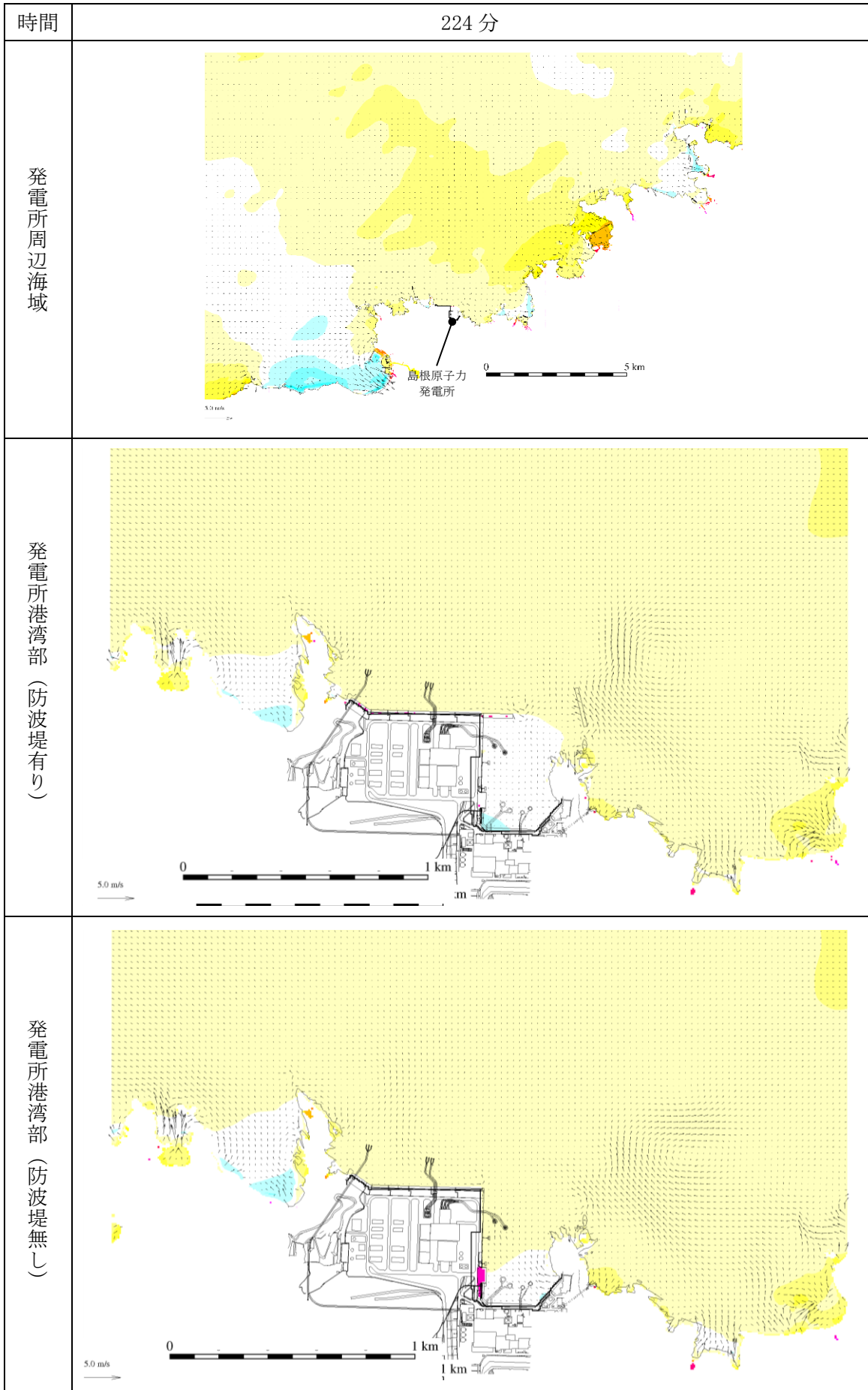
図 1-249 基準津波 1 の水位変動・流向ベクトル
