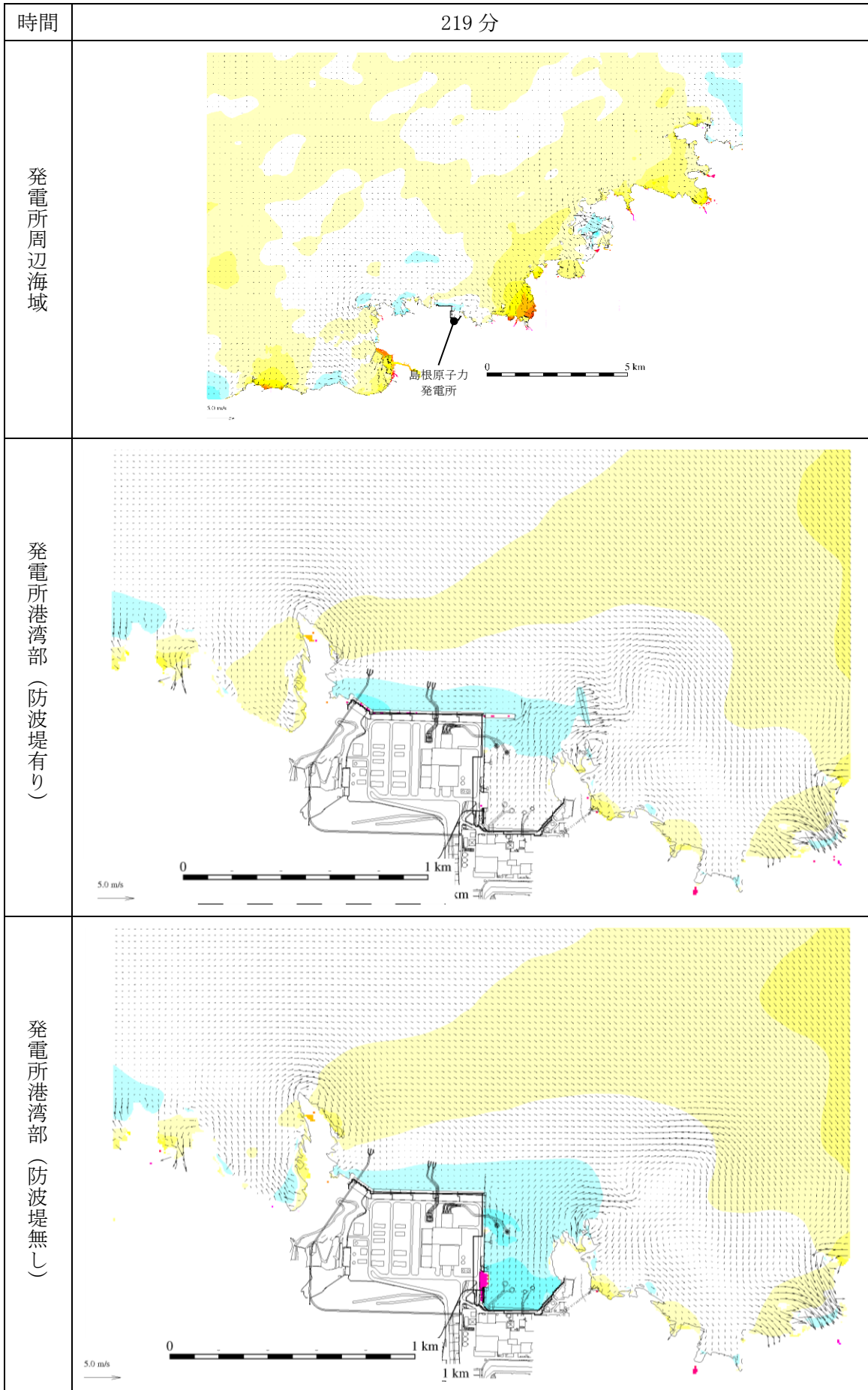
図 1-239 基準津波 1 の水位変動・流向ベクトル
