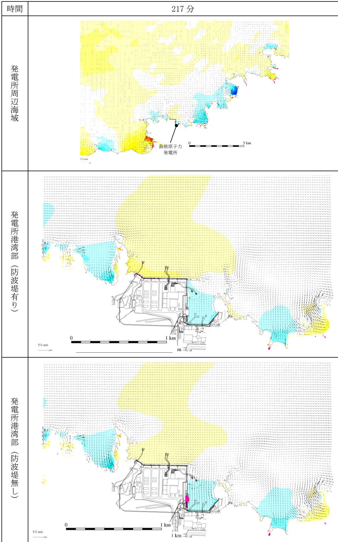
図 1-235 基準津波 1 の水位変動・流向ベクトル
