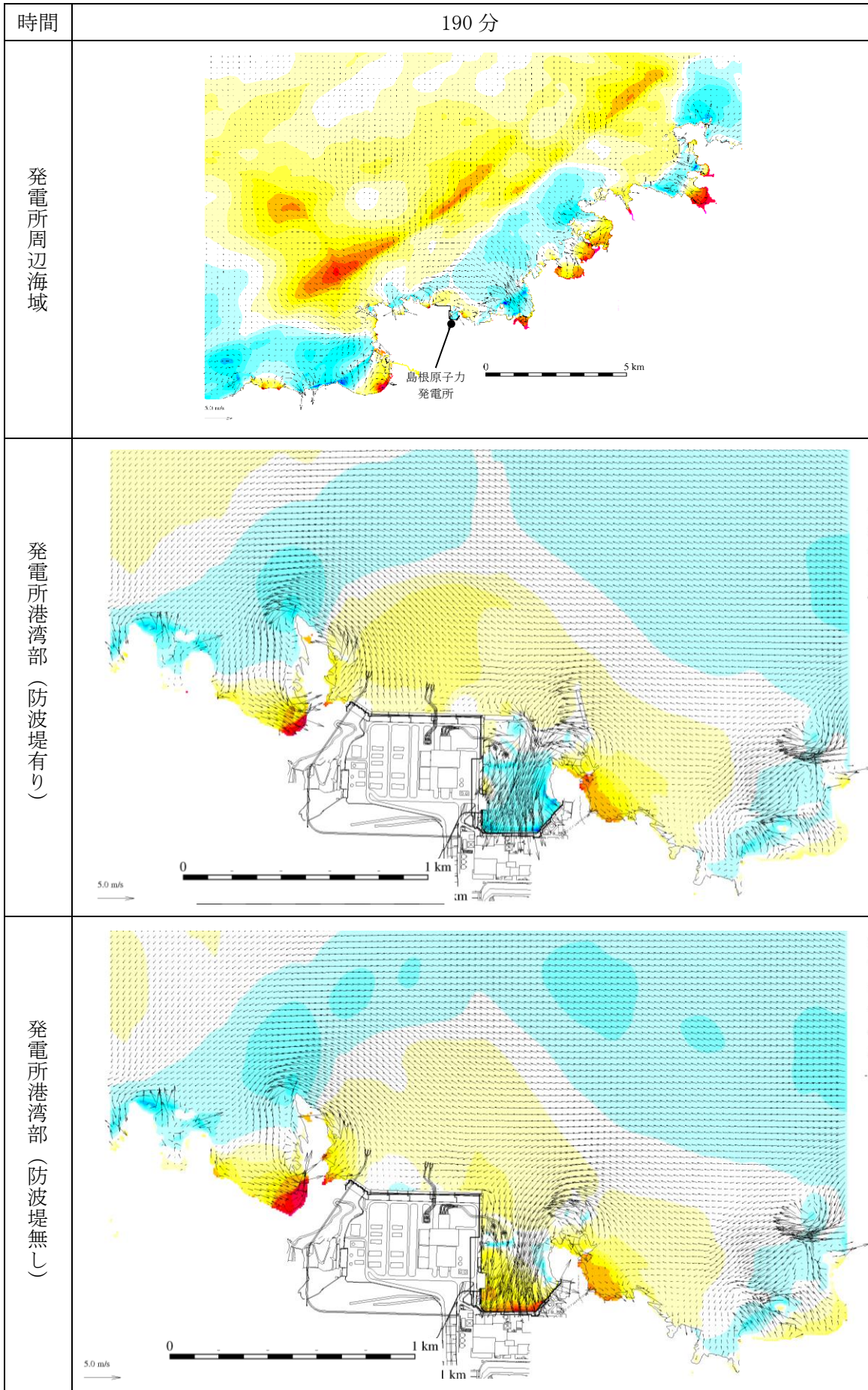
図 1-181 基準津波 1 の水位変動・流向ベクトル
