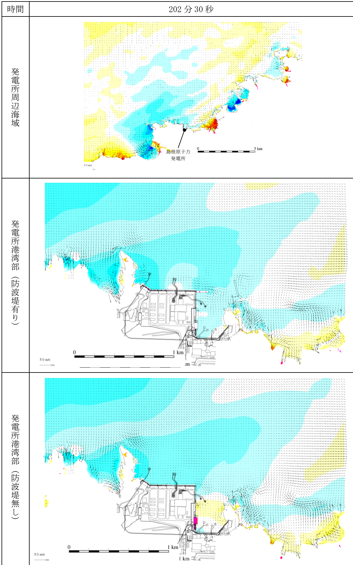
図 1-206 基準津波 1 の水位変動・流向ベクトル
