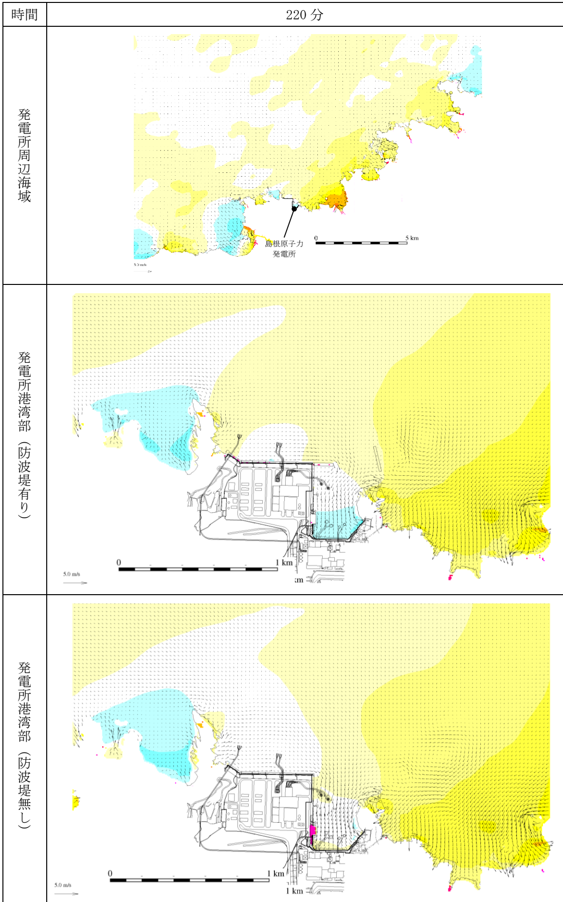
図 1-241 基準津波 1 の水位変動・流向ベクトル
