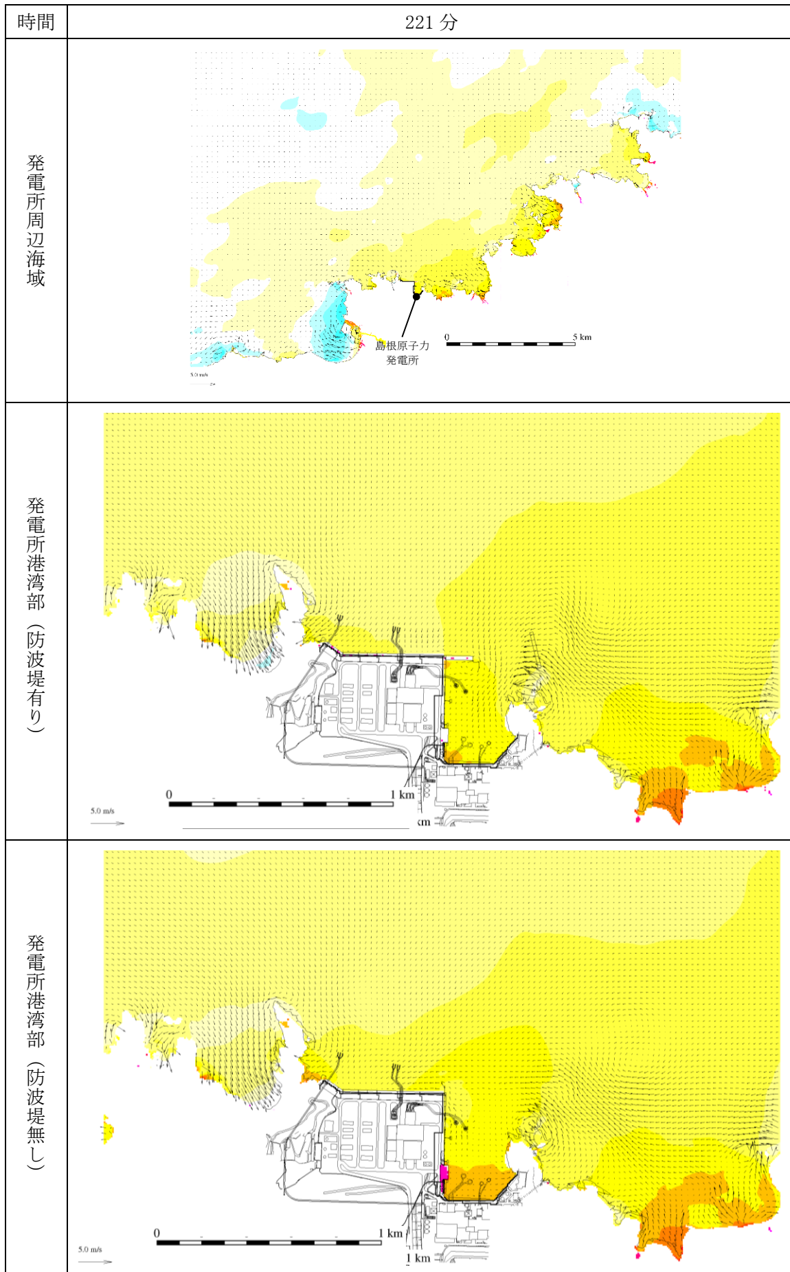
図 1-243 基準津波 1 の水位変動・流向ベクトル
