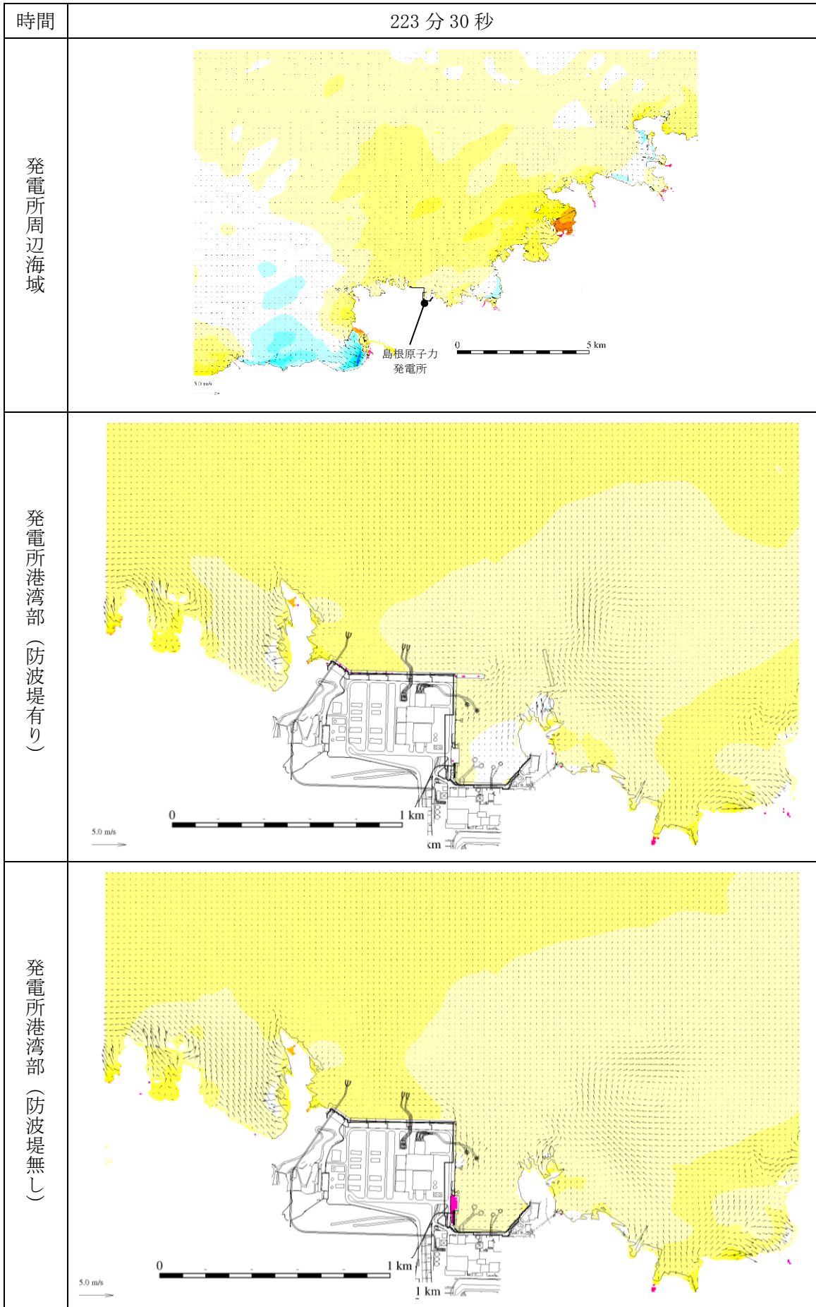
図 1-248 基準津波 1 の水位変動・流向ベクトル
