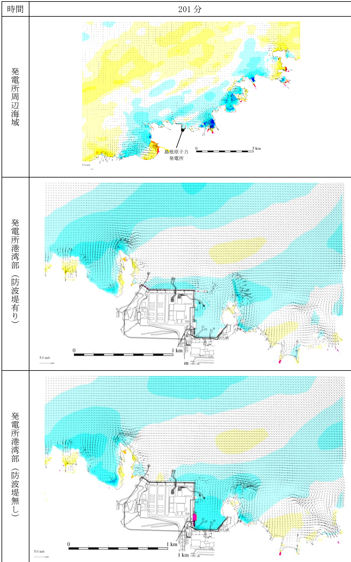
図 1-203 基準津波 1 の水位変動・流向ベクトル
