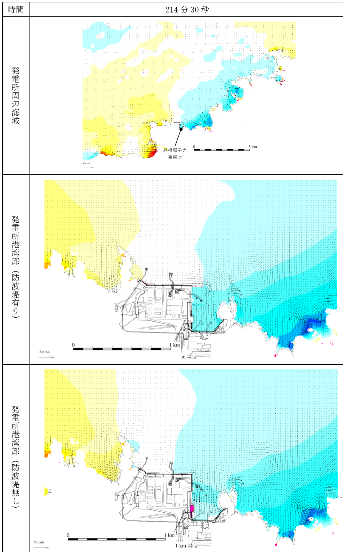
図 1-230 基準津波 1 の水位変動・流向ベクトル
