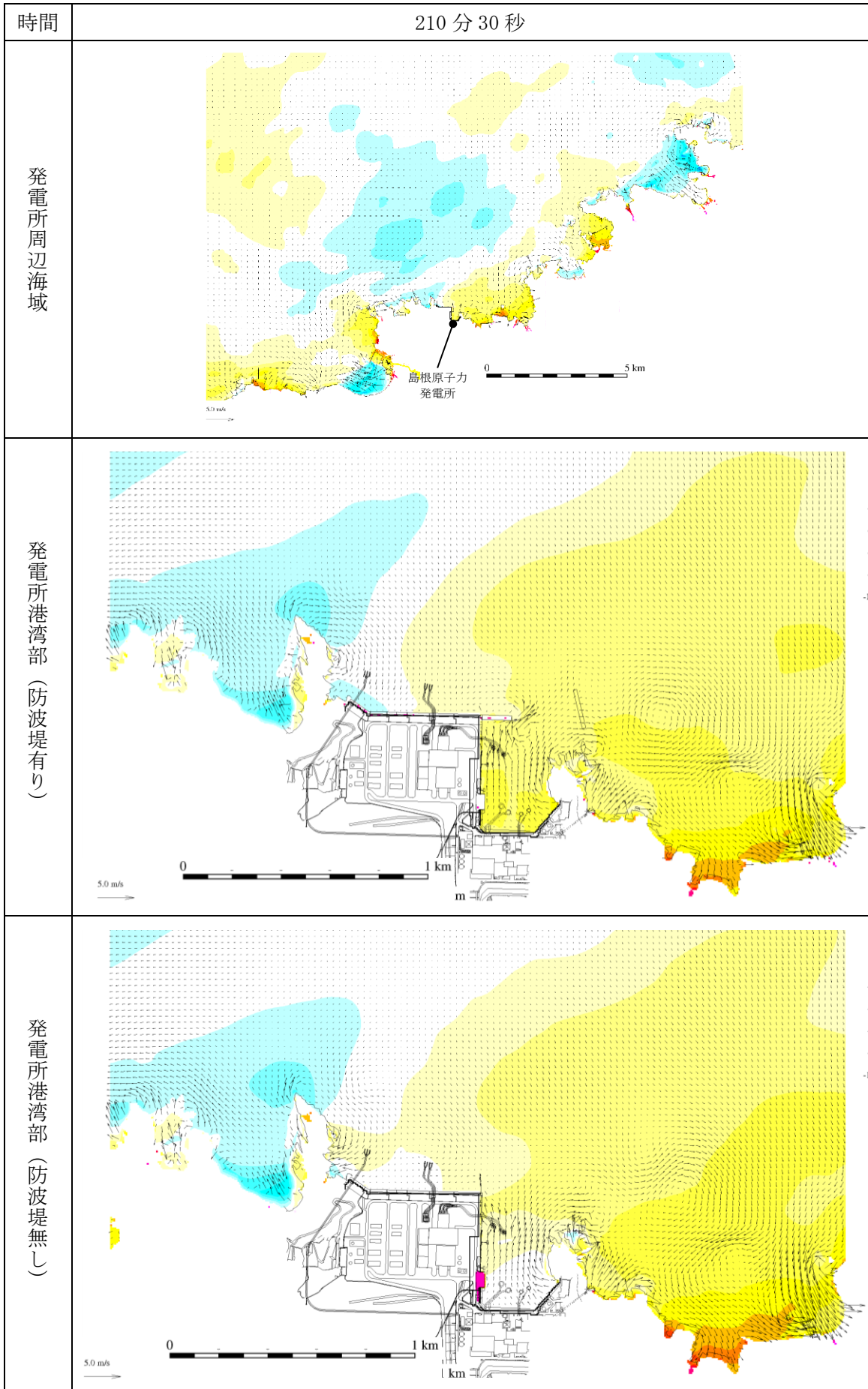
図 1-222 基準津波 1 の水位変動・流向ベクトル
