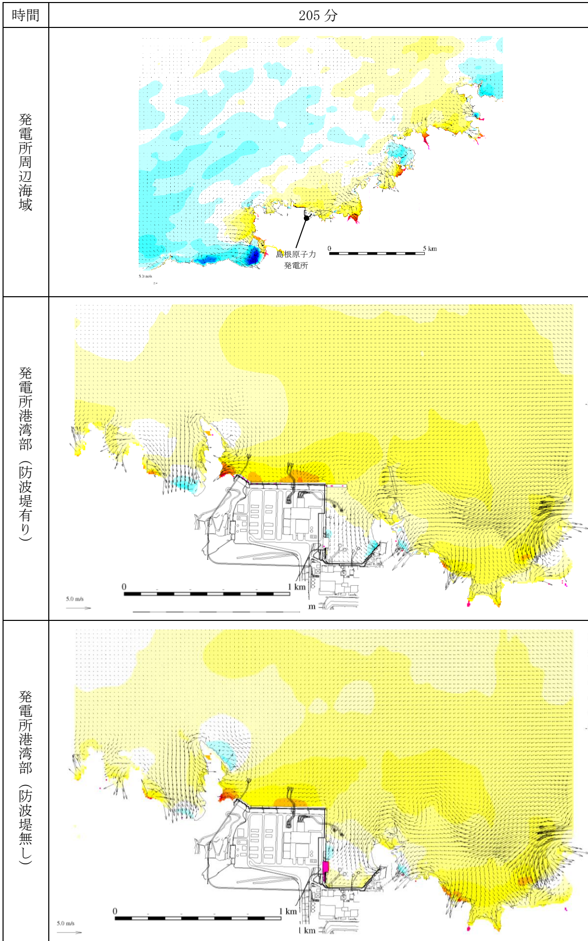
図 1-211 基準津波 1 の水位変動・流向ベクトル
