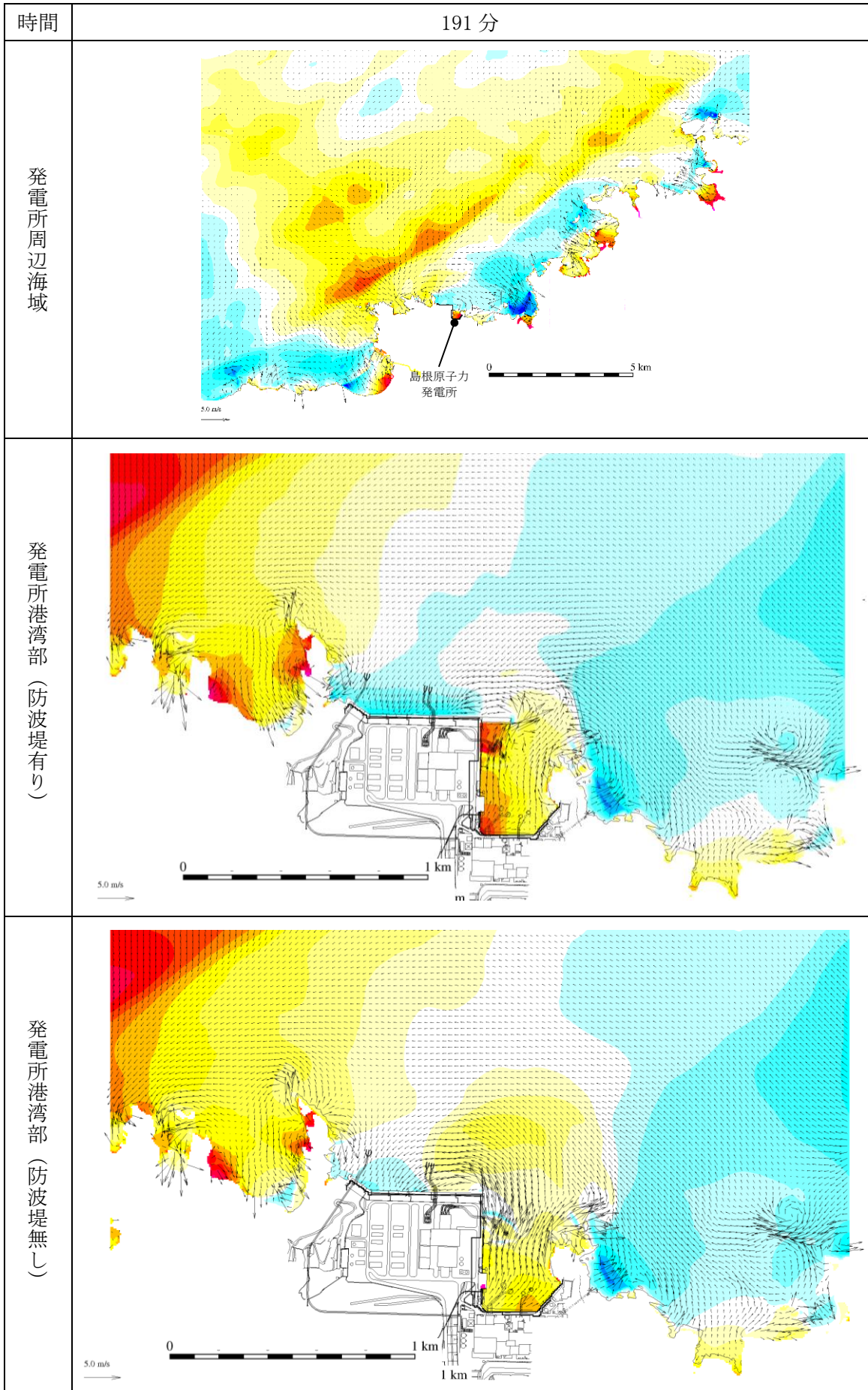
図 1-183 基準津波 1 の水位変動・流向ベクトル
