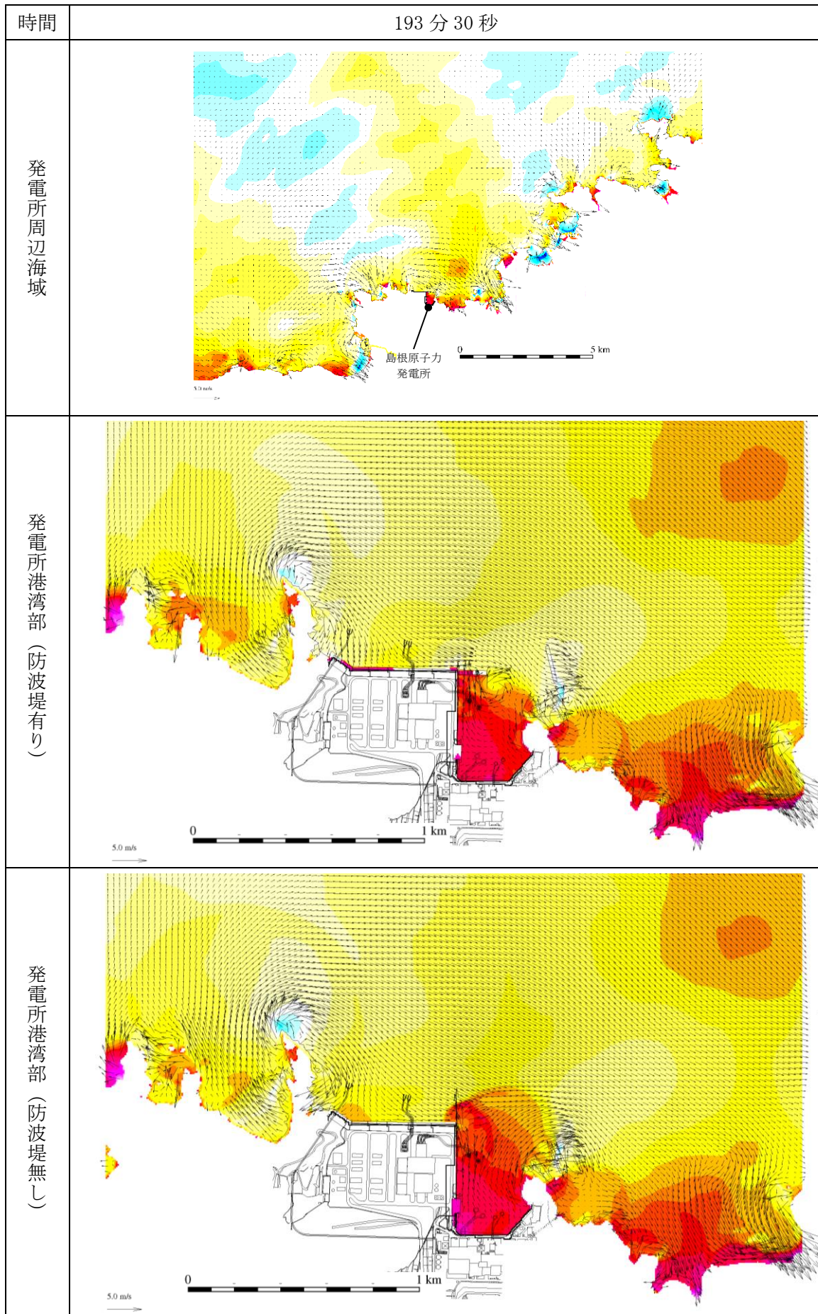
図 1-188 基準津波 1 の水位変動・流向ベクトル
