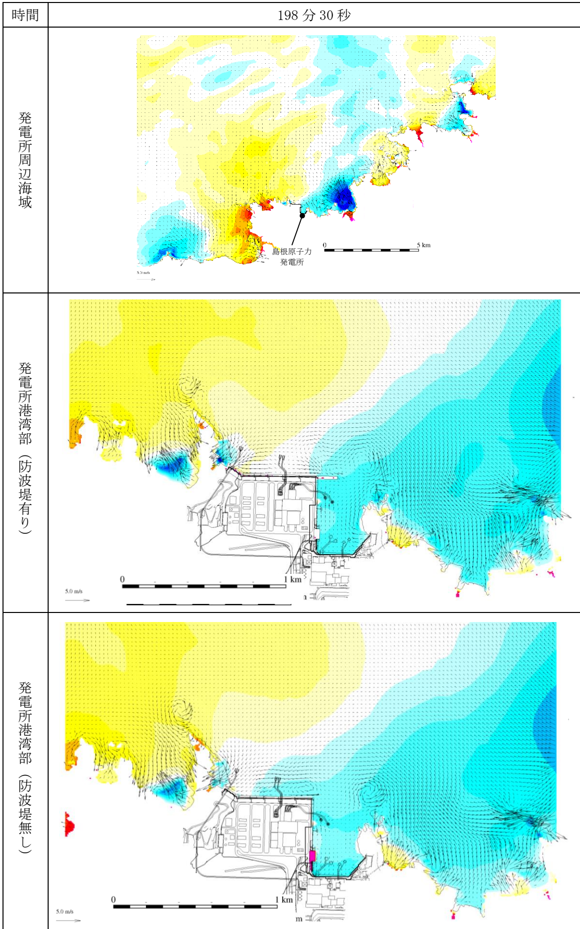
図 1-198 基準津波 1 の水位変動・流向ベクトル
