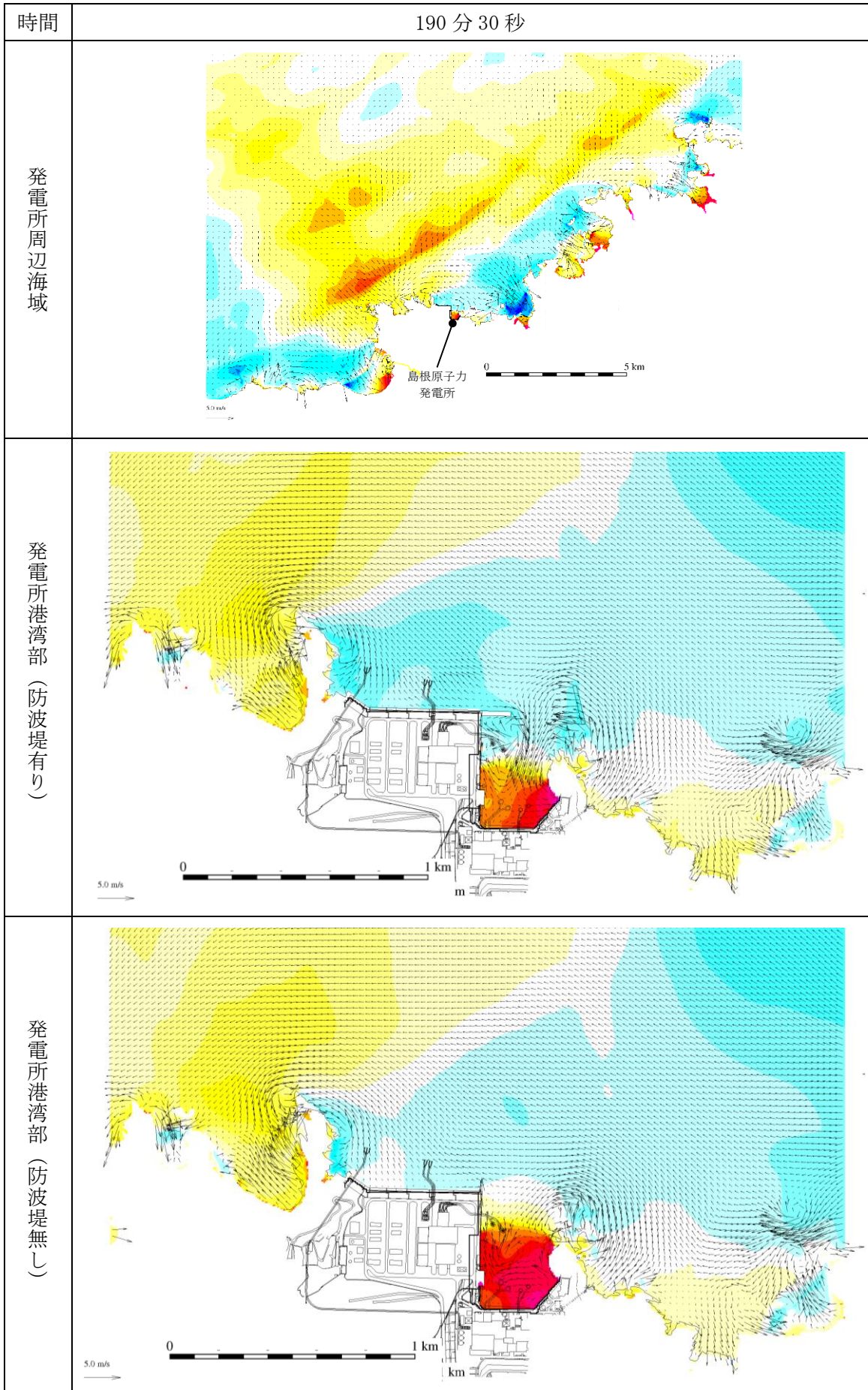
図 1-182 基準津波 1 の水位変動・流向ベクトル
