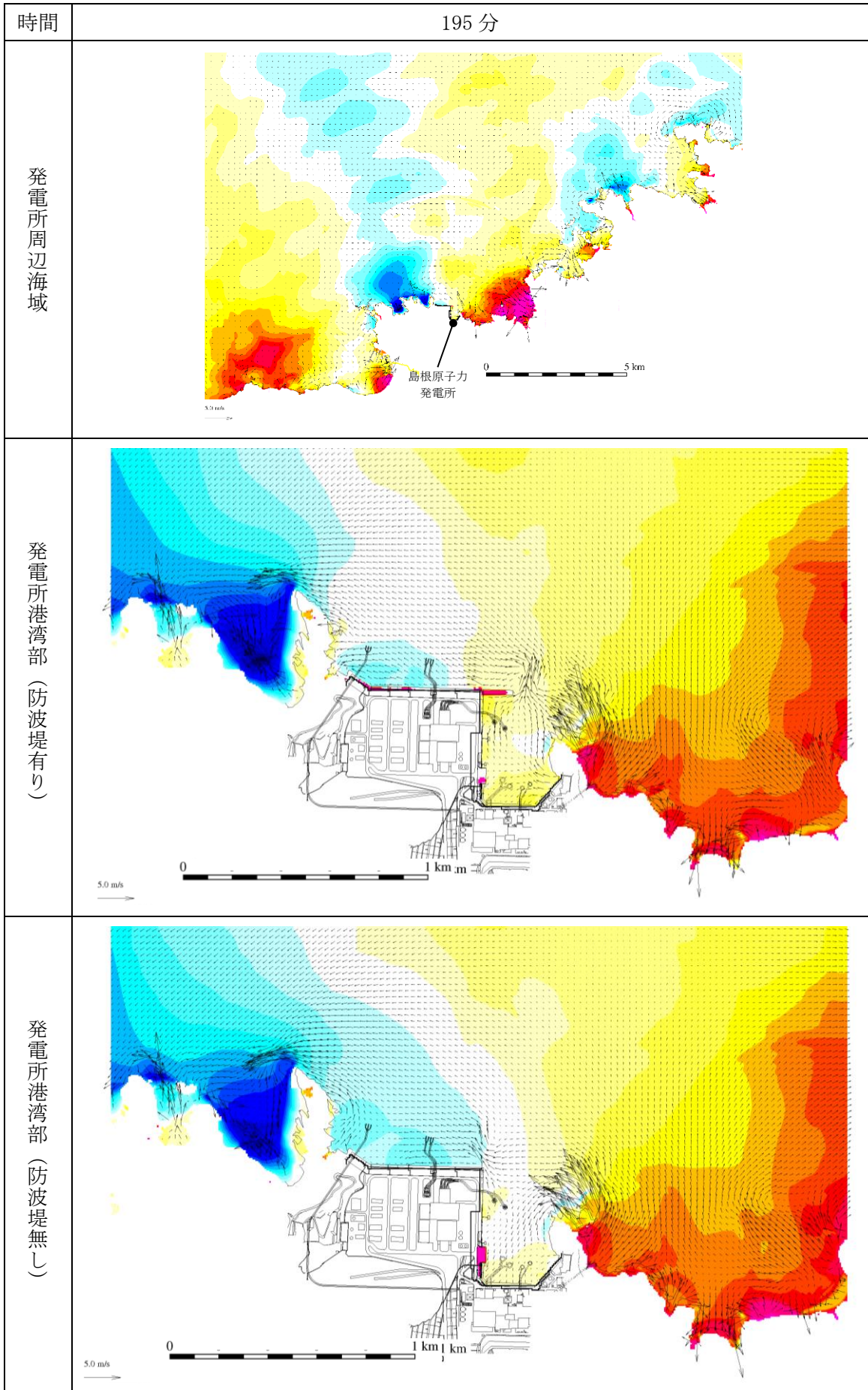
図 1-191 基準津波 1 の水位変動・流向ベクトル
