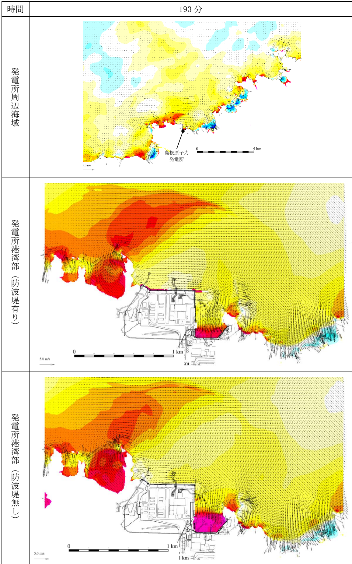
図 1-187 基準津波 1 の水位変動・流向ベクトル
