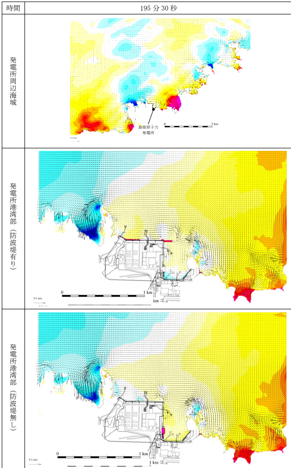
図 1-192 基準津波 1 の水位変動・流向ベクトル
