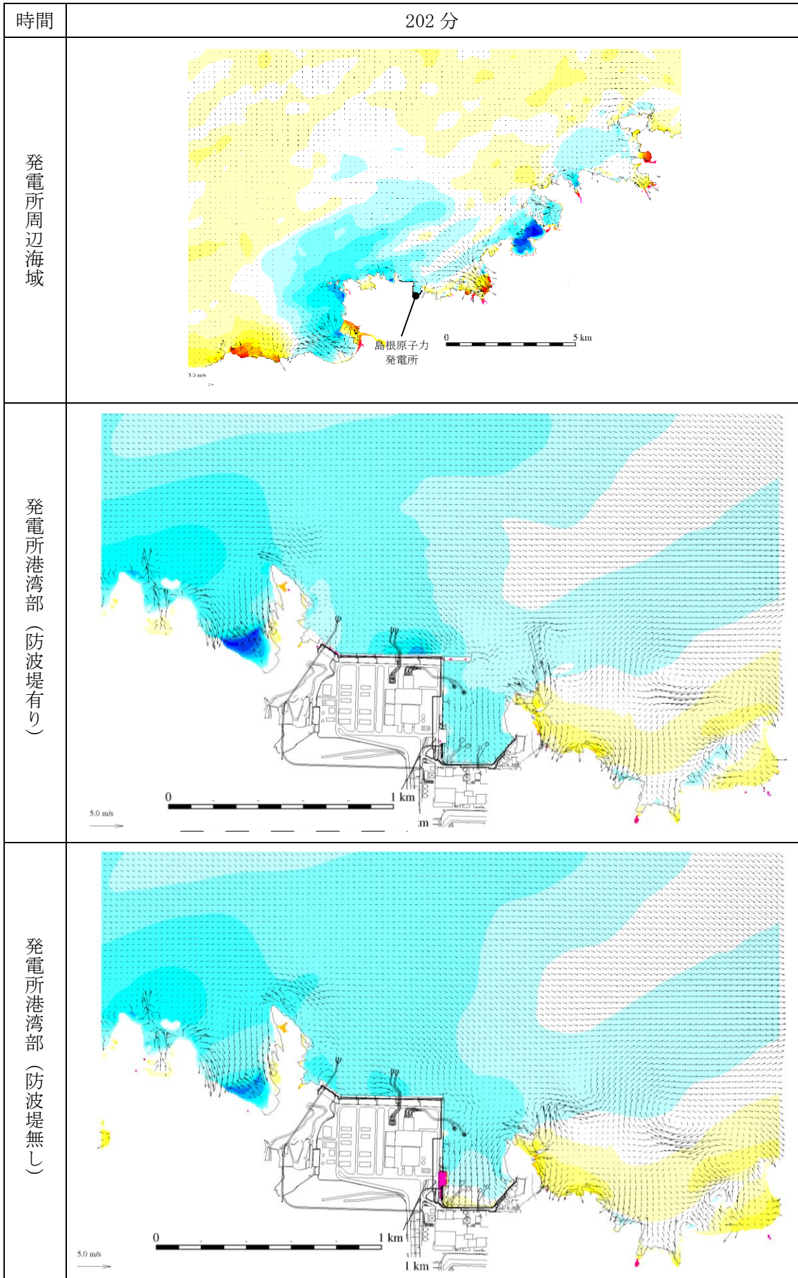
図 1-205 基準津波 1 の水位変動・流向ベクトル
