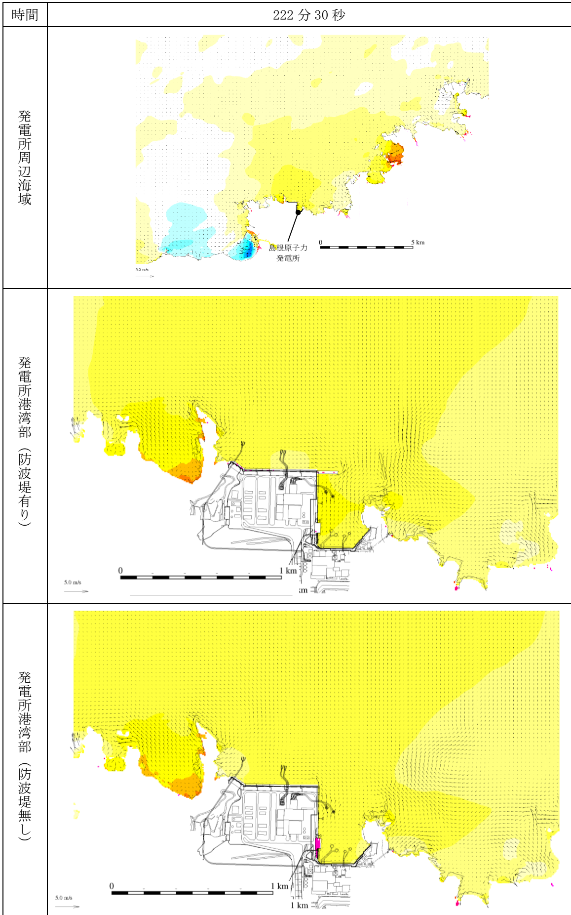
図 1-246 基準津波 1 の水位変動・流向ベクトル
