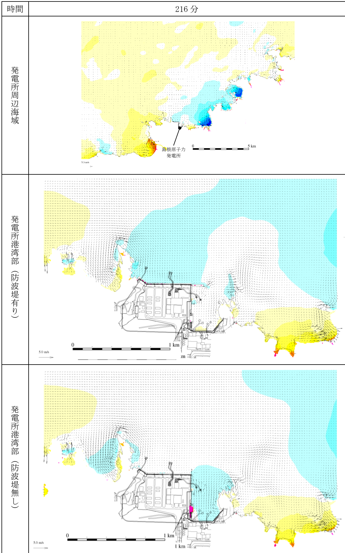
図 1-233 基準津波 1 の水位変動・流向ベクトル
