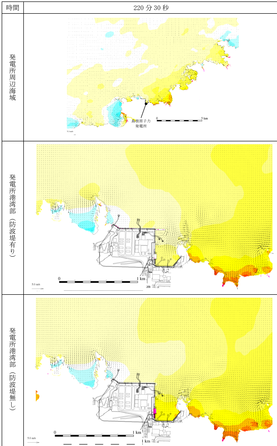
図 1-242 基準津波 1 の水位変動・流向ベクトル
