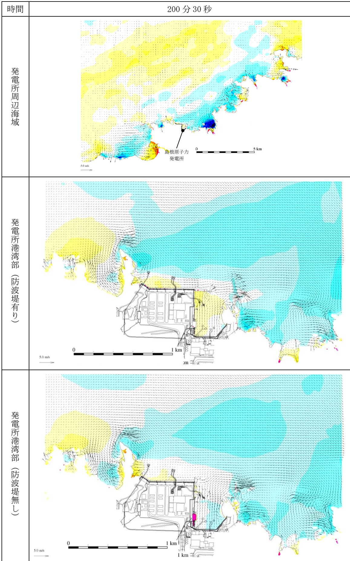
図 1-202 基準津波 1 の水位変動・流向ベクトル
