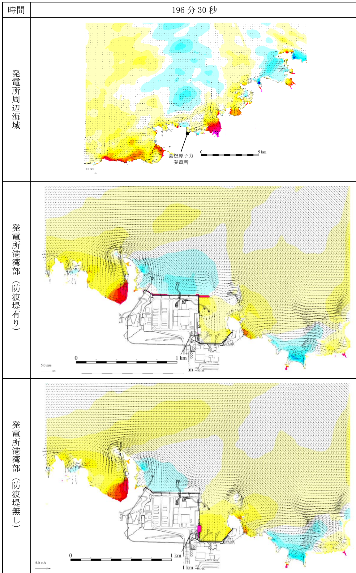
図 1-194 基準津波 1 の水位変動・流向ベクトル
