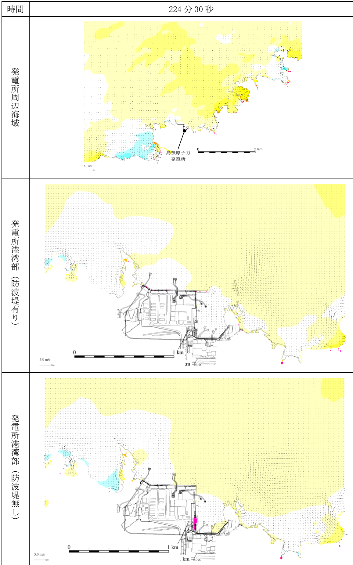
図 1-250 基準津波 1 の水位変動・流向ベクトル
