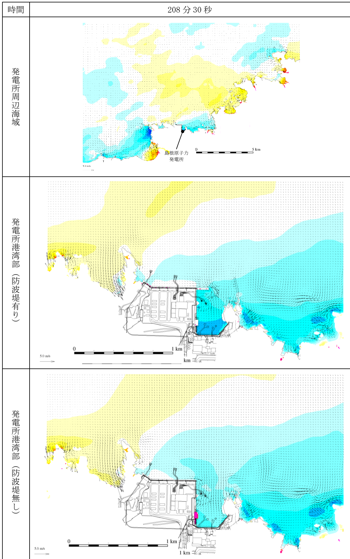
図 1-218 基準津波 1 の水位変動・流向ベクトル
