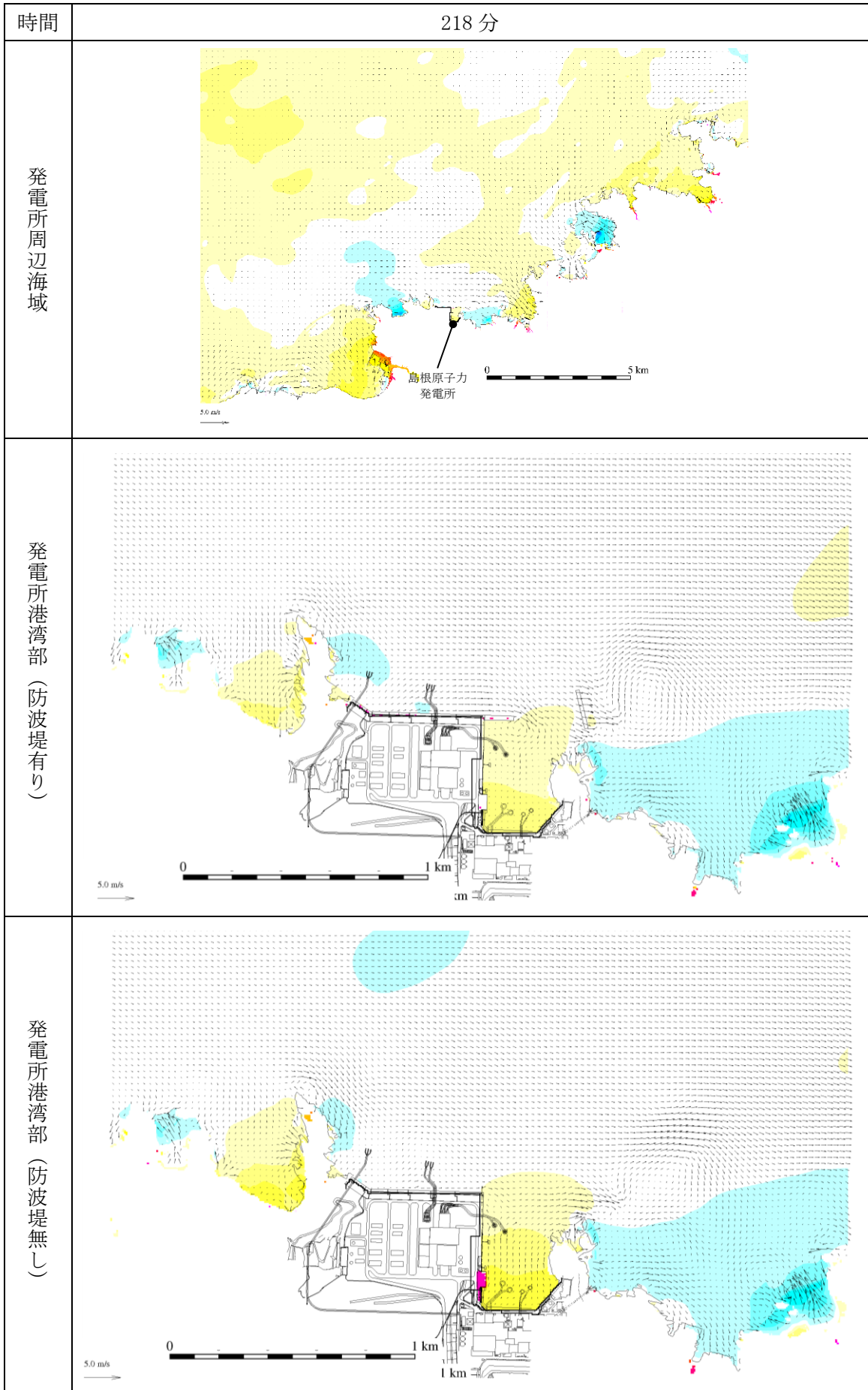
図 1-237 基準津波 1 の水位変動・流向ベクトル
