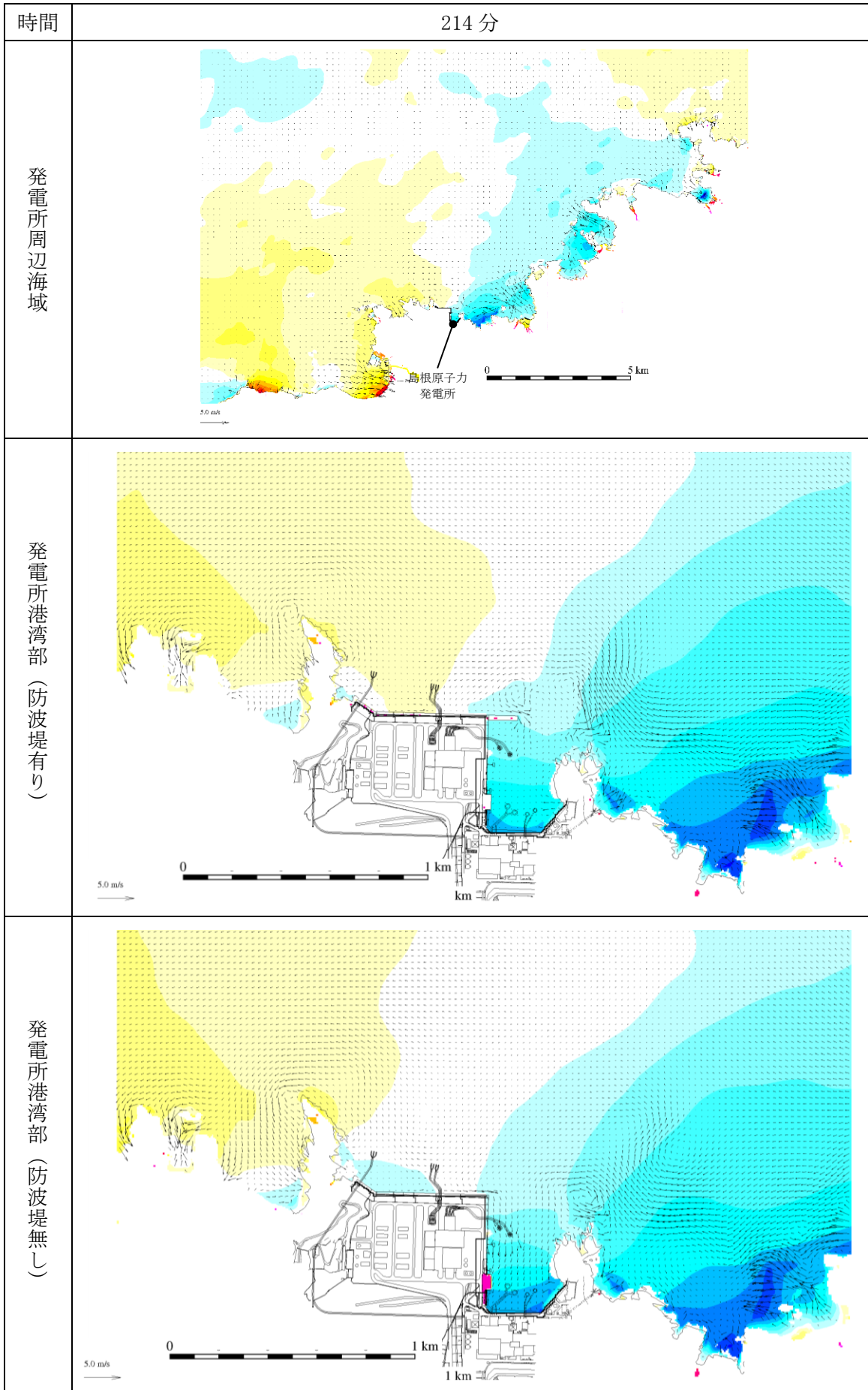
図 1-229 基準津波 1 の水位変動・流向ベクトル
