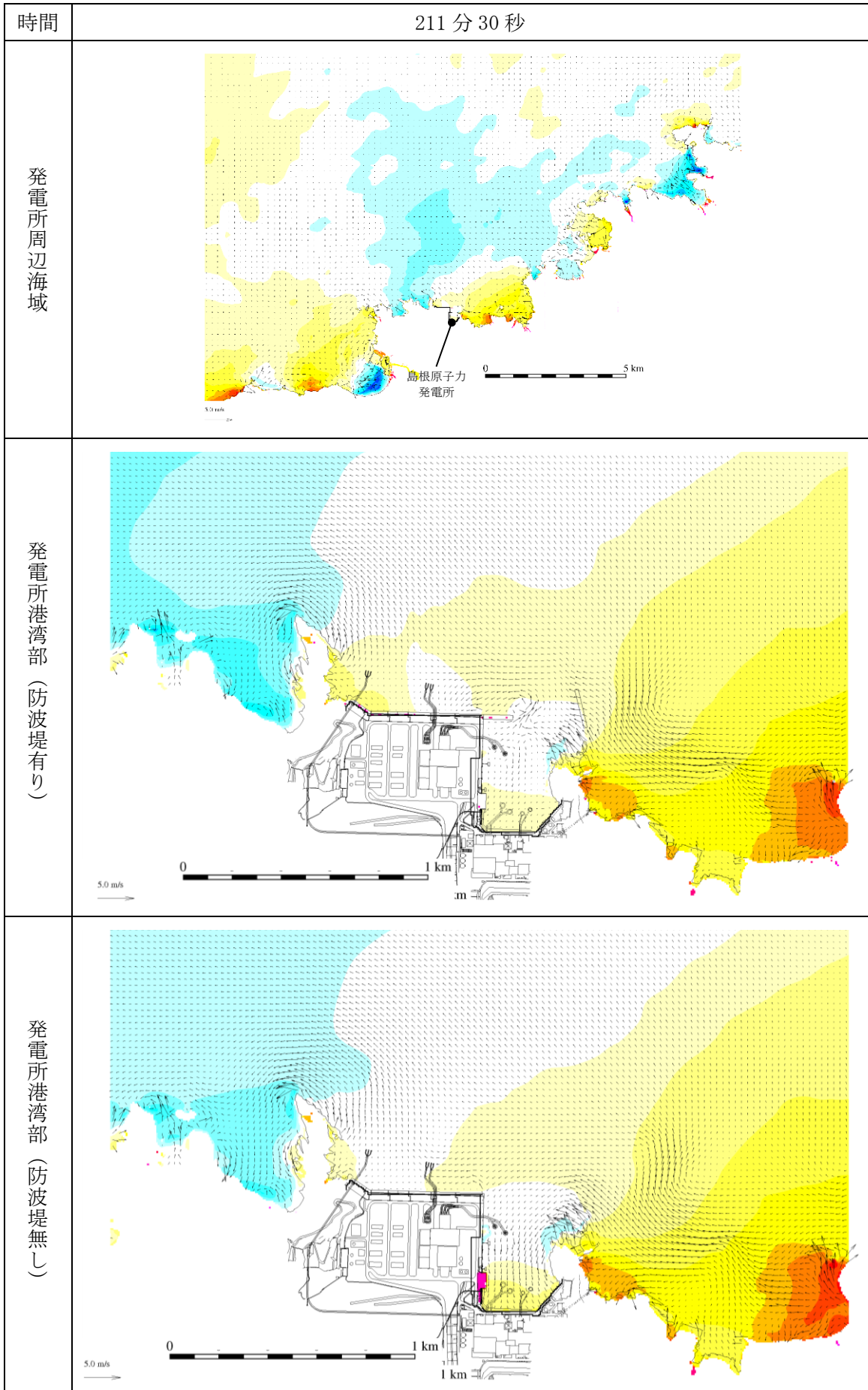
図 1-224 基準津波 1 の水位変動・流向ベクトル
