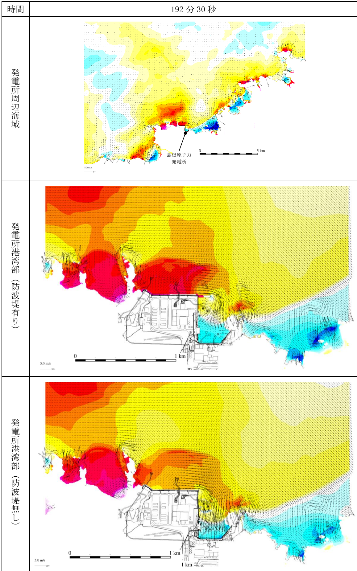
図 1-186 基準津波 1 の水位変動・流向ベクトル
