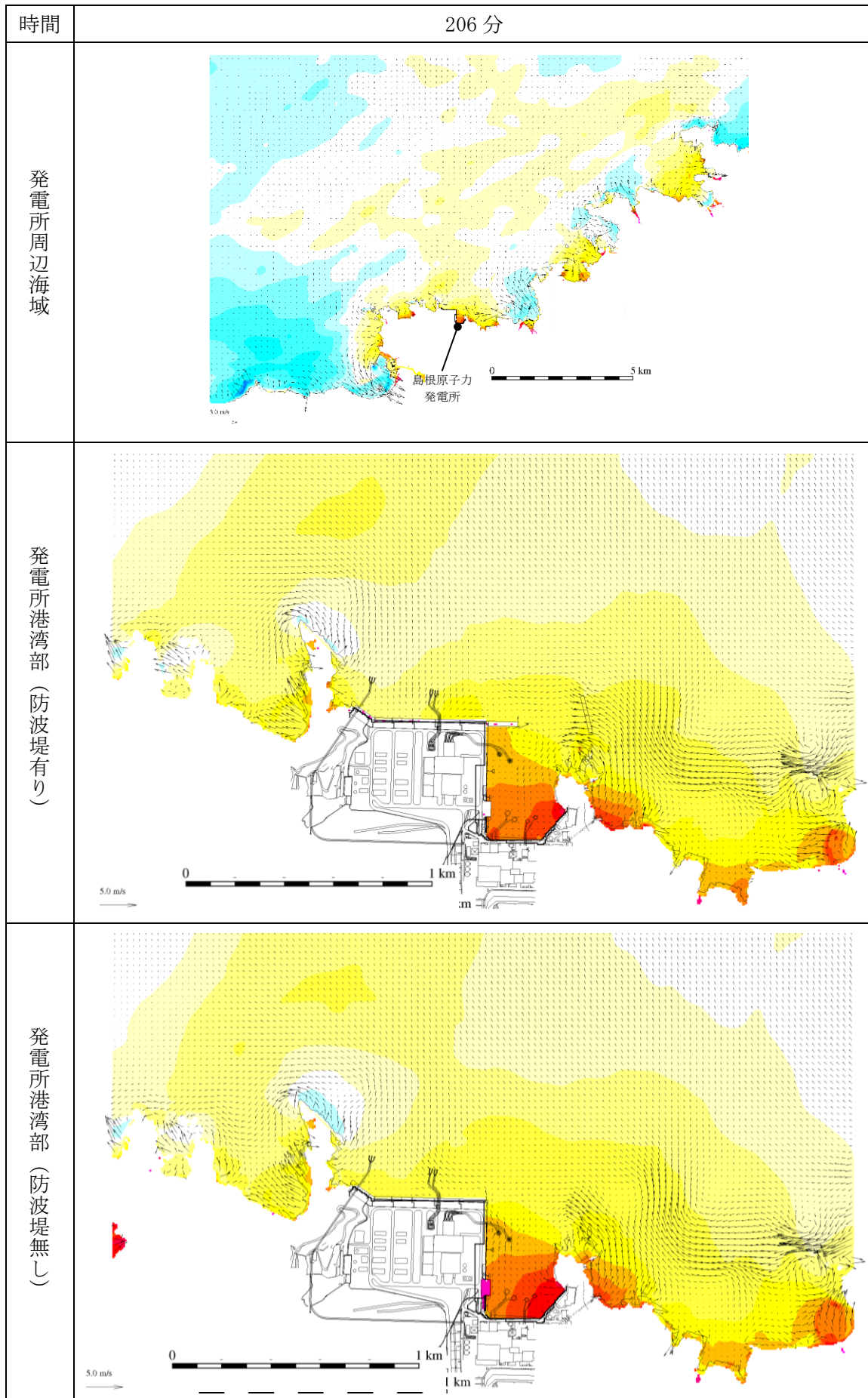
図 1-213 基準津波 1 の水位変動・流向ベクトル
