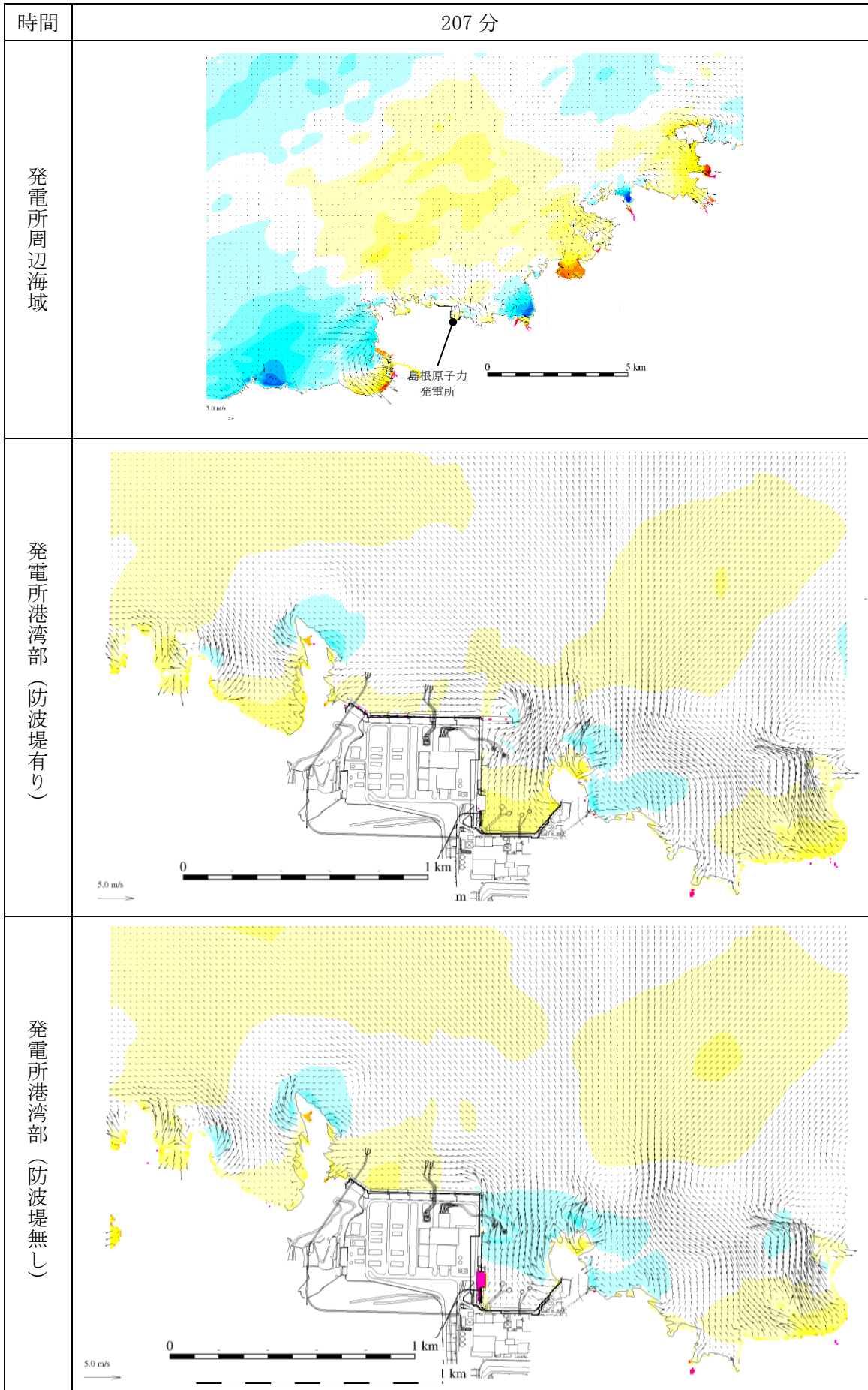
図 1-215 基準津波 1 の水位変動・流向ベクトル
