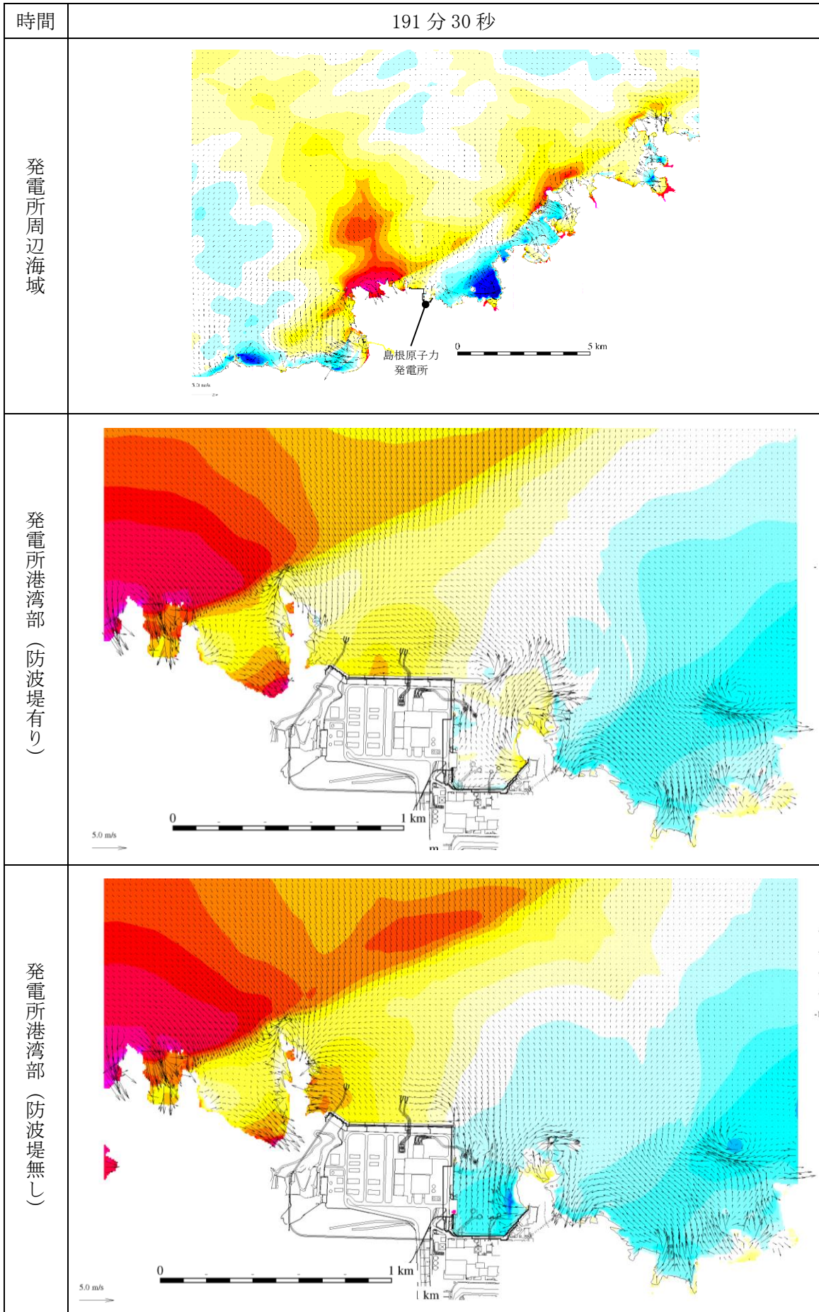
図 1-184 基準津波 1 の水位変動・流向ベクトル
