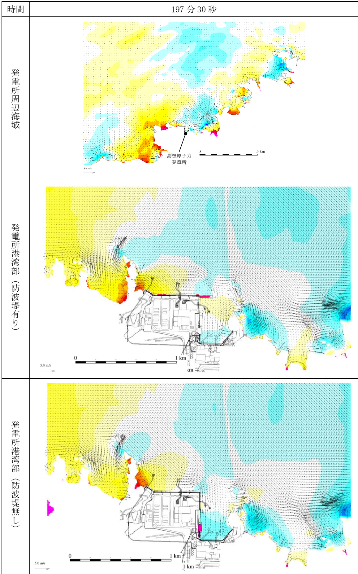
図 1-196 基準津波 1 の水位変動・流向ベクトル
