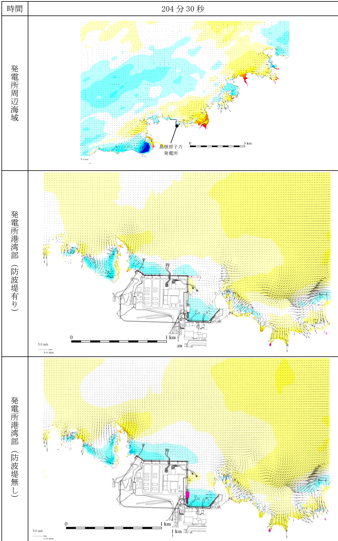
図 1-210 基準津波 1 の水位変動・流向ベクトル
