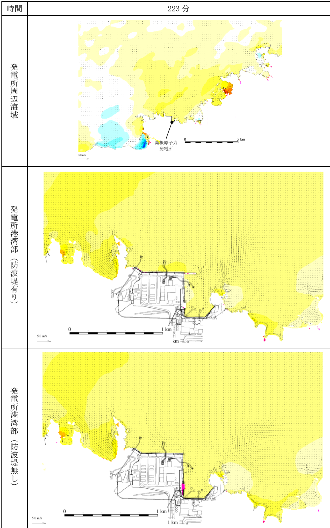
図 1-247 基準津波 1 の水位変動・流向ベクトル
