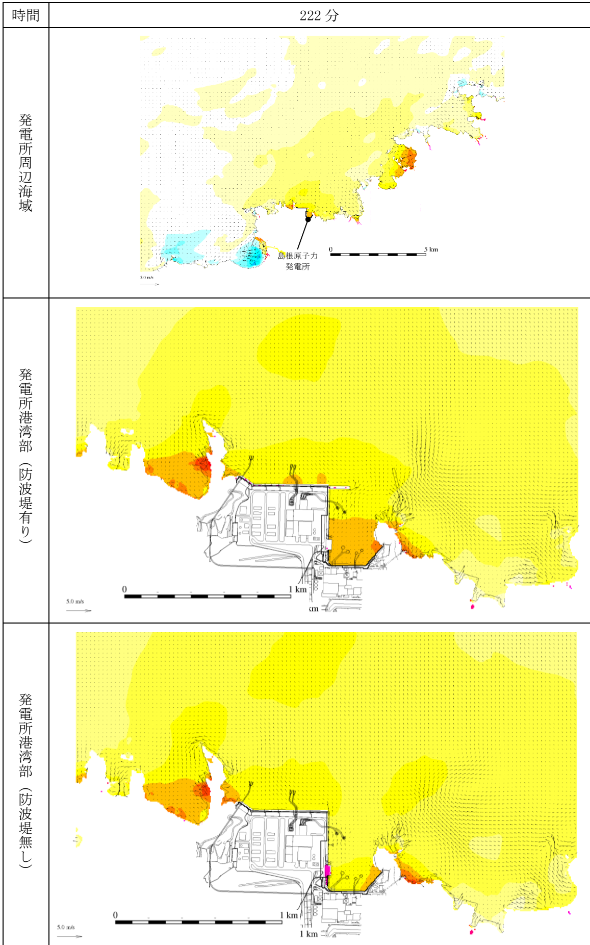
図 1-245 基準津波 1 の水位変動・流向ベクトル
