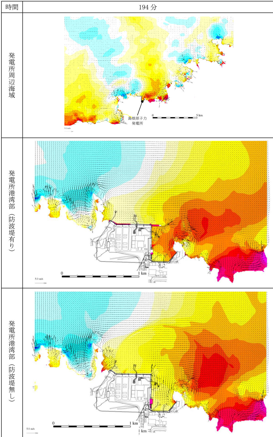
図 1-189 基準津波 1 の水位変動・流向ベクトル
