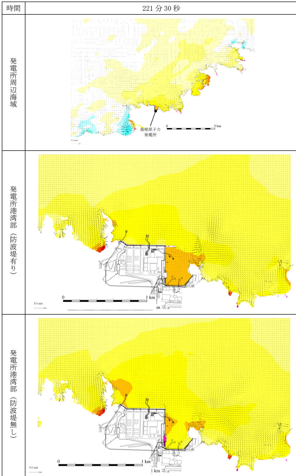
図 1-244 基準津波 1 の水位変動・流向ベクトル
