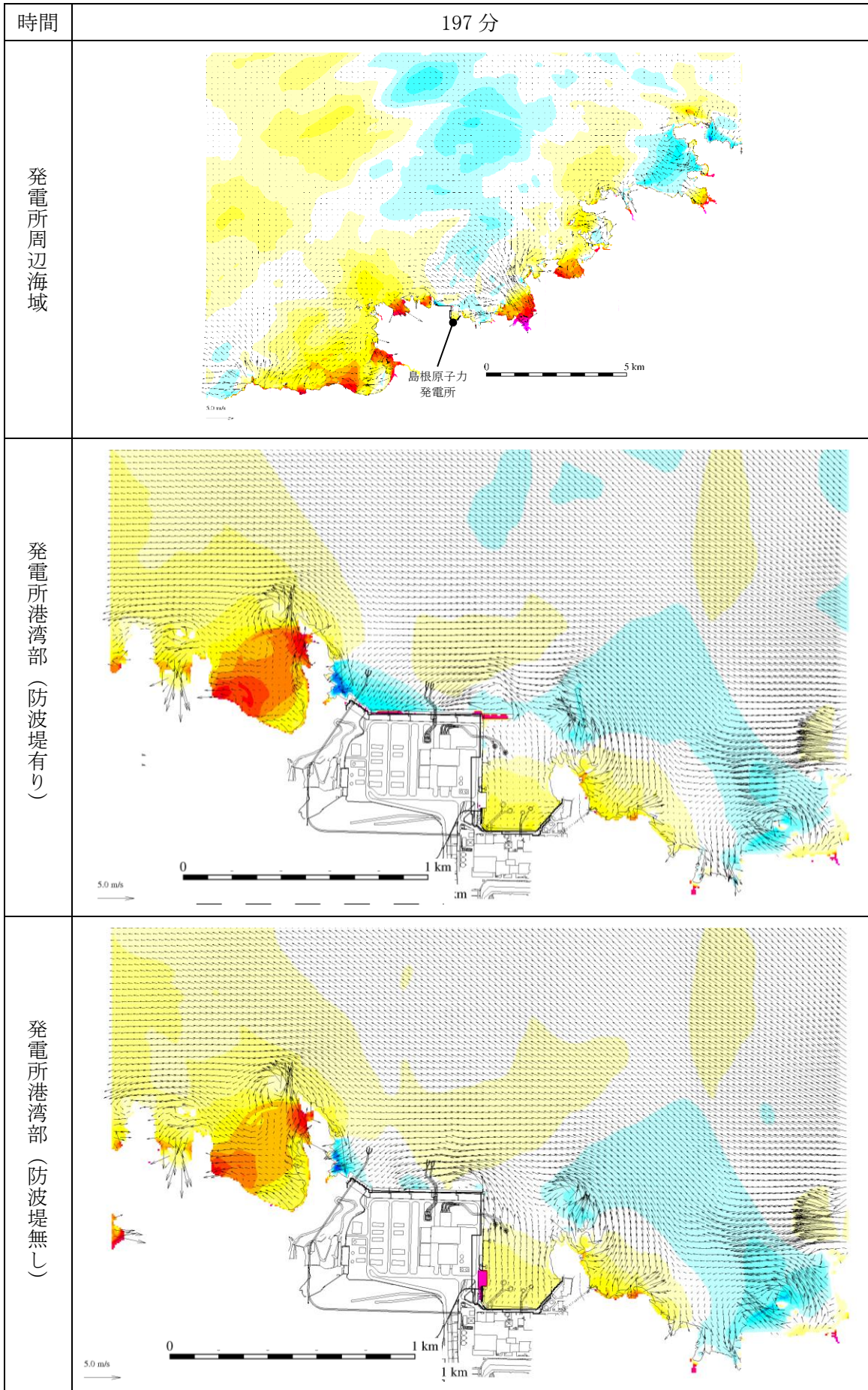
図 1-195 基準津波 1 の水位変動・流向ベクトル
