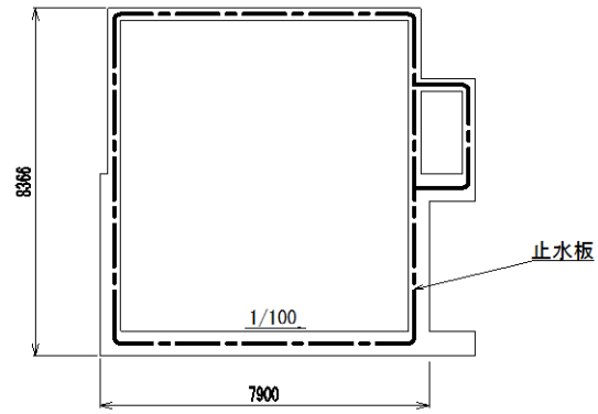
(正面図)
