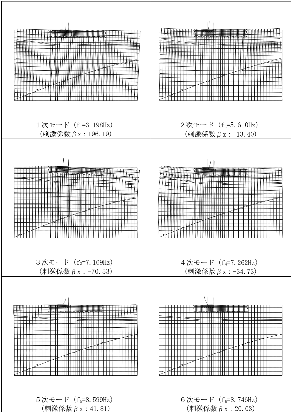
図 2.3-13 固有値解析結果におけるモード図
