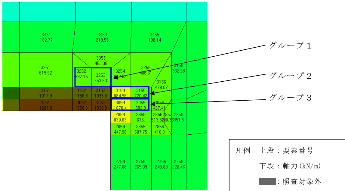
(a) 断面力分布全体図 (遮蔽壁 (本体))
