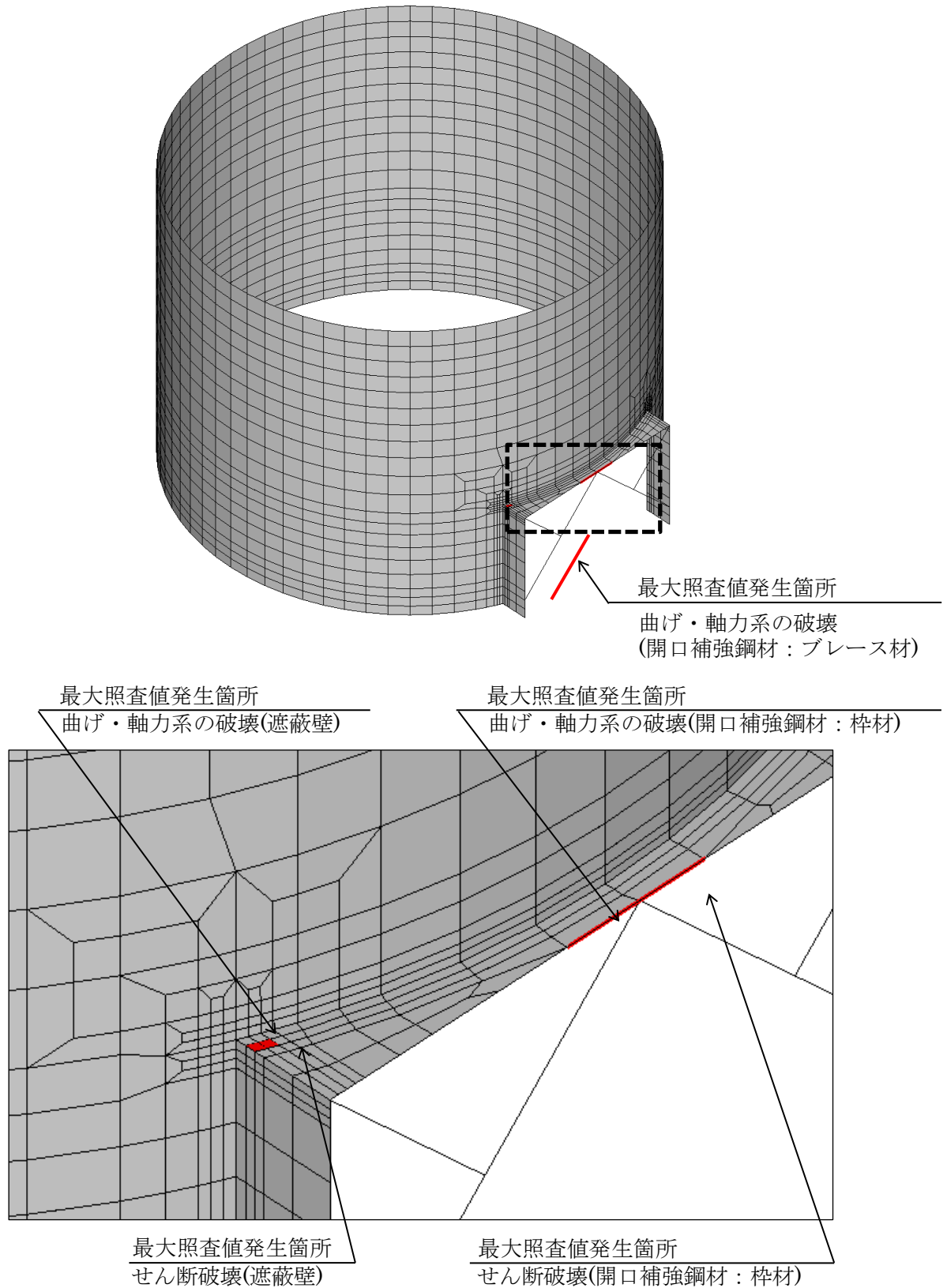
図 2.6-13 最大照査値発生箇所位置図 (鳥瞰図, 南東側から望む)
