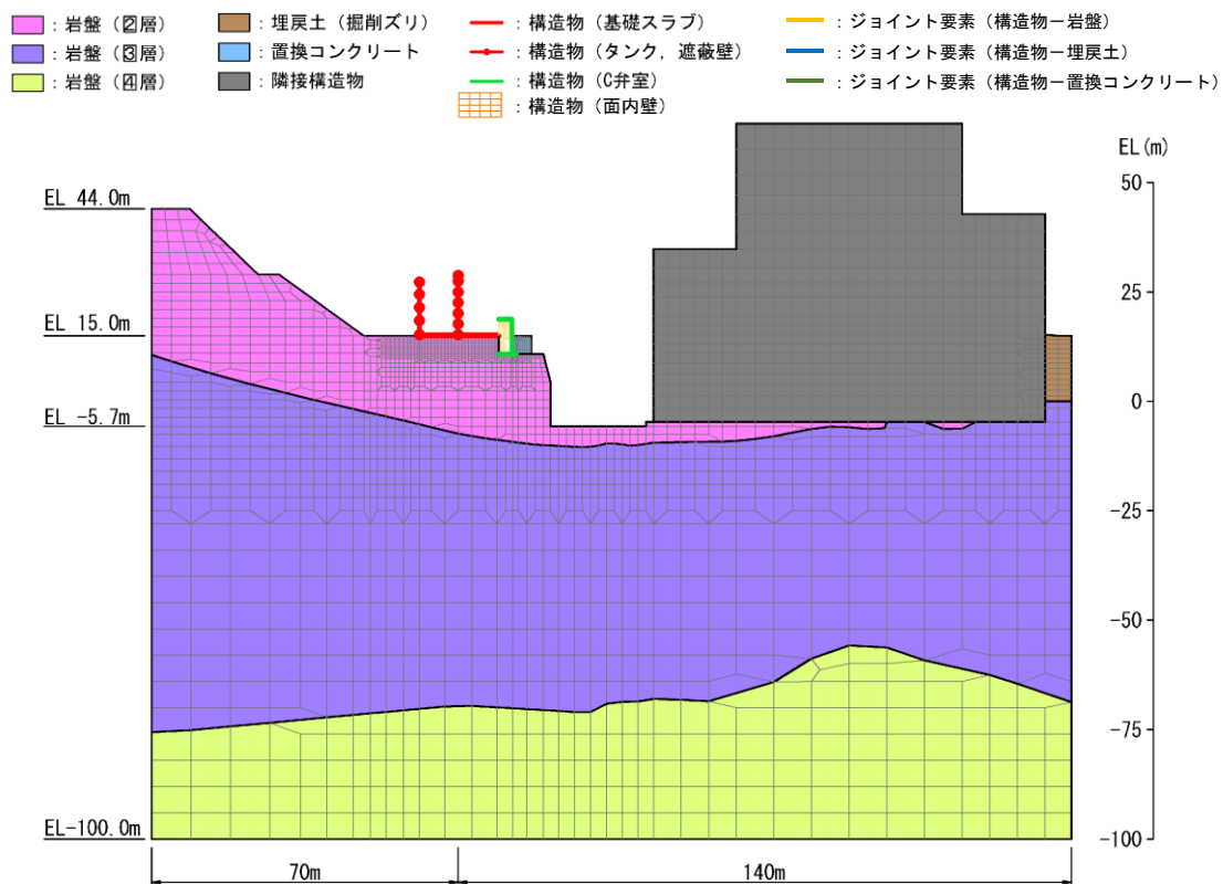
(全体図)
