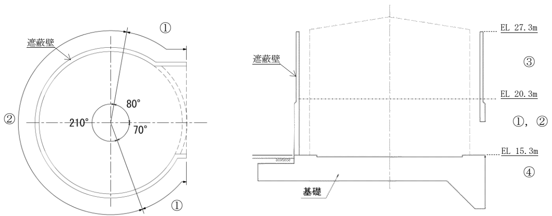
(遮蔽壁, 基礎)
