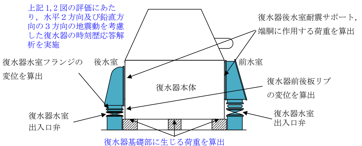
図 7.12-3 地震時の復水器時刻歴応答解析のイメージ (C. 3次元 FEMモデルを用いた時刻歴応答解析)
