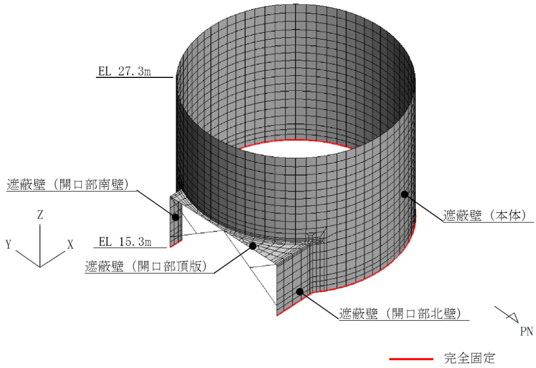
図 3-1(1) 評価対象箇所の概念図 (復水貯蔵タンク遮蔽壁)
