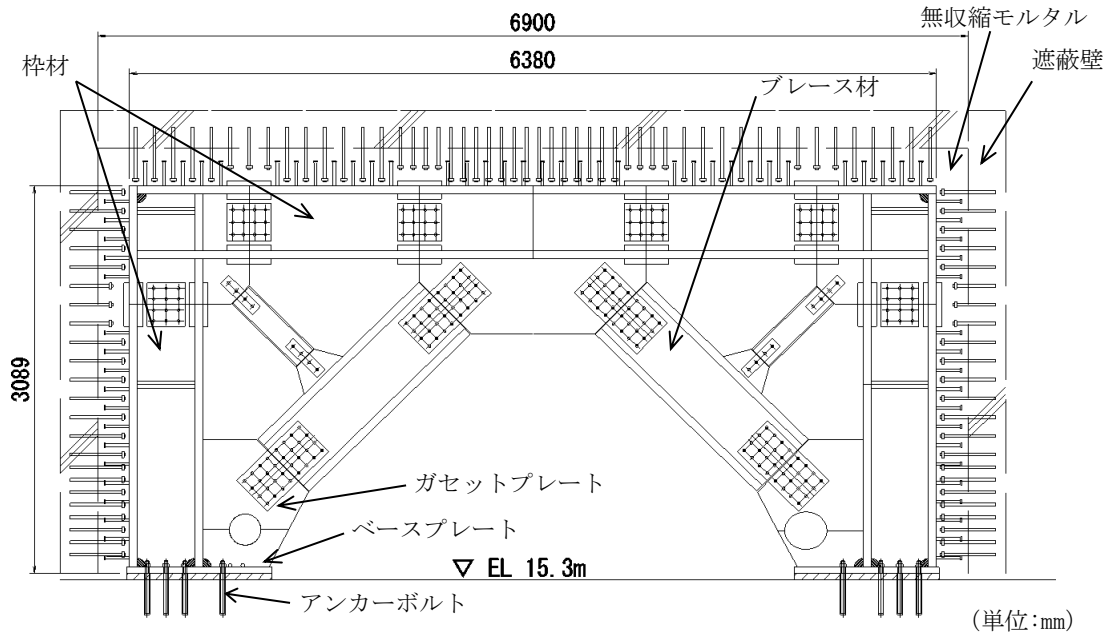
図 2.2-5 補助復水貯蔵タンク遮蔽壁の開口補強鋼材による耐震補強（正面図）
