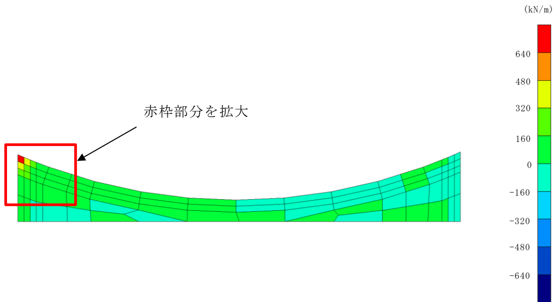
(a) せん断力分布全体図（遮蔽壁（開口部頂板））
