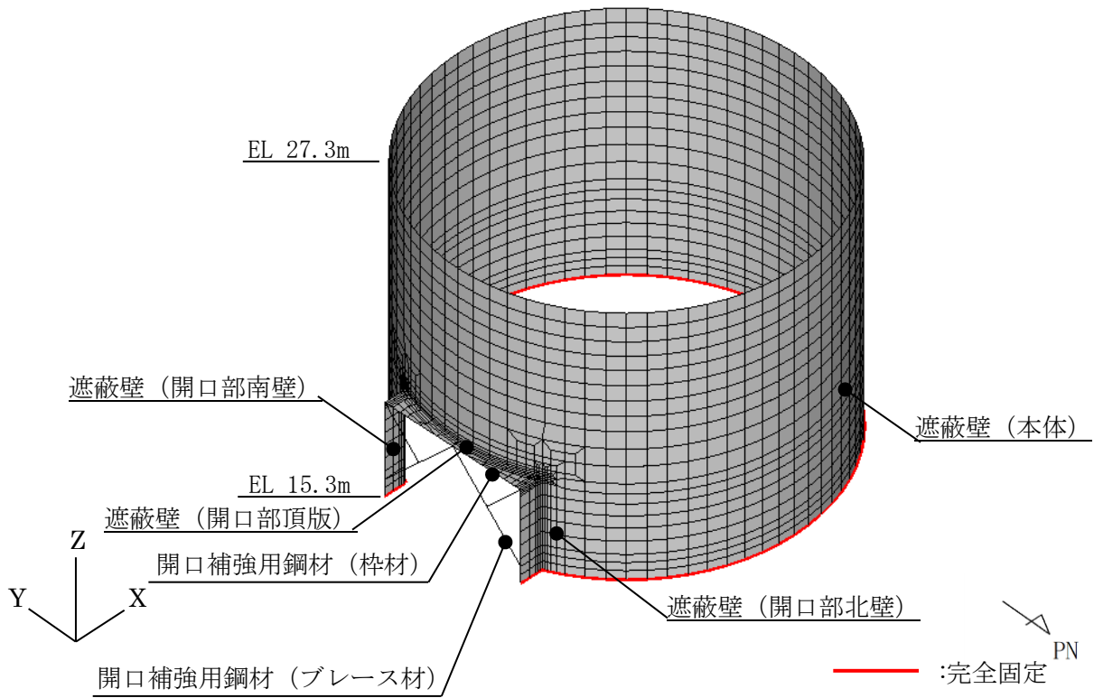
図 2.4-2(1) 3次元静的FEM解析モデル (鳥瞰図, 北東側から望む)
