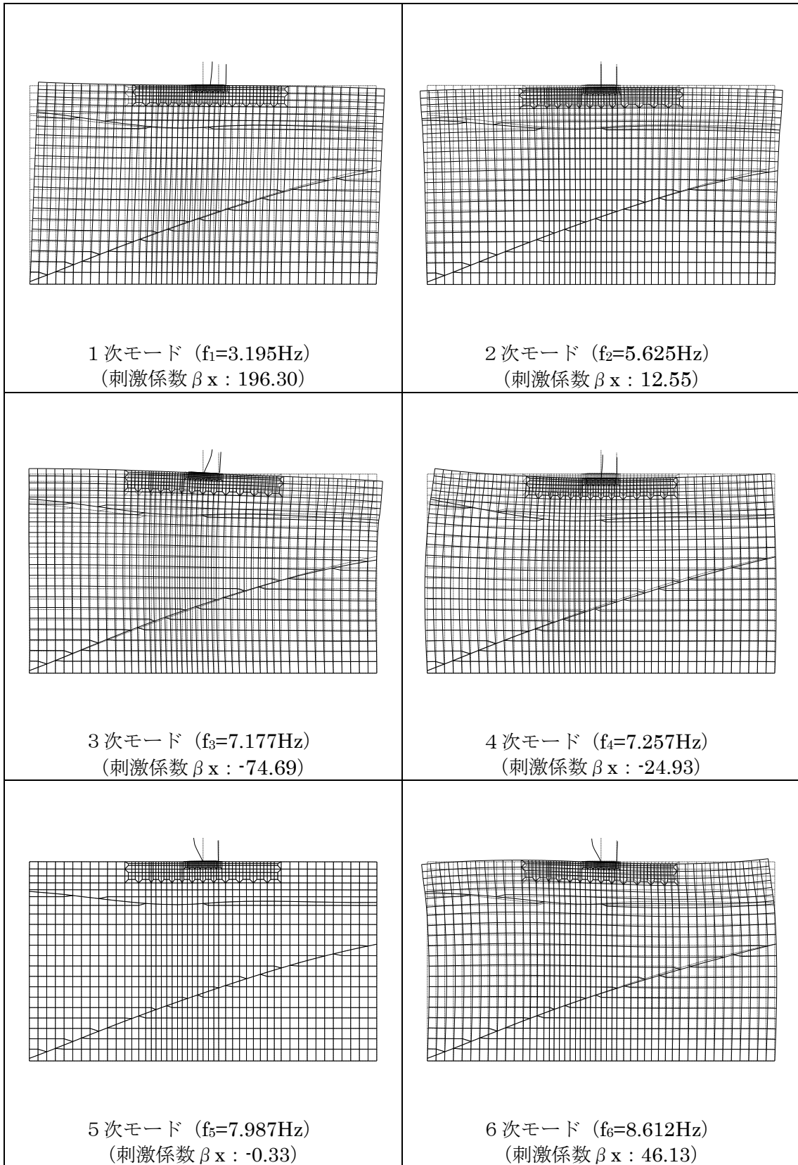
図 1.3-13 固有値解析結果におけるモード図
