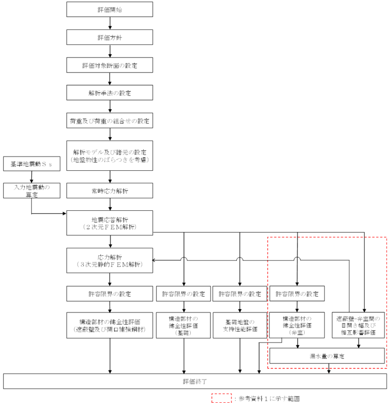
図2-4 復水貯蔵タンク遮蔽壁等の耐震評価フロー
