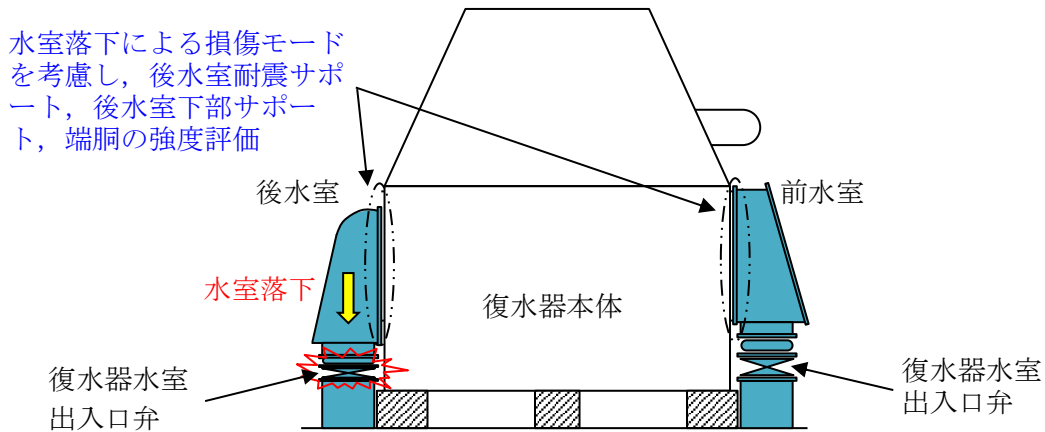
図 7.12-1 地震時の復水器水室出入口弁への影響イメージ (A. 復水器水室落下の影響)
