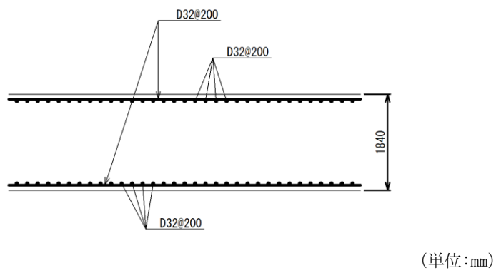
図 2.2-6(2) 補助復水貯蔵タンク遮蔽壁の概略配筋図 (基礎)
