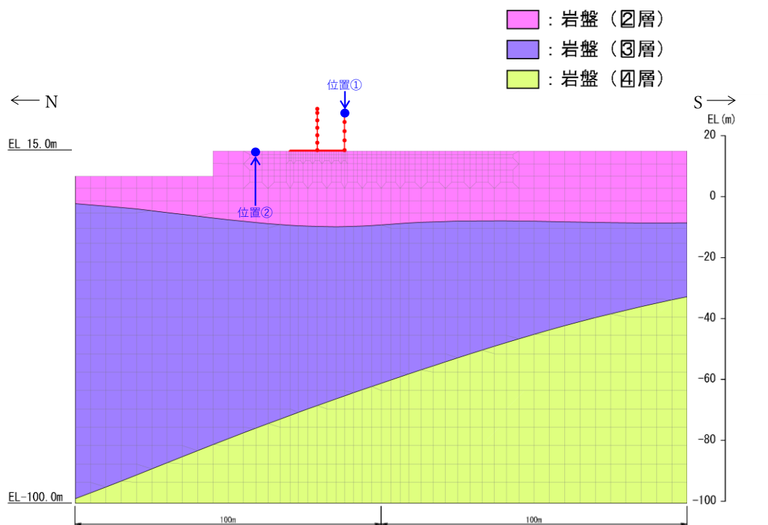
図3 対象構造物北側の小規模な法面をモデル化したモデル（モデル①）
