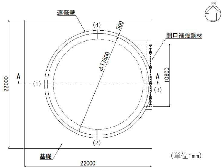
図 1.2-2 復水貯蔵タンク遮蔽壁の平面図
