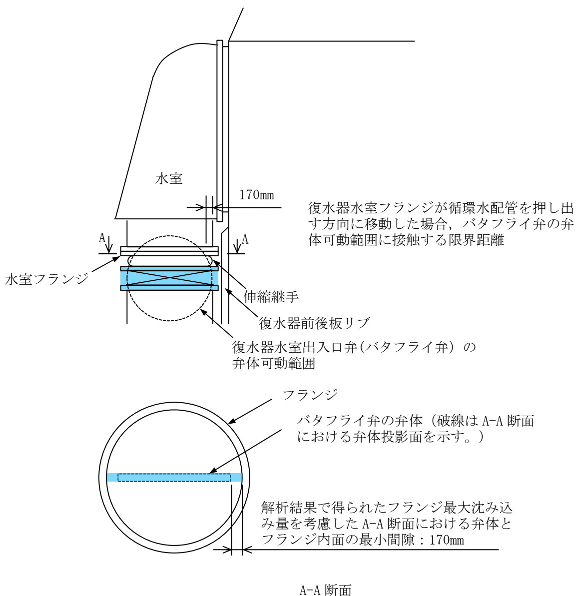
図 7.12-28 復水器水室フランジ許容変位
