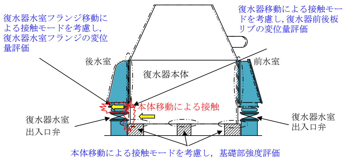
図 7.12-2 地震時の復水器水室出入口弁への影響イメージ (B. 復水器本体移動による接触影響)
