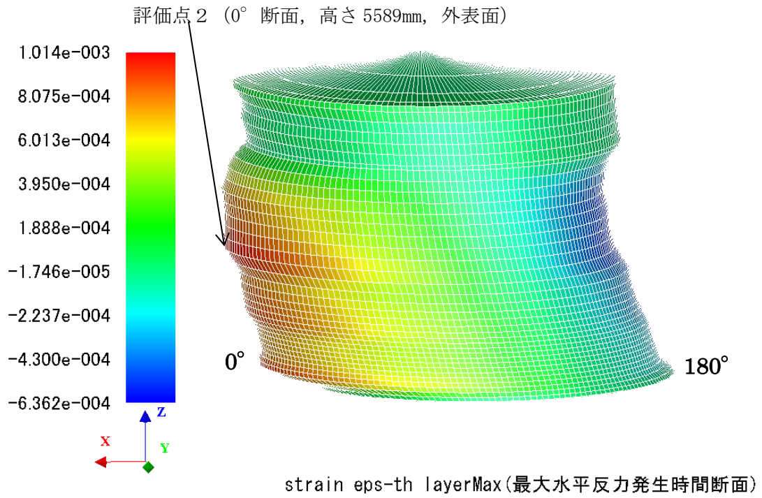
図 5-10 最大水平反力発生時外表面周方向ひずみ (変形倍率 200 倍)
