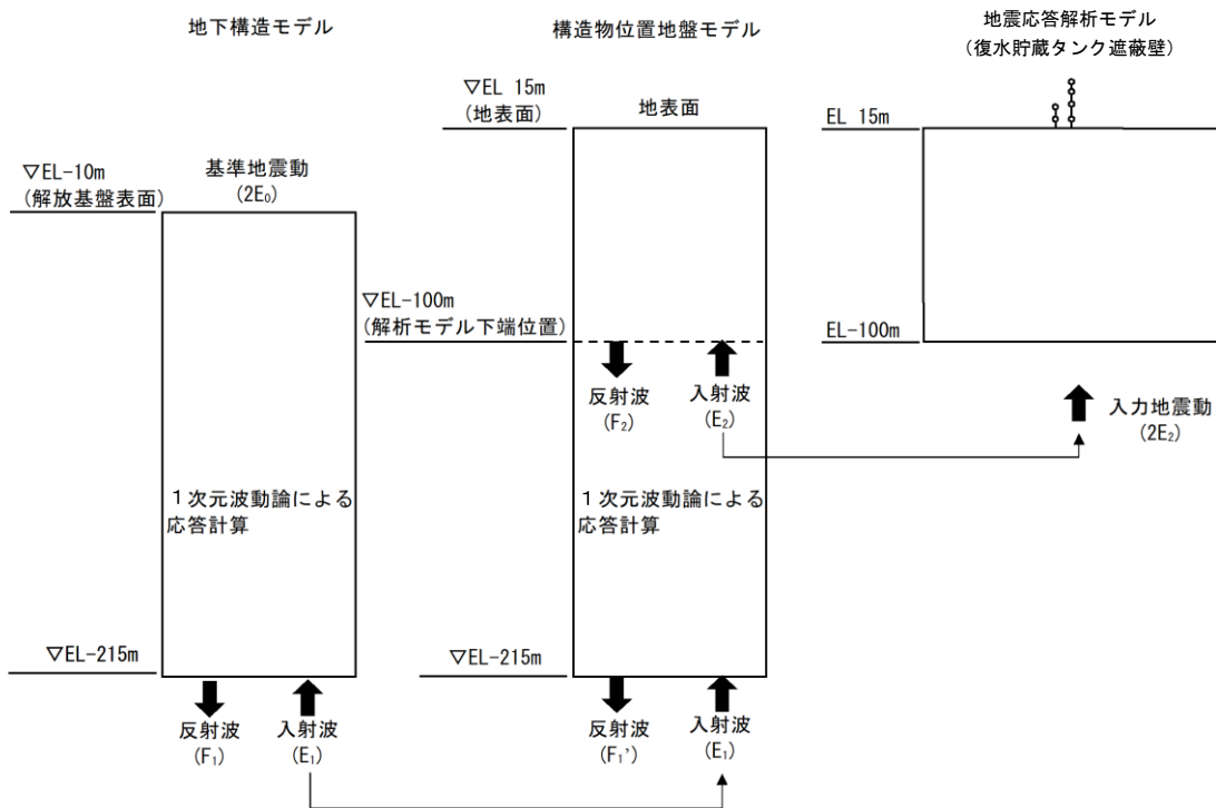
図 1.3-19 入力地震動算定の概念図
