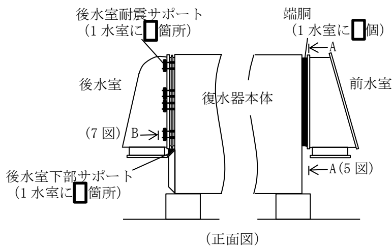
図 7.12-4 評価部位取付形状
