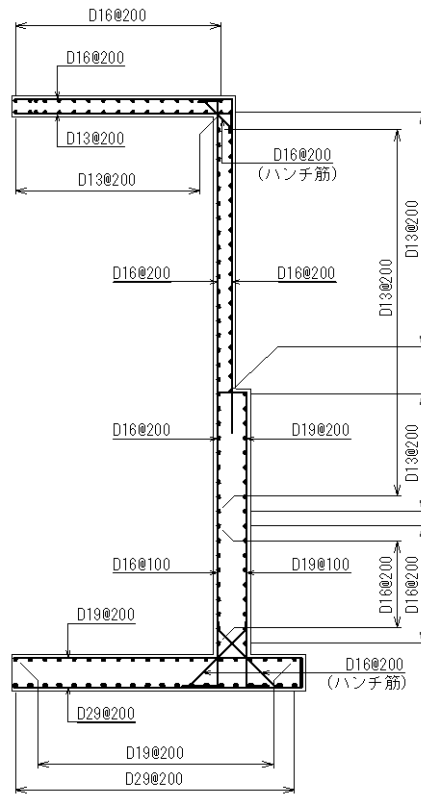
図 2.2-12(4) トーラス水受入タンク遮蔽壁の概略配筋図 (弁室)
