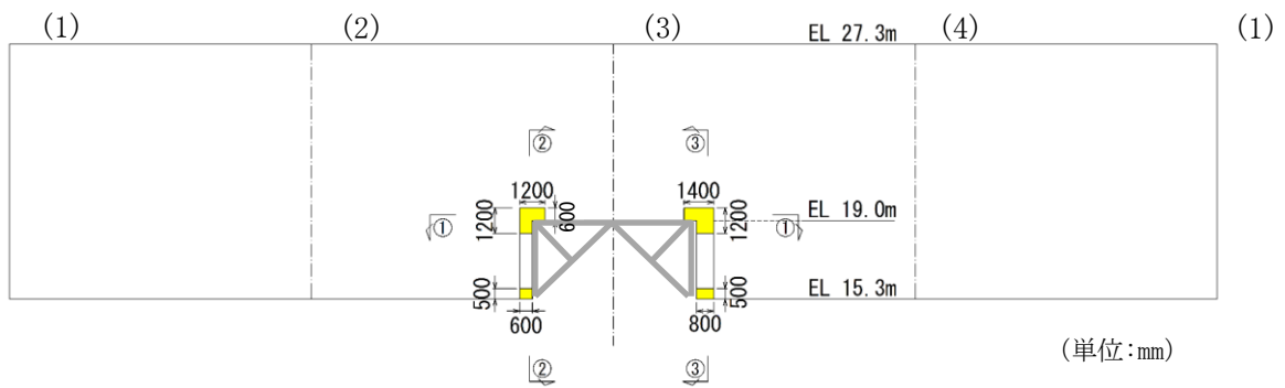
(展開図)
