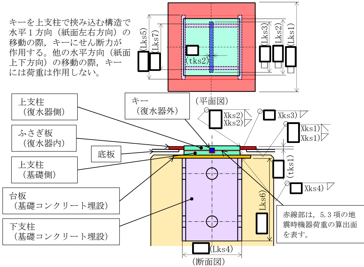
図 7.12-16 キーサポート⑦⑧平面図，断面図
