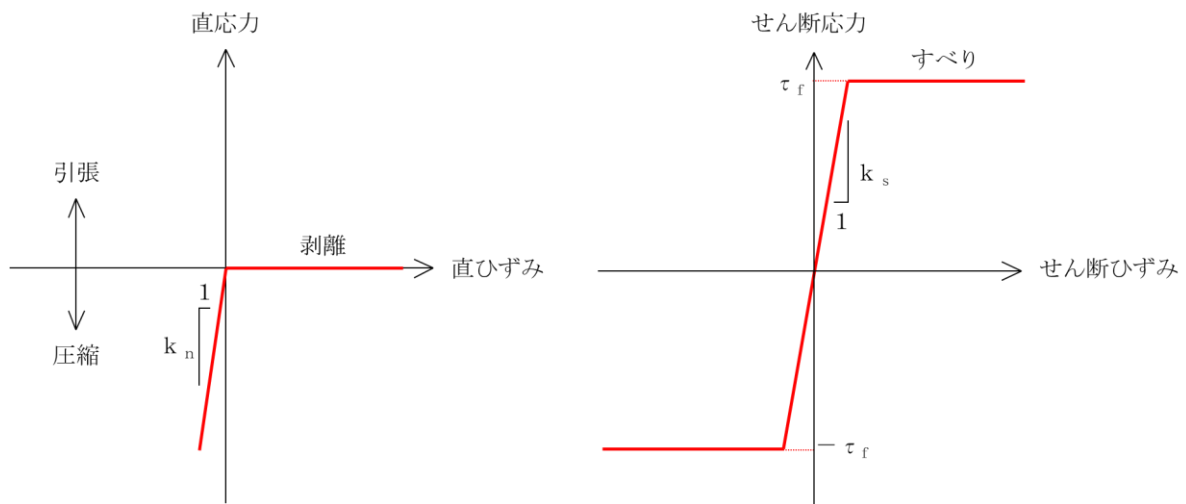
図 1.3-9 ジョイント要素の力学特性
