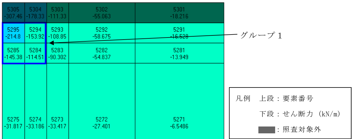
(b) せん断力分布拡大図（遮蔽壁（開口部南壁））
