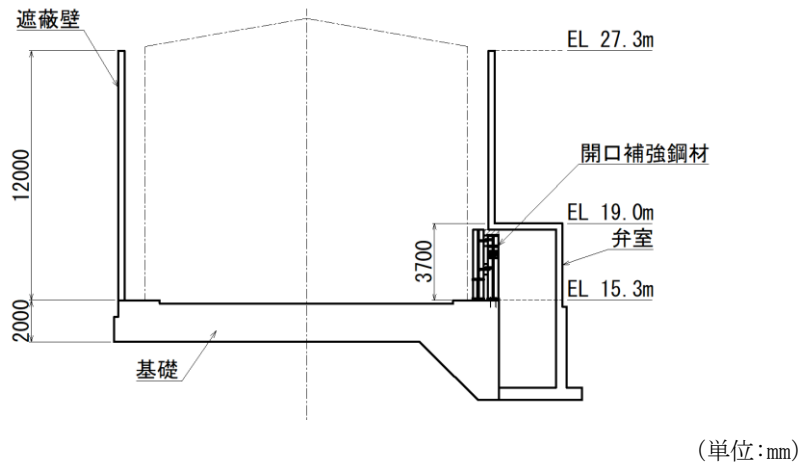
図 2.2-3 補助復水貯蔵タンク遮蔽壁の断面図 (A-A 断面, 東西)
