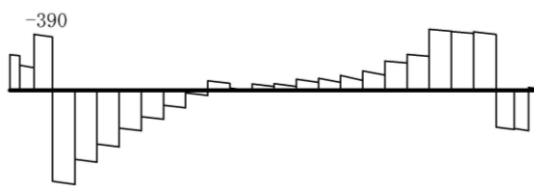
数值：評価位置における断面力 (b) 軸力 (kN) (+ : 引張, - : 圧縮)
