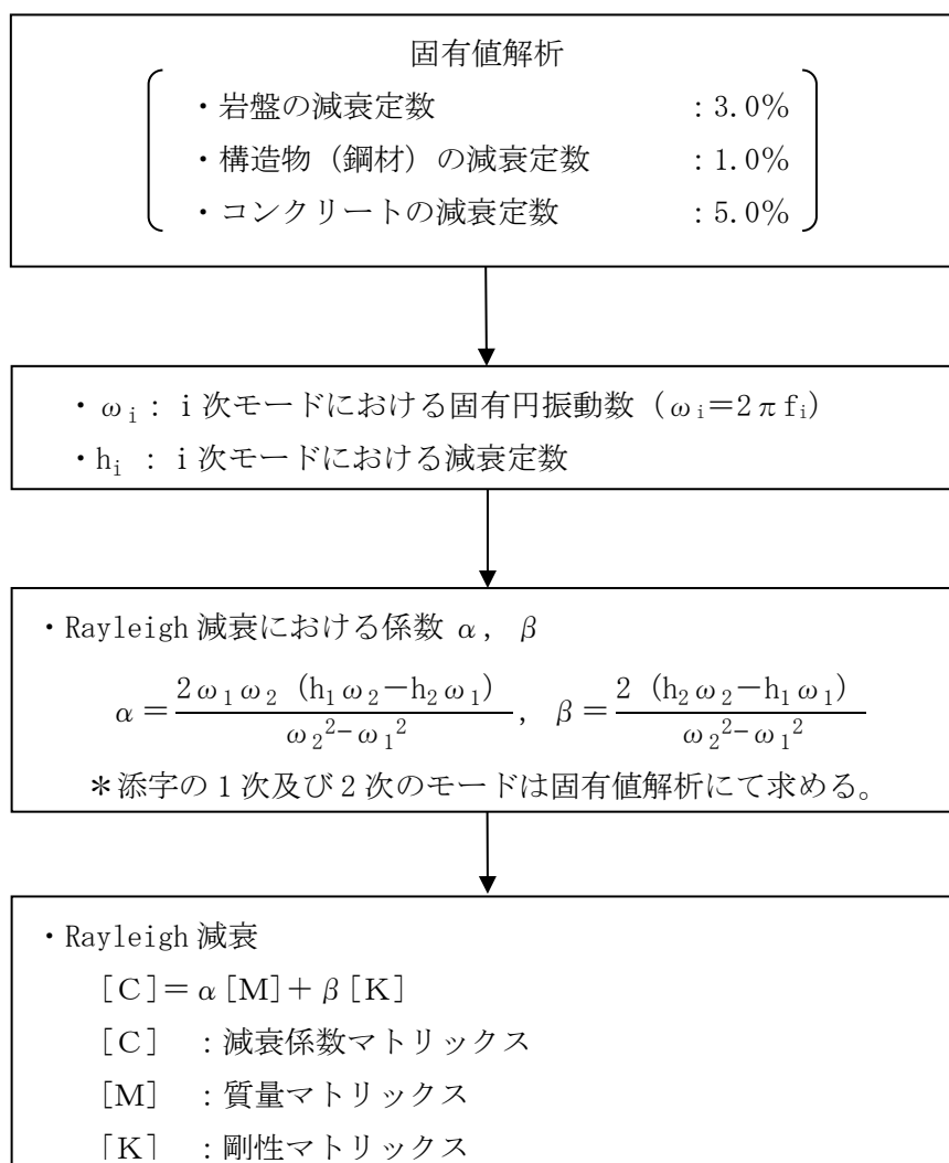
図 1.3-12 Rayleigh 減衰の設定フロー
