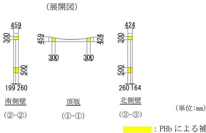
図 1-4 トーラス水受入タンク遮蔽壁の PHb による耐震補強の概要
