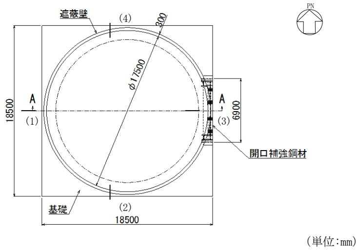
図 2.2-2 補助復水貯蔵タンク遮蔽壁の平面図
