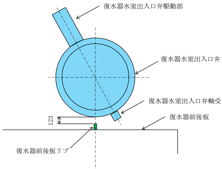
図 7.12-29 復水器前後板リブ許容変位
