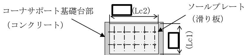
図 7.12-25 コーナサポート部ソールプレート寸法図
