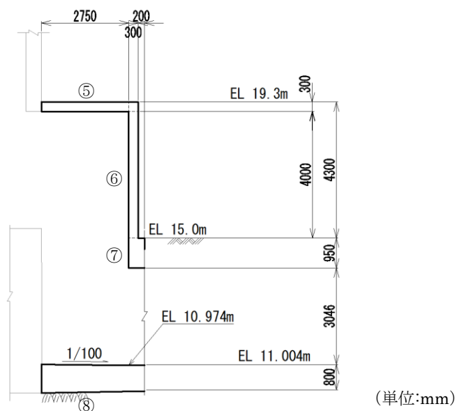
(弁室)
