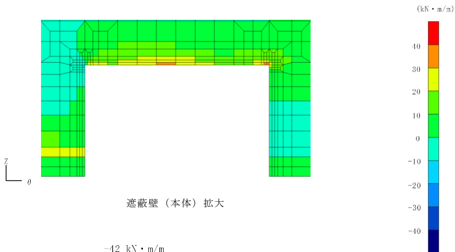
遮蔽壁 (本体)
