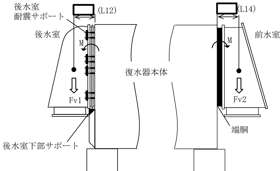
図 7.12-12 地震力が鉛直方向に作用した場合
