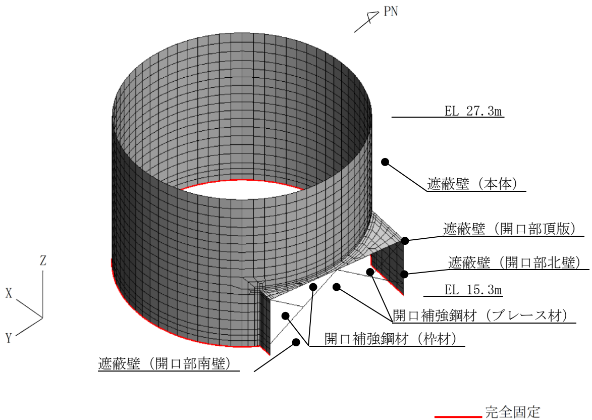
図 1.4-2(2) 3次元静的FEM解析モデル (鳥瞰図, 南東側から望む)
