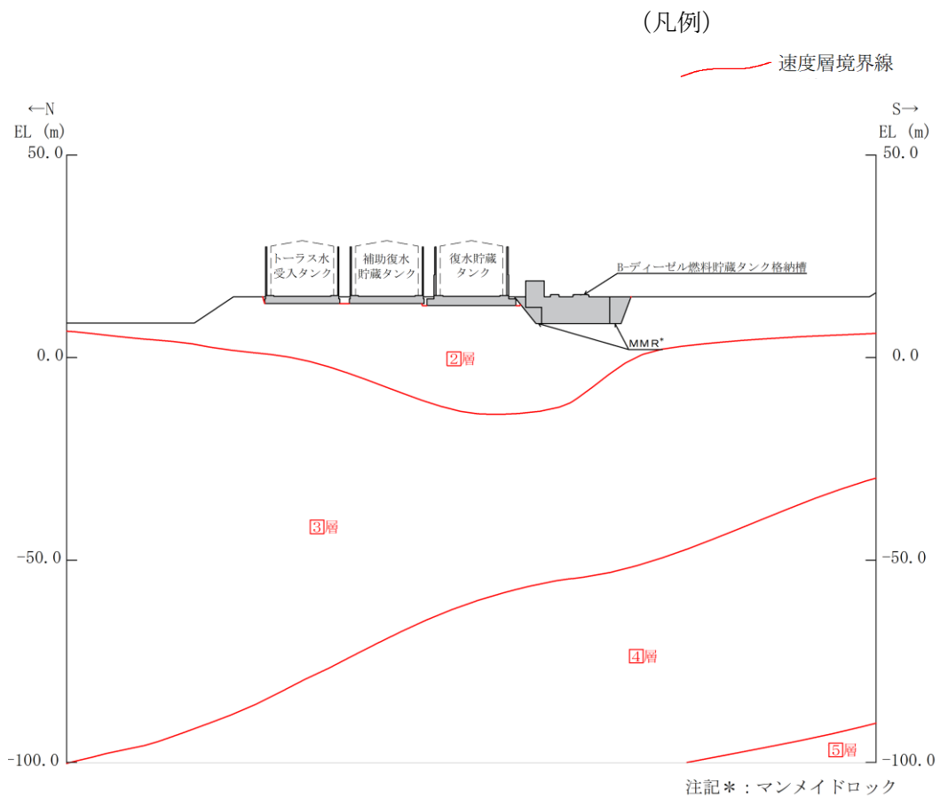
図 2.2-17 補助復水貯蔵タンク遮蔽壁の評価対象断面図 (A-A 断面)
