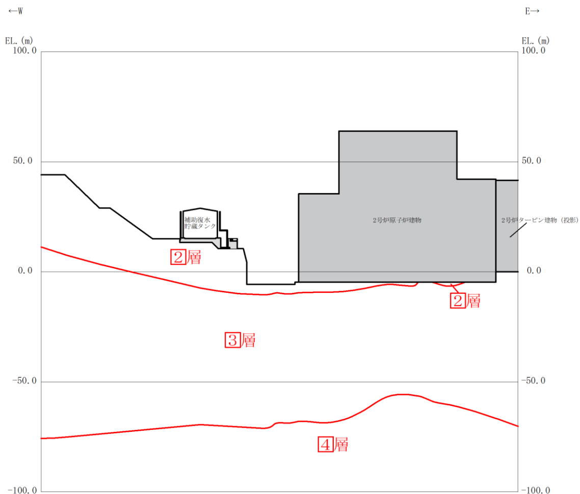
図3-6 地質断面図 (B-B断面)
