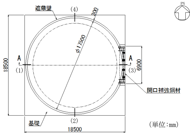
(平面図)
