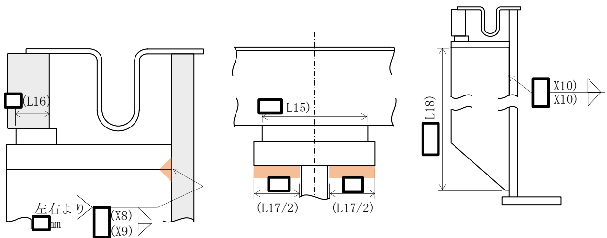
図 7.12-7 後水室耐震サポートの形状 (代表例)
