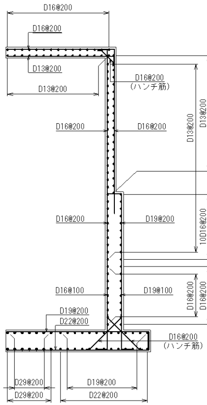
図 2.2-6(4) 補助復水貯蔵タンク遮蔽壁の概略配筋図 (弁室)
