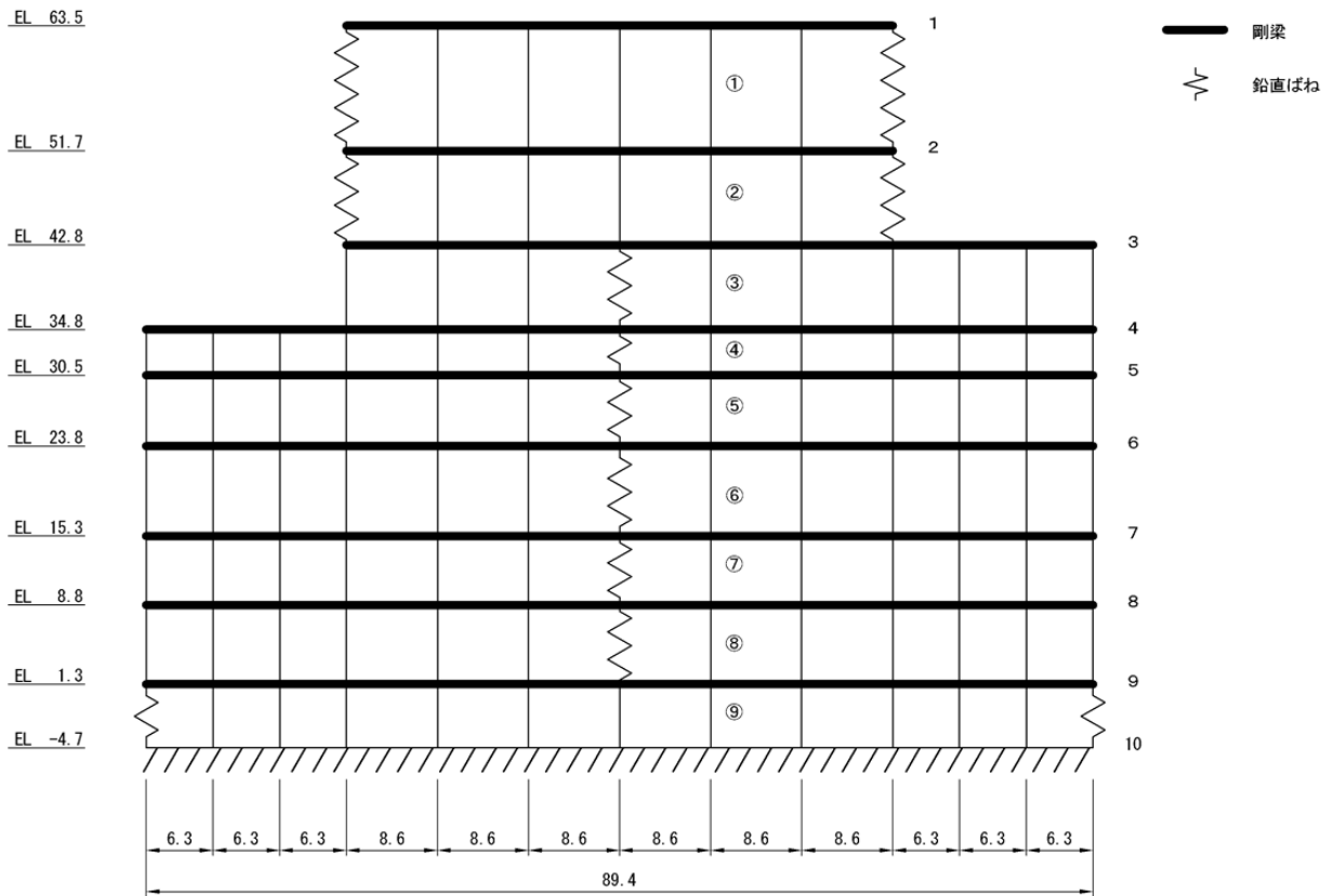
図 3-5 原子炉建物の有限要素モデル
