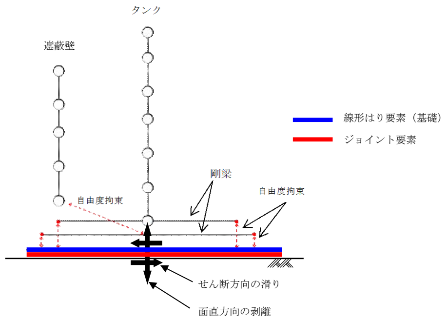
図 1.3-10 ジョイント要素の配置概念図
