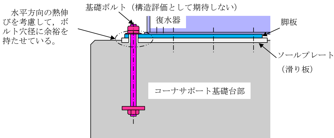
図 7.12-24 鉛直下向き荷重を受ける基礎台の概略断面図
