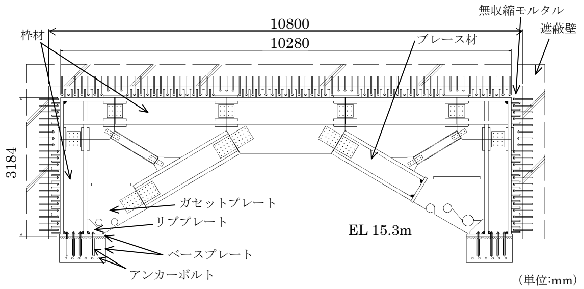
図 1.2-5 復水貯蔵タンク遮蔽壁の開口補強鋼材による耐震補強概念図 (正面図)
