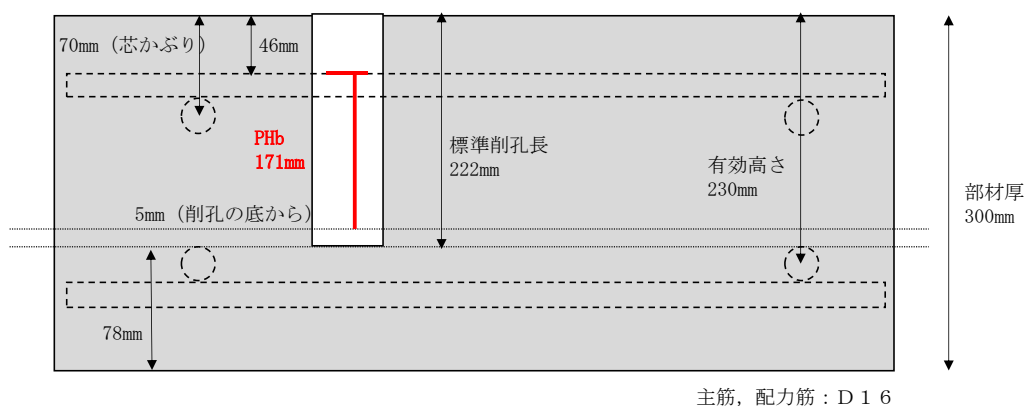
図1-1 PHbの構造概要
