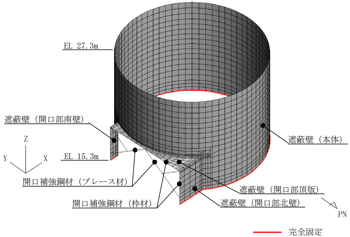
図 1.4-2(1) 3次元静的FEM解析モデル (鳥瞰図, 北東側から望む)
