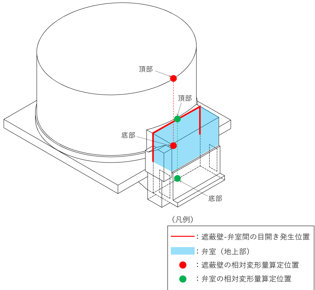
図 4-5 目開き発生位置の概念図
