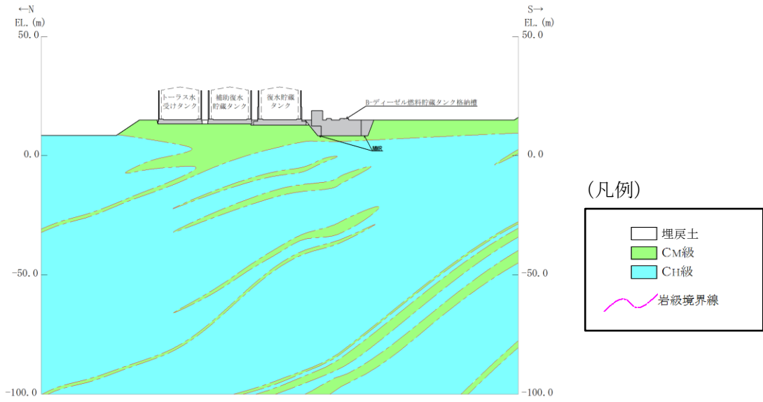
(岩級図)
