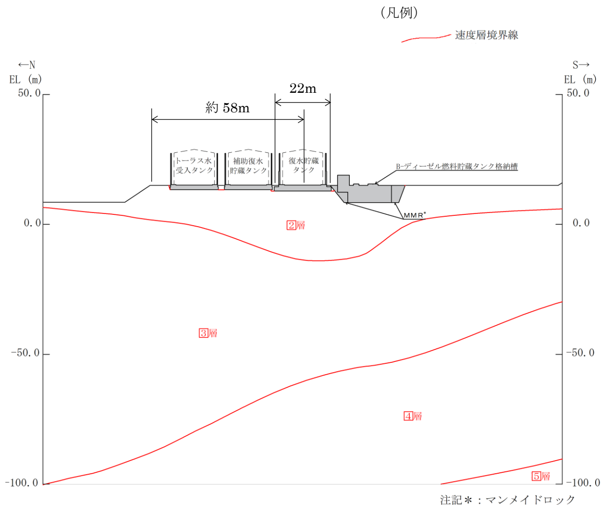
図 1.3-7 地表面形状設定の考え方
