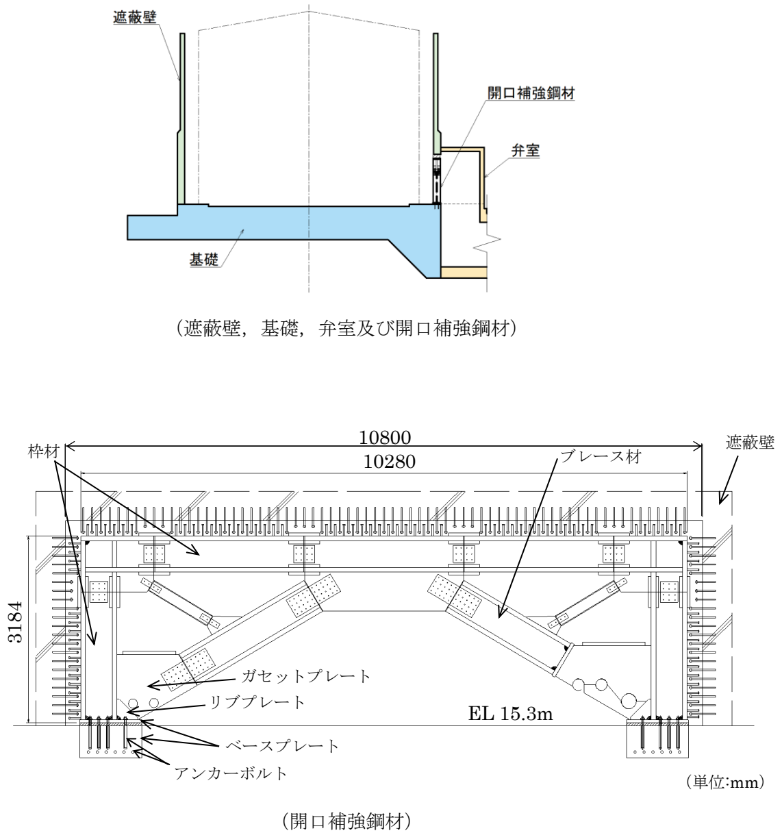
図 1.2-12 評価対象部位
