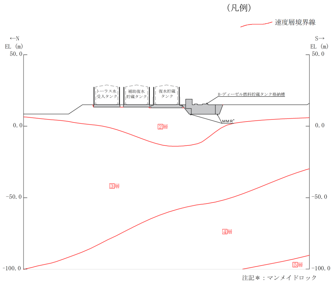
図 1.2-11 復水貯蔵タンク遮蔽壁の評価対象断面図 (A-A 断面)
