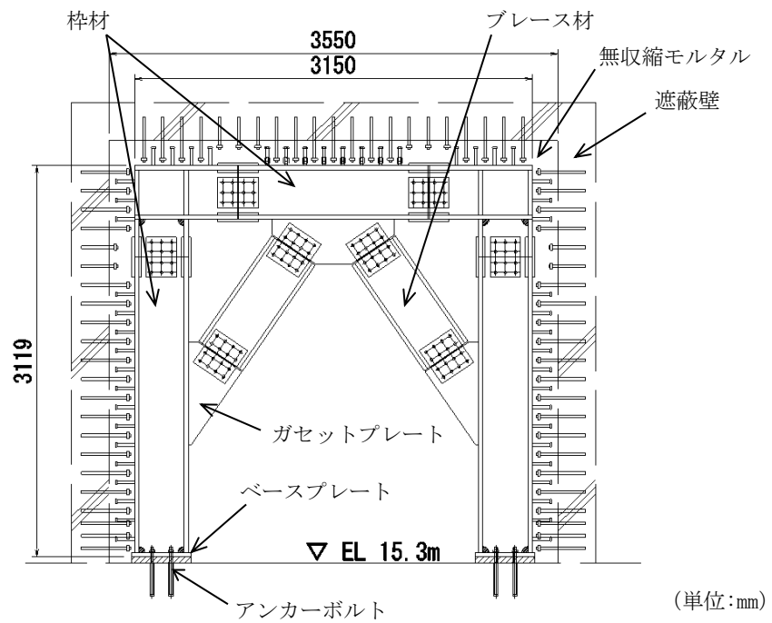
図 2.2-11 トーラス水受入タンク遮蔽壁の開口補強鋼材による耐震補強（正面図）
