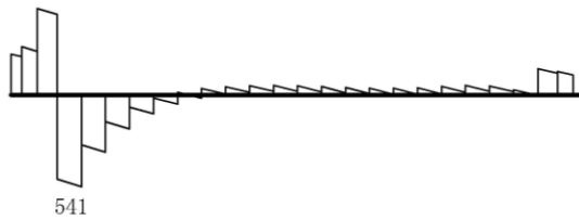
数值：評価位置における断面力 (c) せん断力 (kN)
