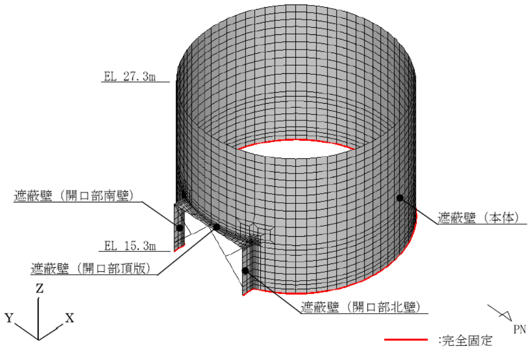
図 3-1(2) 評価対象箇所の概念図 (補助復水貯蔵タンク遮蔽壁)
