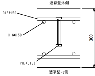
図 2.2-6(3) 補助復水貯蔵タンク遮蔽壁の概略配筋図 (PHb 工法)
