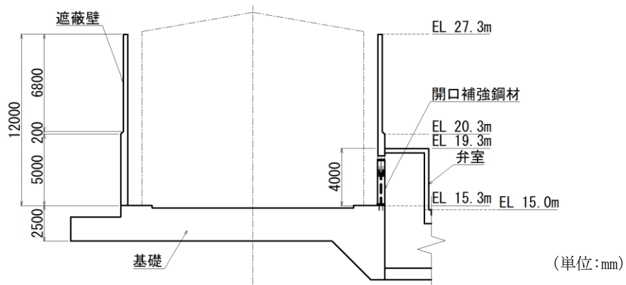
図 1.2-3 復水貯蔵タンク遮蔽壁の断面図 (A-A 断面, 東西)
