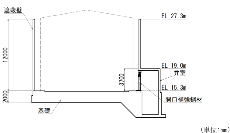
図 2.2-9 トーラス水受入タンク遮蔽壁の断面図 (A-A 断面, 東西)
