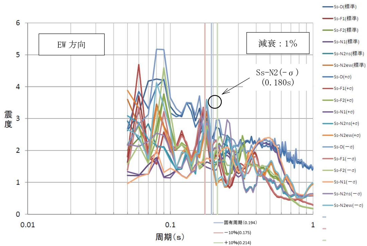
図 7.12-32 床応答スペクトル
