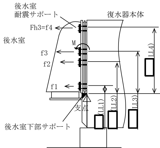
図 7.12-13 後水室耐震サポートにかかる水平力（鉛直曲げモーメント）
