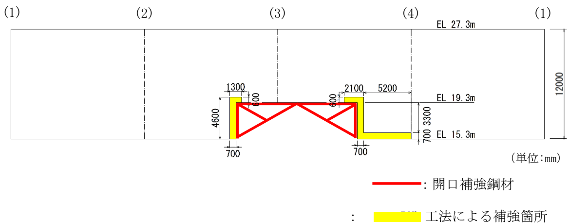
図 1.2-4 復水貯蔵タンク遮蔽壁の Phb 工法による耐震補強箇所及び開口補強鋼材概念図 (展開図)
