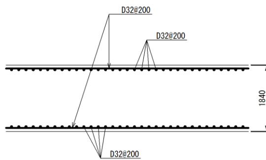
図 2.2-12(1) トーラス水受入タンク遮蔽壁の概略配筋図
