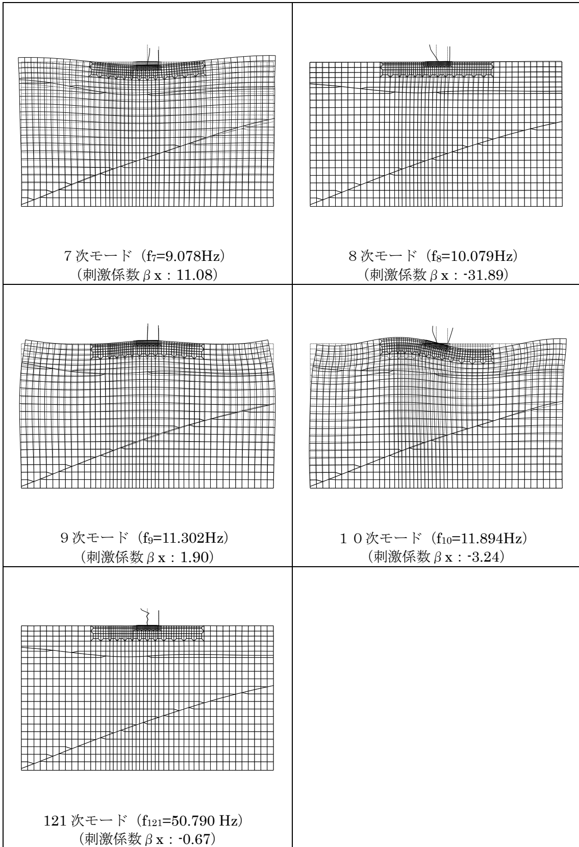
図 1.3-14 固有値解析結果におけるモード図
