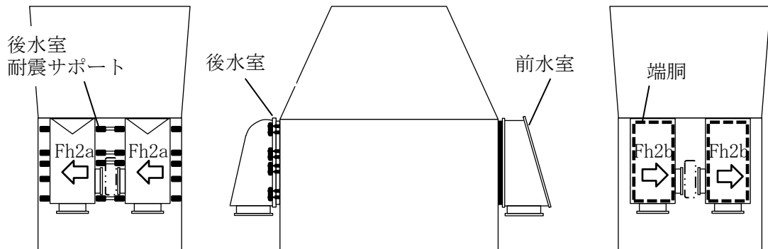
図 7.12-10 地震力が復水器細管軸直方向に作用した場合
