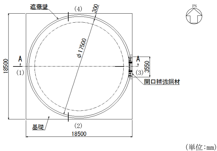
図 2.2-8 トーラス水受入タンク遮蔽壁の平面図
