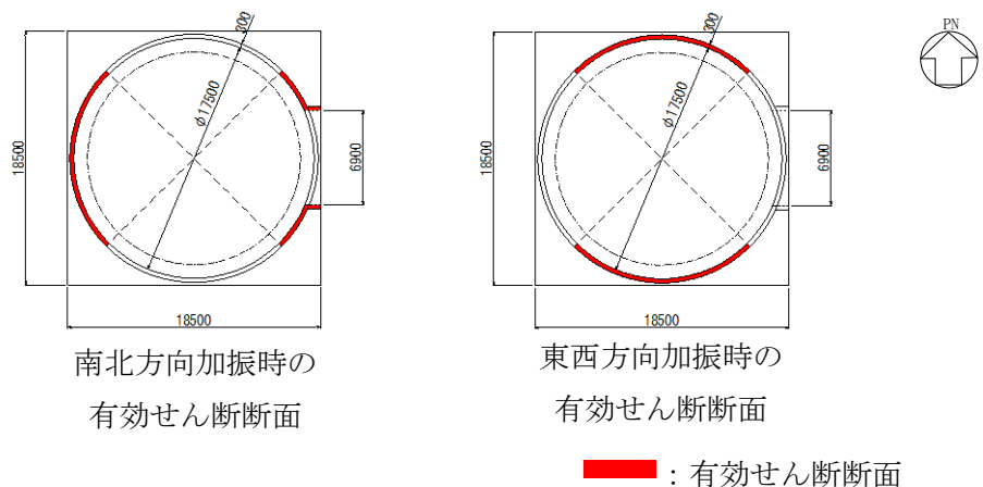
図 2.2-15 有効せん断断面積の比較
