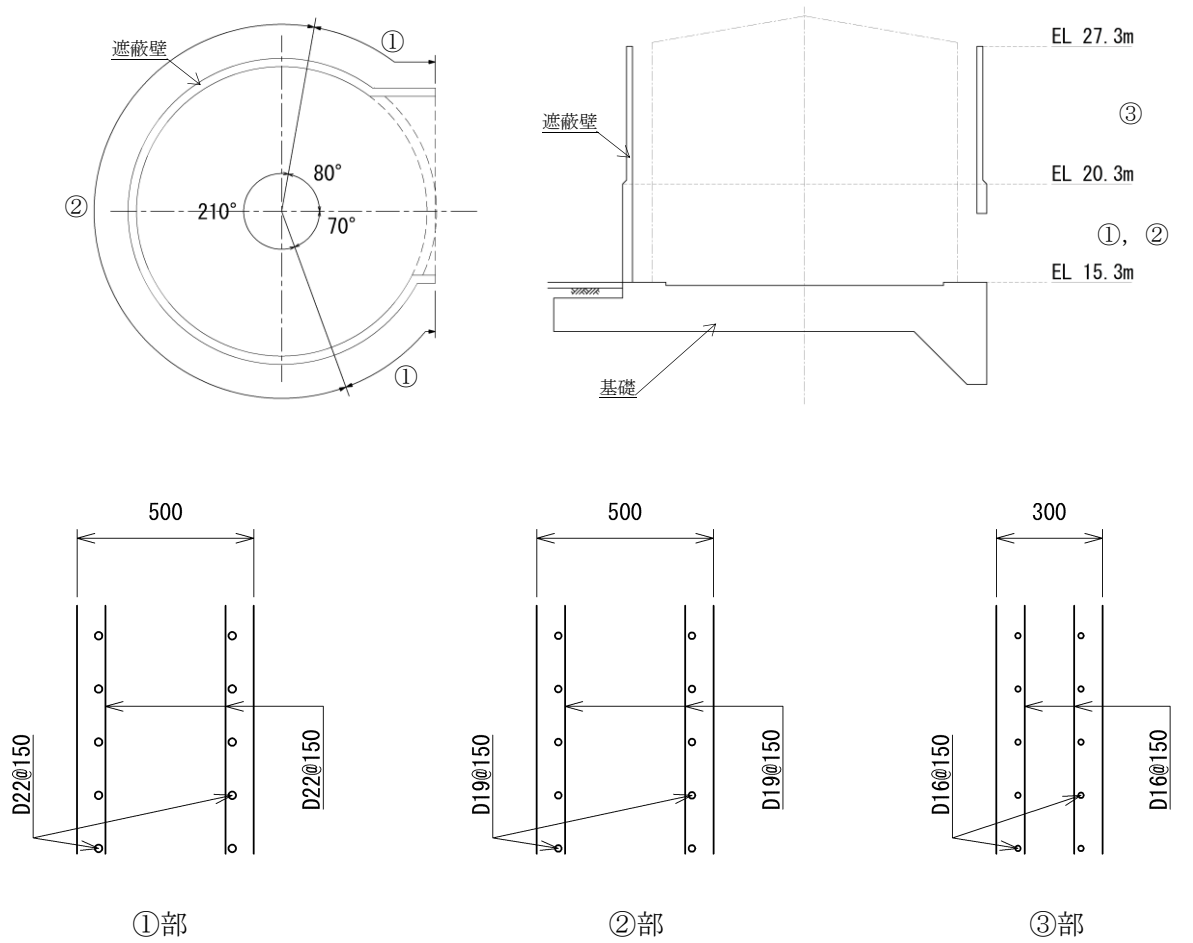
図 1.2-6(1) 復水貯蔵タンク遮蔽壁の概略配筋図 (遮蔽壁)
