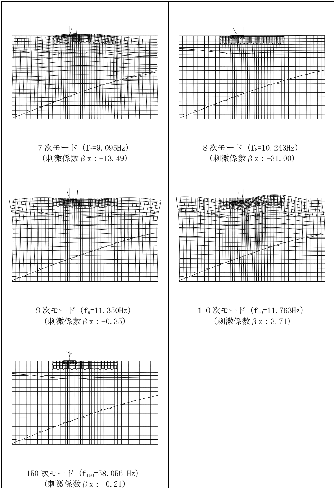
図 2.3-14 固有値解析結果におけるモード図
