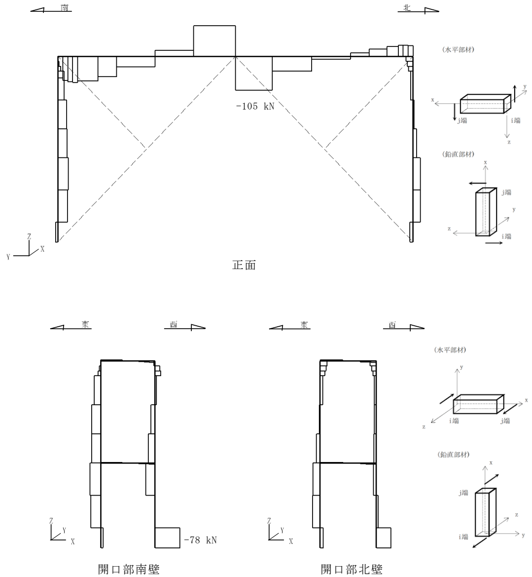
図 2.6-10 断面力分布図 (杵材) (せん断力 (kN) : Q_z ) (解析ケース①, S_s - D (++) )
