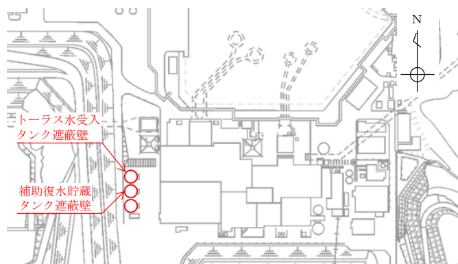
図1-2 補助復水貯蔵タンク遮蔽壁及びトールラス水受入タンク遮蔽壁の配置図
