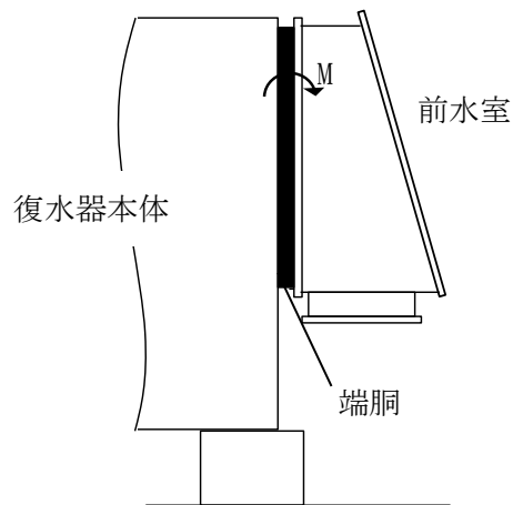
図 7.12-14 端胴にかかる曲げモーメント（鉛直曲げモーメント）
