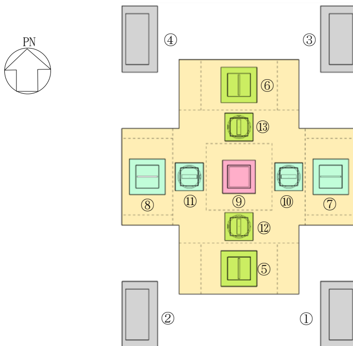
図 7.12-26 細管軸直方向 (EW 方向) に卓越した地震動による地震時機器荷重(2/2)
