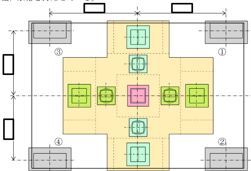
図 7.12-23 鉛直下向き荷重を受ける復水器基礎台配置図 (平面図)
