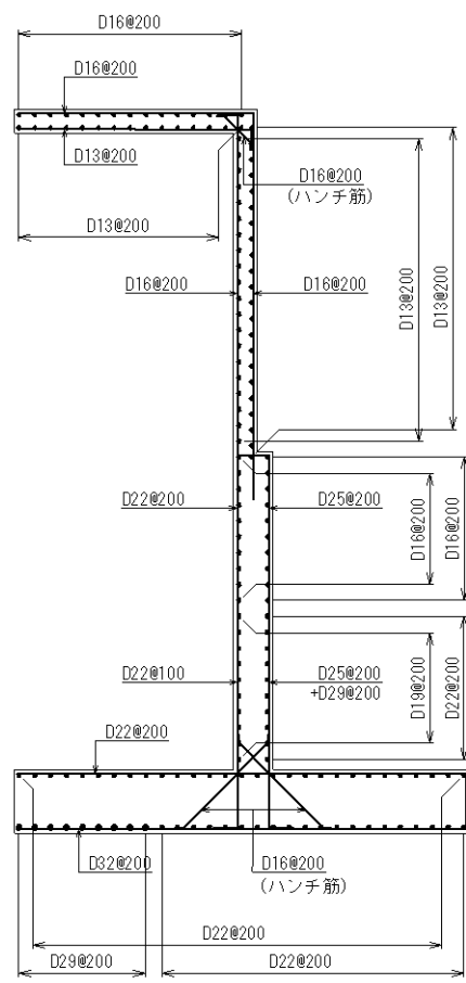
図 1.2-6(4) 復水貯蔵タンク遮蔽壁の概略配筋図 (弁室)
