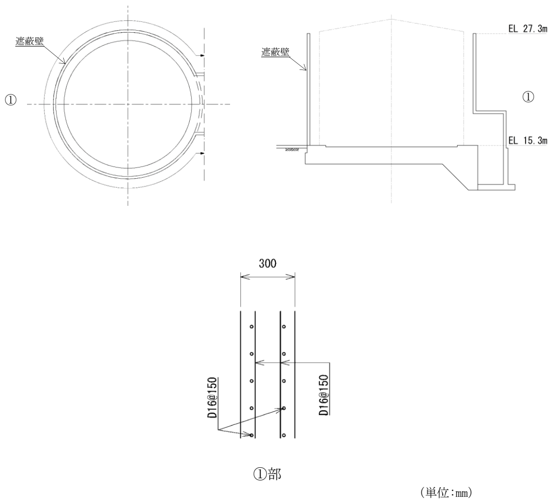
図 2.2-6(1) 補助復水貯蔵タンク遮蔽壁の概略配筋図
