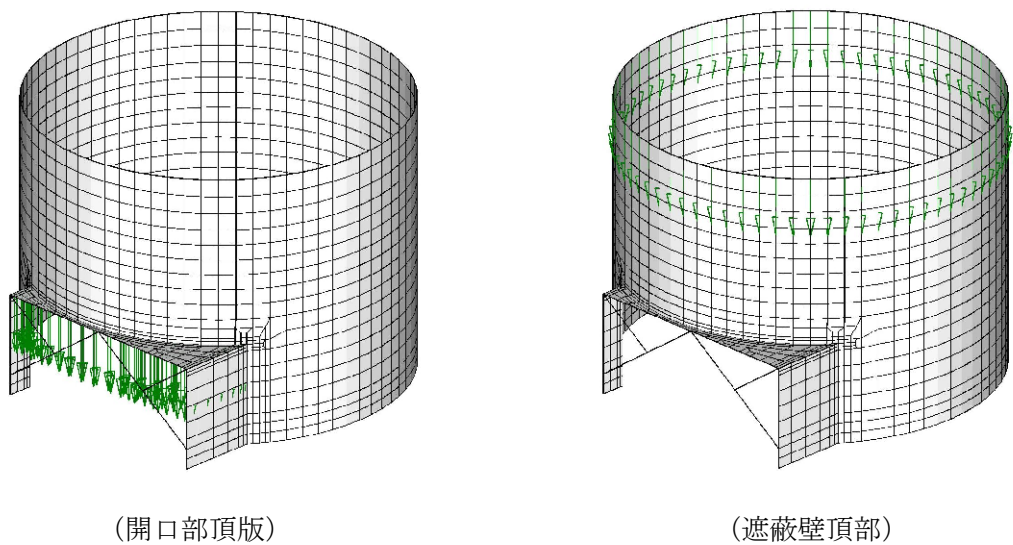
図 1.4-6 荷重載荷図 (積雪荷重)
