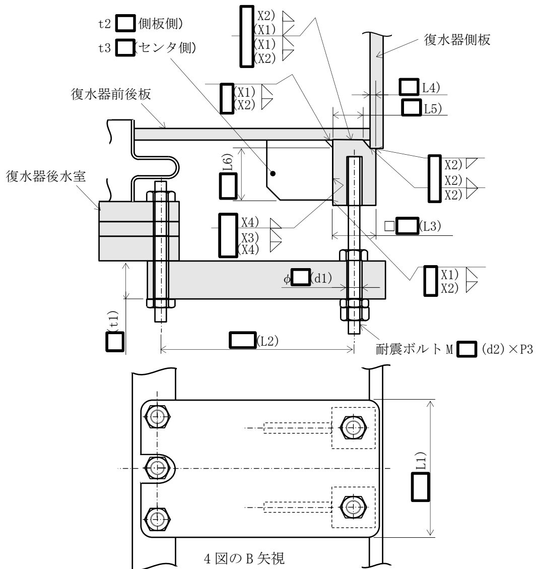
図 7.12-7 後水室耐震サポートの形状 (代表例)
