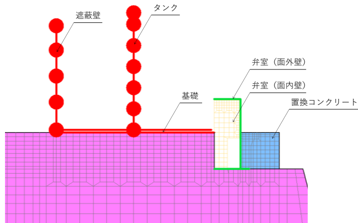
(拡大図)
