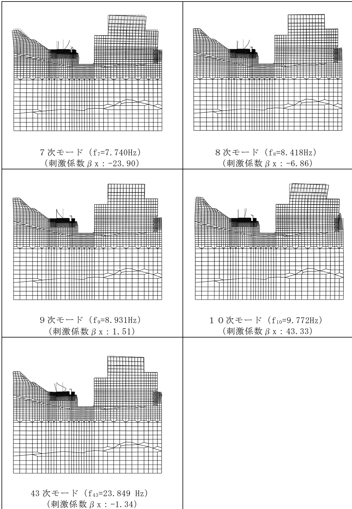
図 3-17 固有値解析におけるモード図 (B-B断面, 弁室面内壁無し)
