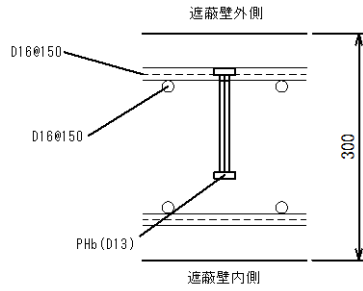
図 2.2-12(3) トーラス水受入タンク遮蔽壁の概略配筋図 (PHb 工法)
