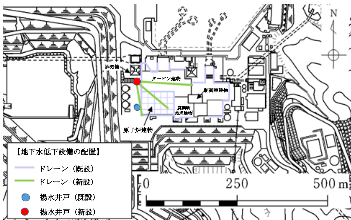
図7.5-1 地下水水位低下設備の概略図
