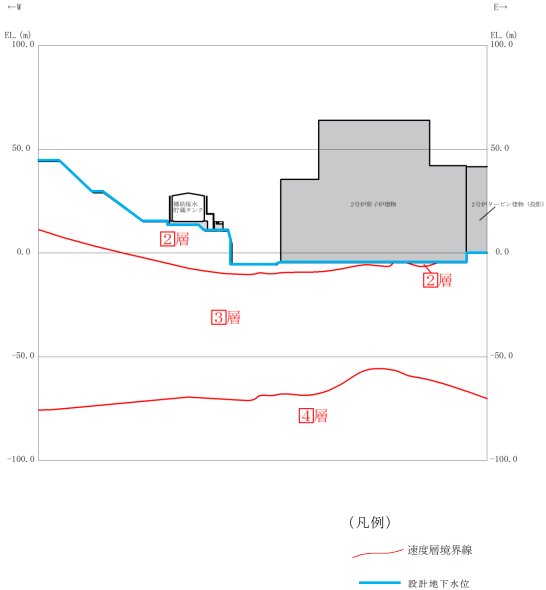
図2-3 設計地下水位 (B-B断面)
