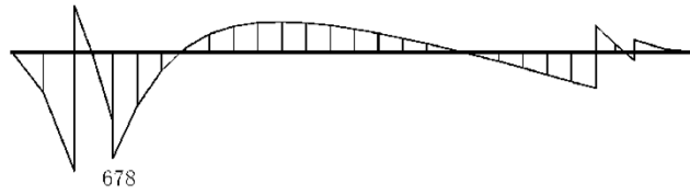
数值：評価位置における断面力 (a) 曲げモーメント (kN・m)
