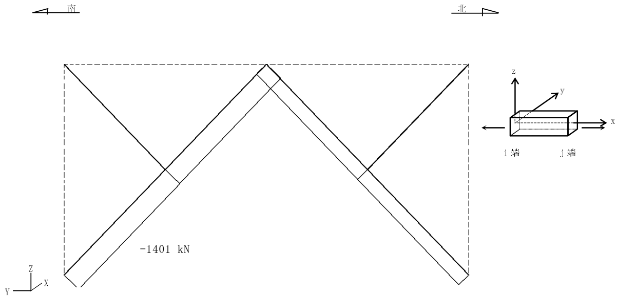
図 2.6-12 断面力分布図 (ブレース材) (軸力 (kN) : N) (解析ケース①, S s - D (++) )
