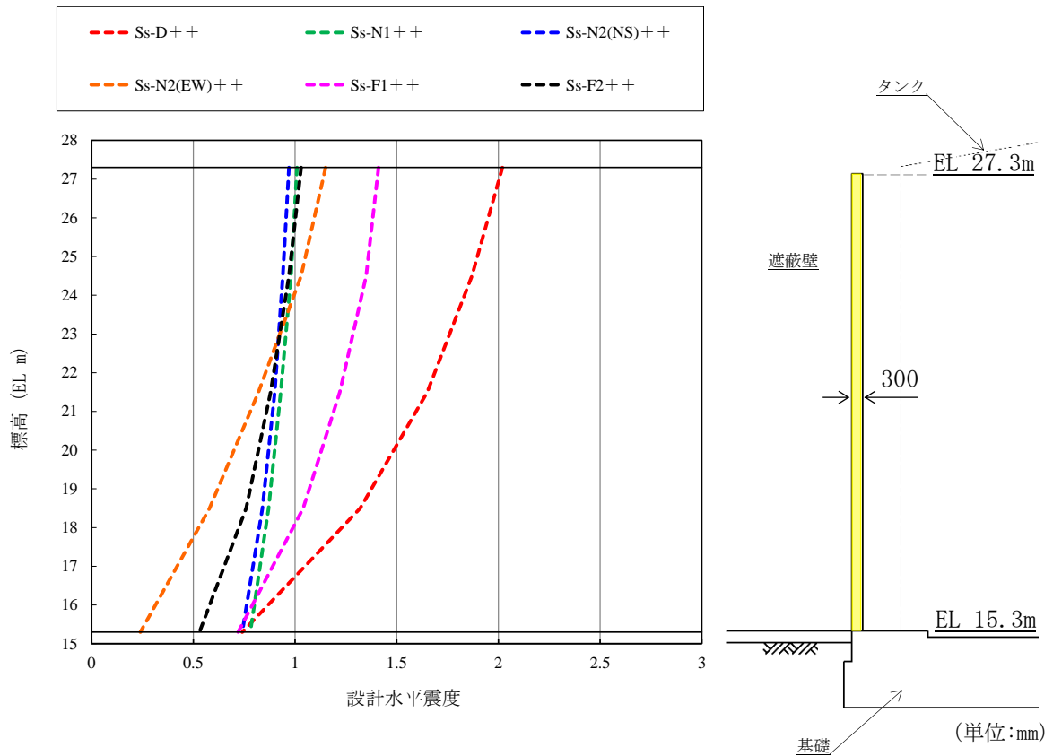
図 2.3-40 水平相対変位最大時刻における設計水平震度
