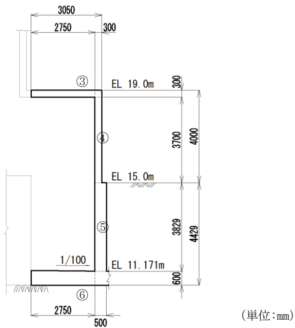
(弁室)
