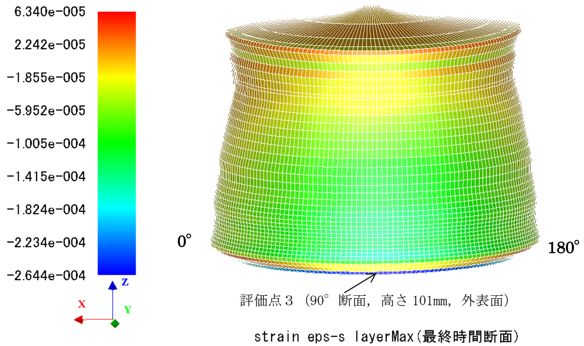
図 5-18 解析終了時外表面軸方向ひずみ (変形倍率 500 倍)
