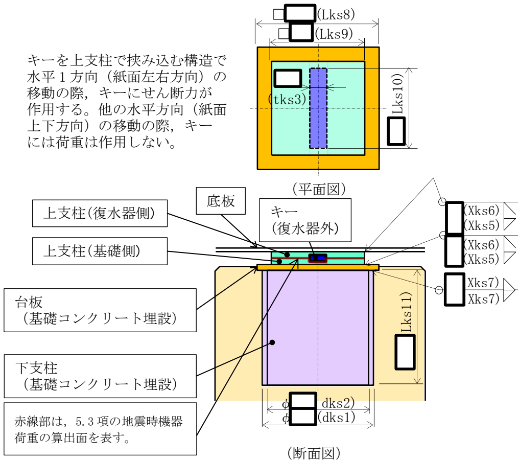
図 7.12-17 キーサポート⑩⑪平面図，断面図
