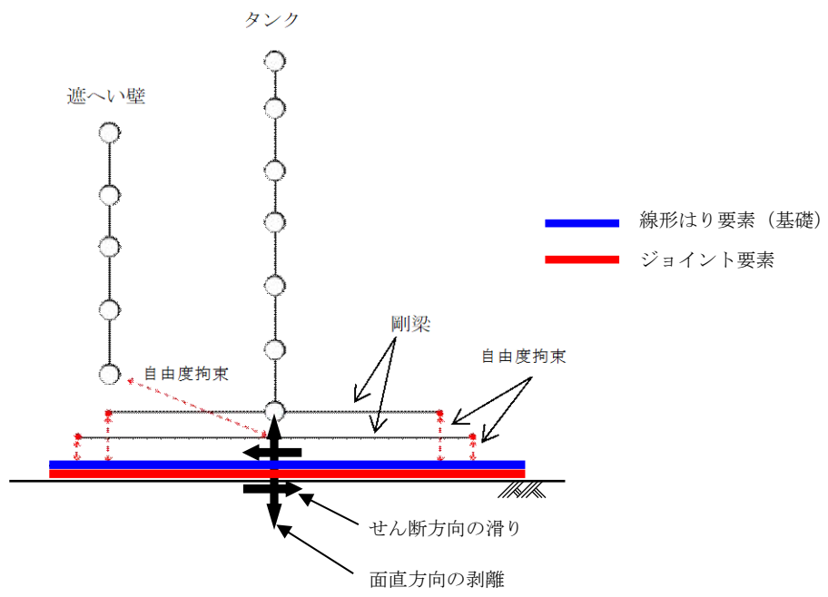
図 2.3-10 ジョイント要素の配置概念図
