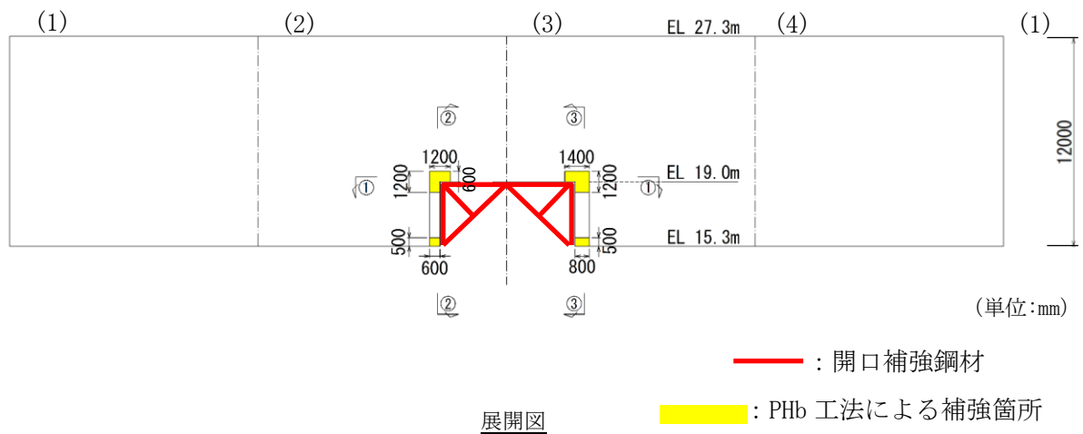
図 2.2-4(1) 補助復水貯蔵タンク遮蔽壁の PHb 工法による耐震補強箇所 (展開図)
