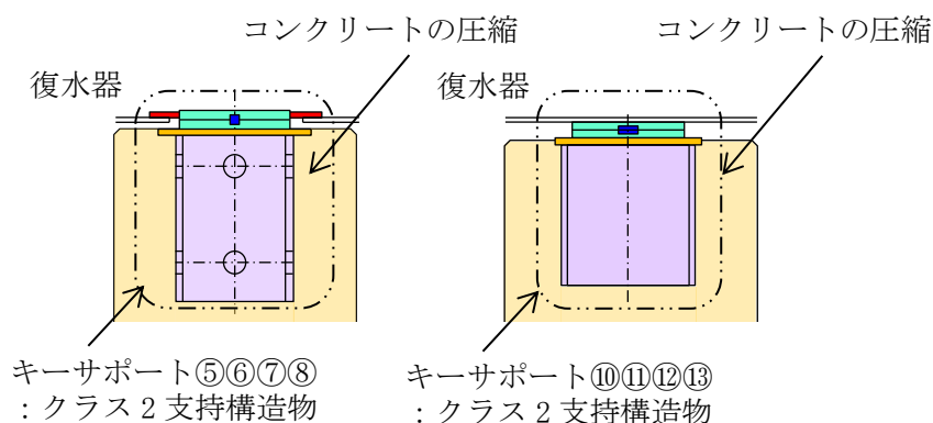
図 7.12-21 基礎部耐震サポートの評価部位と評価条件
