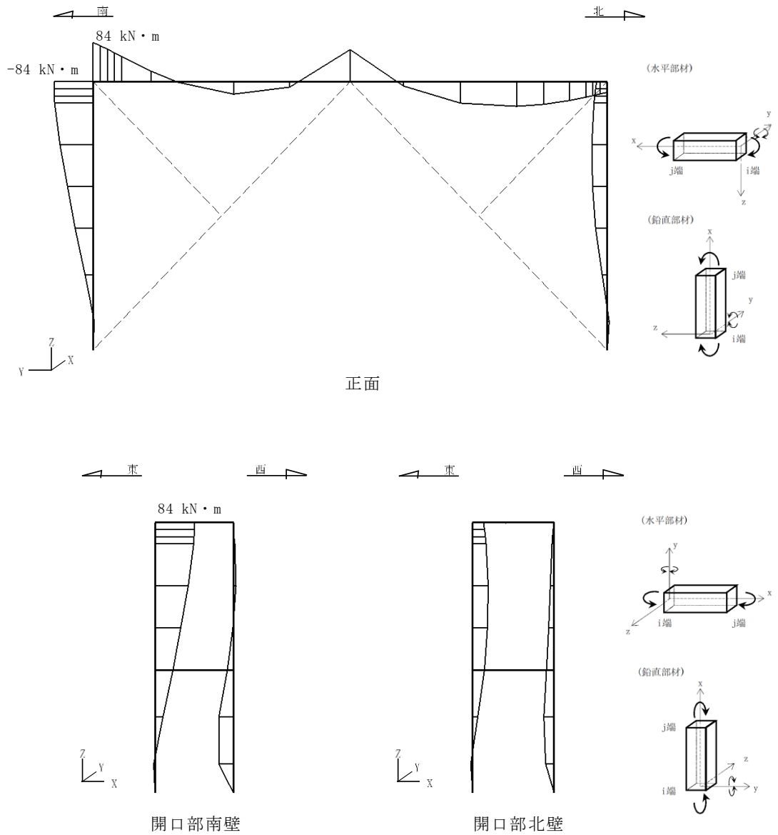
図 2.6-7 断面力分布図 (枠材) (曲げモーメント (kN・m) : M_y ) (解析ケース①, S_s - D (++) )
