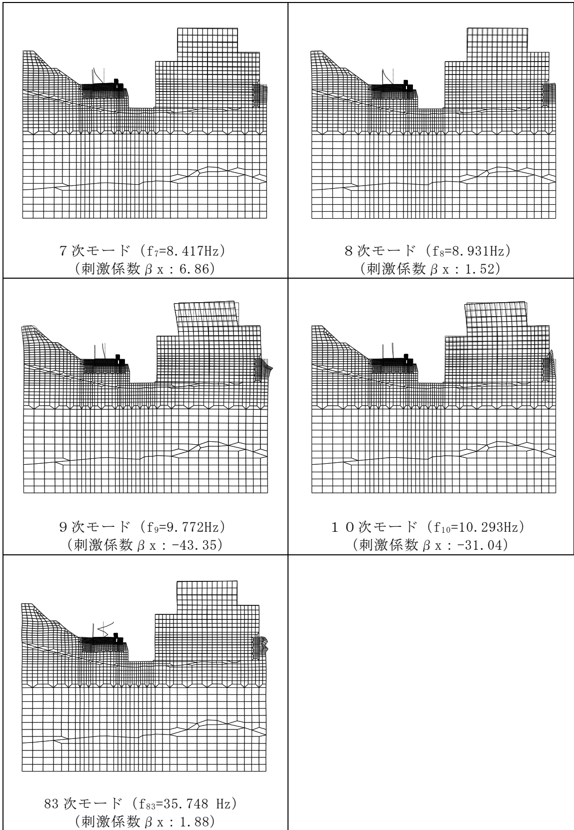
図 3-14 固有値解析におけるモード図 (B-B断面, 弁室面内壁有り)
