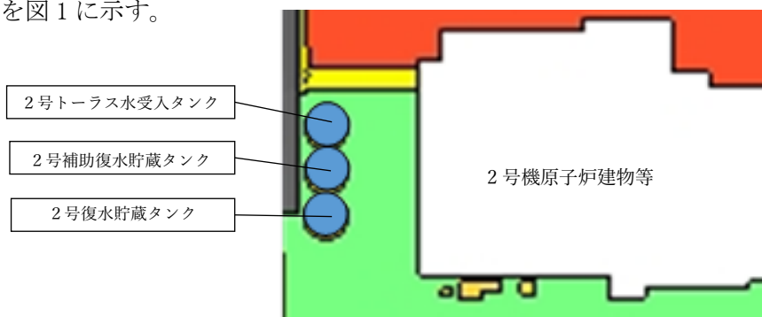
図1 2号復水貯蔵タンク等のモデル化位置
