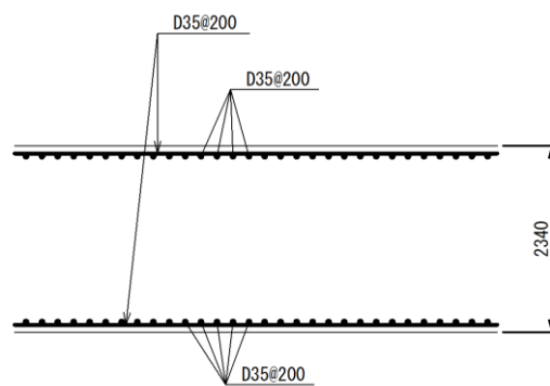
図 1.2-6(2) 復水貯蔵タンク遮蔽壁の概略配筋図 (基礎)
