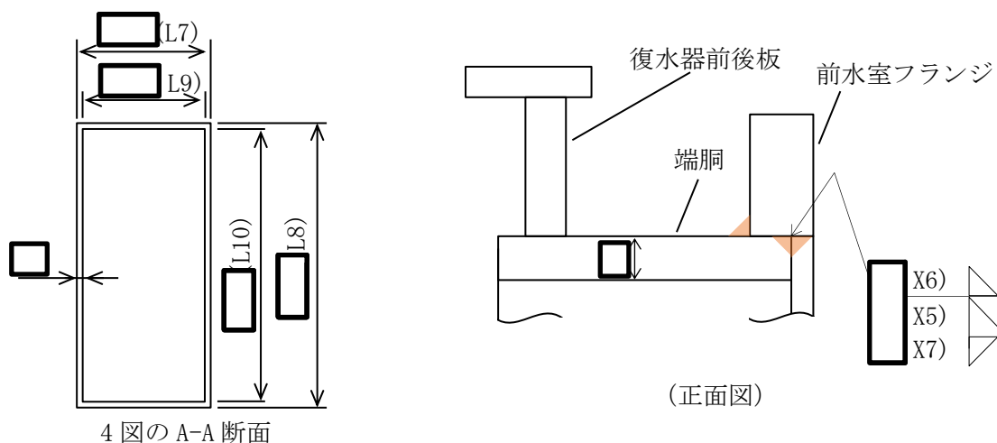
図 7.12-6 端胴の溶接形状
