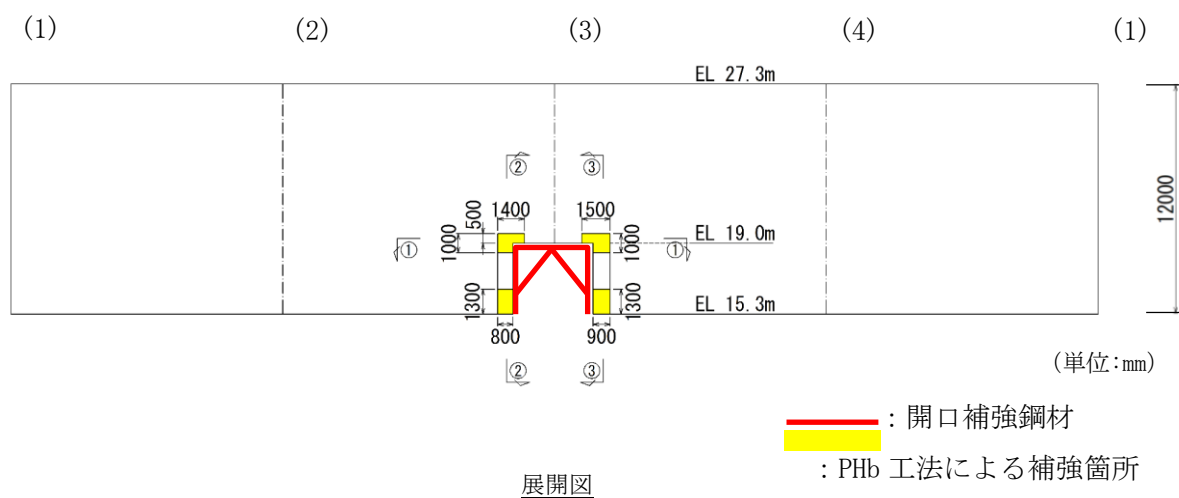
図 2.2-10(1) トーラス水受入タンク遮蔽壁の PHb 工法による耐震補強箇所
