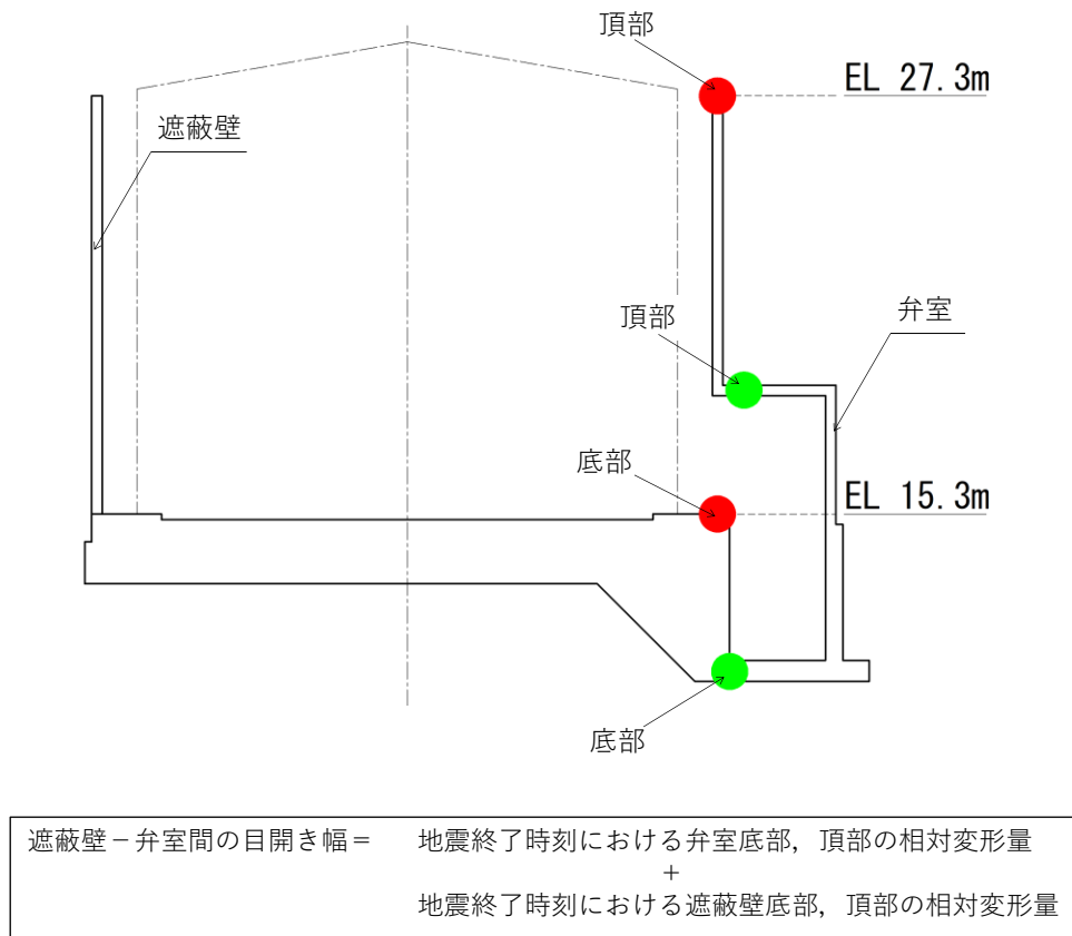
図4-4 目開き幅算定の概念図
