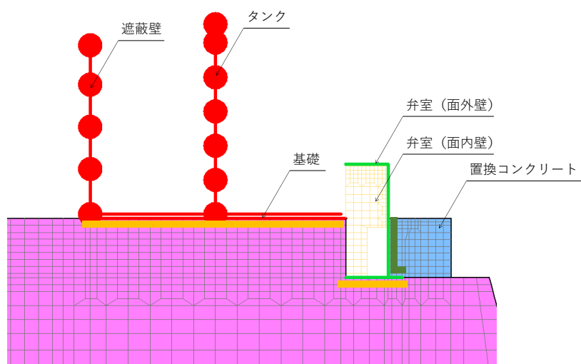
(拡大図)
