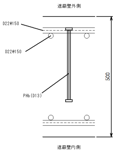
図 1.2-6(3) 復水貯蔵タンク遮蔽壁の概略配筋図 (PHb 工法)
