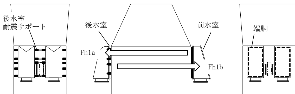
図 7.12-9 地震力が復水器細管軸方向に作用した場合
