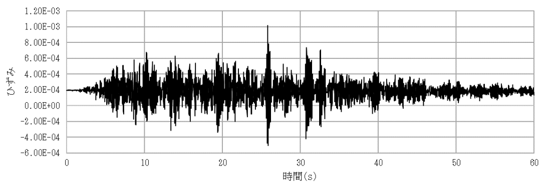
図 5-15 評価点 2 における周方向ひずみ時刻歴
