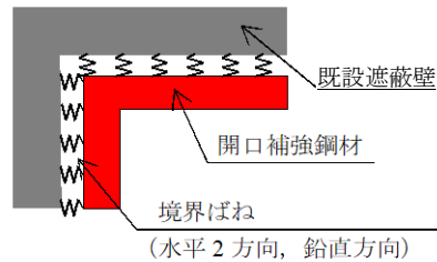
図 1.4-1 開口補強鋼材と遮蔽壁間の概念図
