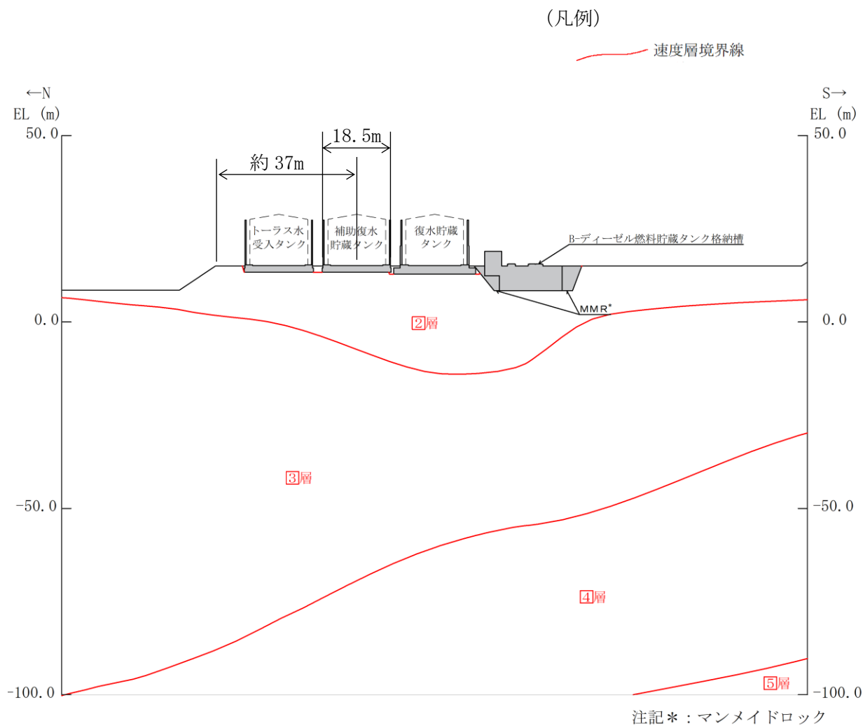
図 2.3-7 地表面形状設定の考え方
