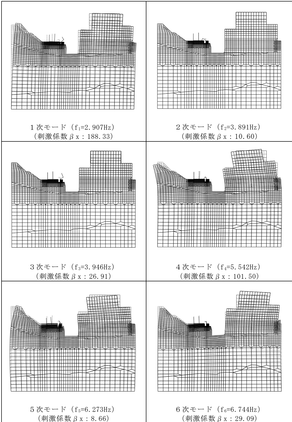
図 3-16 固有値解析におけるモード図 (B-B 断面, 弁室面内壁無し)
