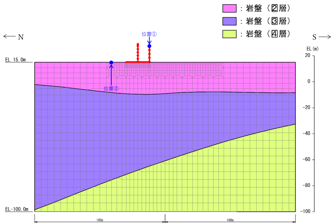
図4 本文で用いたモデル（モデル②）
