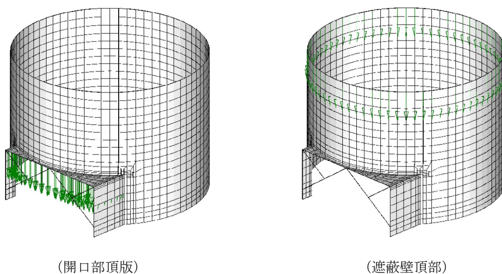
図 2.4-7 荷重載荷図 (積雪荷重)
