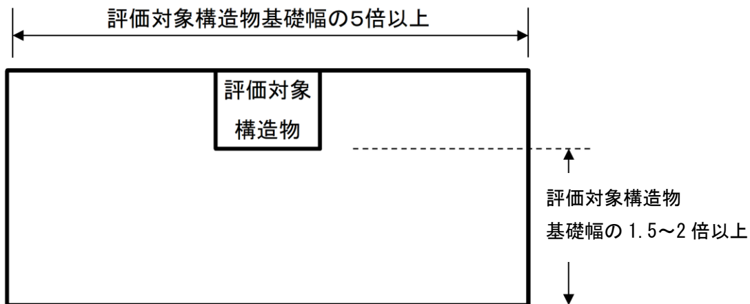
図 1.3-2 モデル化範囲の考え方
