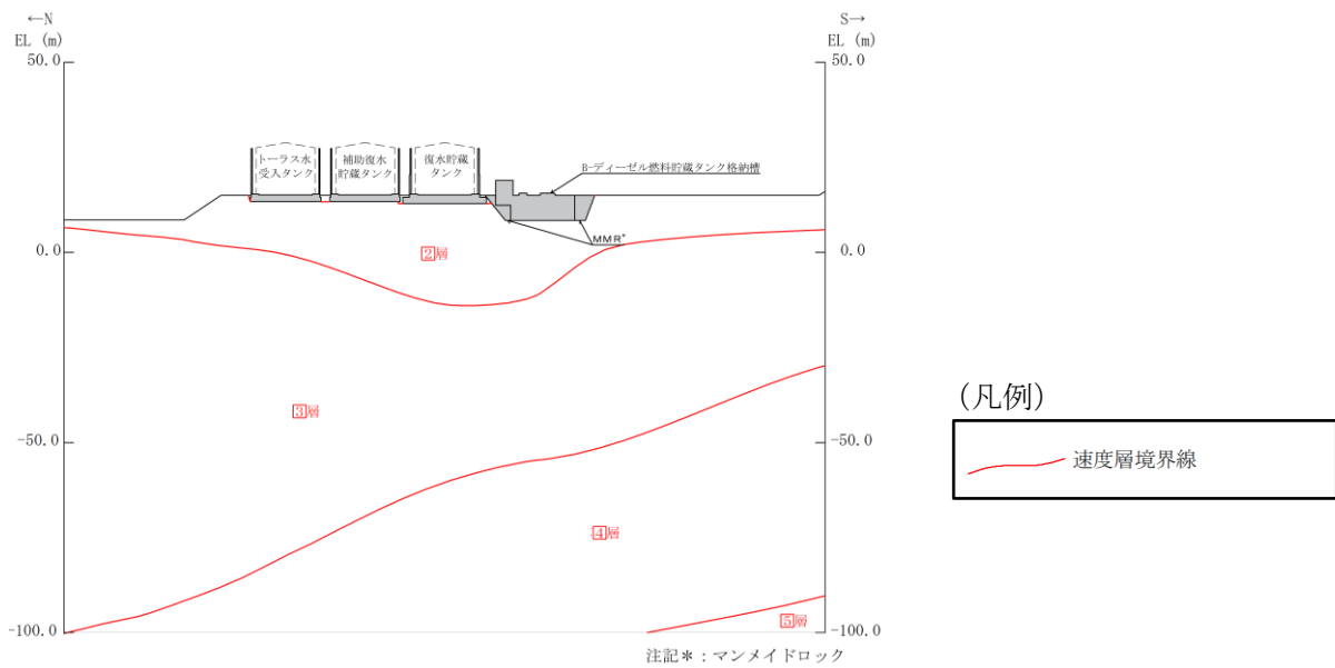
(速度層図)
