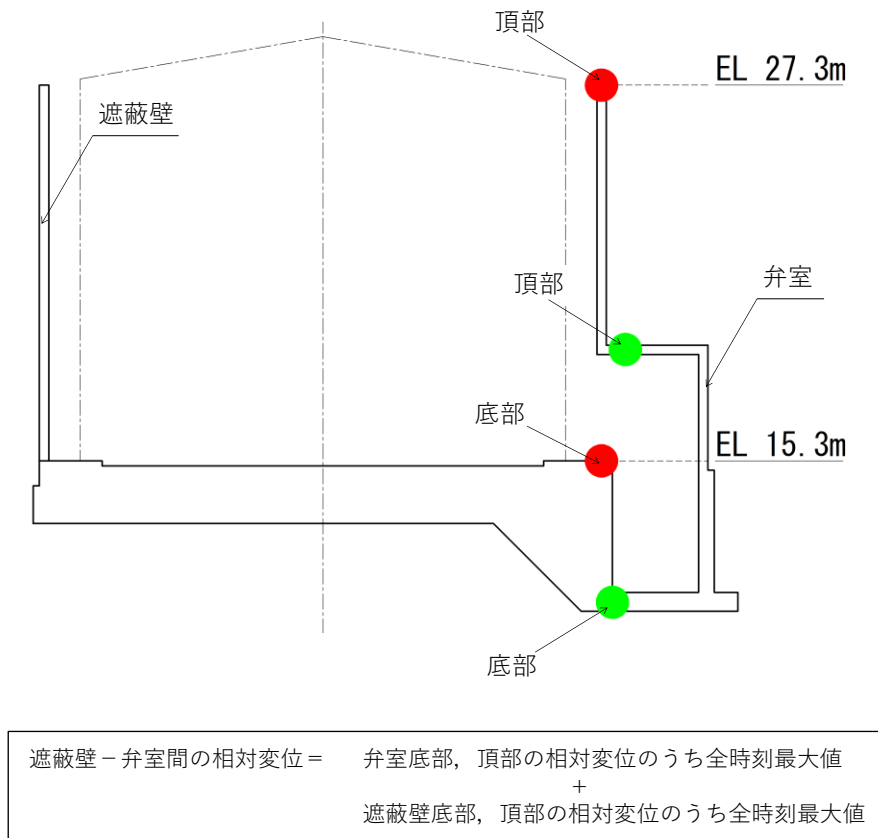
図4-6 遮蔽壁－弁室間の相対変位算定の概念図(1/2)
