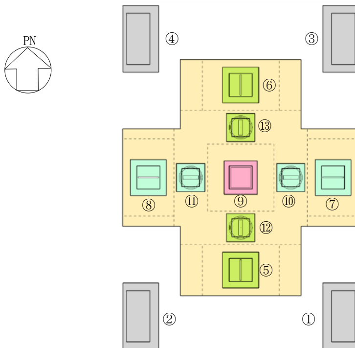
図 7.12-26 細管軸方向 (NS 方向) に卓越した地震動による地震時機器荷重(1/2)
