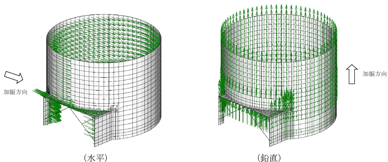
図 2.4-8 荷重载荷図（地震時荷重）
