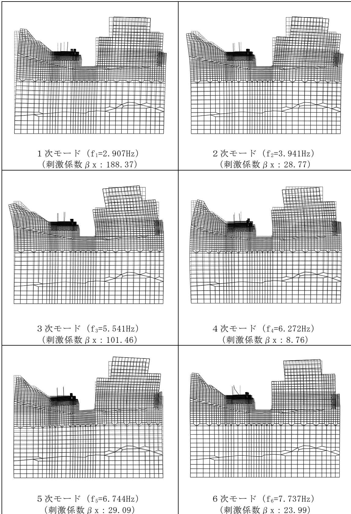
図 3-13 固有値解析におけるモード図 (B-B断面, 弁室面内壁有り)
