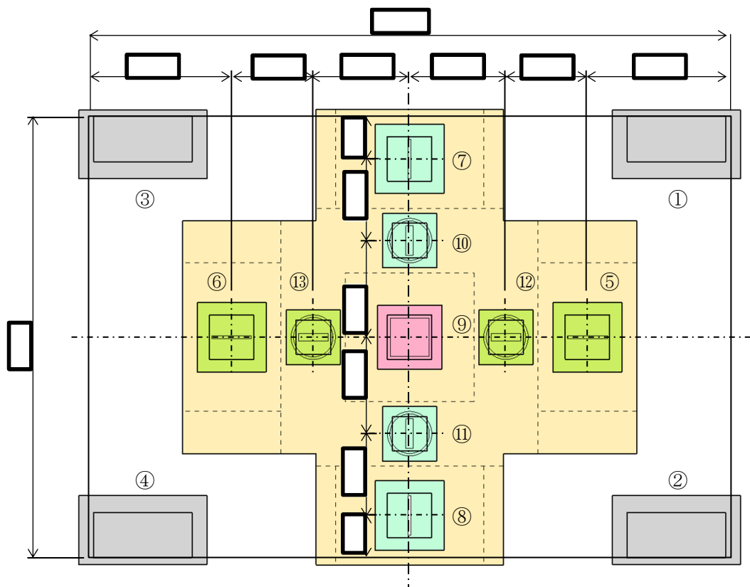
図 7.12-22 基礎部耐震サポート配置図
