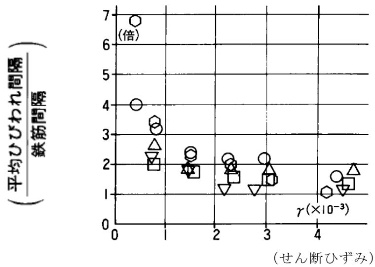
図 4-3 平均ひび割れ間隔 / 鉄筋間隔
