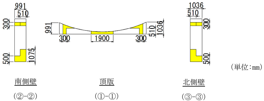
(展開図)
