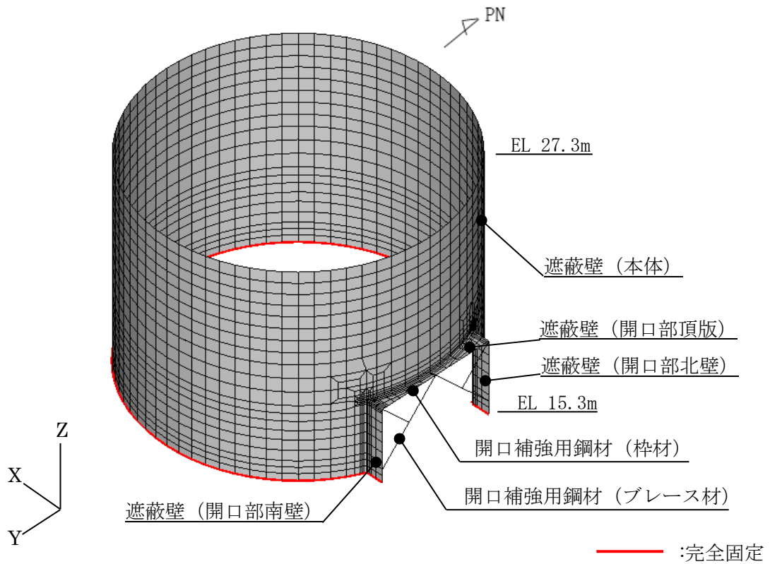
図 2.4-2(2) 3次元静的FEM解析モデル (鳥瞰図, 南東側から望む)
