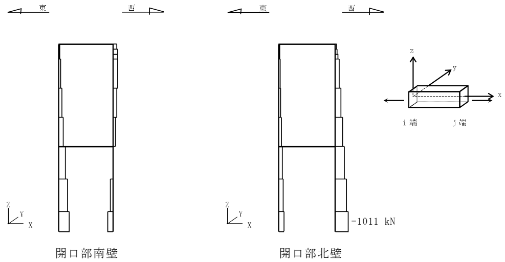
図 2.6-11 断面力分布図 (枠材) (軸力 (kN) : N) (解析ケース①, S s - D (++) )
