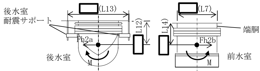
図 7.12-11 水室上から見た図(水平曲げモーメント)
