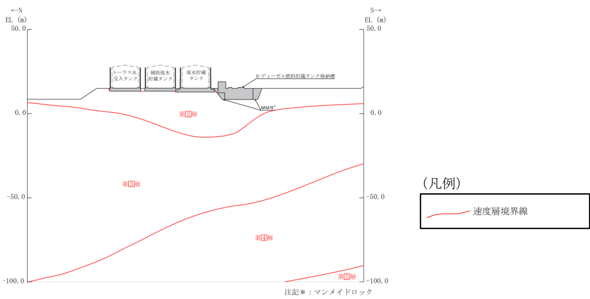
(速度層図)
