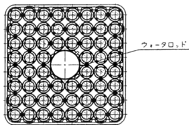
B-B 矢視図
