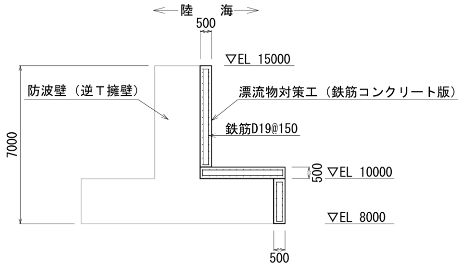
(概略配筋図 (断面図))
