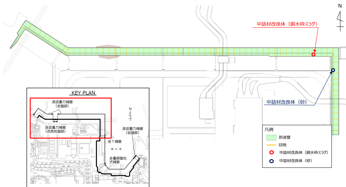
図3-2 中詰材改良体の試料採取位置
