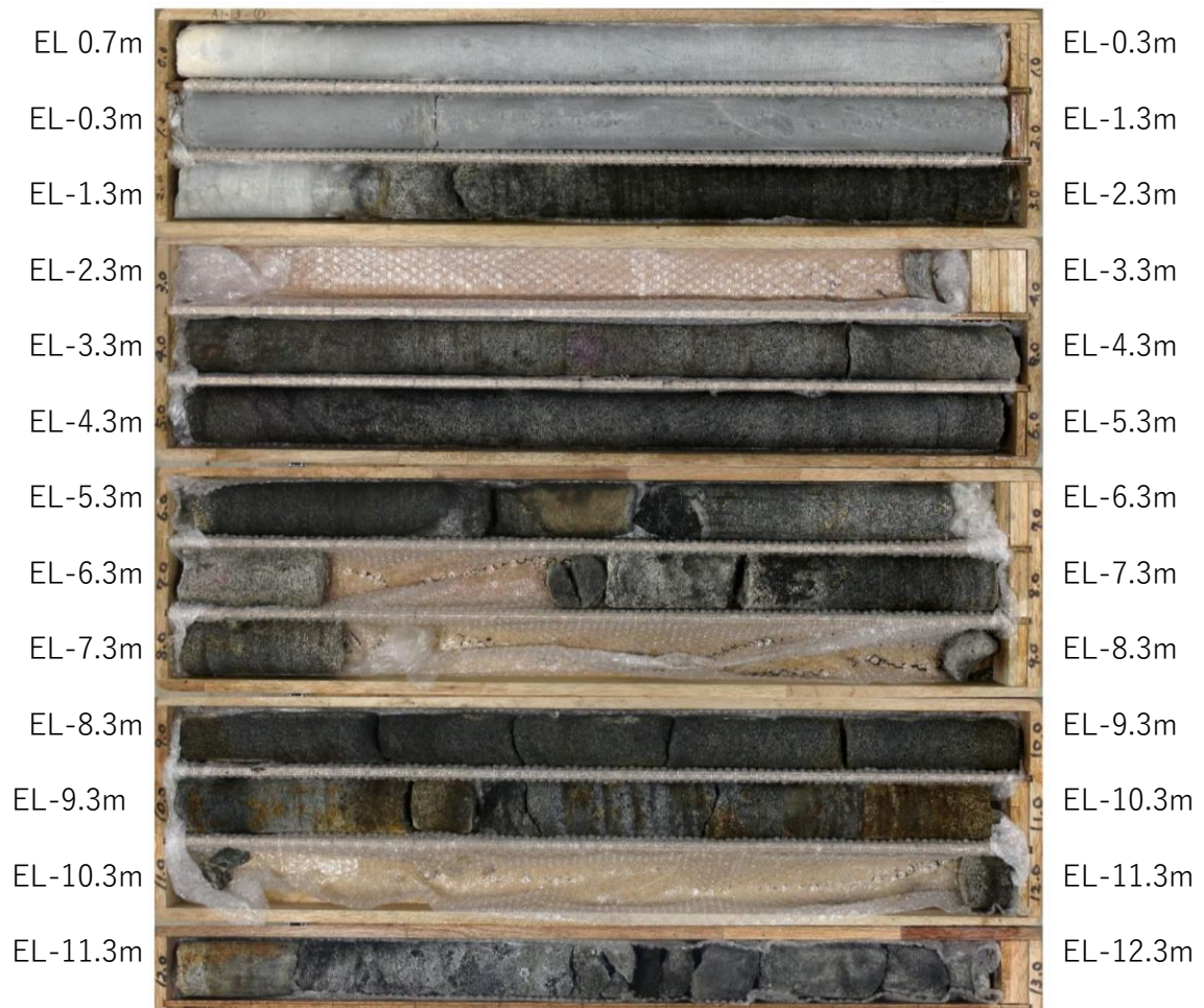
図 3-3 (1) 中詰材改良体 (銅水砕スラグ)
