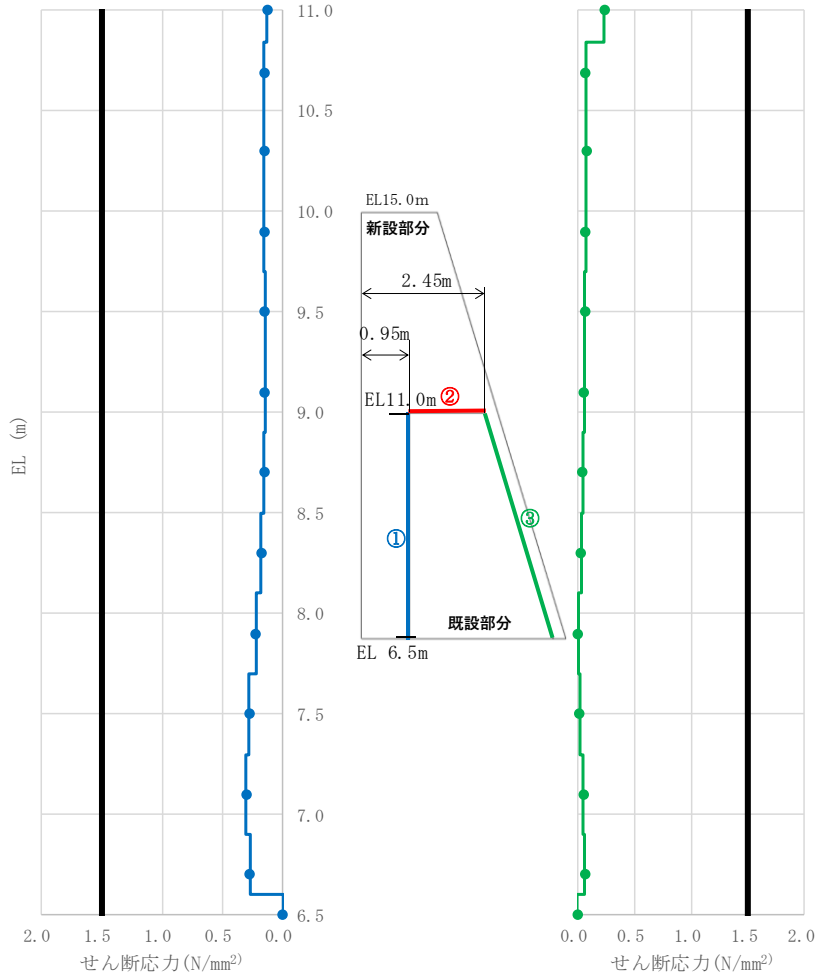
図 4.3.2-5(2) 新設部分と既設部分の境界部における発生応力図 (せん断応力) (地震時① 地震荷重作用方向：海方向)
