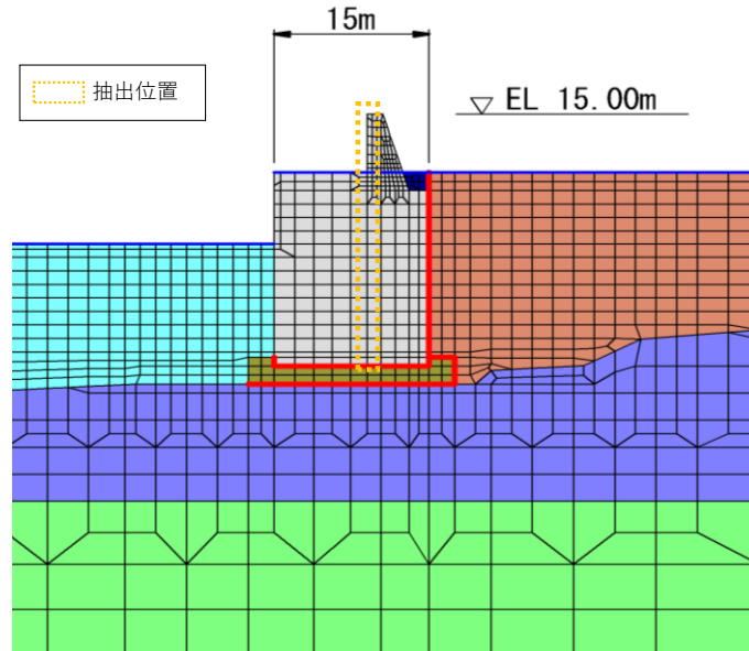
図 5.2.2-3(3) 応答加速度の抽出位置 (④-④断面)
