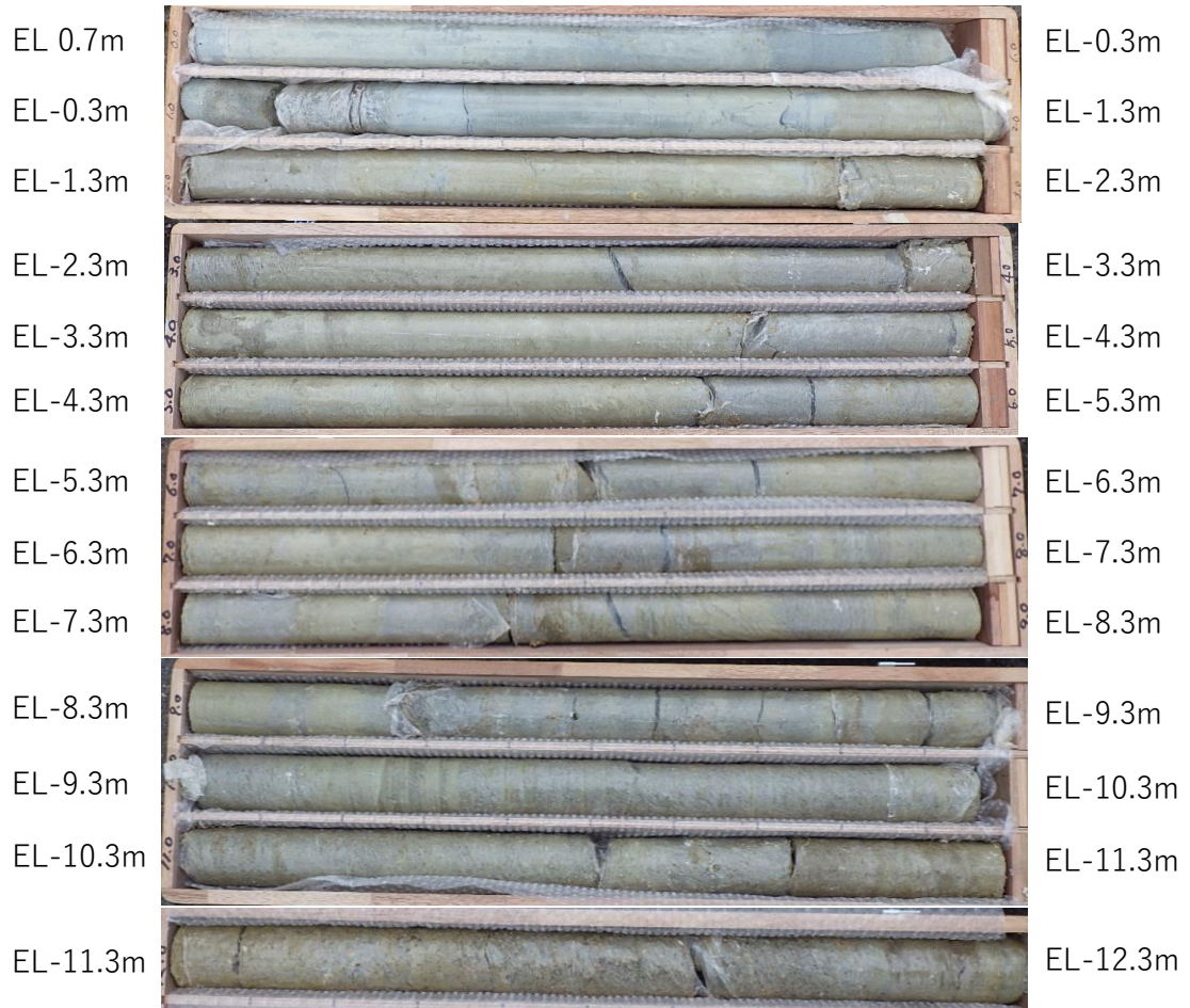
図 4-4 チェックボーリングのサンプリングコア
