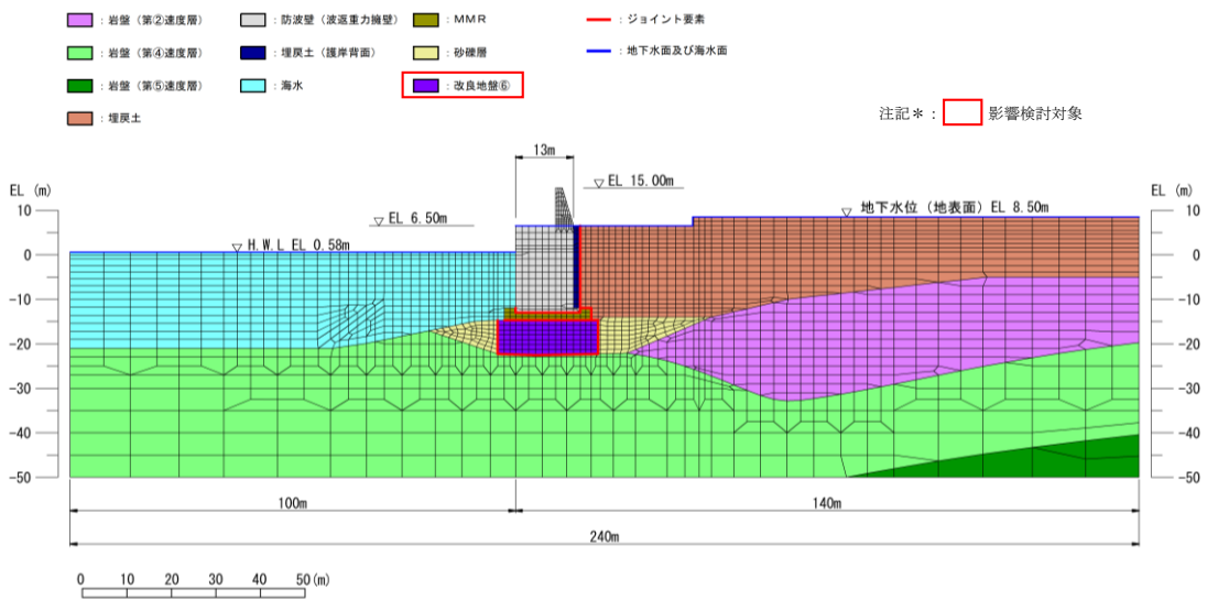
図 6.1.2-1 地震応答解析モデル（②-②断面）
