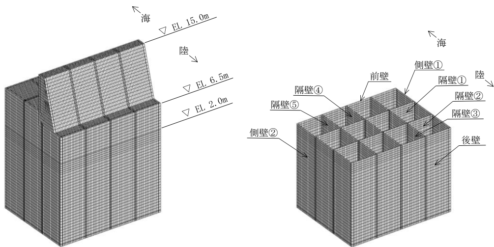
図 5.2.1-1(3) ケーソンの構造部材 (④-④断面)
