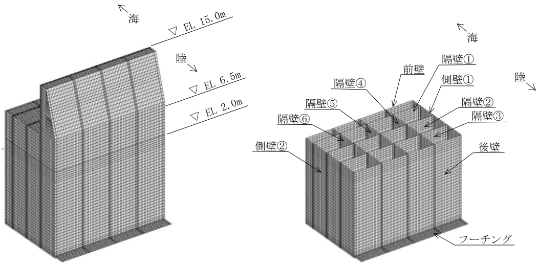
図 5.2.1-1(1) ケーソンの構造部材 (②-②断面)
