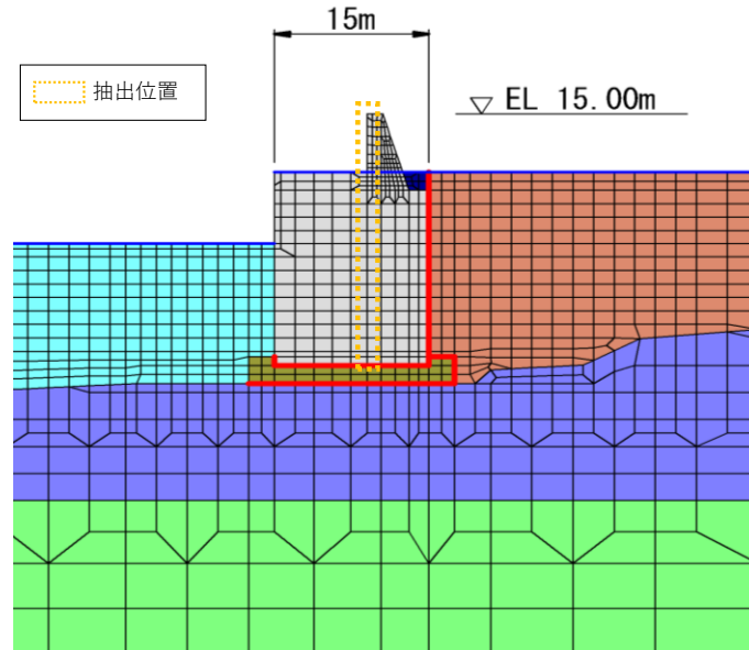
図 5.1.3-3(3) 応答加速度の抽出位置 (④-④断面)
