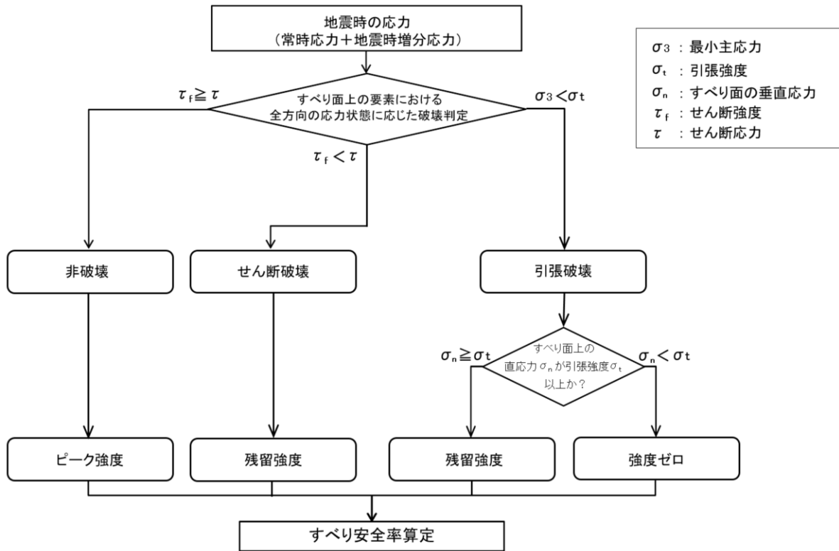
図 4.1.8-3 すべり安全率算定のフロー
