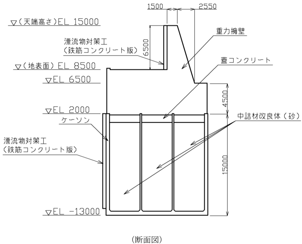
図 3.1-9(5) 防波壁 (波返重力擁壁) の構造図 (④-④断面)
