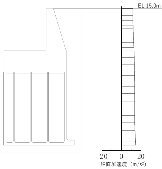
鉛直加速度
