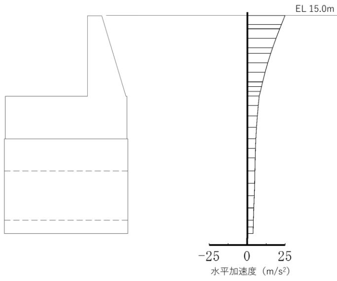
水平加速度
