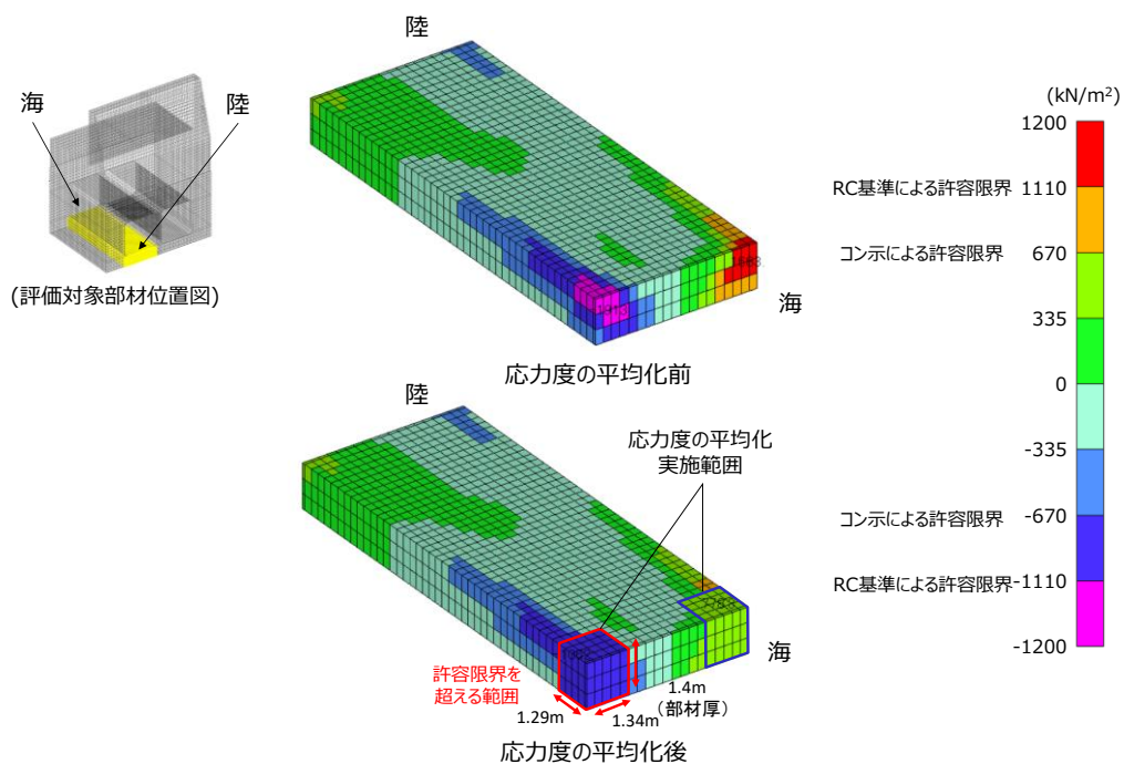
図 5.2.4-4 せん断（面外）応力度コンター図
