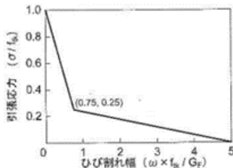
図 5.1.4-9 コンクリートの破壊エネルギー （「コンクリート標準示方書 2017」より引用）
