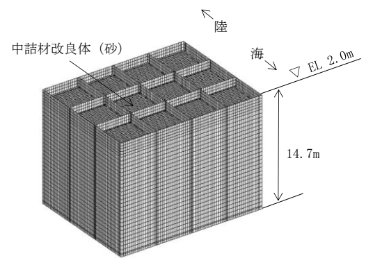
ケーソンのモデル図 (海側) *
