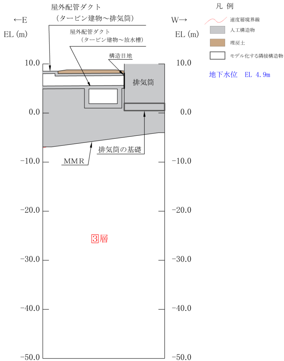
(速度層図)
