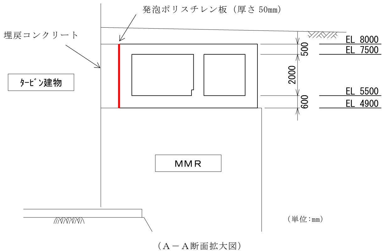
図4-17 2号機タービン建物と屋外配管ダクト（タービン建物～排気筒）間の発泡ポリスチレン板（50mm）の設置状況
