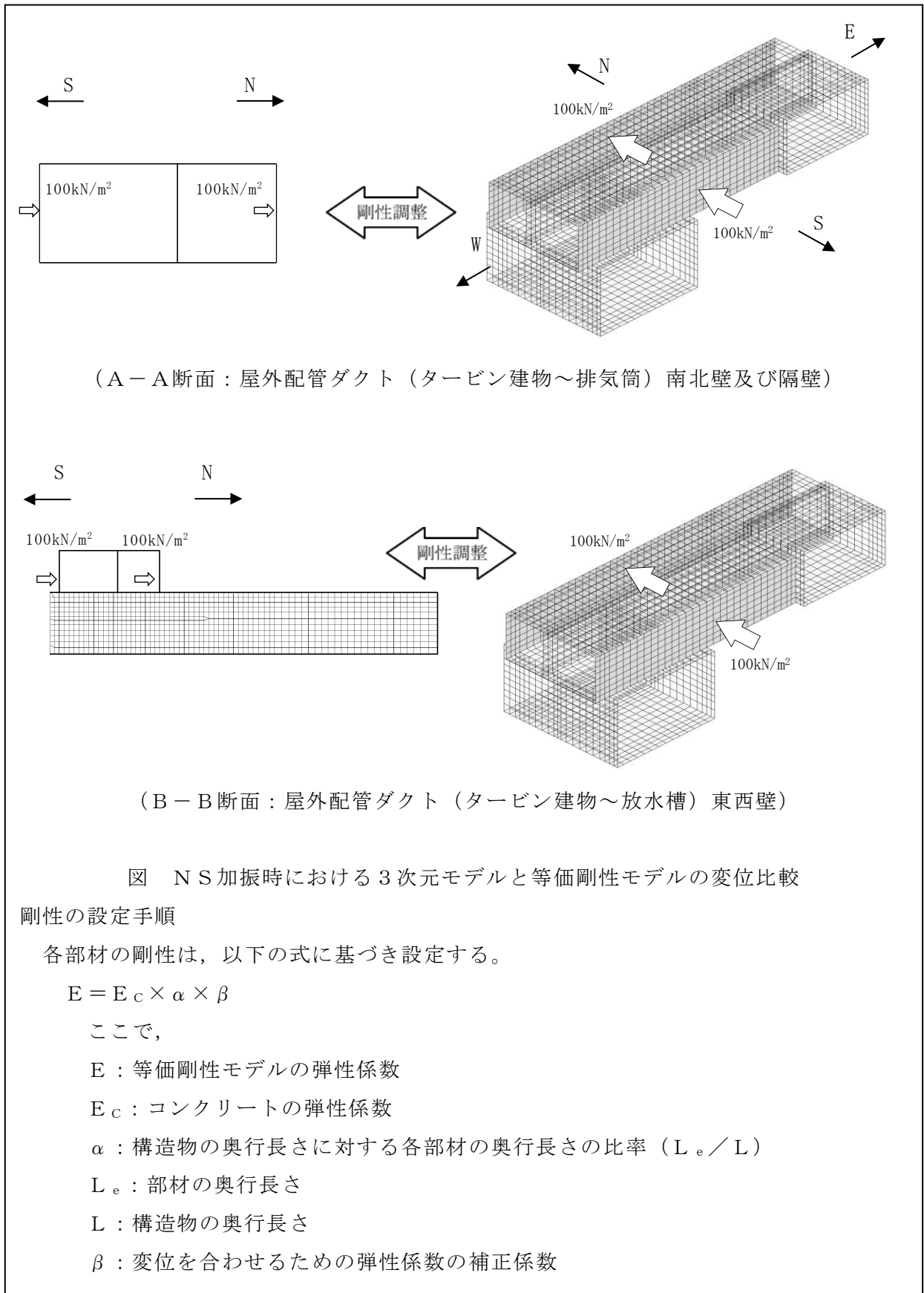
図 4-7 (1) 剛性の調整方法
