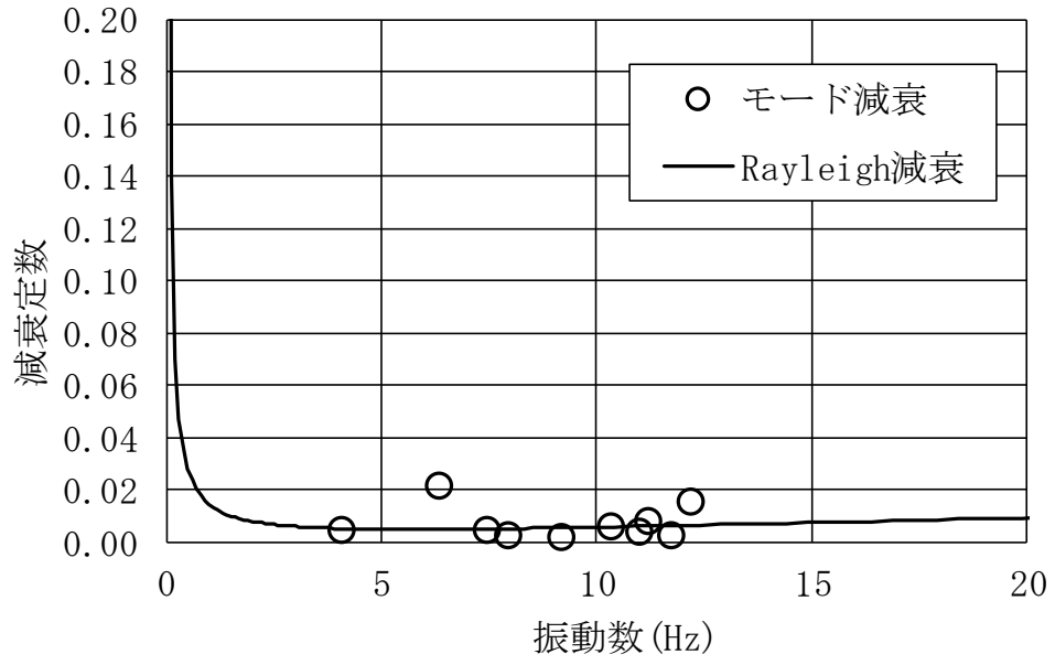
図 4-31 設定した Rayleigh 減衰 (C-C 断面)
