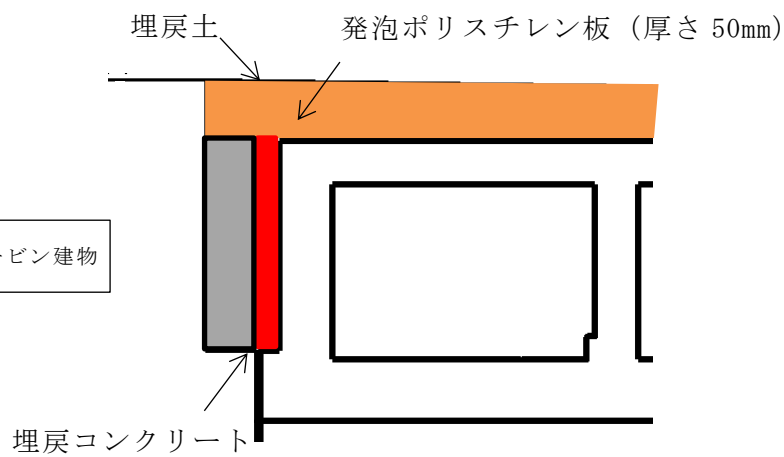
(B-B断面 対策工概念図)
