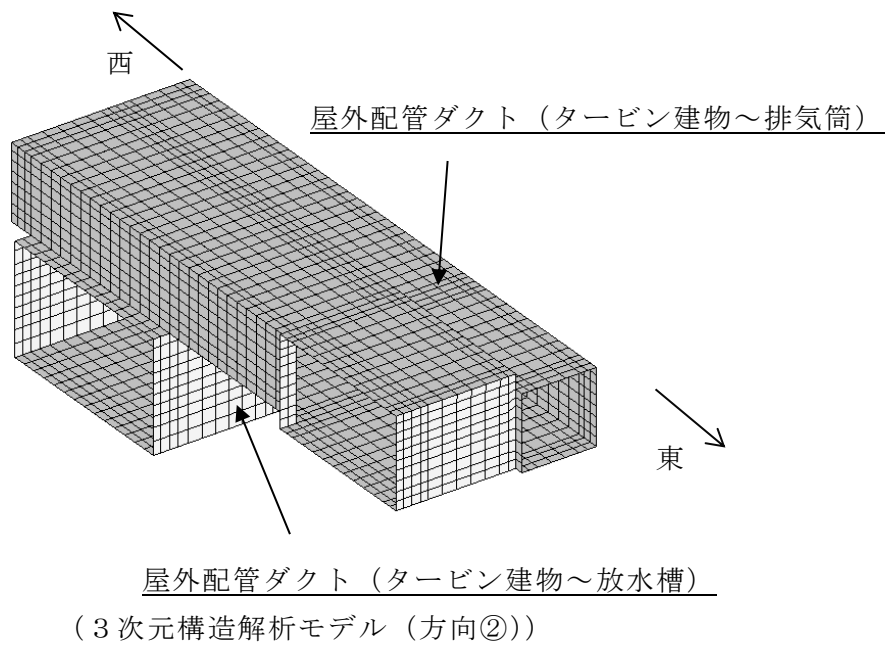
図 1-4 一体化部のイメージ図
