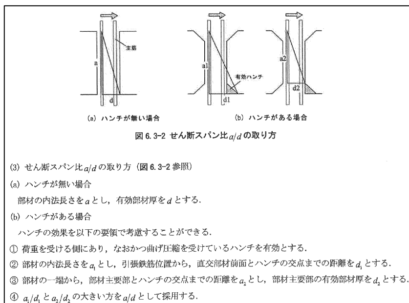
図 6-3 せん断スパン比の取り方
