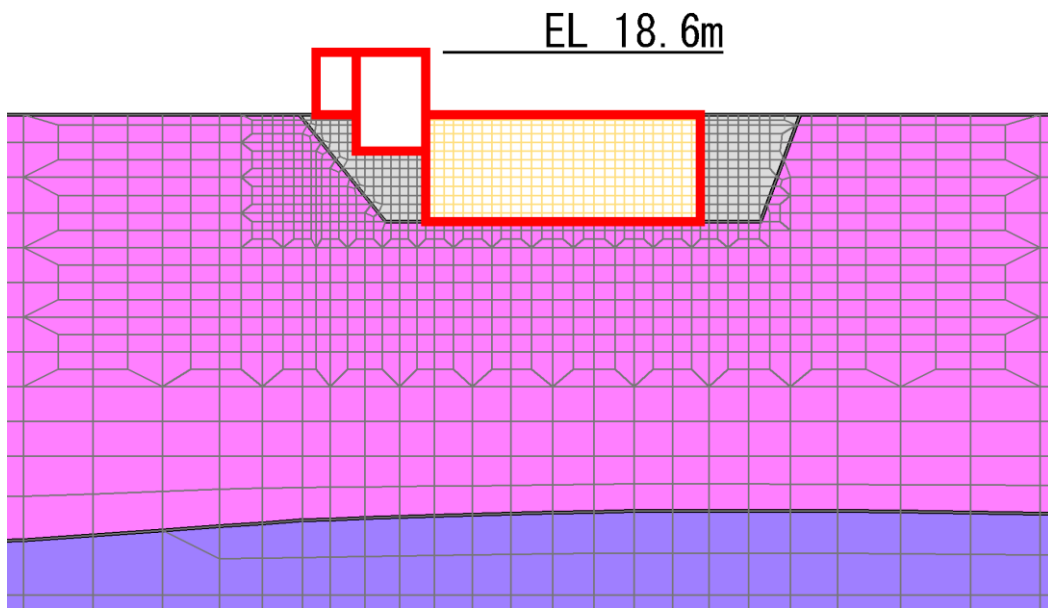
(拡大図)
