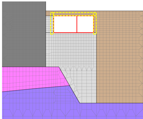
(NS方向 : A-A断面)
