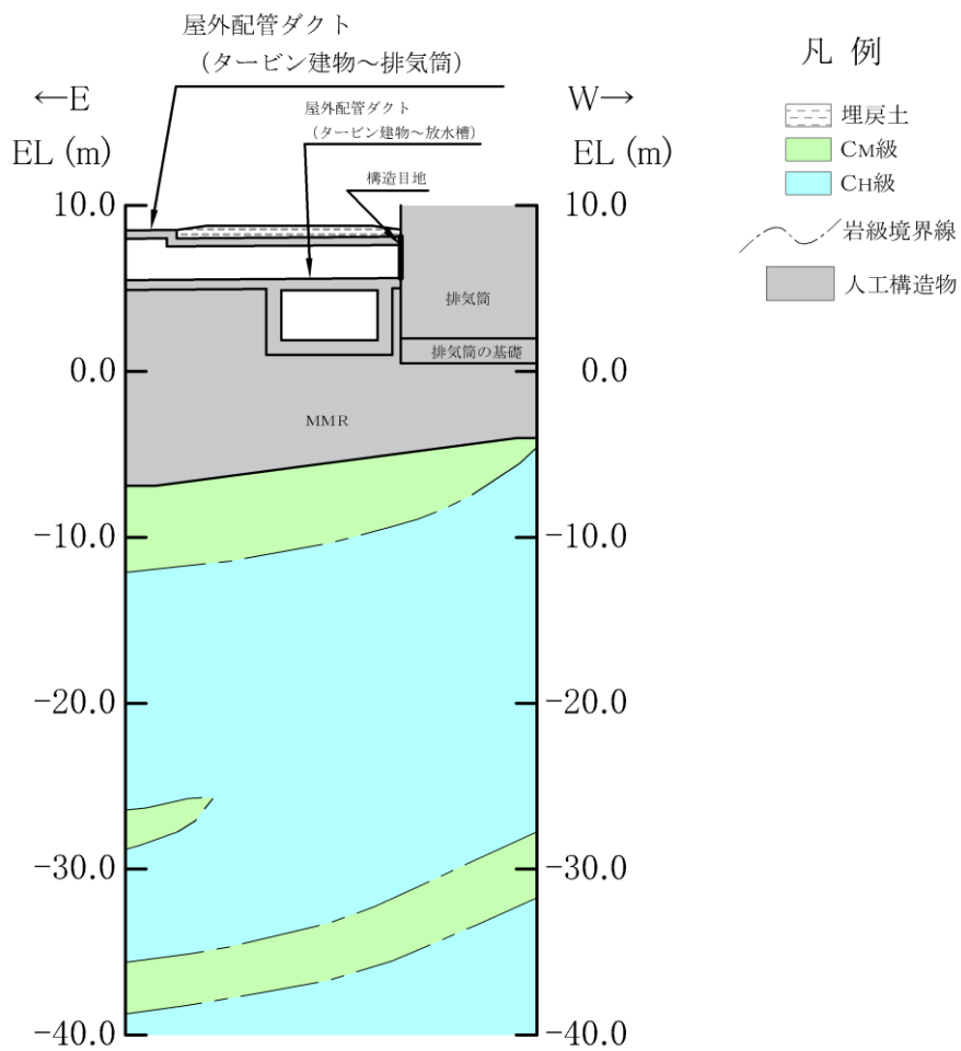
(岩級図)
