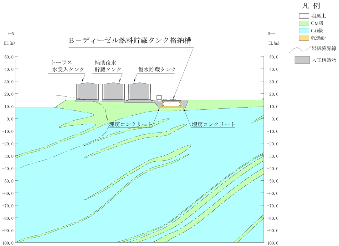
(岩級図)
