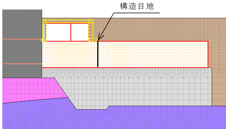
(NS方向 : B-B断面)
