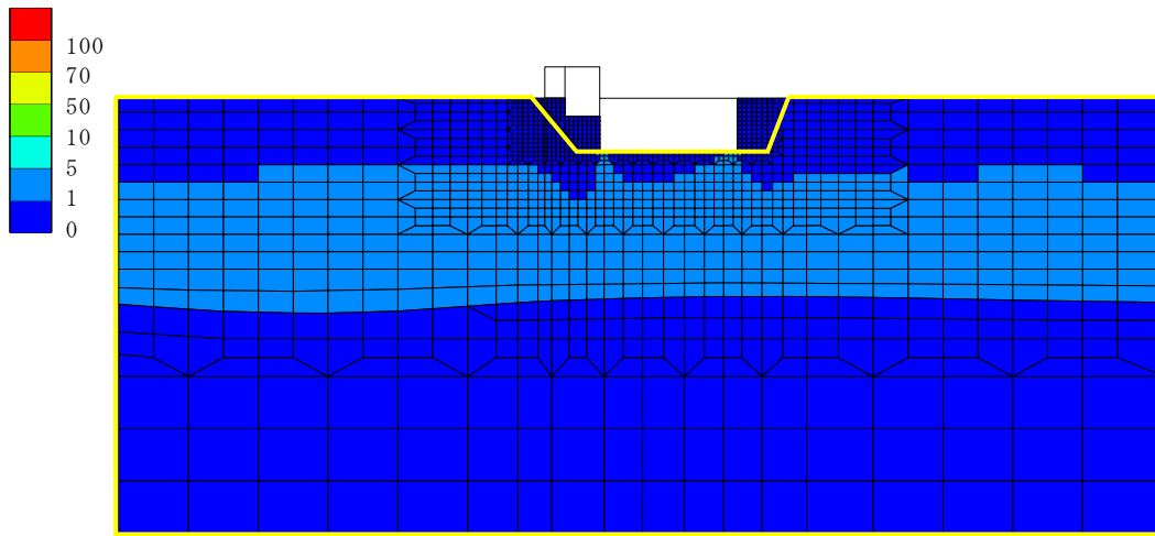
(a) 全体図
