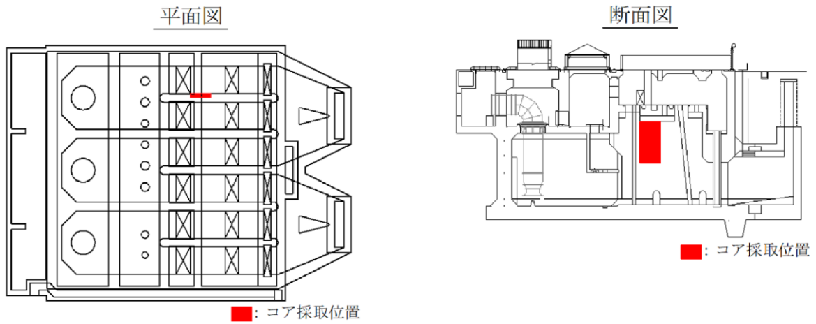
図 3-66 コア採取位置図
