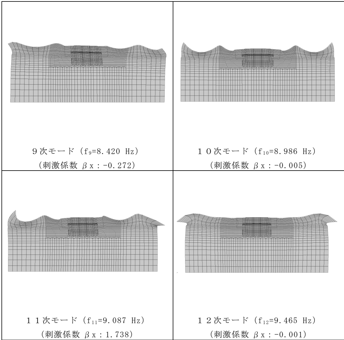
図 3-31(3) 固有値解析結果 (モード図) (B-B断面)
