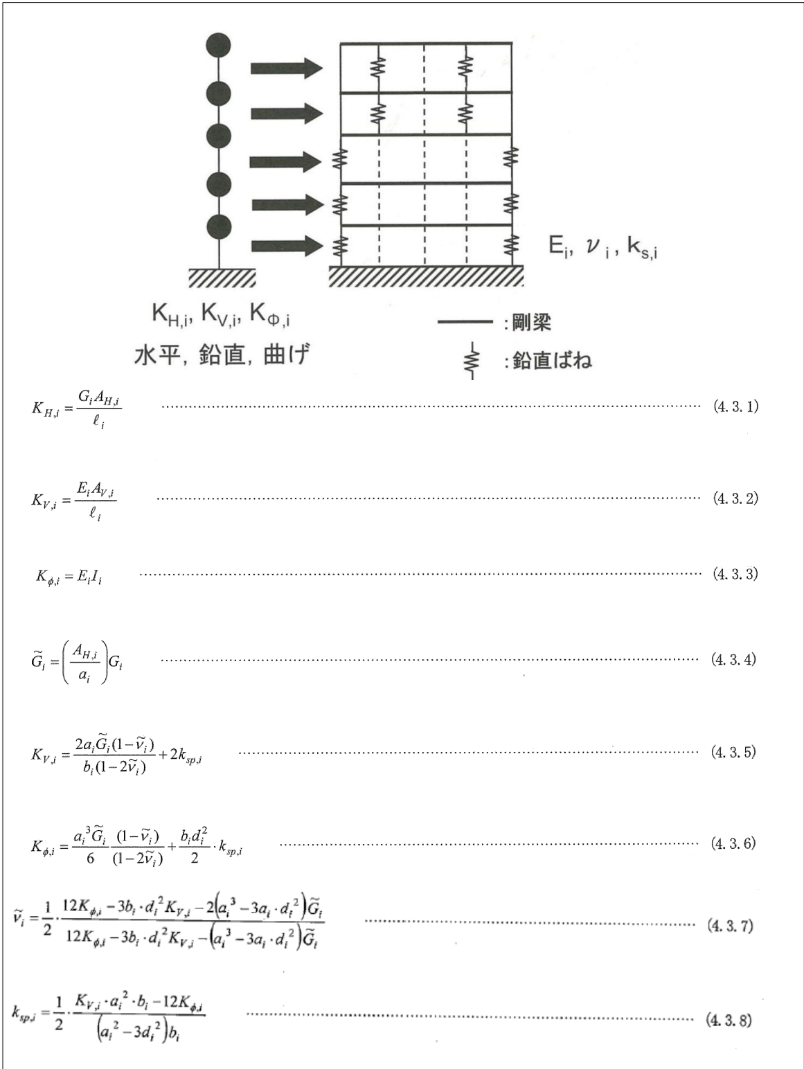
図 3-21 質点系モデルから有限要素モデルへのモデル化概要 (「原子力発電所の基礎地盤及び周辺斜面の安定性評価技術<技術資料> ((社)土木学会, 原子力土木委員会, 2009年2月)」より抜粋)
