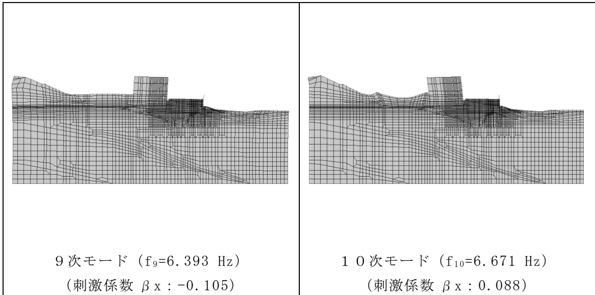
図 3-33(3) 固有値解析結果 (モード図) (D-D断面)
