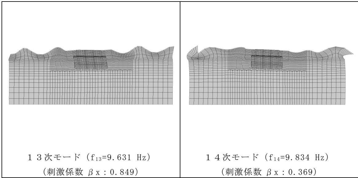
図 3-31(4) 固有値解析結果 (モード図) (B-B 断面)
