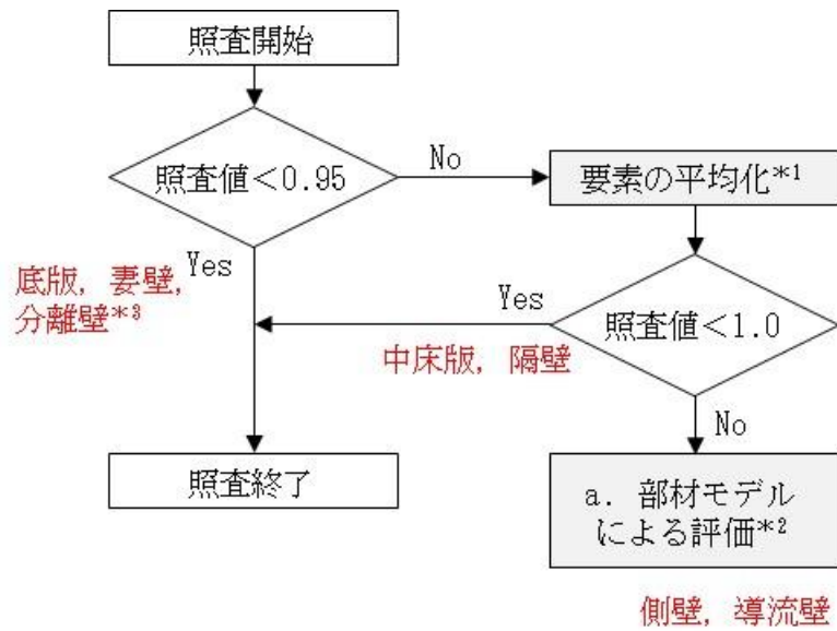
図 6-22 部材毎の最終検査方法（曲げ・軸力系の破壊に対する検査）
