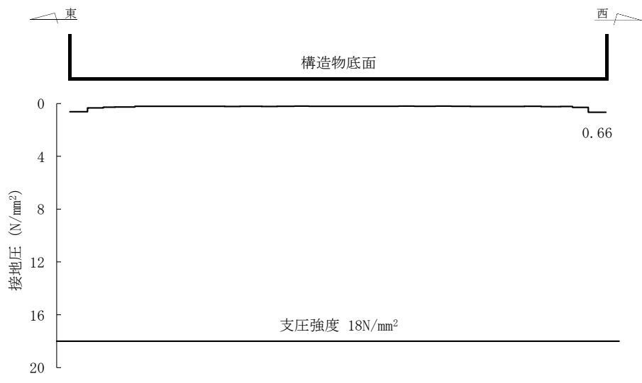
図 6-63 MMR ( f'_{ck}=18 ) (既設) の最大接地圧分布図 (解析ケース⑤, S_s - D (++) , ストレーナエリア)
