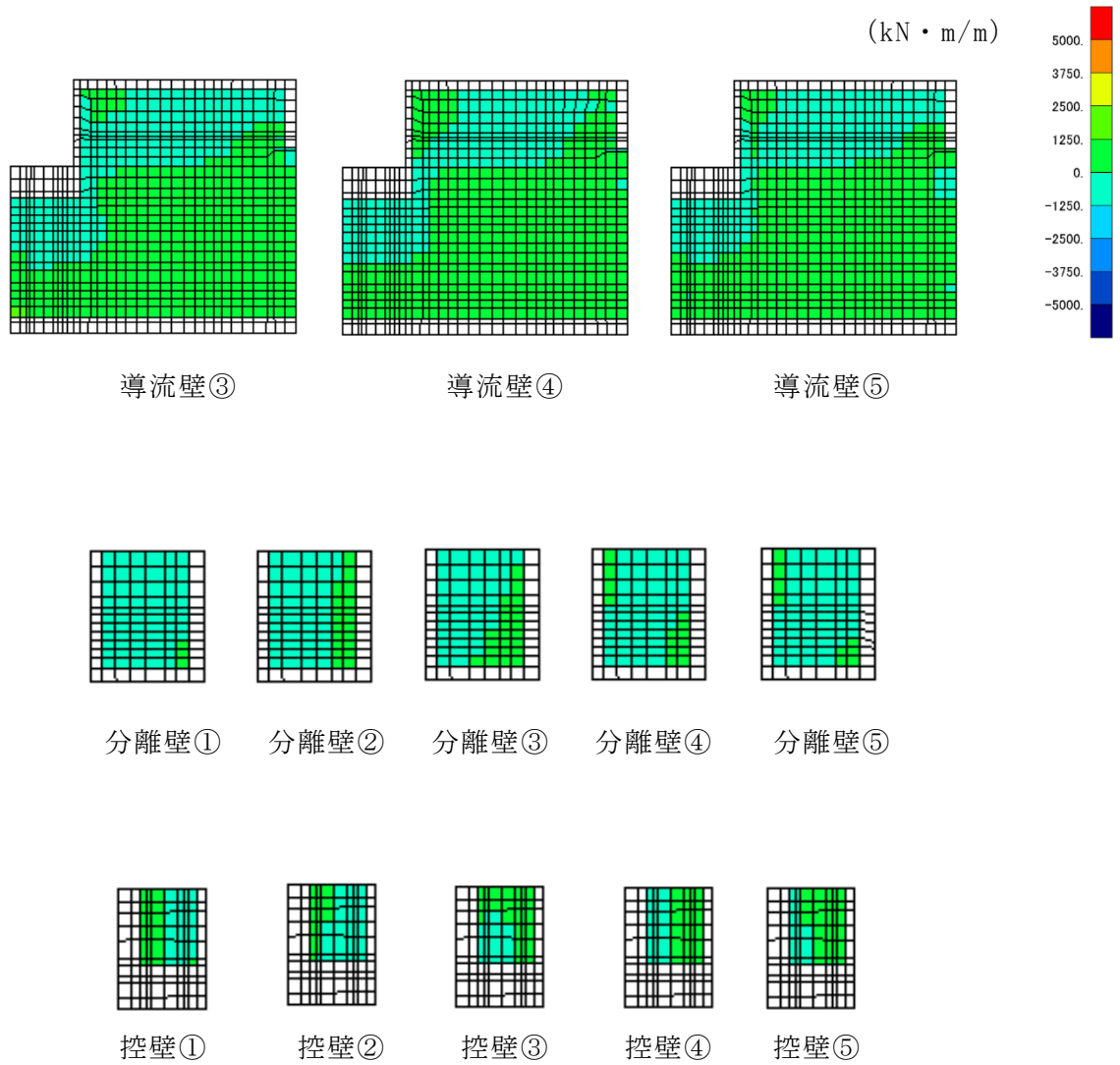
図 6-42 せん断破壊に対する照査値最大時の断面力分布図 (曲げモーメント (kN · m) : M_y ) (側壁, 解析ケース②, S_s - D (-+) )
