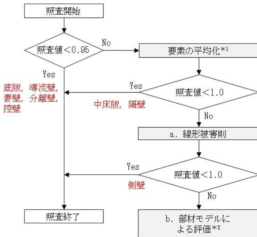
図 6-23 部材毎の最終照査方法
