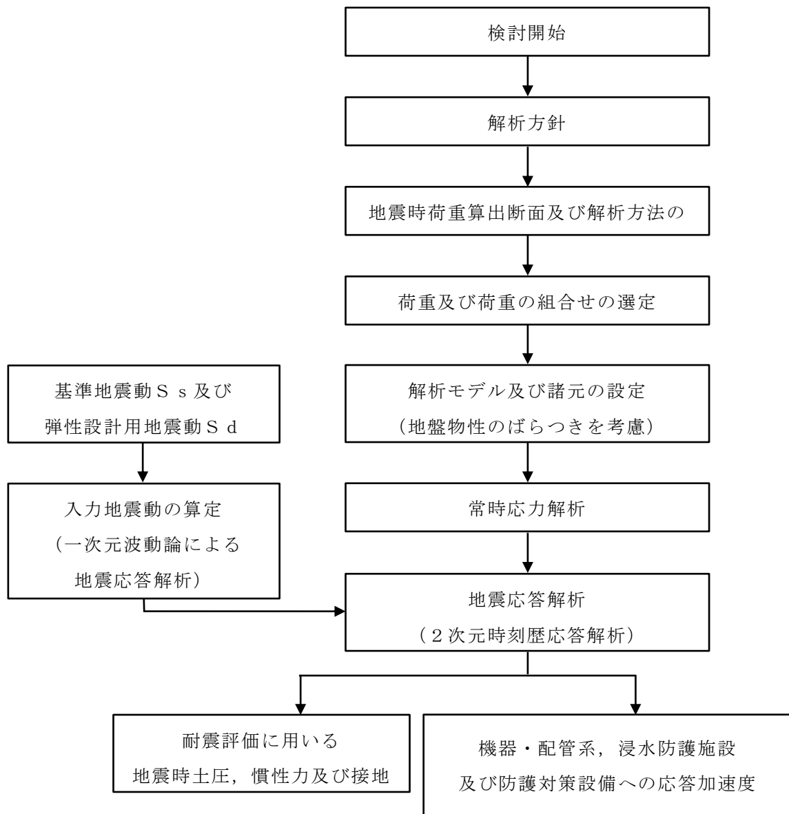
図 2-22 取水槽の地震応答解析フロー
