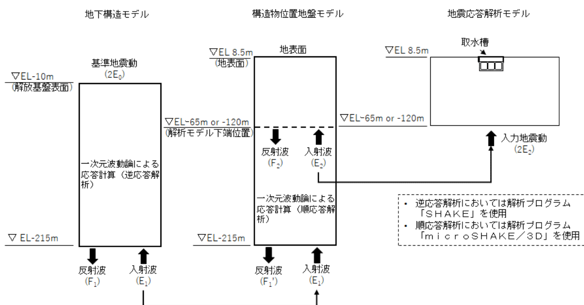
図5-1 入力地震動算定の概念図
