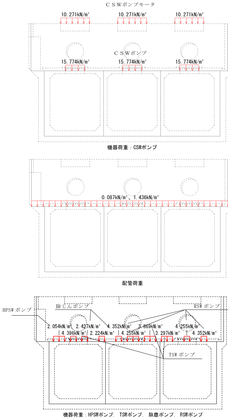
図 3-40 機器・配管の荷重図 (海水ポンプエリア)
