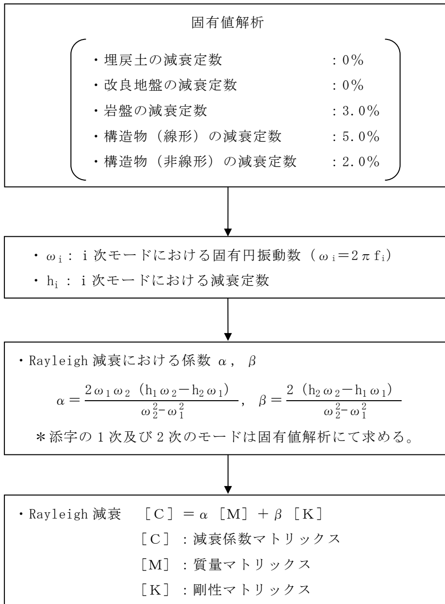
図 3-29 Rayleigh 減衰の設定フロー
