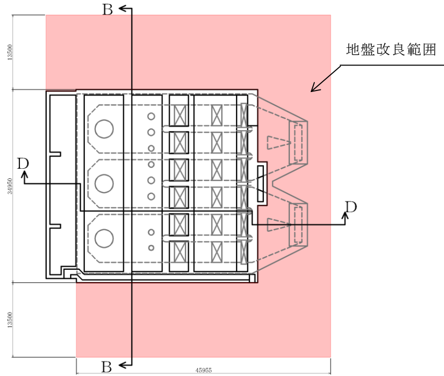
(平面図)
