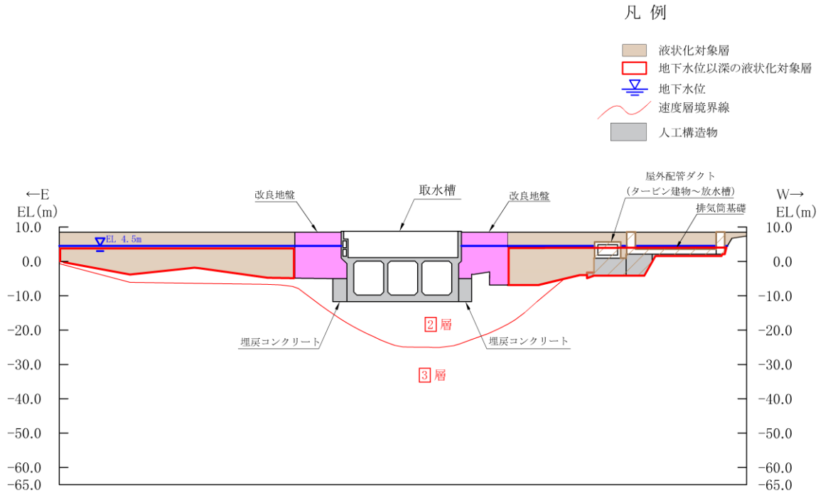
図 2-27 取水槽 地震時荷重算出断面図 (B-B 断面)
