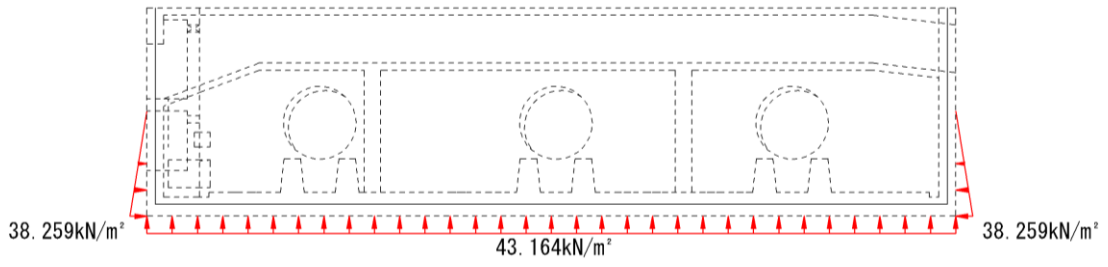
図 3-54 外水圧図 (ストレナーエリア)
