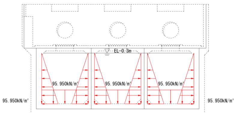
図 3-57 内水圧図（海水ポンプエリア）
