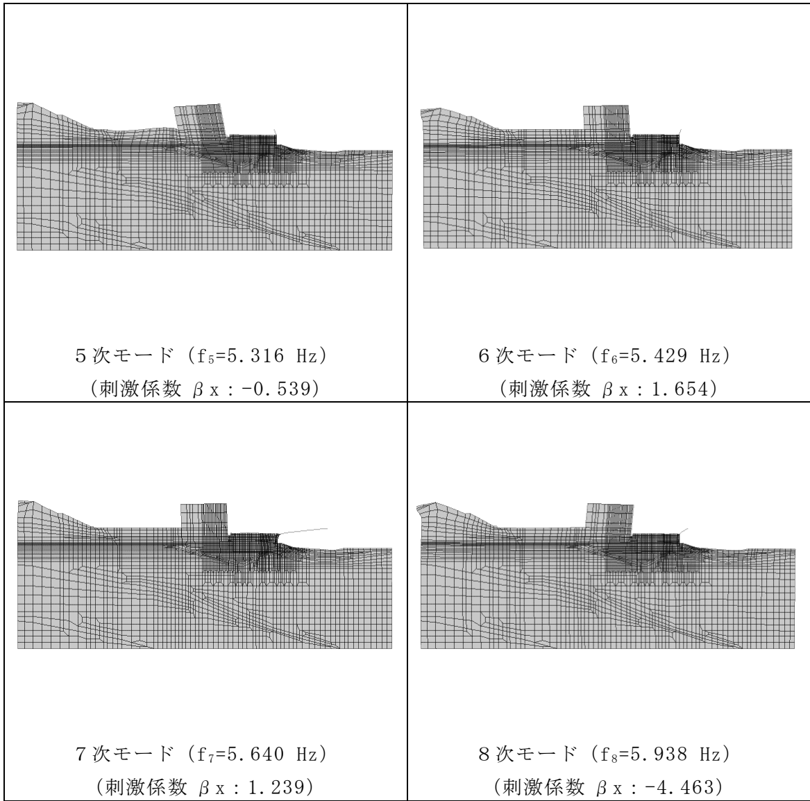
図 3-33(2) 固有値解析結果 (モード図) (D-D断面)
