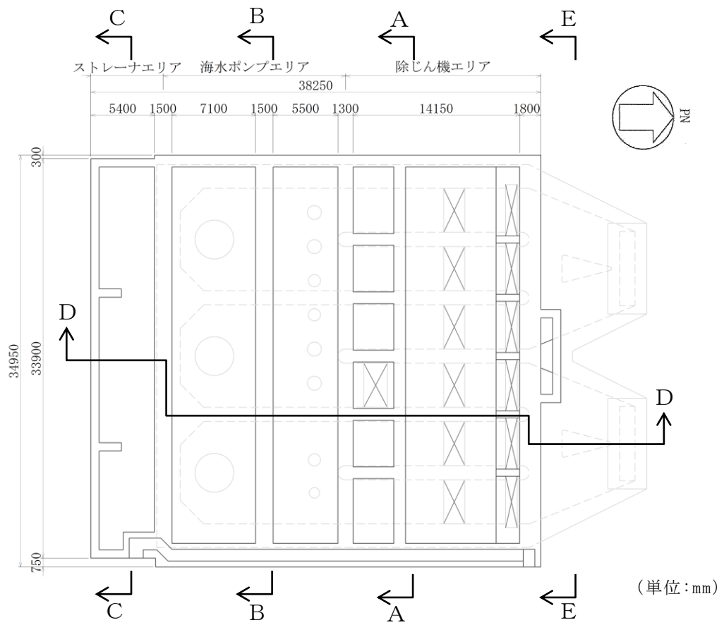
図 2-2 取水槽 平面図
