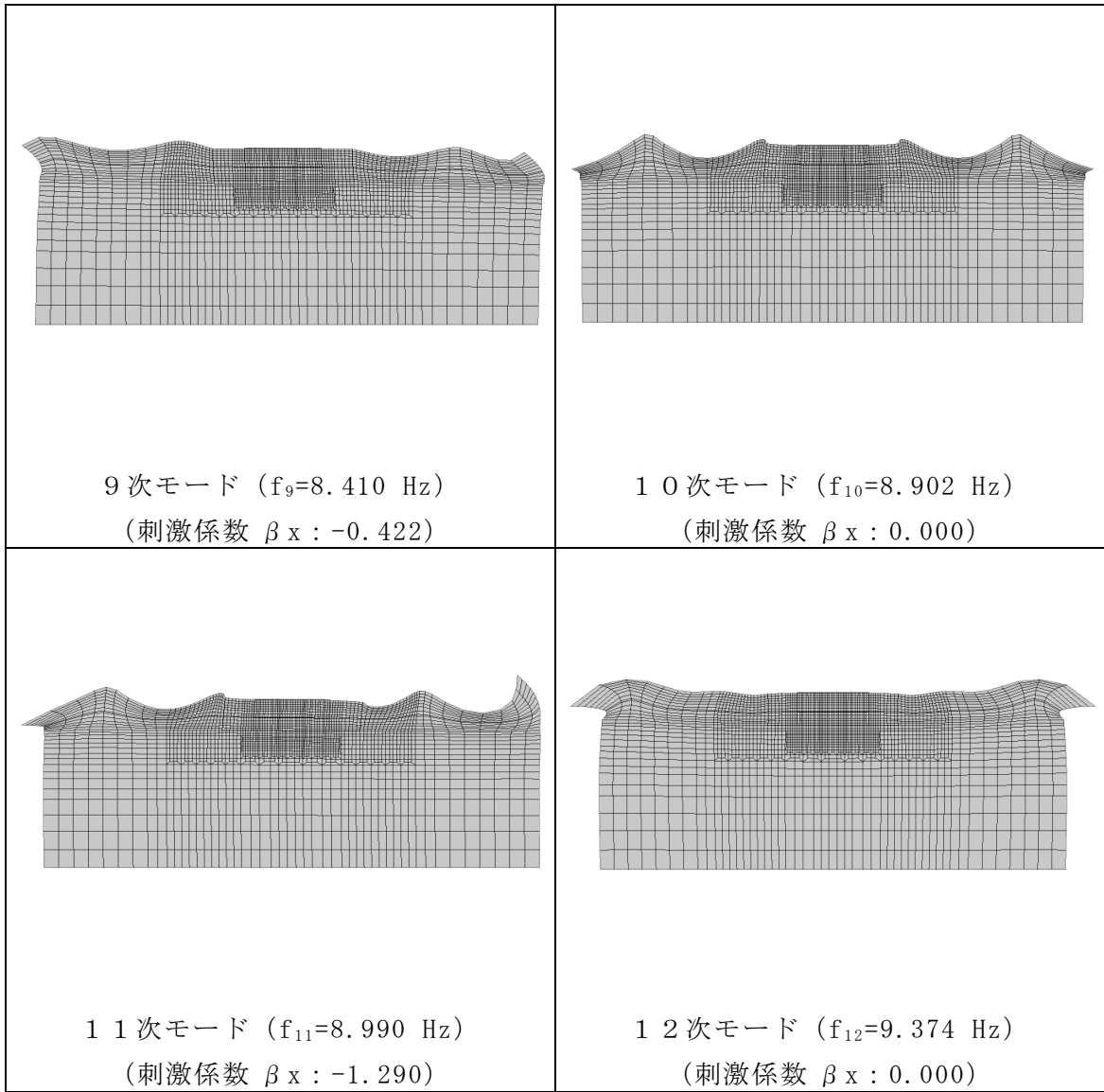
図 3-32(3) 固有値解析結果 (モード図) (C-C断面)
