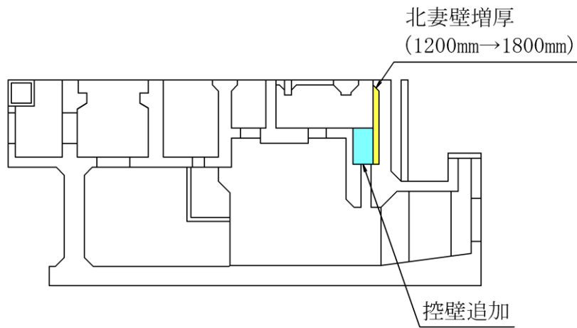
(H-H断面)
