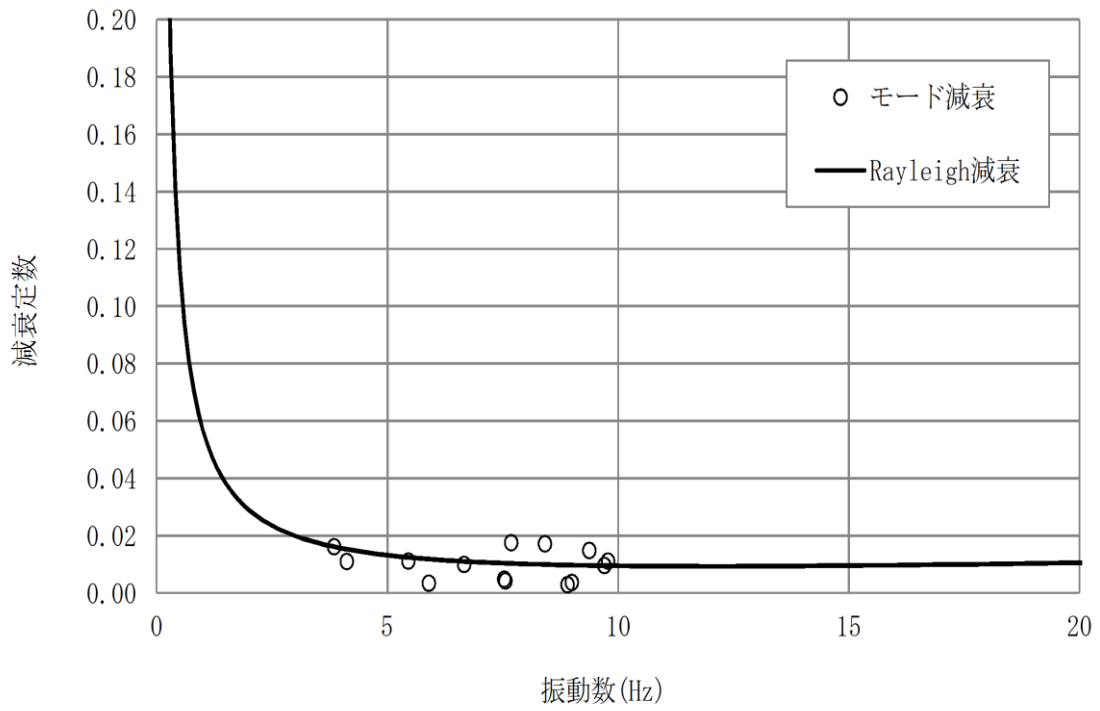
図 3-36 設定した Rayleigh 減衰 (C-C 断面)
