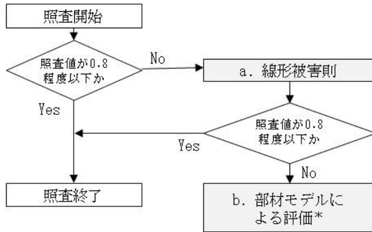
図 5-69 せん断破壊による照査フロー (PHb 設置あり)
