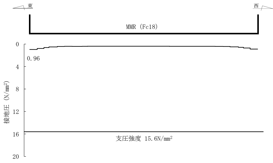
図 6-64 MMR ( f'_{ck}=15.6 ) (既設) の最大接地圧分布図 (解析ケース⑤, S_s - D (-+) , ストレーナエリア)
