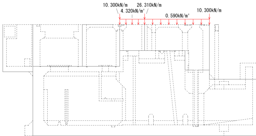
图 3-46 浸水防止設備 荷重図 (南北断面)
