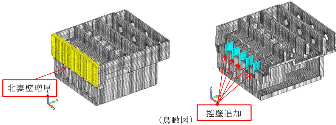
図 2-20 取水槽妻壁補強概要図
