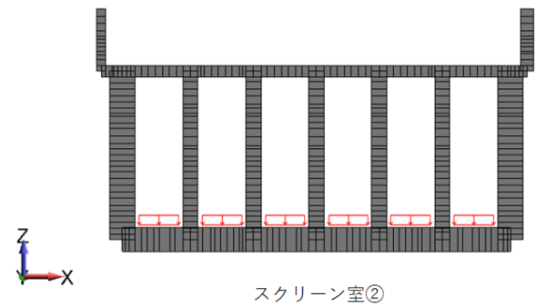
図 4-18 内水圧の概念図 (東西方向)
