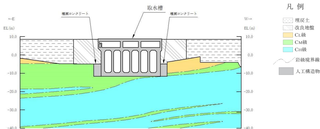
図5-62 地質断面図 (A-A断面)
