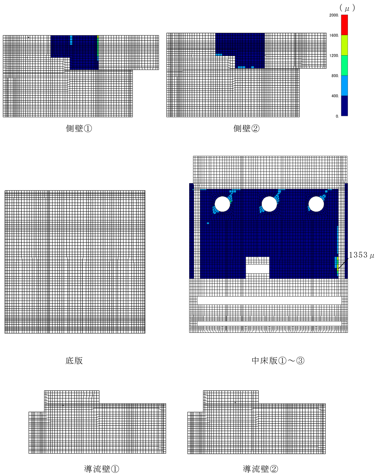
図 6-32 曲げ・軸力系の破壊に対する照査値最大時のひずみ分布図 (主筋ひずみ) (中床版, 解析ケース②, S_s - D (-+) )
