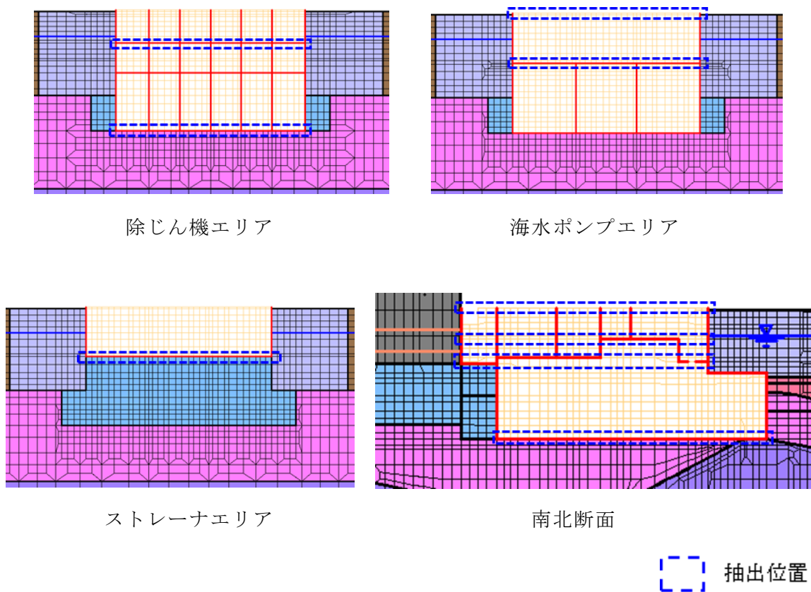
図4-23 応答加速度の抽出位置
