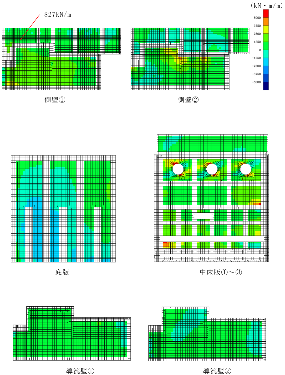
図 6-44 せん断破壊に対する照査値最大時の断面力分布図
