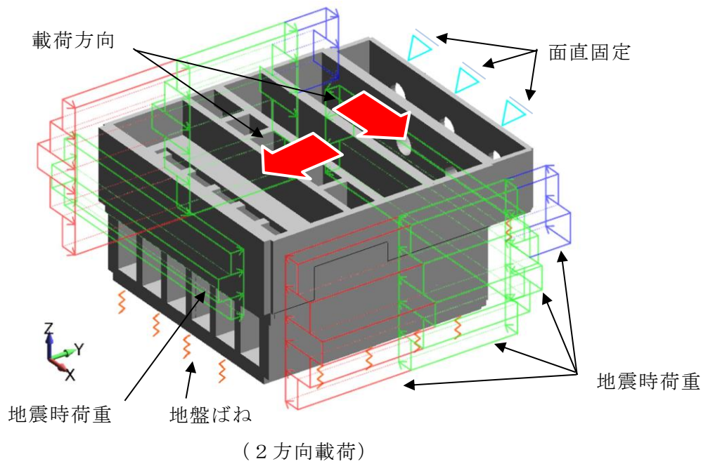
図 4-7 地盤ばね設定のイメージ図
