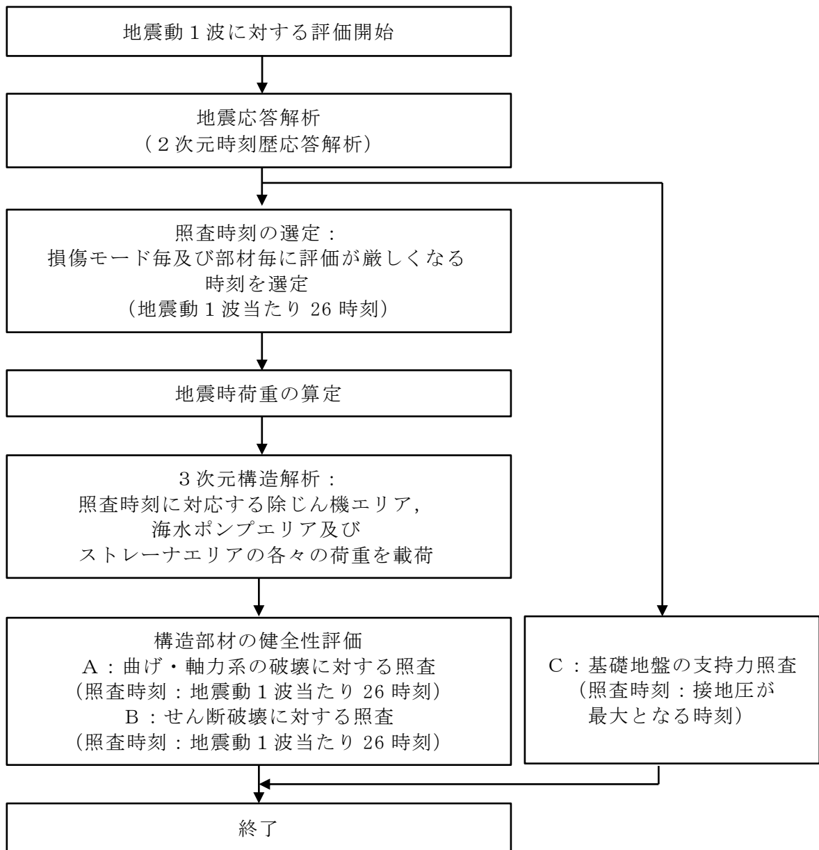
図 2-24 基本フロー (地震動 1 波に対する評価フロー)
