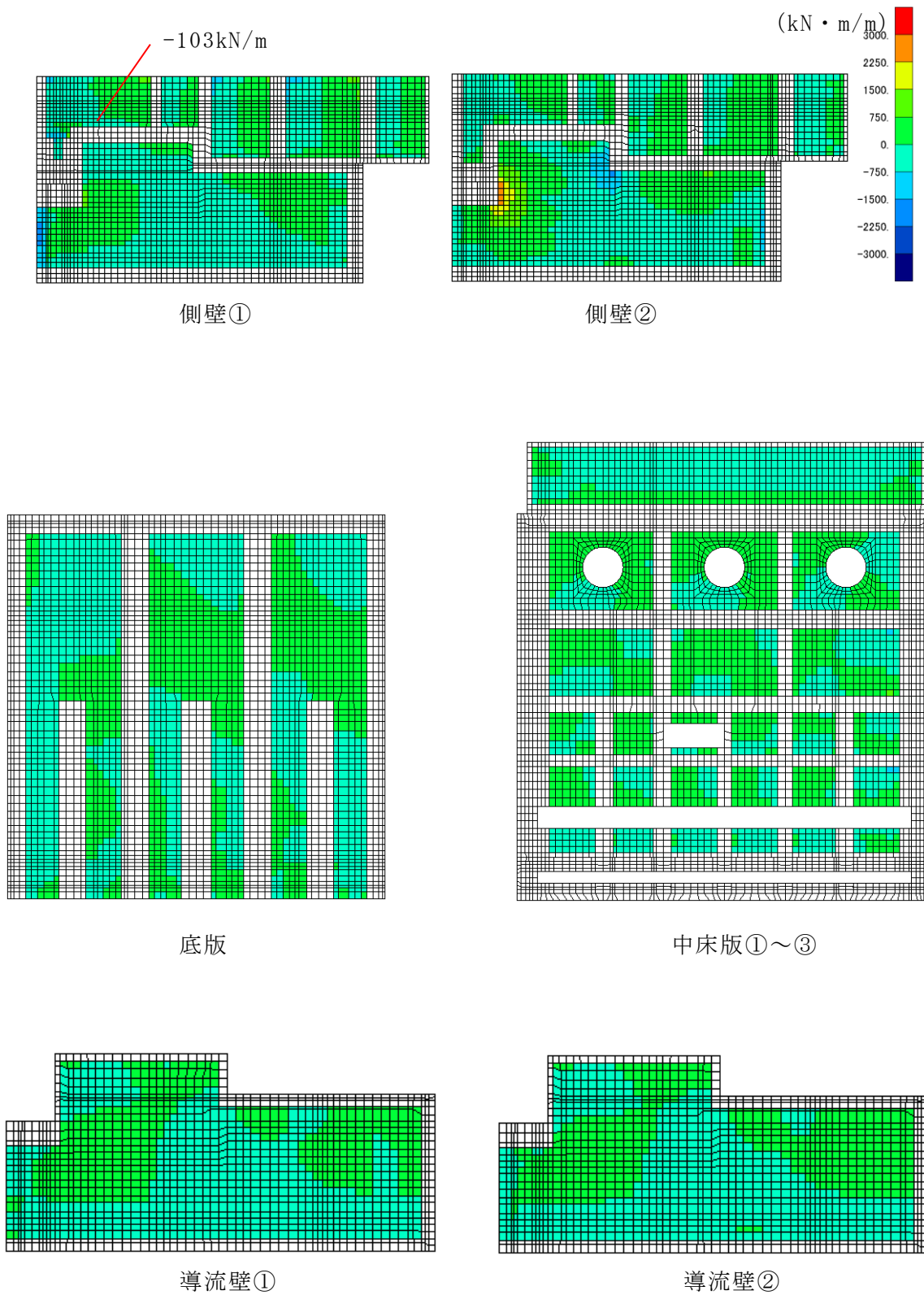
図 6-53 せん断破壊に対する照査値最大時の断面力分布図
