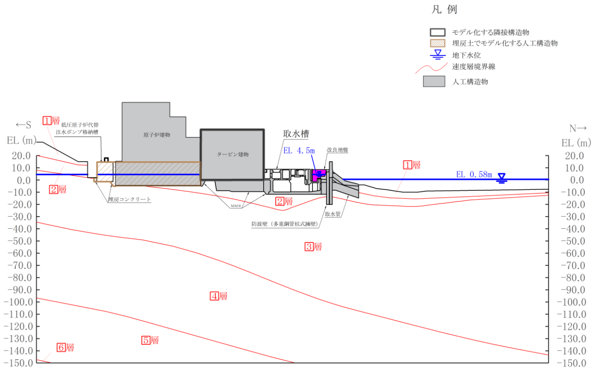
(a) 地震時荷重算出地質断面図
