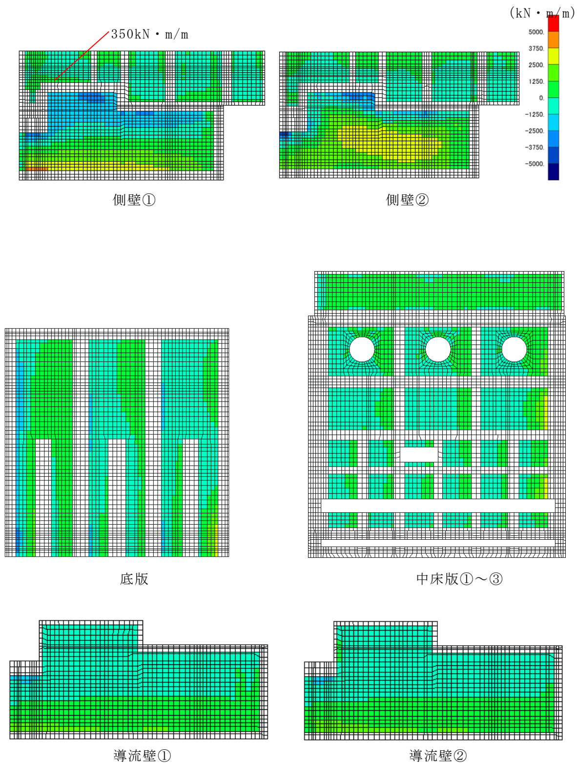
図 6-38 せん断破壊に対する照査値最大時の断面力分布図 (曲げモーメント (kN・m) : M_x ) (側壁, 解析ケース②, S_s - D (-+) )
