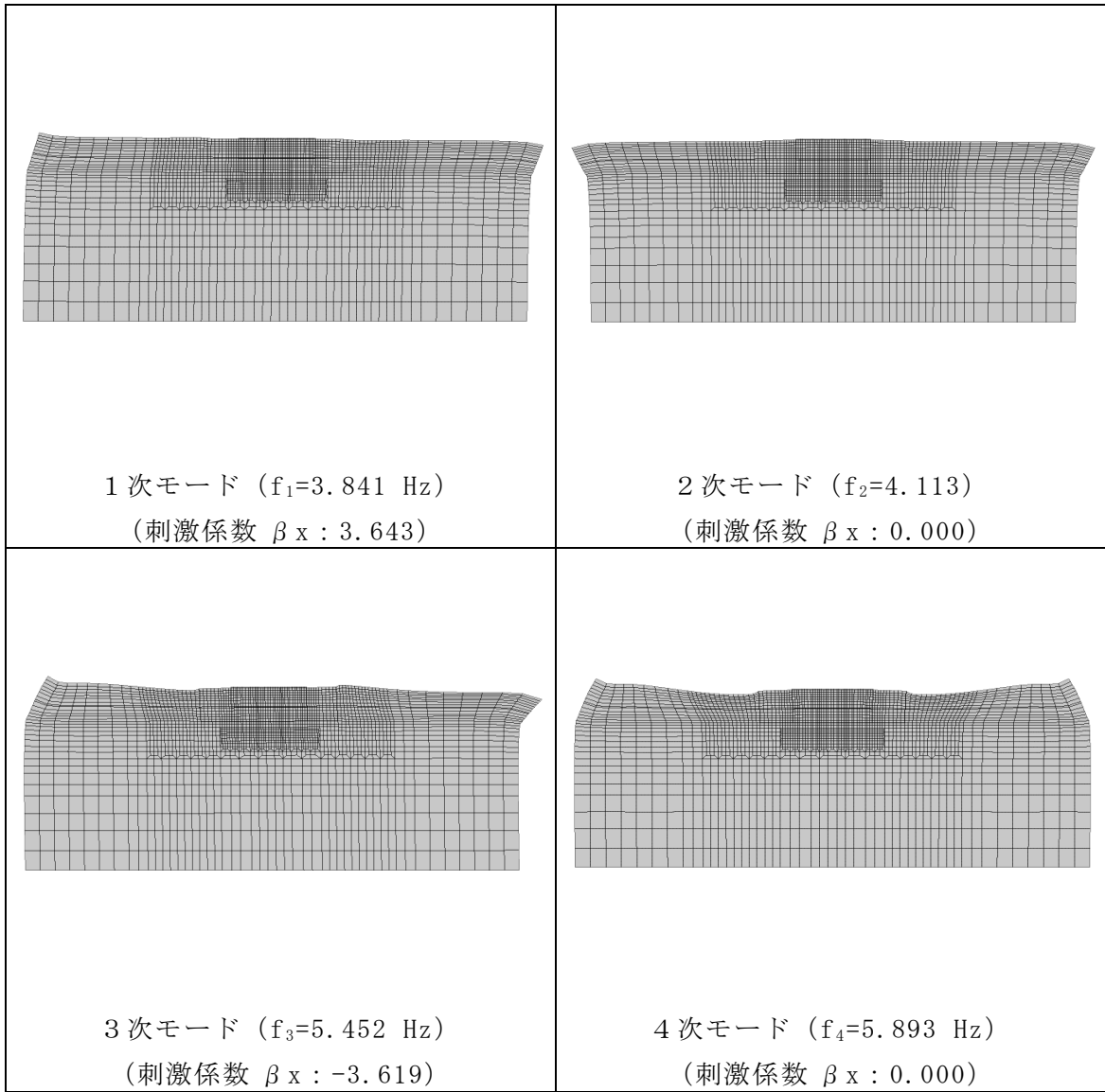
図 3-32(1) 固有値解析結果 (モード図) (C-C断面)
