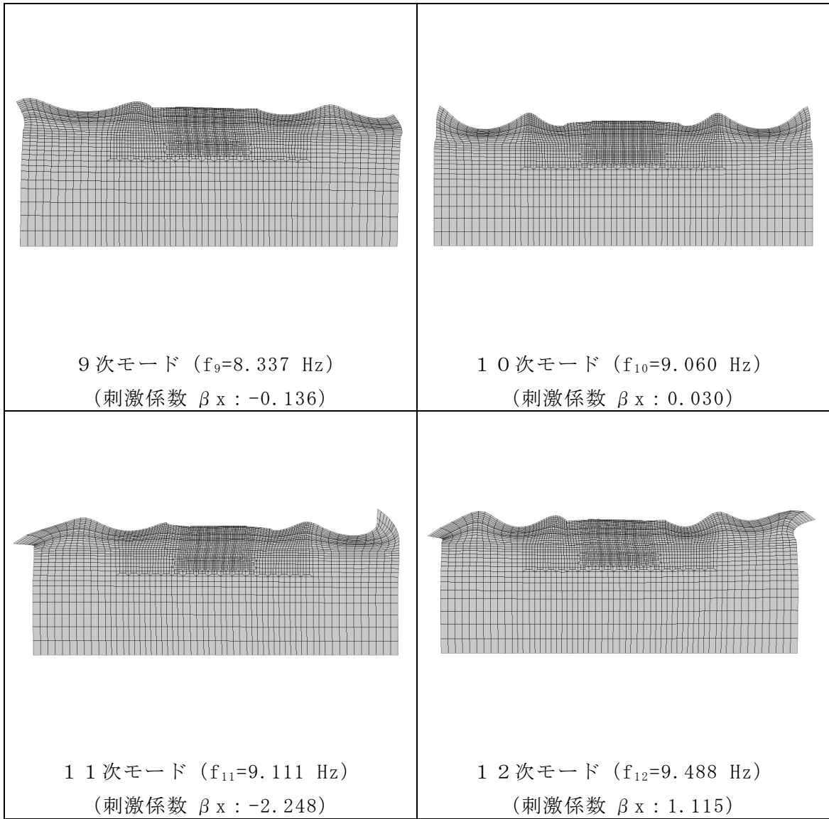
図 3-30(3) 固有値解析結果 (モード図) (A-A断面)
