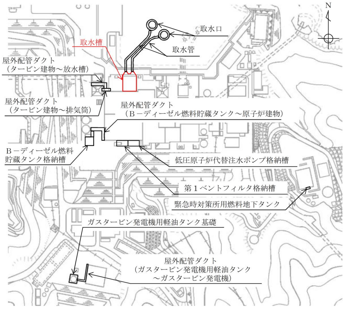
図 2-1 取水槽 位置図
