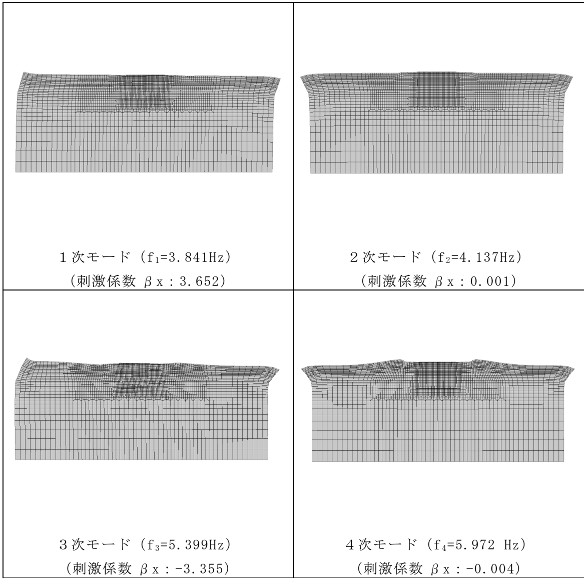
図 3-30(1) 固有値解析結果 (モード図) (A-A 断面)
