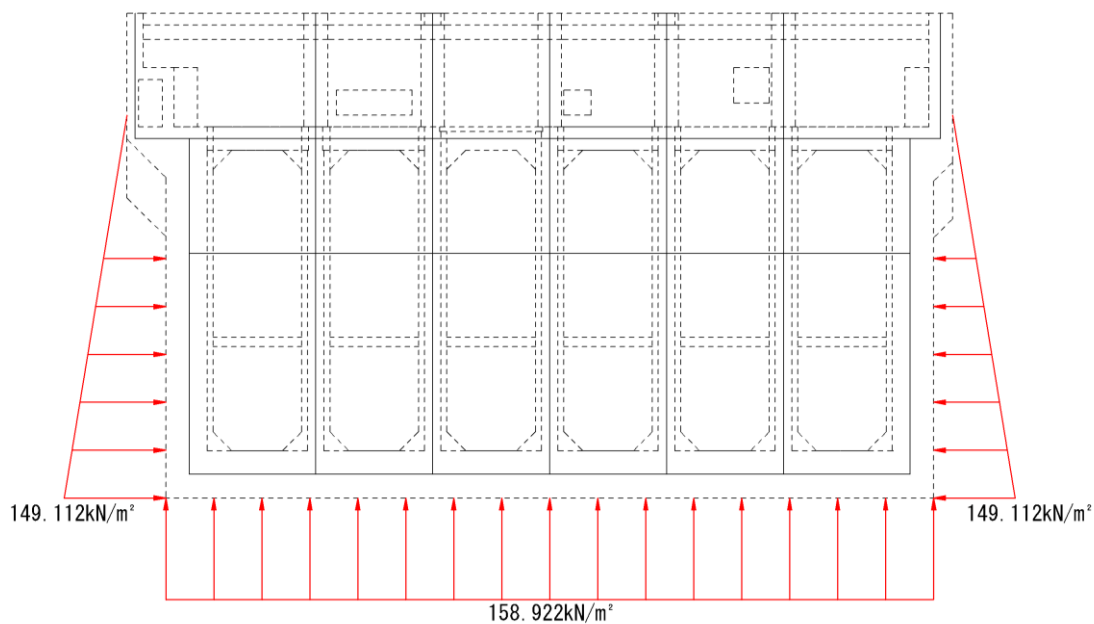
図3-52 外水圧図（除じん機エリア）
