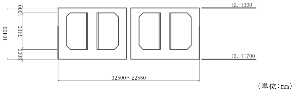
図 2-7 取水槽 断面図 (E-E 断面)
