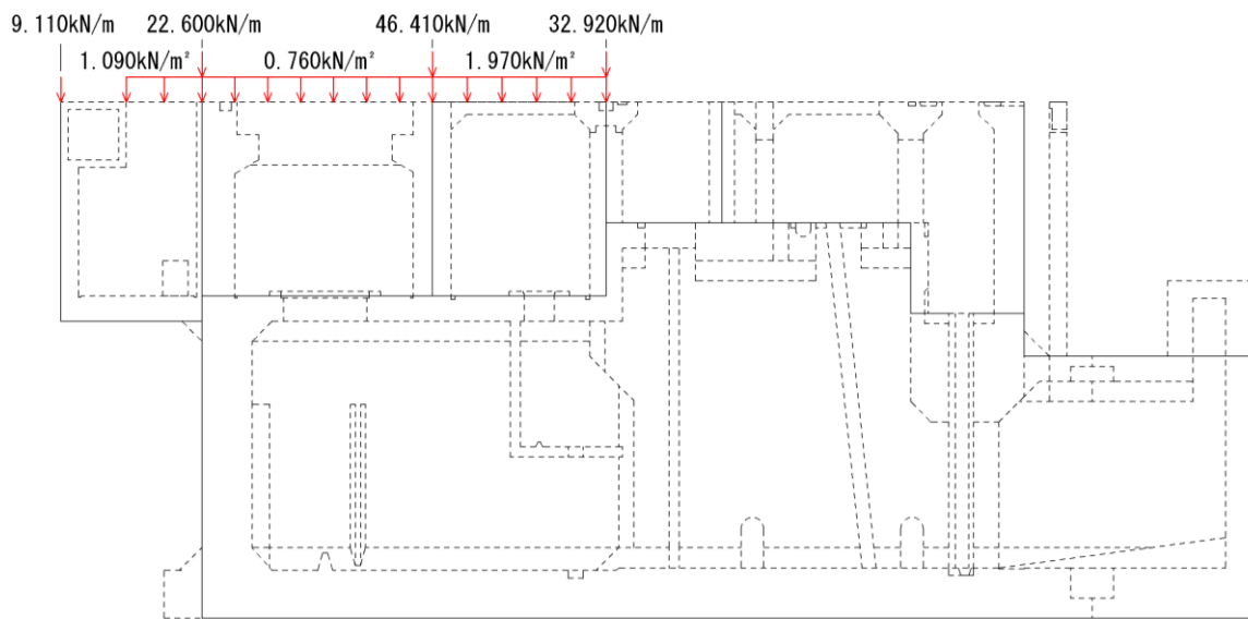
図 3-51 竜巻防護対策設備 荷重図 (南北断面)
