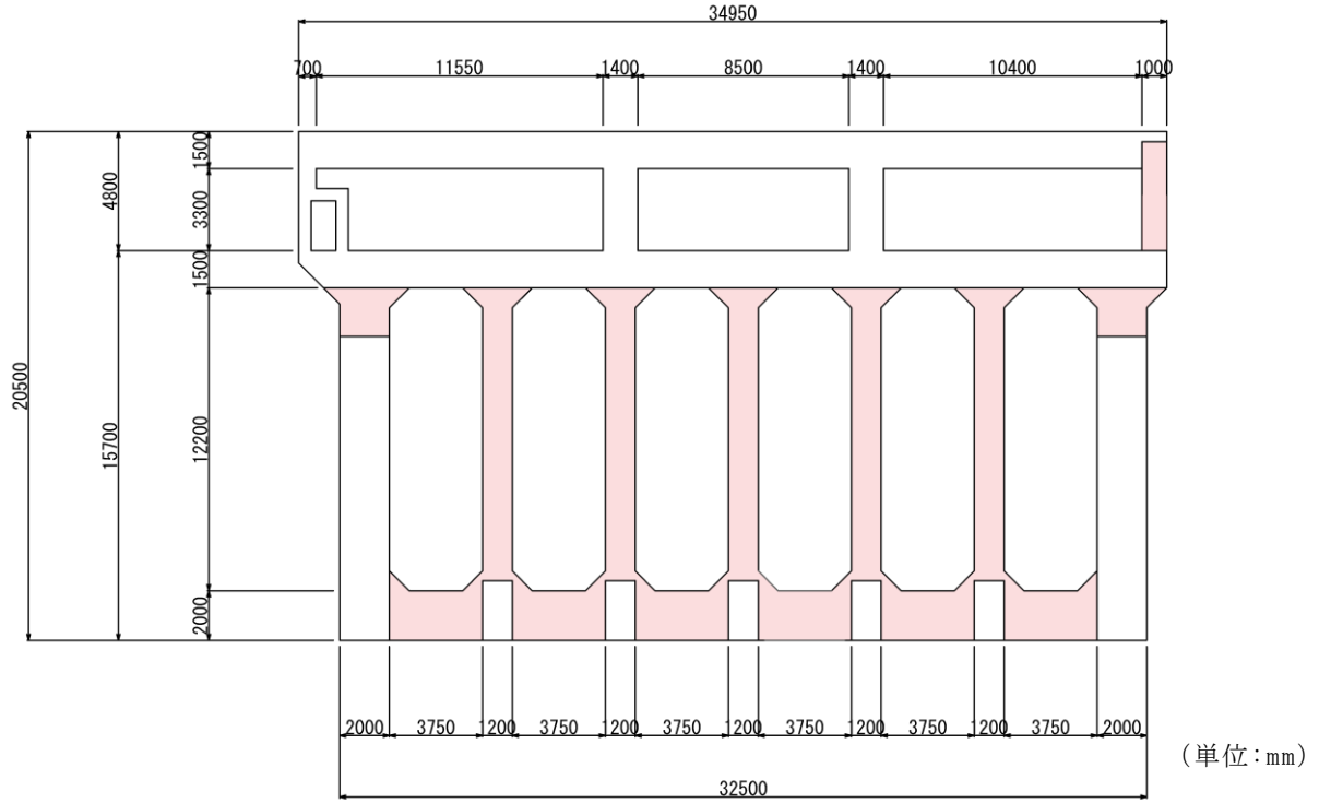
図 2-14 補強計画図 (断面図 (A-A 断面))
