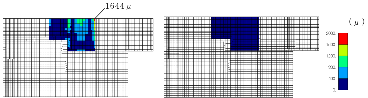
側壁①
