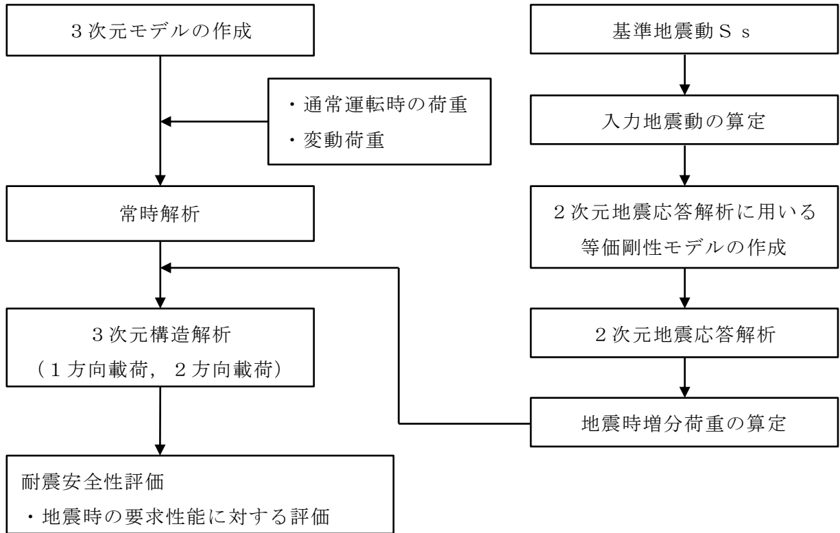
図 4-16 地震時増分荷重を 3 次元構造解析モデルへ載荷するまでのフロー
