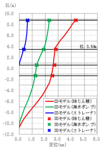
図 3-19 剛性調整結果
