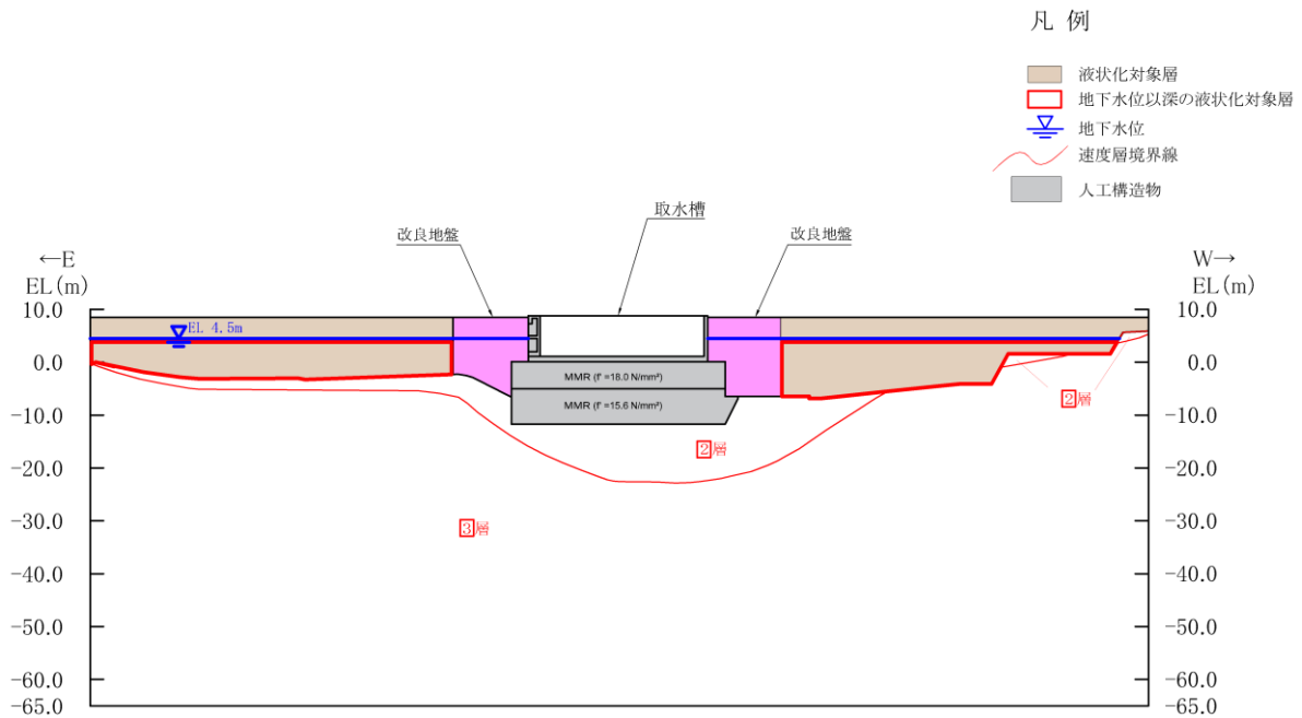
図 3-23 取水槽の周辺地盤（ストレーナエリア（C-C断面））
