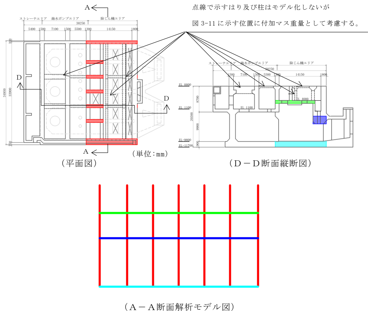
図 3-10 線形はり要素でモデル化する部材 (除じん機エリア (A-A 断面))
