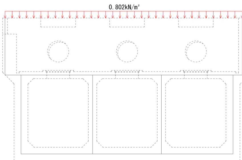
図3-60 積雪荷重図（海水ポンプエリア）
