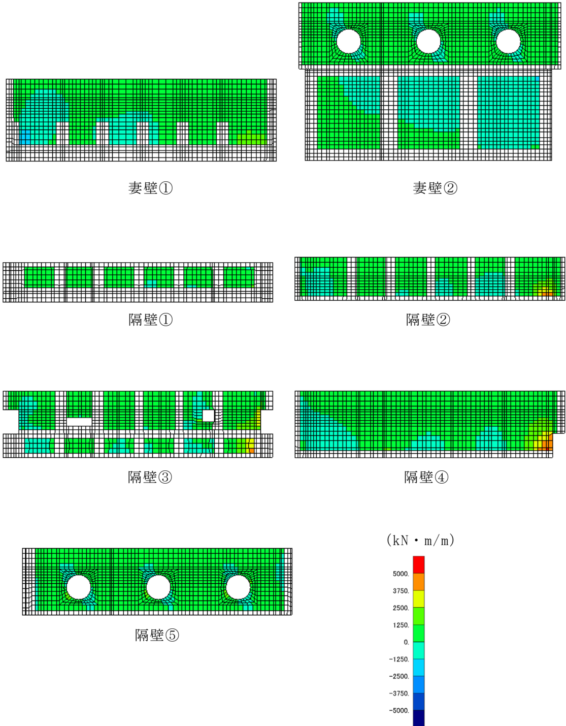
図 6-49 せん断破壊に対する照査値最大時の断面力分布図
