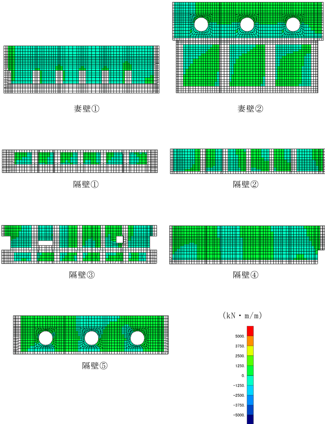
図 6-40 せん断破壊に対する照査値最大時の断面力分布図 (曲げモーメント ( \text{kN} \cdot \text{m} ) : M_x ) (側壁, 解析ケース②, S_s - D (-+) )
