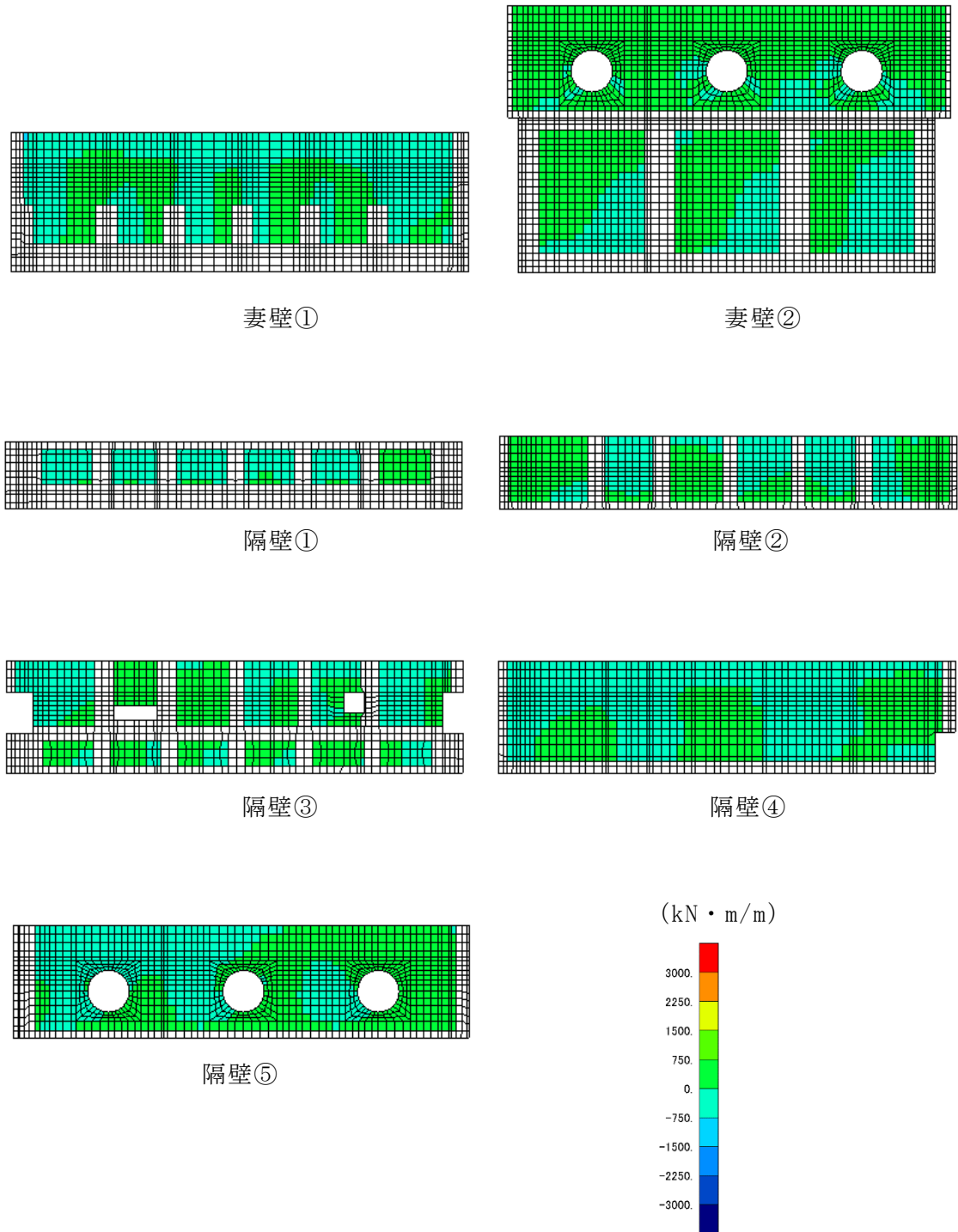
図 6-52 せん断破壊に対する照査値最大時の断面力分布図
