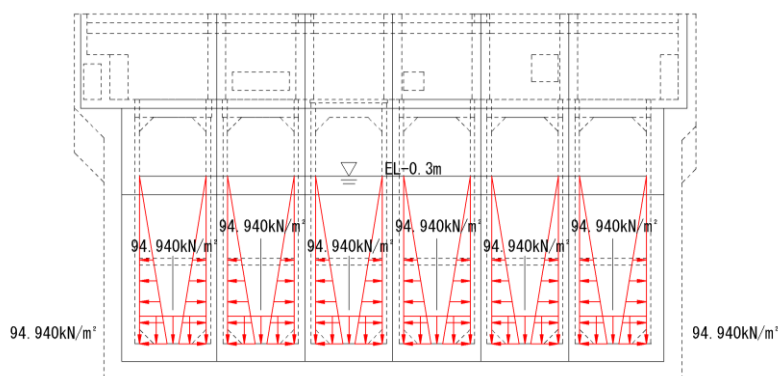
図 3-56 内水圧図（除じん機エリア）
