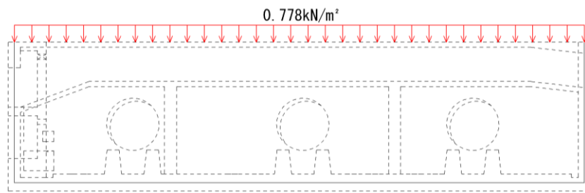
図 3-61 積雪荷重図 (ストレナーナエリア)
