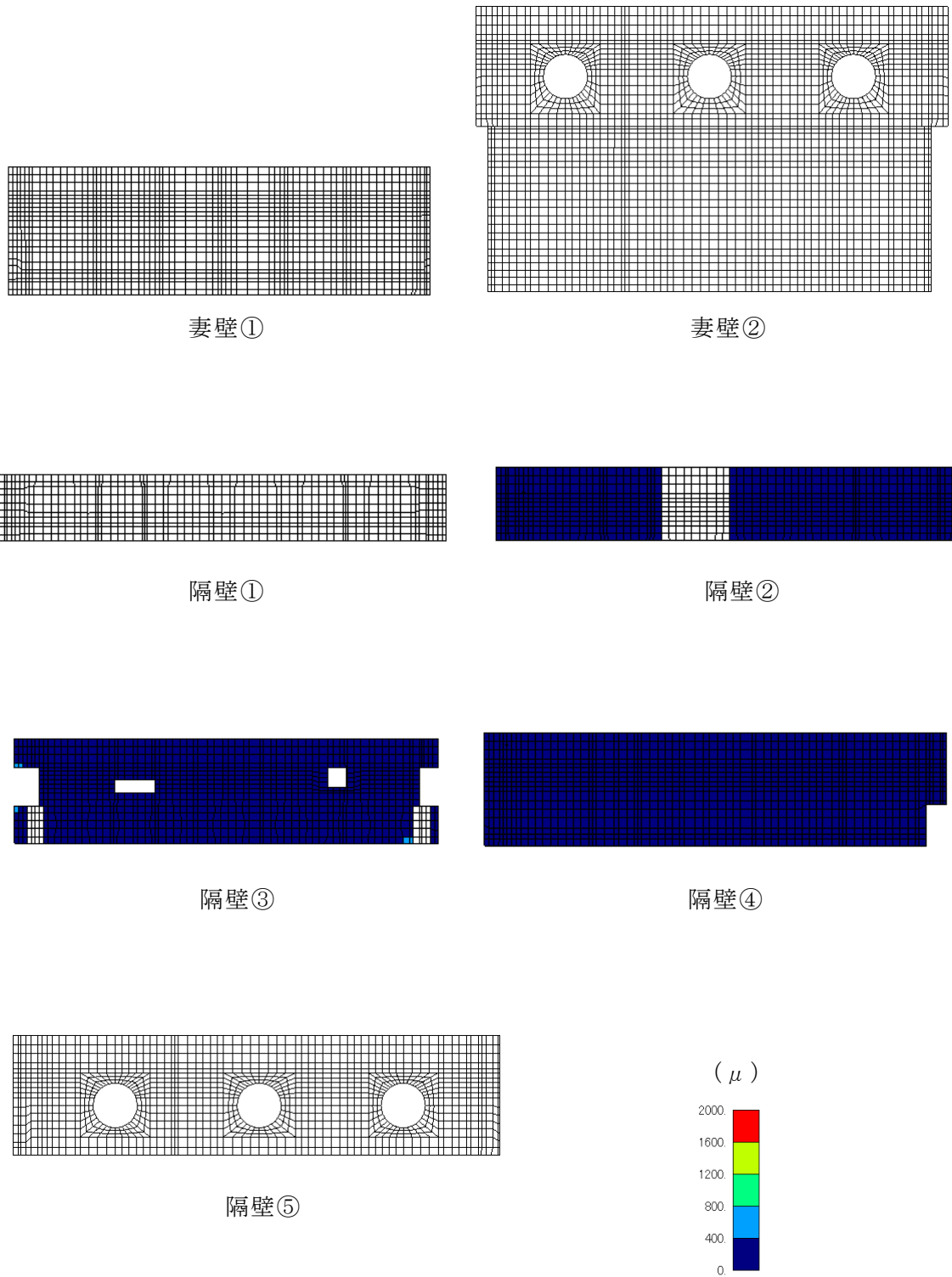
図 6-31 曲げ・軸力系の破壊に対する照査値最大時のひずみ分布図 (コンクリートの圧縮ひずみ) (側壁, 解析ケース④, S_s - D (-+) )
