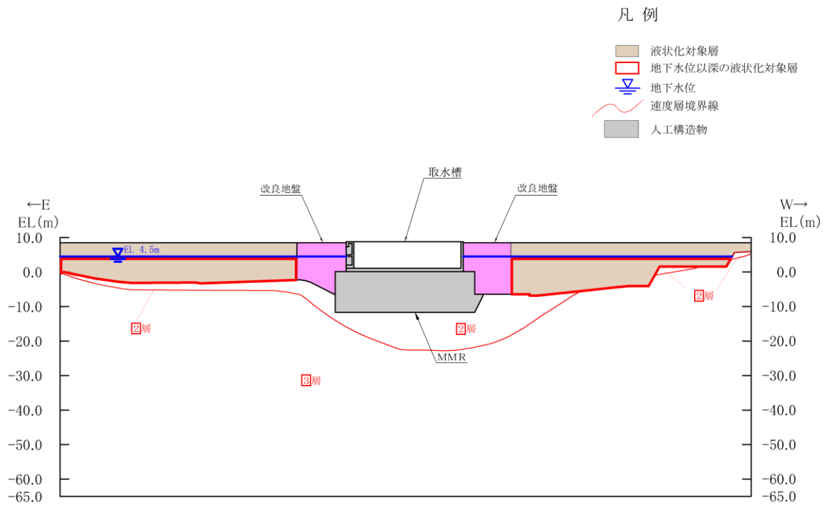
図 2-28 取水槽 地震時荷重算出断面図 (C-C 断面)
