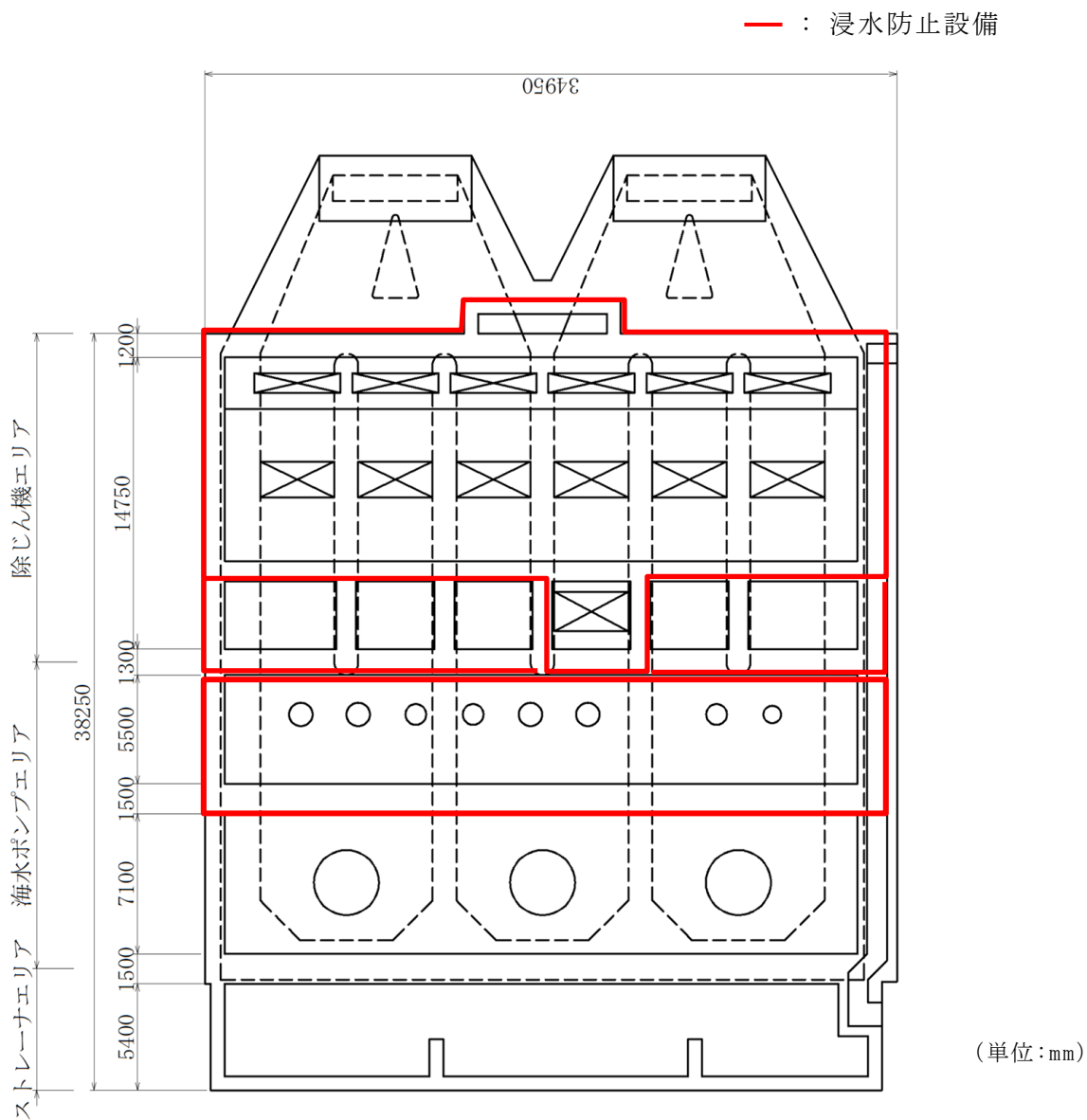
図 3-43 浸水防止設備 位置図
