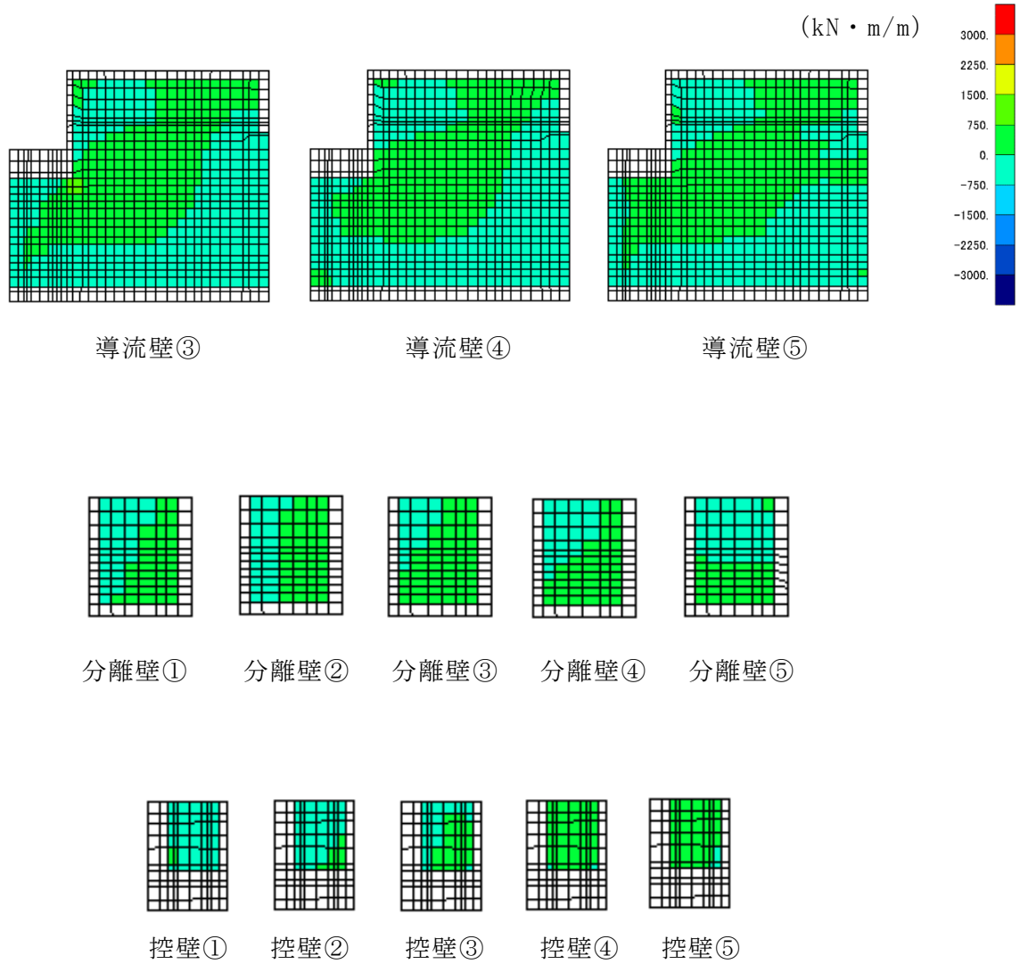
図 6-54 せん断破壊に対する照査値最大時の断面力分布図 (せん断力 (kN/m) : Q_y ) (側壁, 解析ケース②, S_s - D (-+) )
