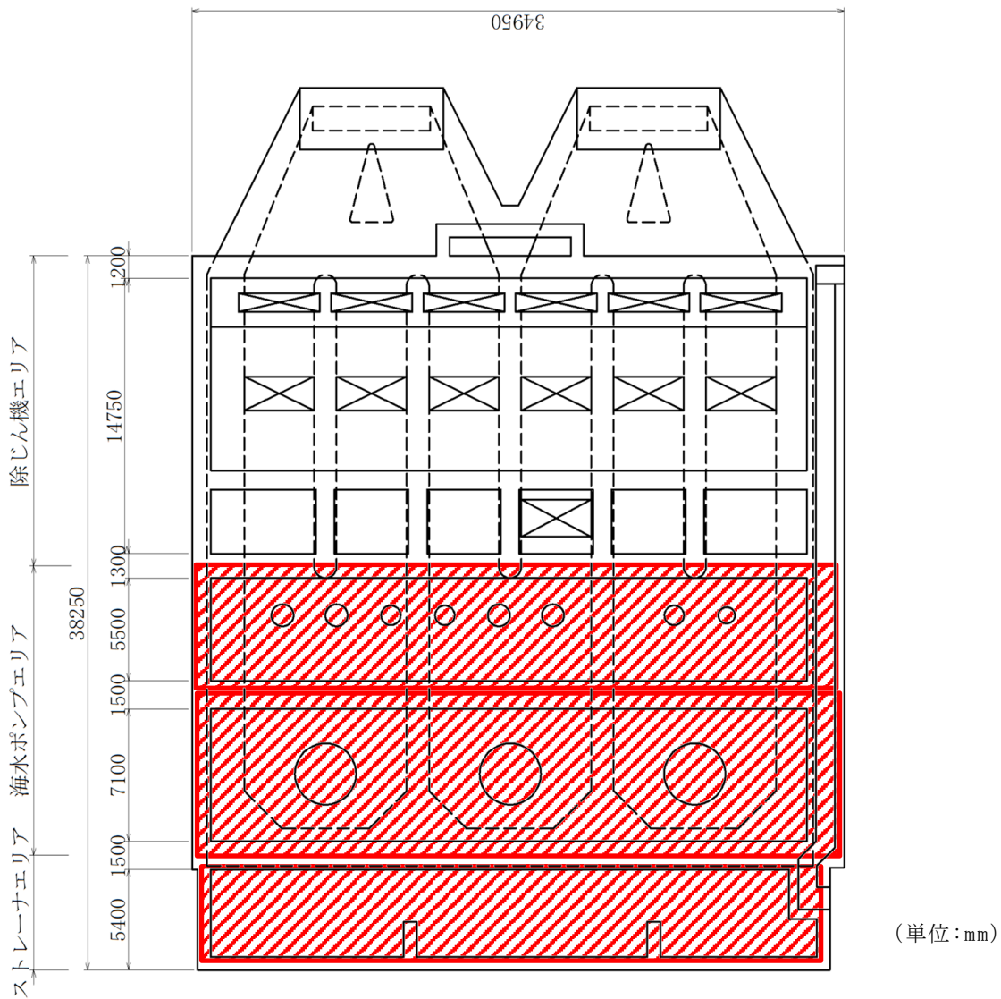
図3-47 竜巻防護対策設備 位置図
