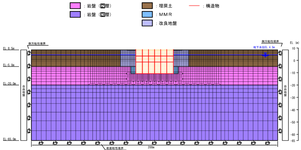
(b) 地震応答解析モデル図
