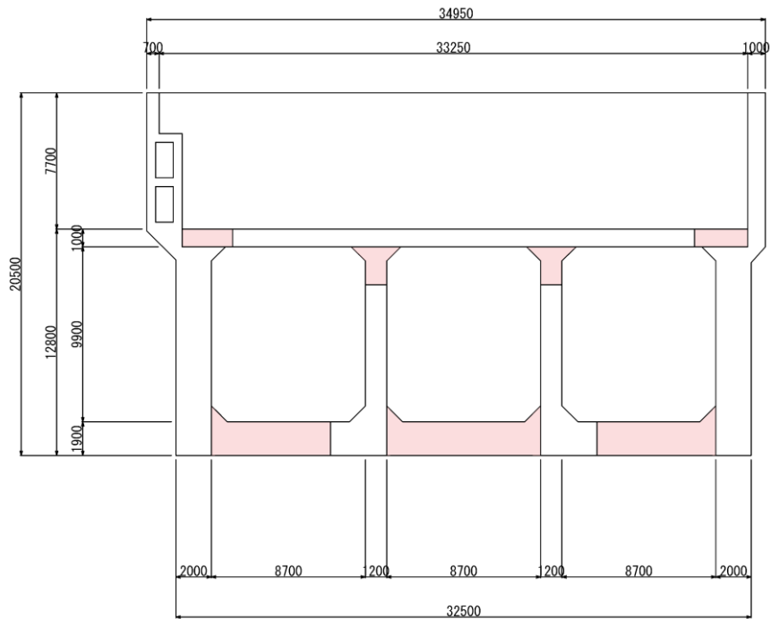
図 5-55 PHb による耐震補強箇所 (断面図 (B-B 断面)) (再掲)
