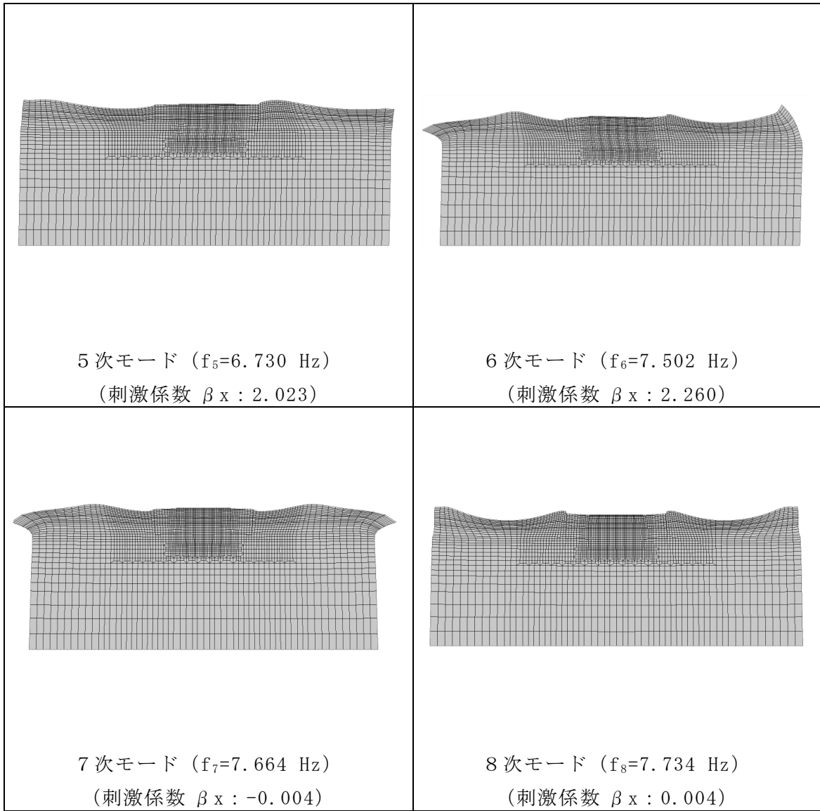
図 3-30(2) 固有値解析結果 (モード図) (A-A断面)
