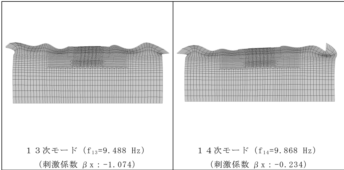
図 3-30(4) 固有値解析結果 (モード図) (A-A断面)
