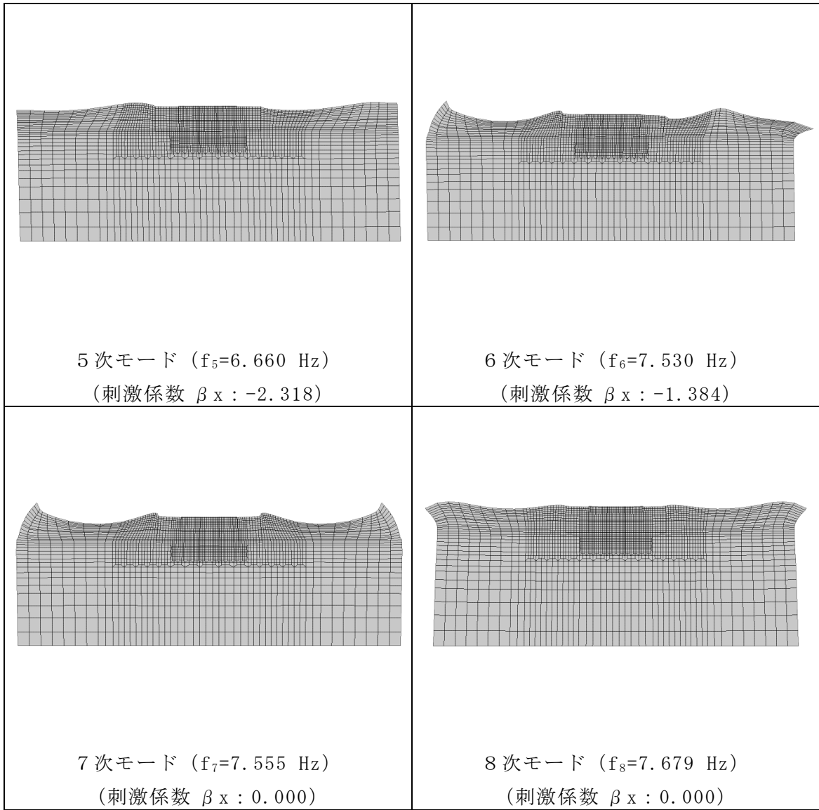
図 3-32(2) 固有値解析結果 (モード図) (C-C断面)
