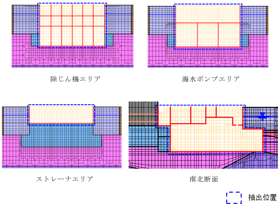
図4-22 応答加速度の抽出位置
