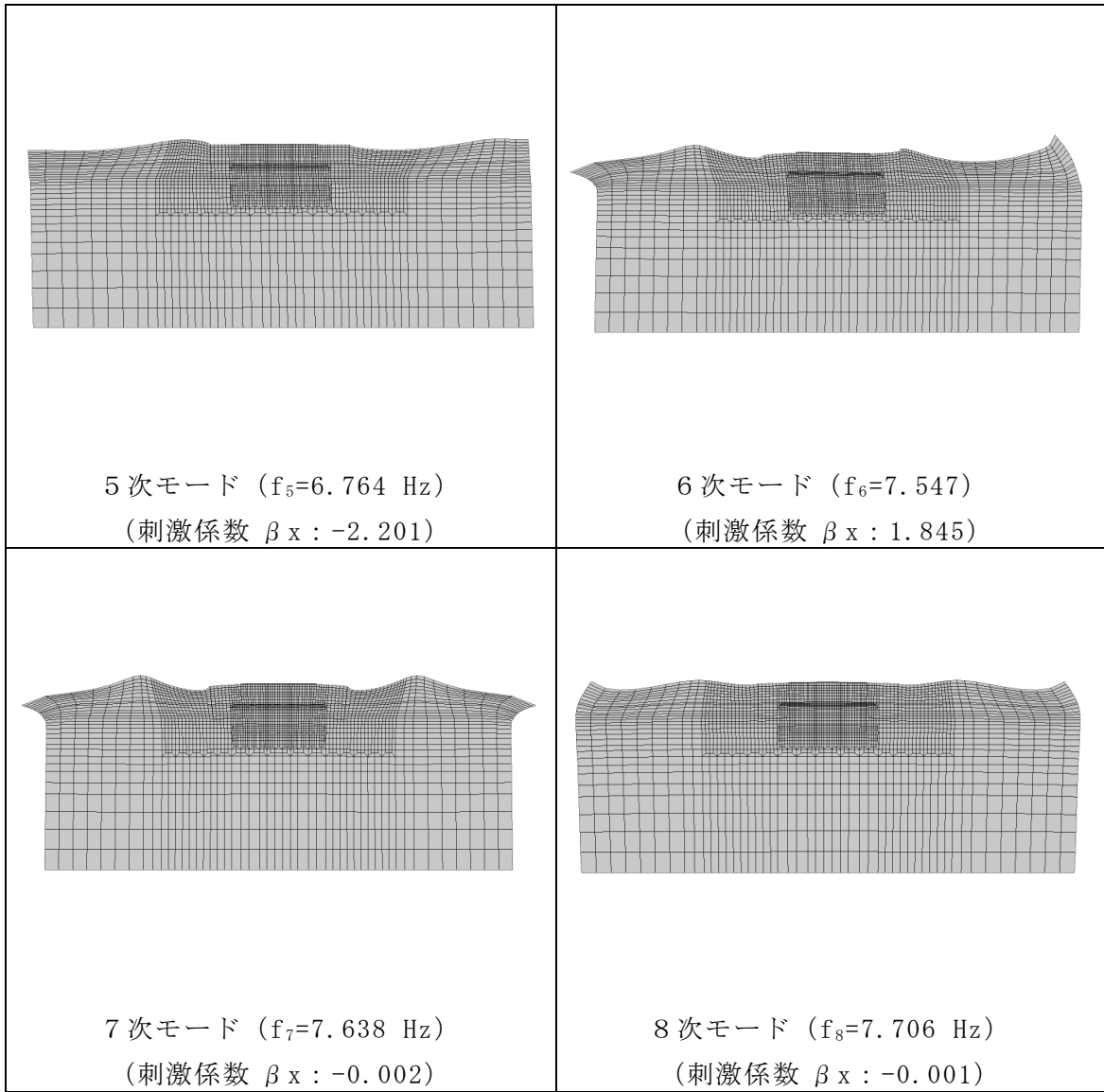
図 3-31(2) 固有値解析結果 (モード図) (B-B断面)
