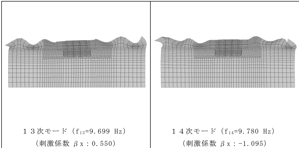
図 3-32(4) 固有値解析結果 (モード図) (C-C 断面)
