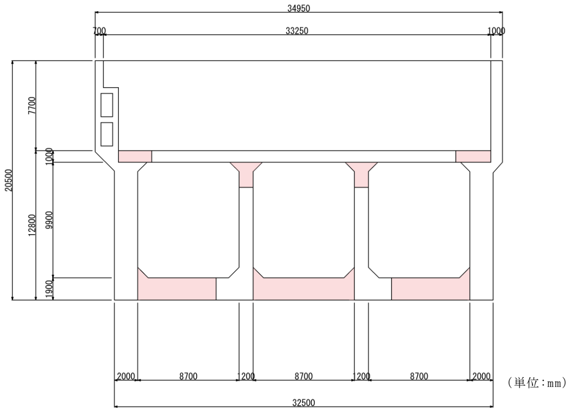
図 2-15 補強計画図 (断面図 (B-B 断面))
