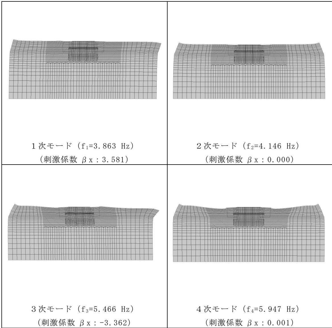
図 3-31(1) 固有値解析結果 (モード図) (B-B断面)
