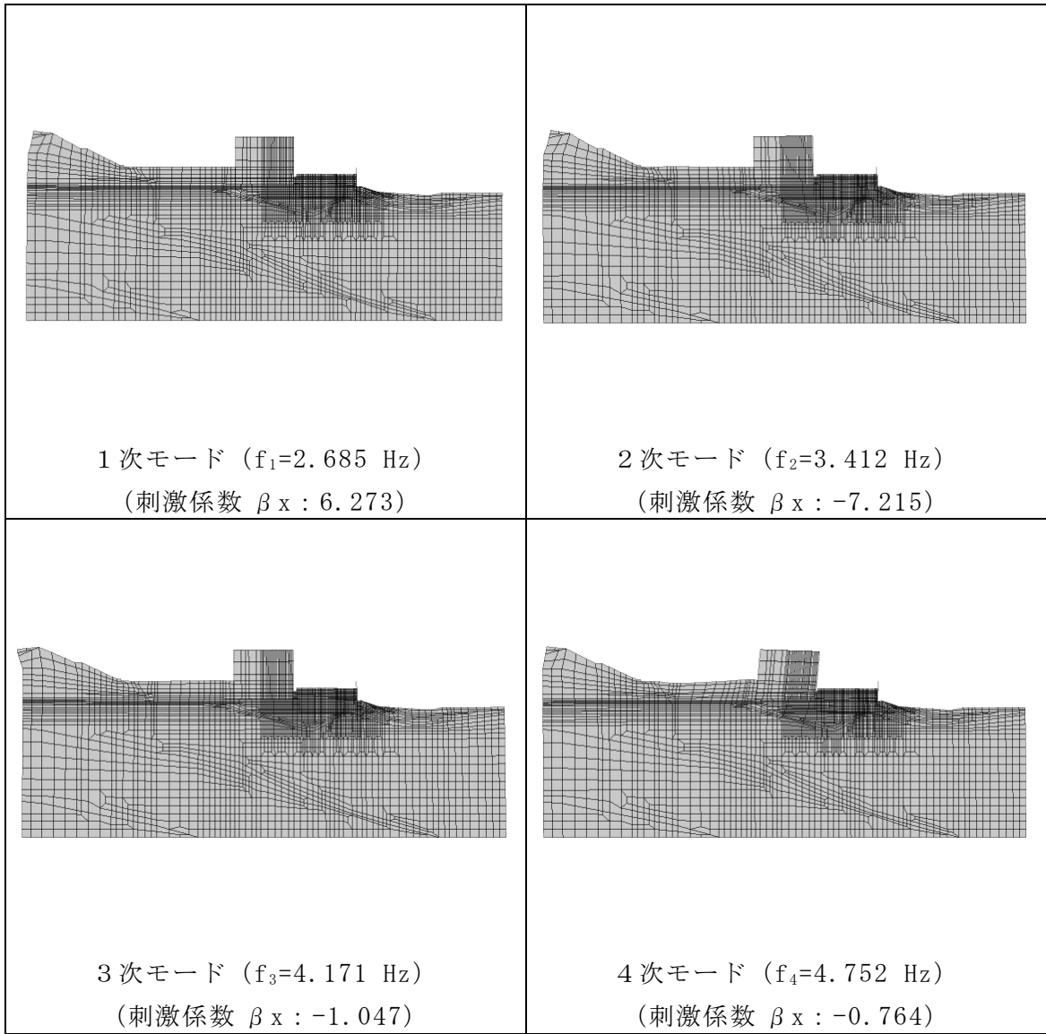
図 3-33(1) 固有値解析結果 (モード図) (D-D断面)
