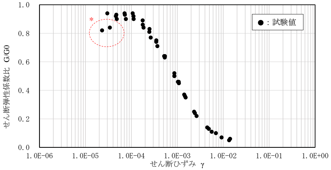
図 2-3 碎石における G/G_0 のひずみ依存特性
