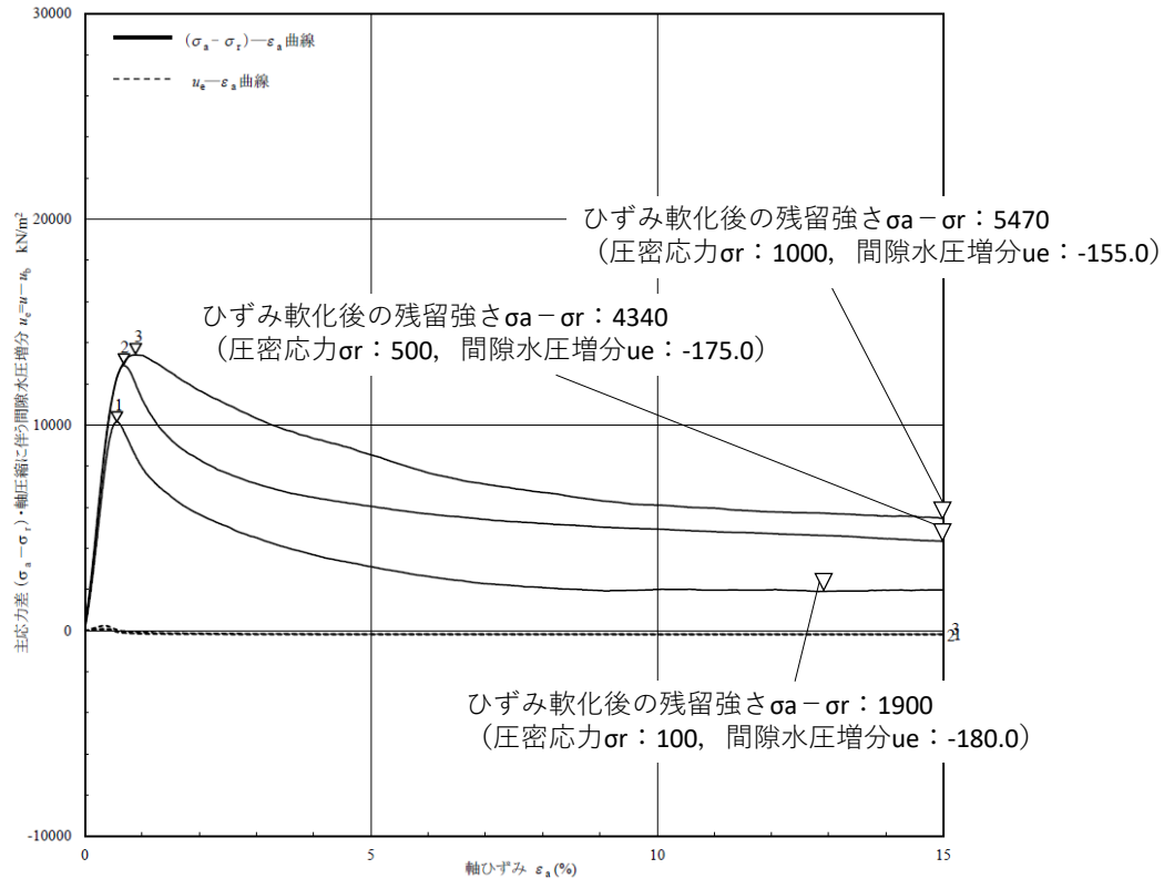
図 2.3.3-1 三軸圧縮試験における軸差応力－軸ひずみ関係
