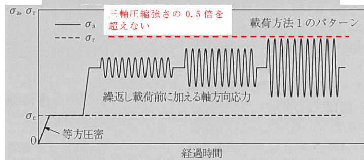
図 4.4.3-4 J G S 2563 载荷方法の模式図等(一部加筆)
