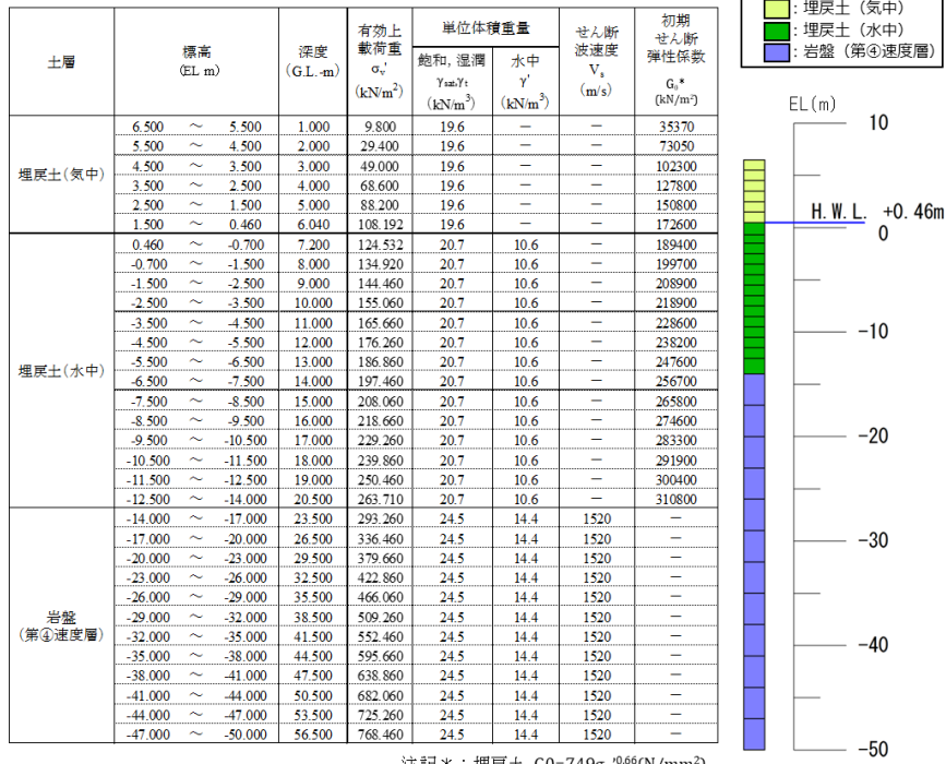
(a) 基本物性 (比較地点①)
