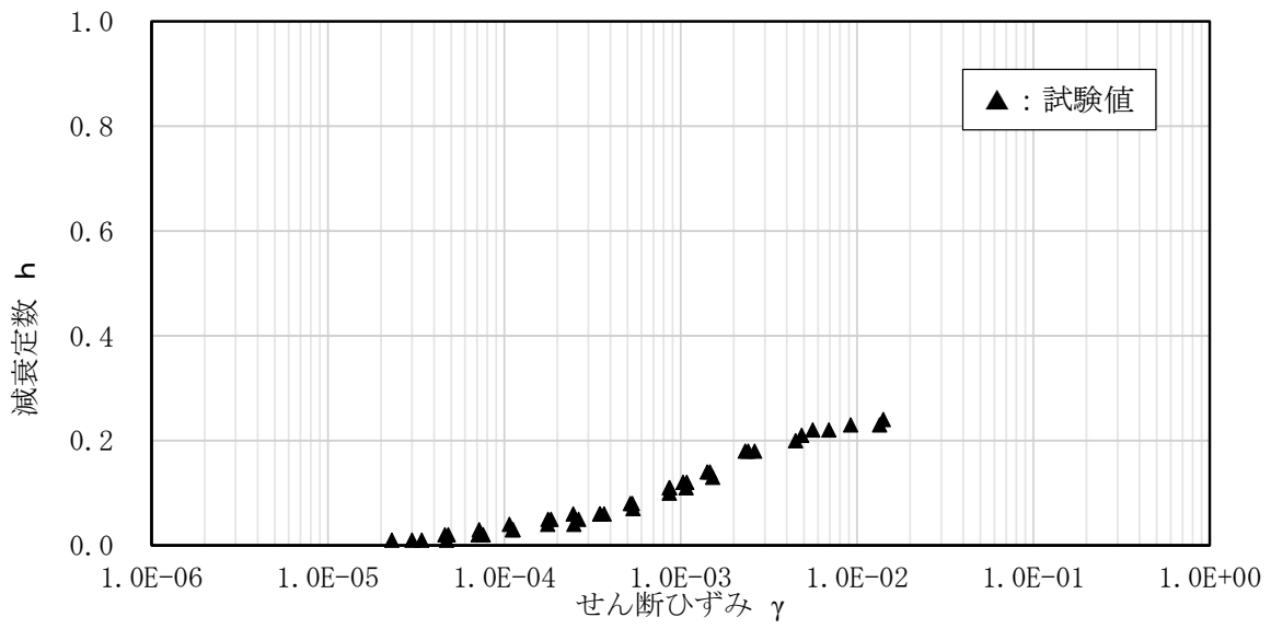
図 2-4 碎石における減衰定数のひずみ依存特性
