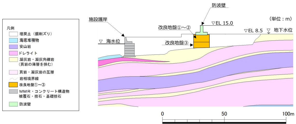
iv-iv 断面 漂流防止装置基礎 (荷揚護岸), 防波壁 (逆T擁壁) (⑥-⑥断面)
