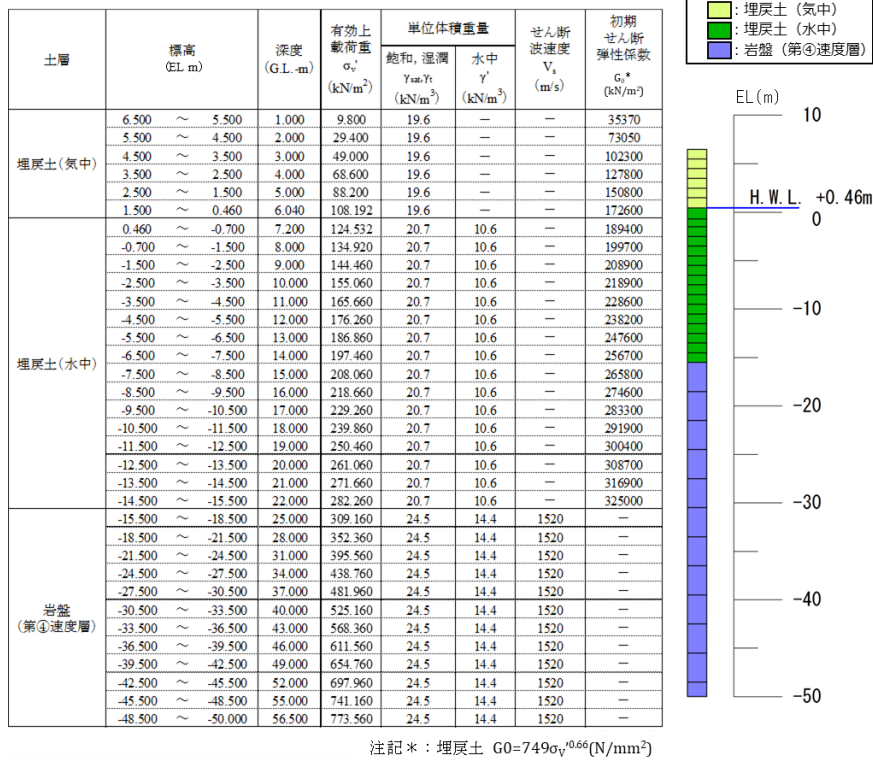
(b) 基本物性 (比較地点②)
