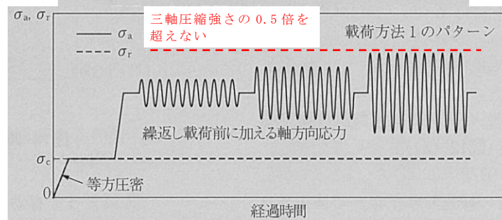
図 4.3.3-4 J G S 2563 载荷方法の模式図等(一部加筆)
