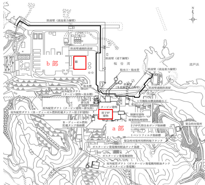
(1) P S 検層実施位置図
