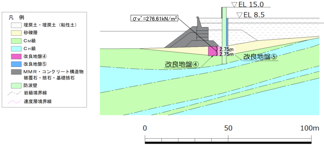
図 4.2.2-1 改良地盤④における G_{ma} 算定に用いる \sigma_v'
