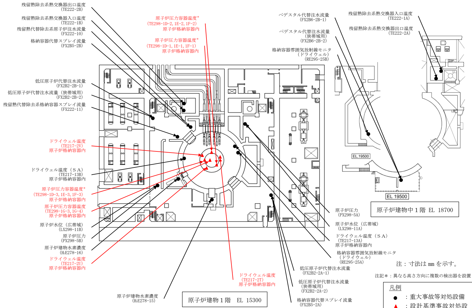
第1図 配置図 (3 / 7)
