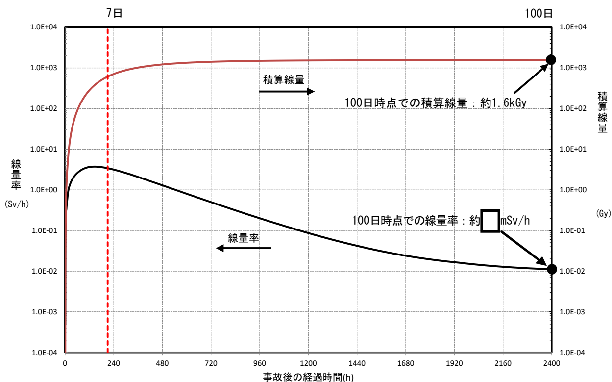
図1 原子炉格納容器内からの漏えいに起因する原子炉建物原子炉棟における事故後の線量率及び積算線量
