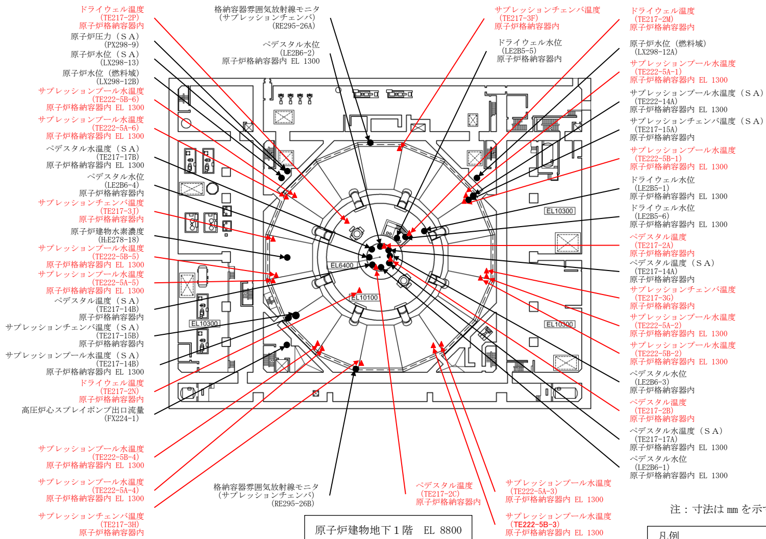
第1図 配置図 (2 / 7)
