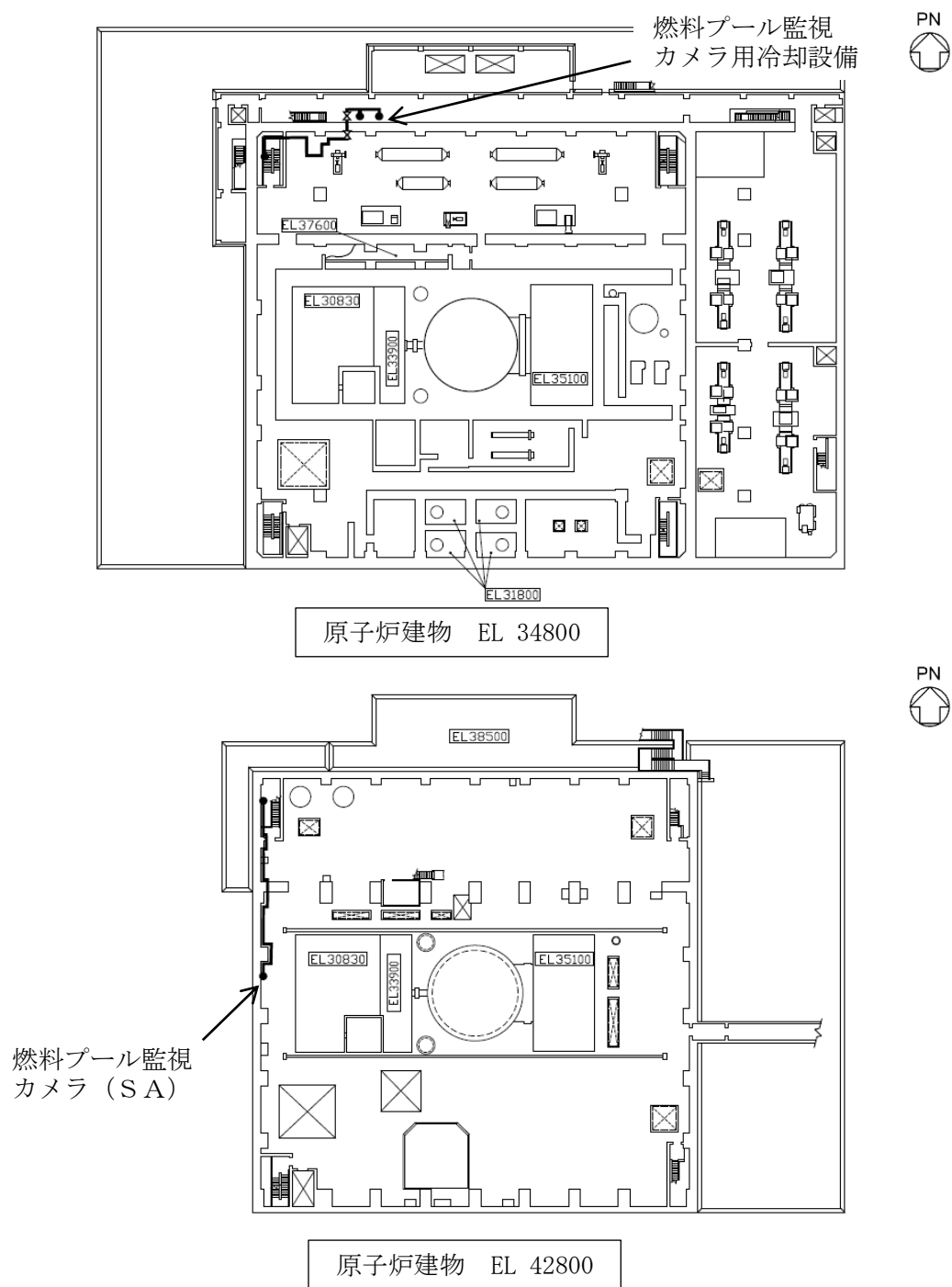
図7-1 燃料プール監視カメラ用冷却設備の配管ルート概略図
