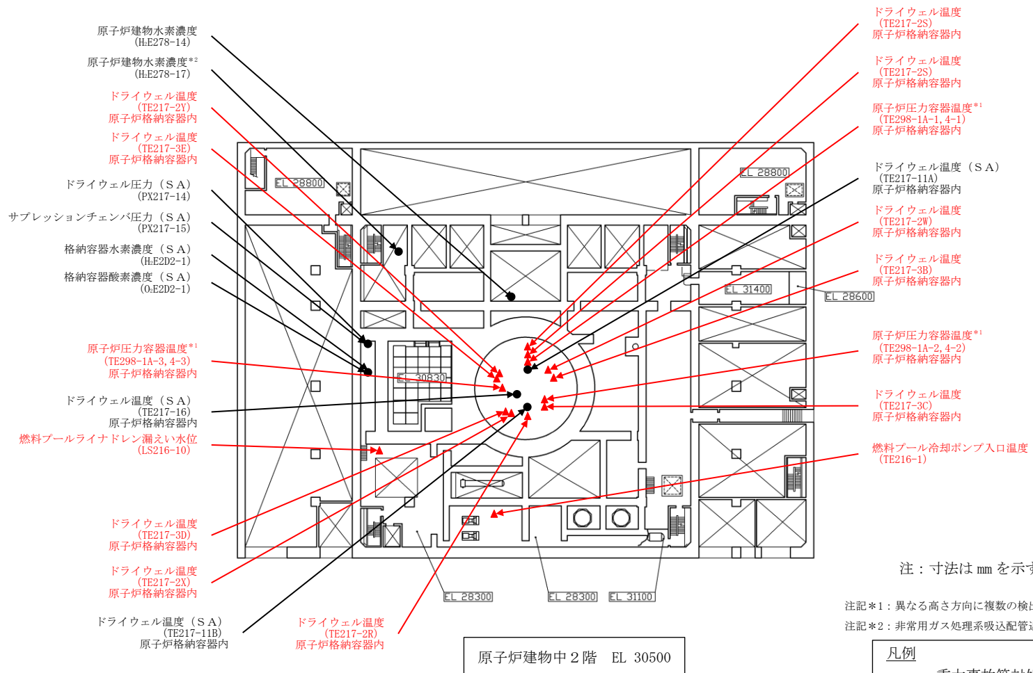
第1図 配置図 (5 / 7)
