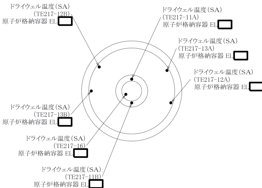
図 1 ドライウエル温度 (SA) の設置場所 (概略図)
