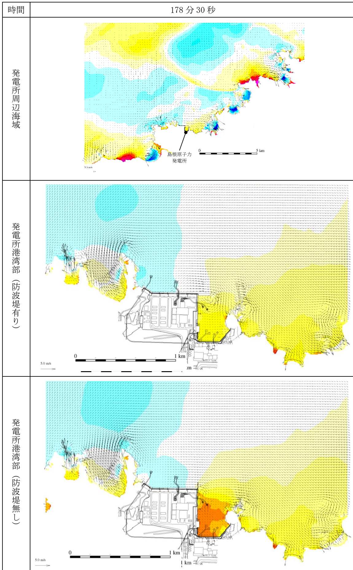
図 1-158 基準津波 1 の水位変動・流向ベクトル
