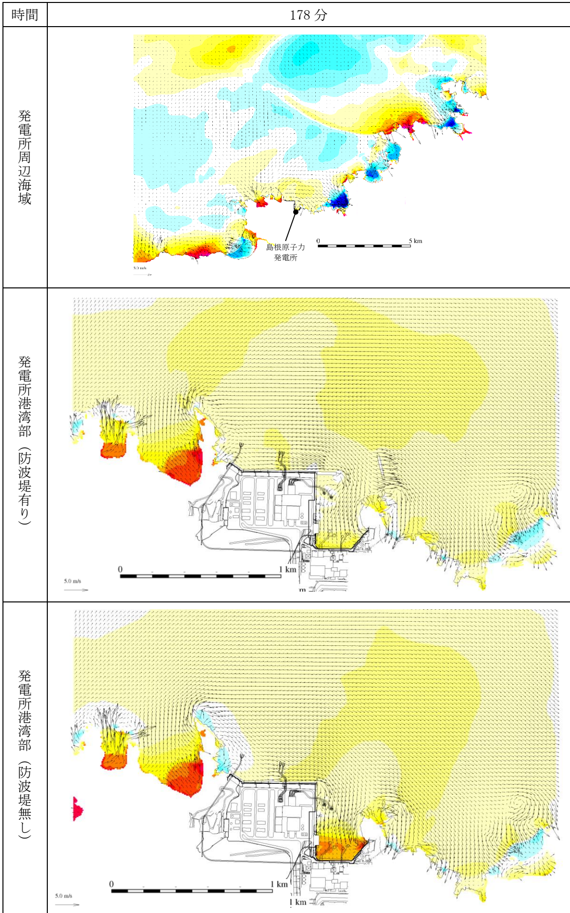
図 1-157 基準津波 1 の水位変動・流向ベクトル
