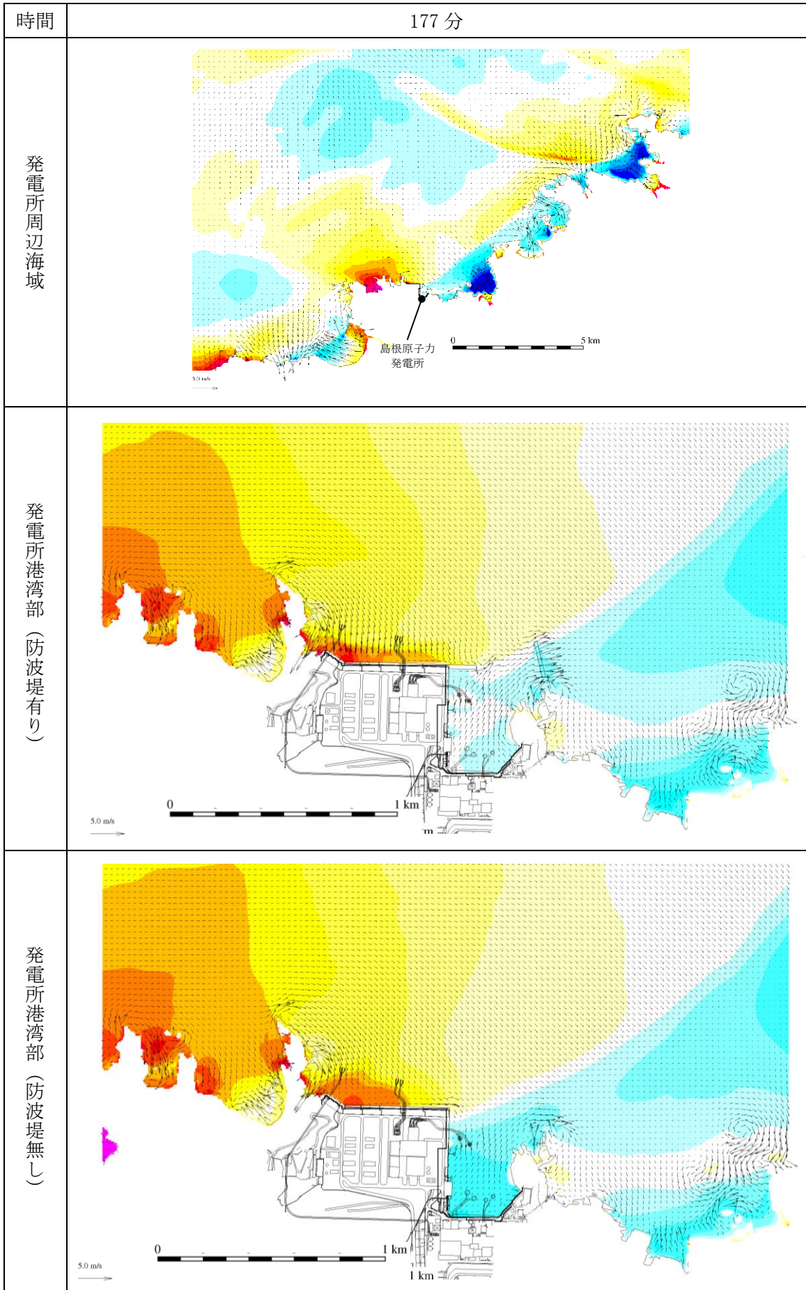
図 1-155 基準津波 1 の水位変動・流向ベクトル
