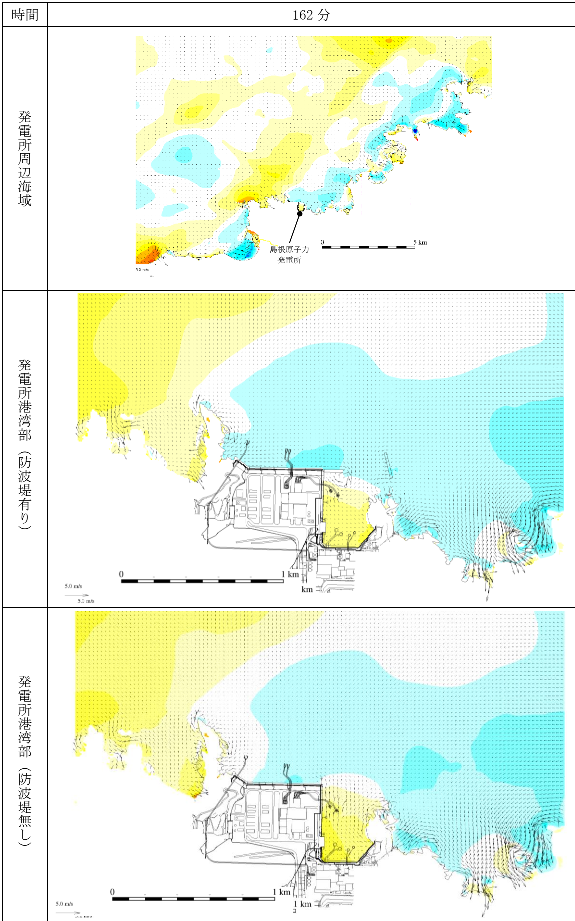
図 1-125 基準津波 1 の水位変動・流向ベクトル
