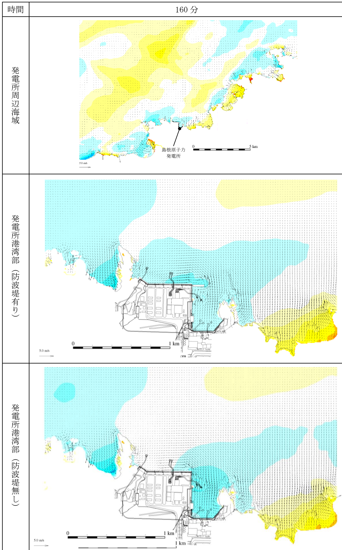
図 1-121 基準津波 1 の水位変動・流向ベクトル
