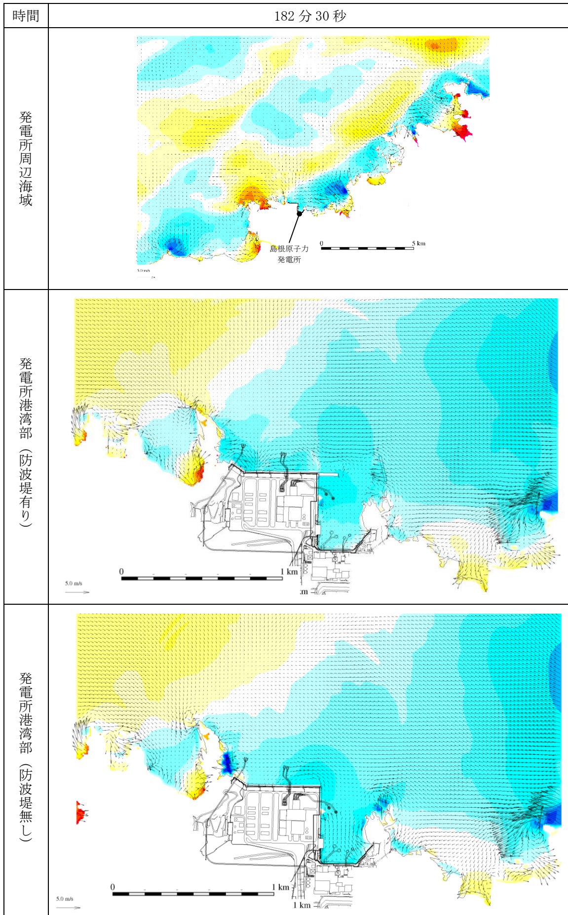
図 1-166 基準津波 1 の水位変動・流向ベクトル
