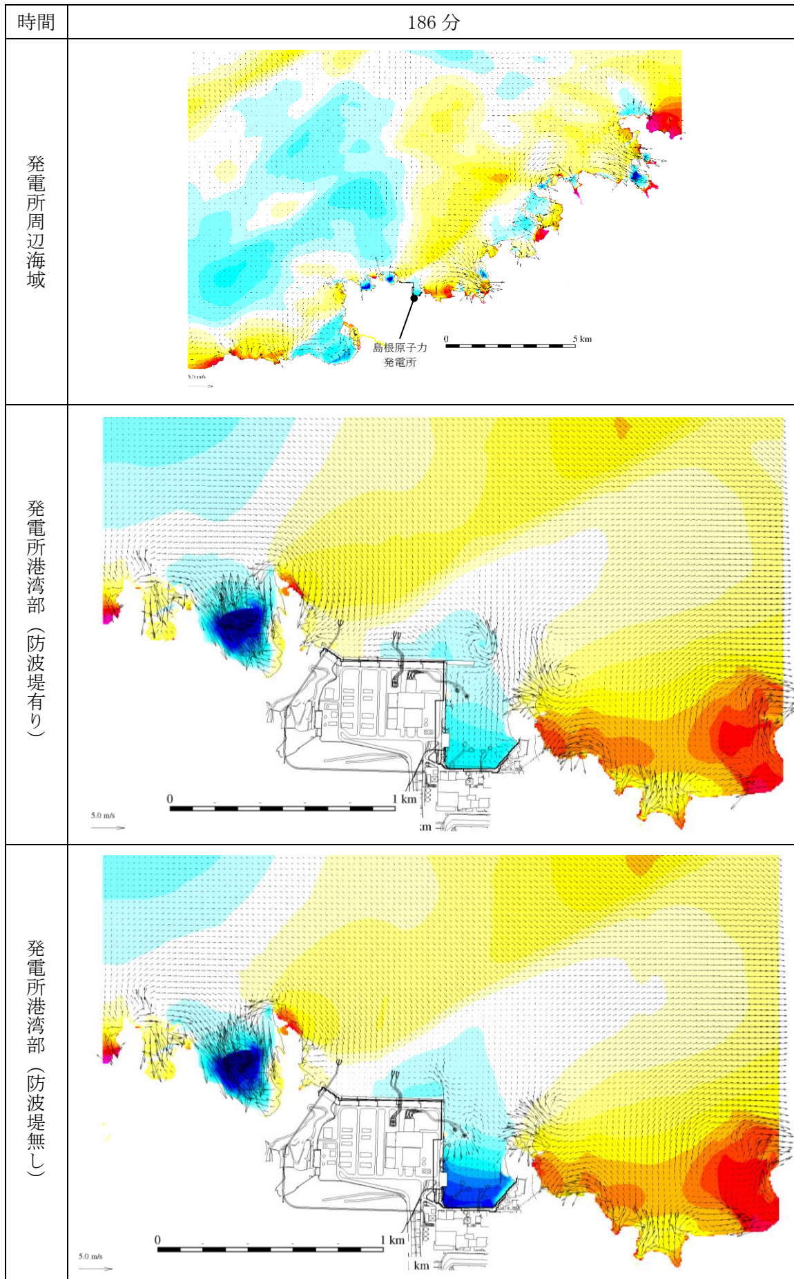
図 1-173 基準津波 1 の水位変動・流向ベクトル
