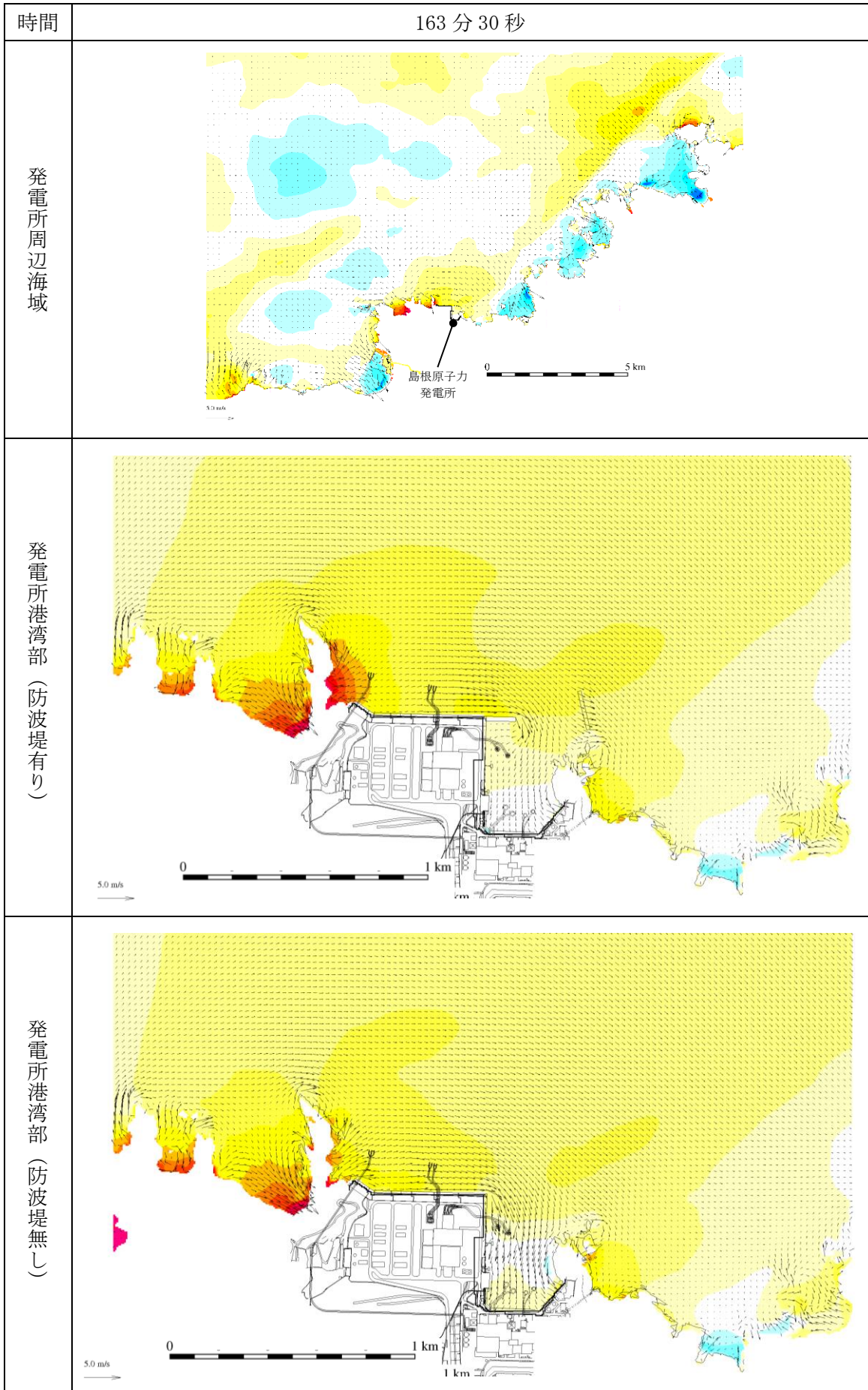
図 1-128 基準津波 1 の水位変動・流向ベクトル
