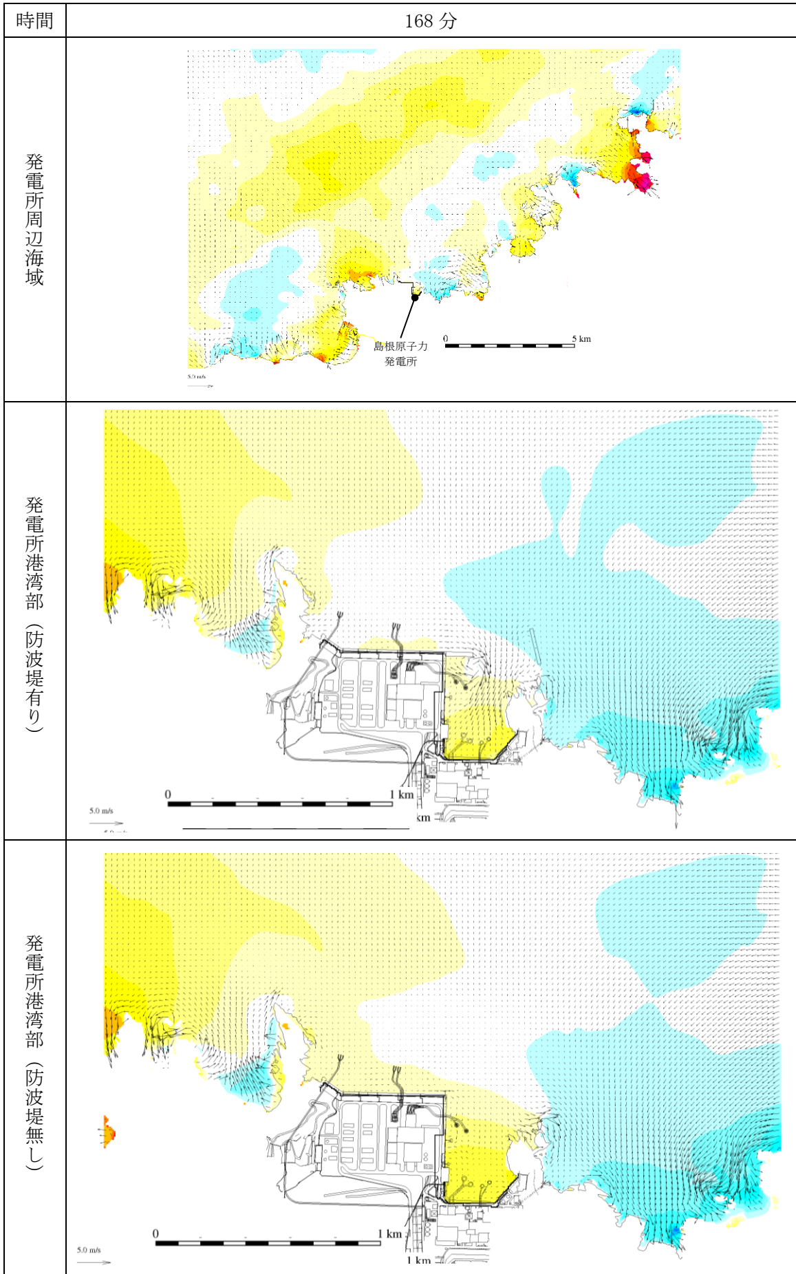
図 1-137 基準津波 1 の水位変動・流向ベクトル
