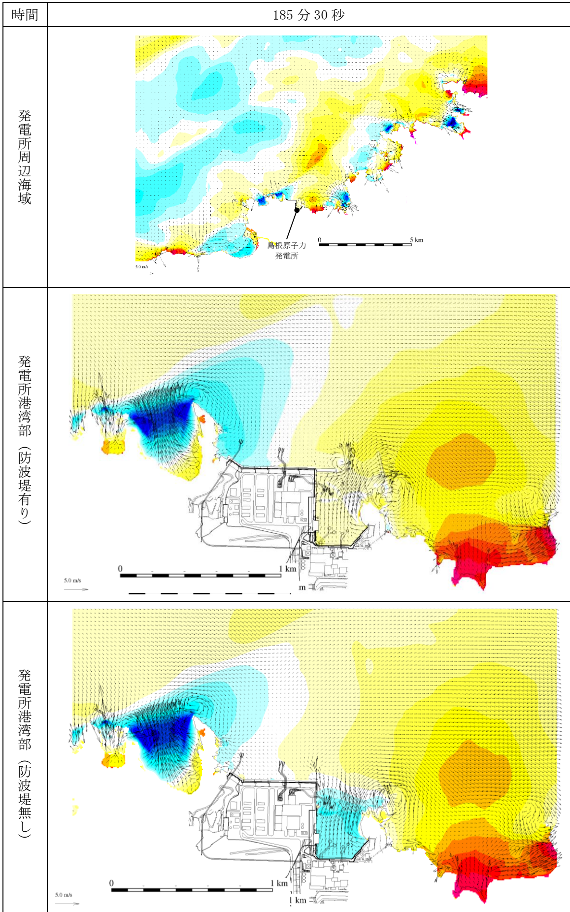
図 1-172 基準津波 1 の水位変動・流向ベクトル
