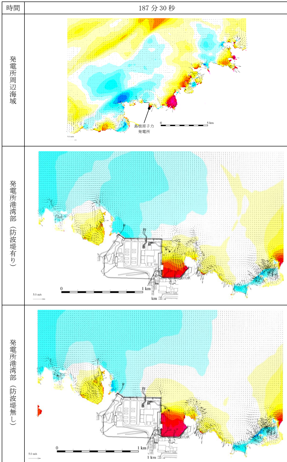
図 1-176 基準津波 1 の水位変動・流向ベクトル
