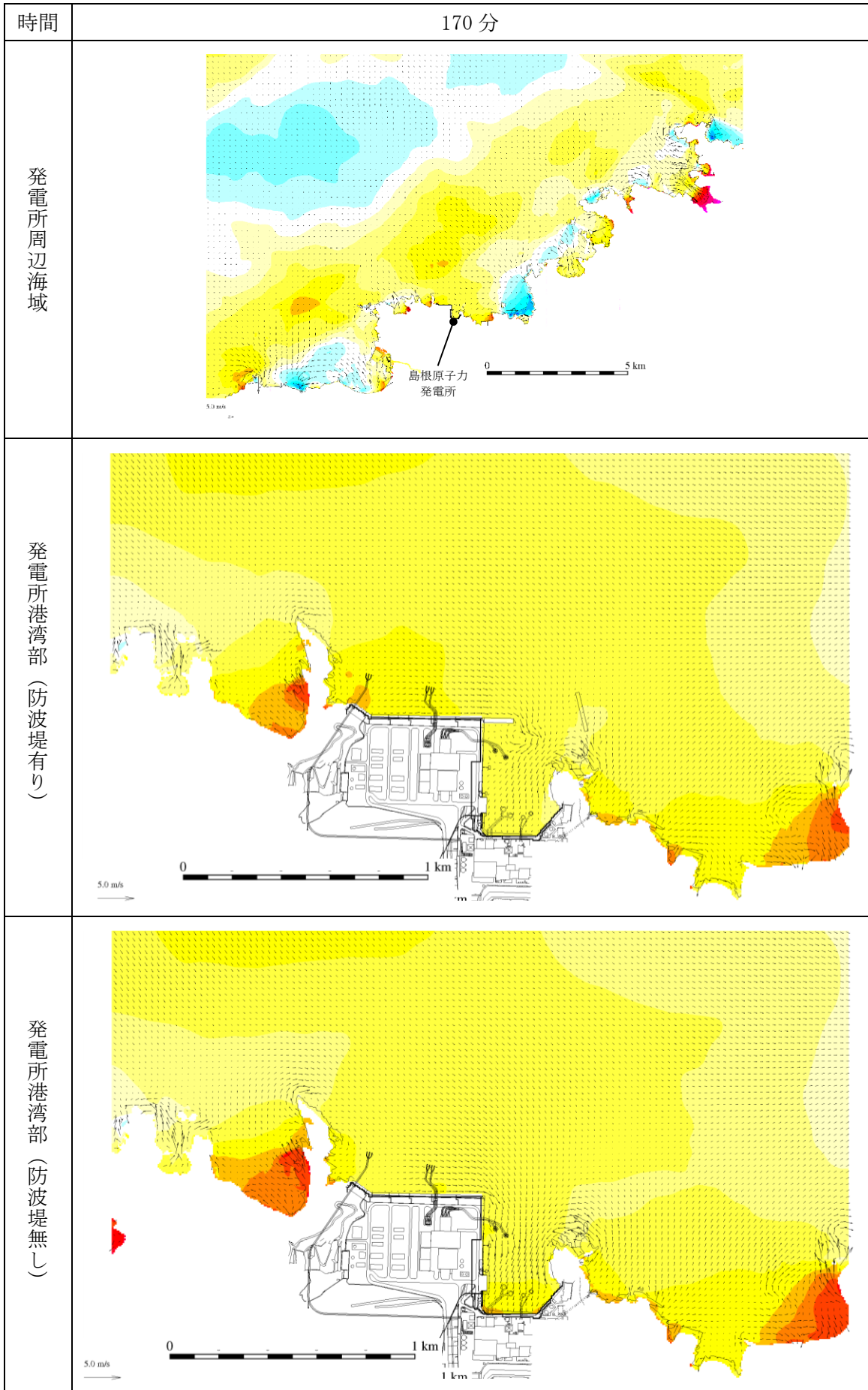
図 1-141 基準津波 1 の水位変動・流向ベクトル
