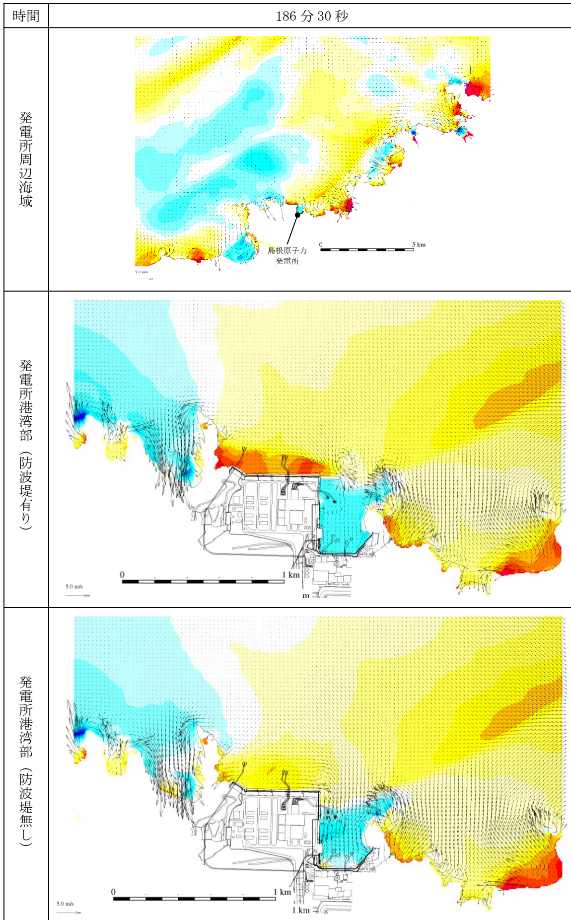
図 1-174 基準津波 1 の水位変動・流向ベクトル
