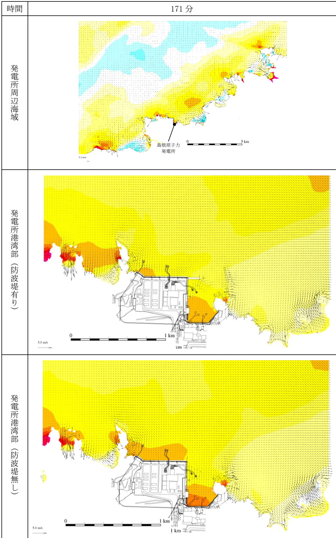
図 1-143 基準津波 1 の水位変動・流向ベクトル
