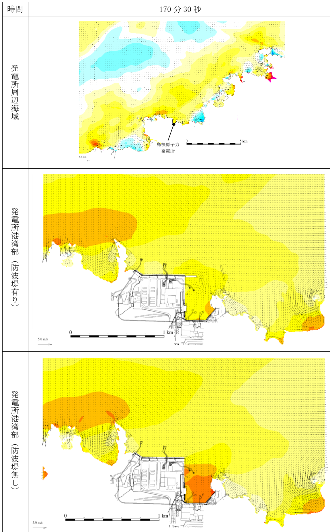
図 1-142 基準津波 1 の水位変動・流向ベクトル
