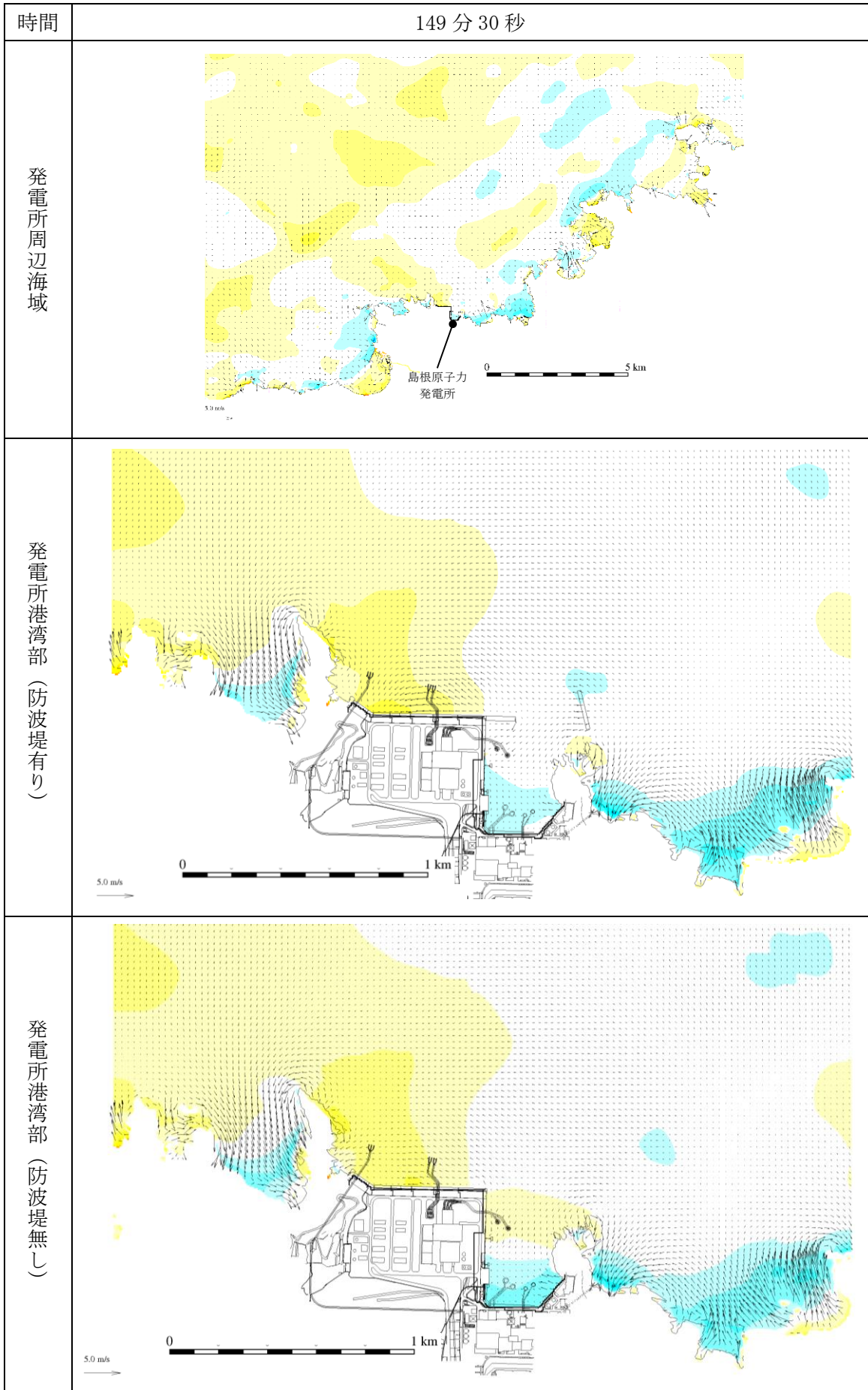
図 1-100 基準津波 1 の水位変動・流向ベクトル
