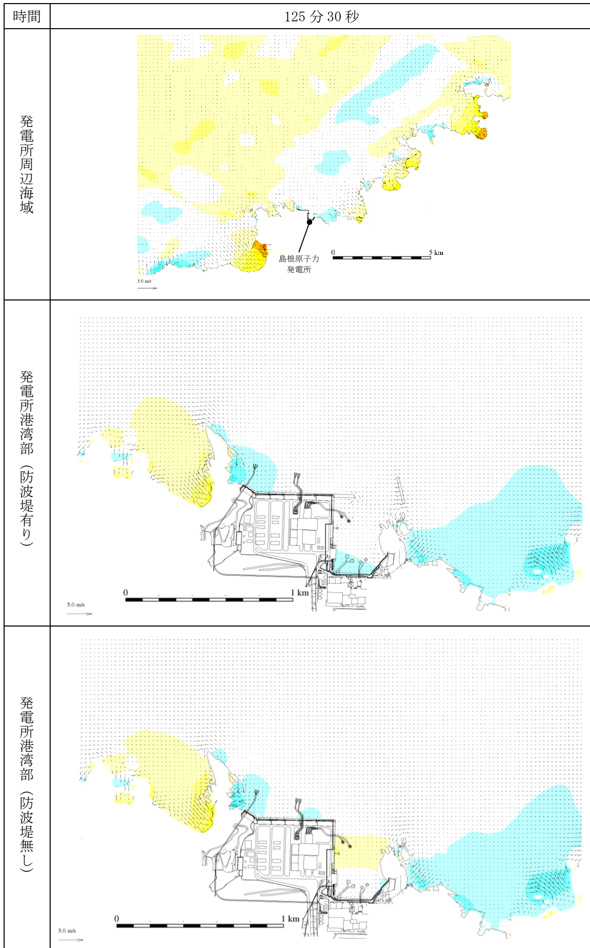
図 1-52 基準津波 1 の水位変動・流向ベクトル
