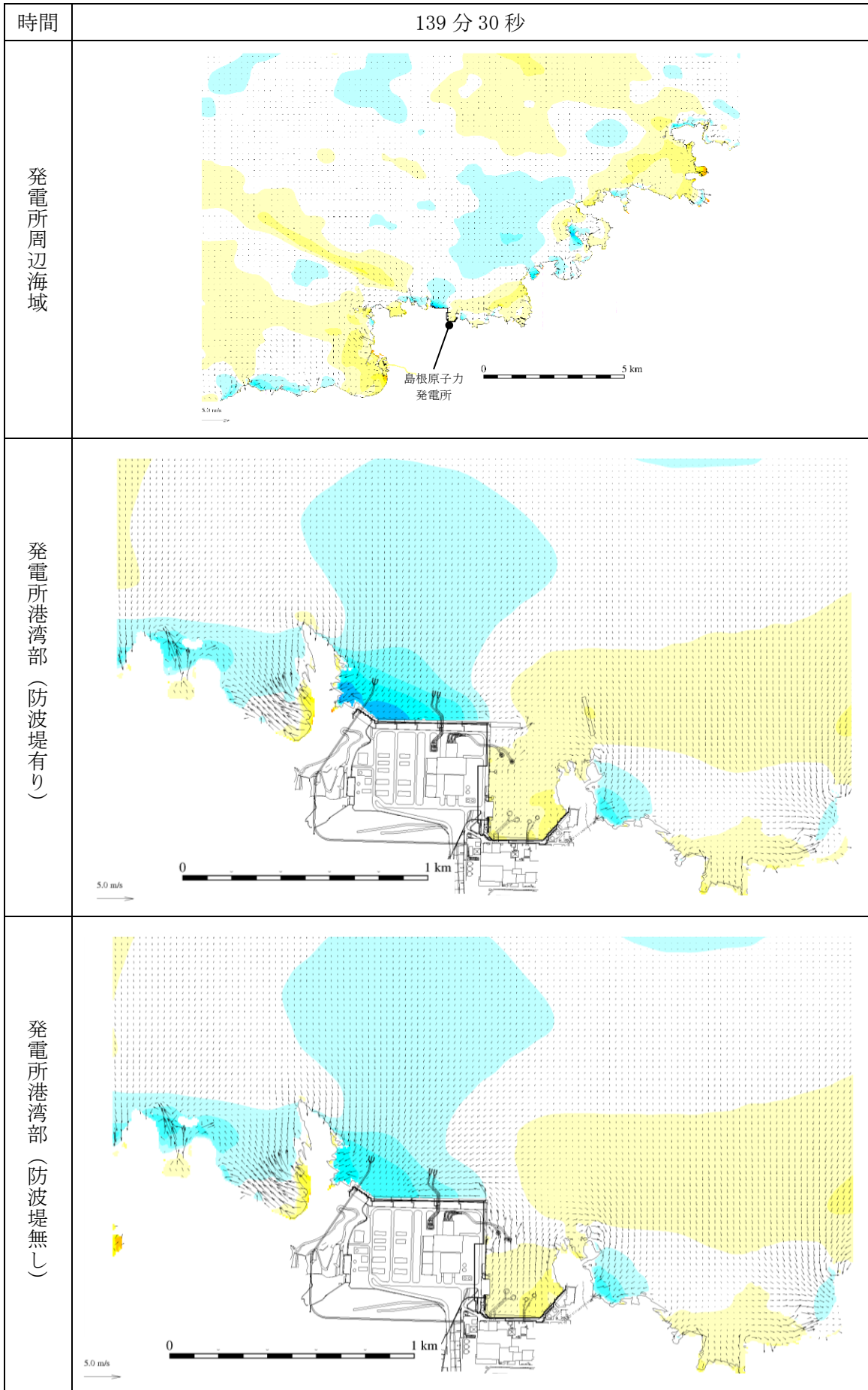
図 1-80 基準津波 1 の水位変動・流向ベクトル
