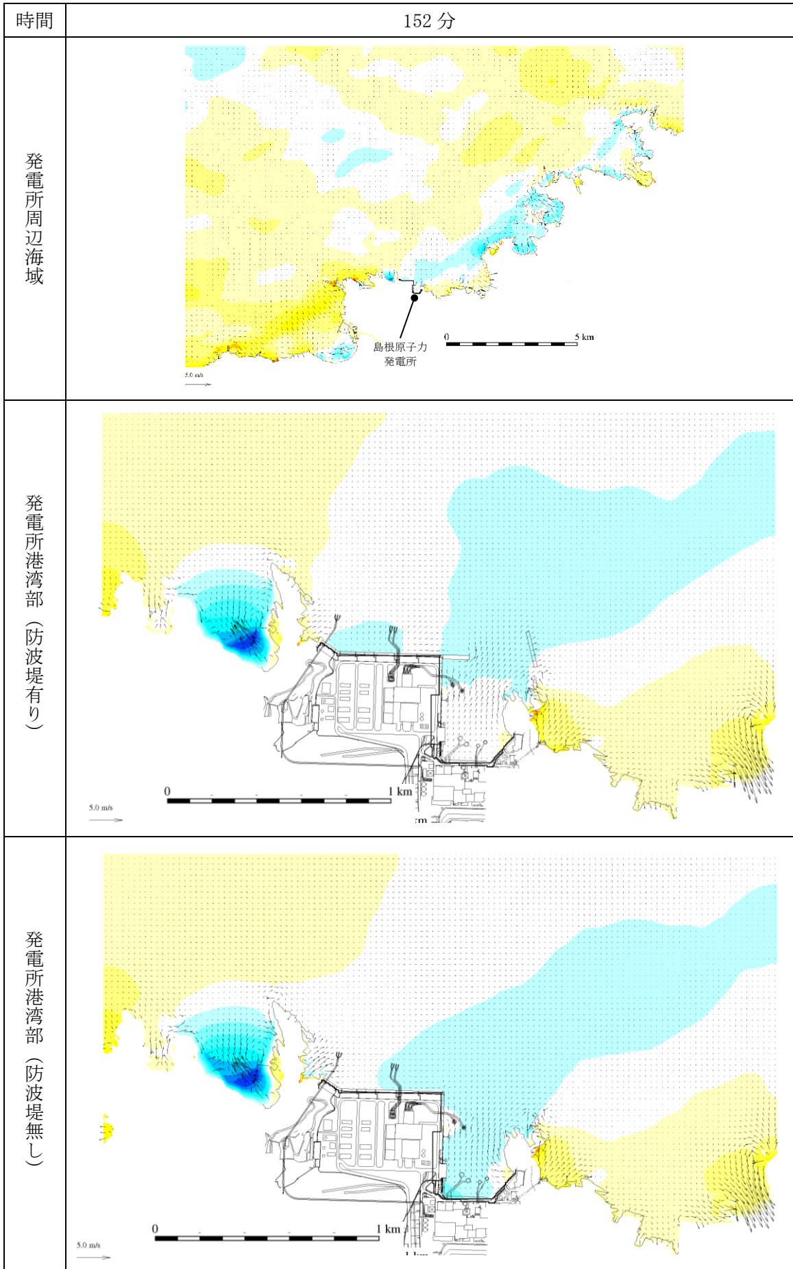
図 1-105 基準津波 1 の水位変動・流向ベクトル
