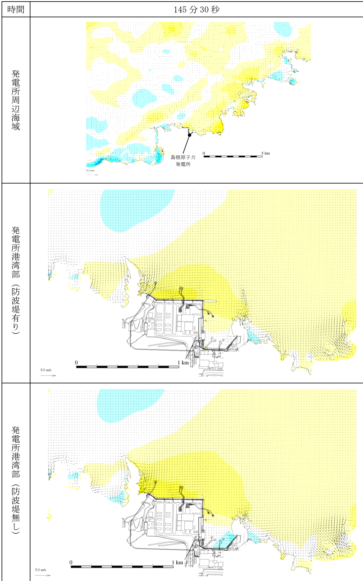
図 1-92 基準津波 1 の水位変動・流向ベクトル
