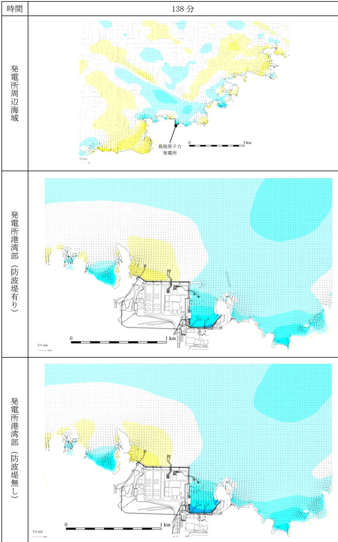
図 1-77 基準津波 1 の水位変動・流向ベクトル
