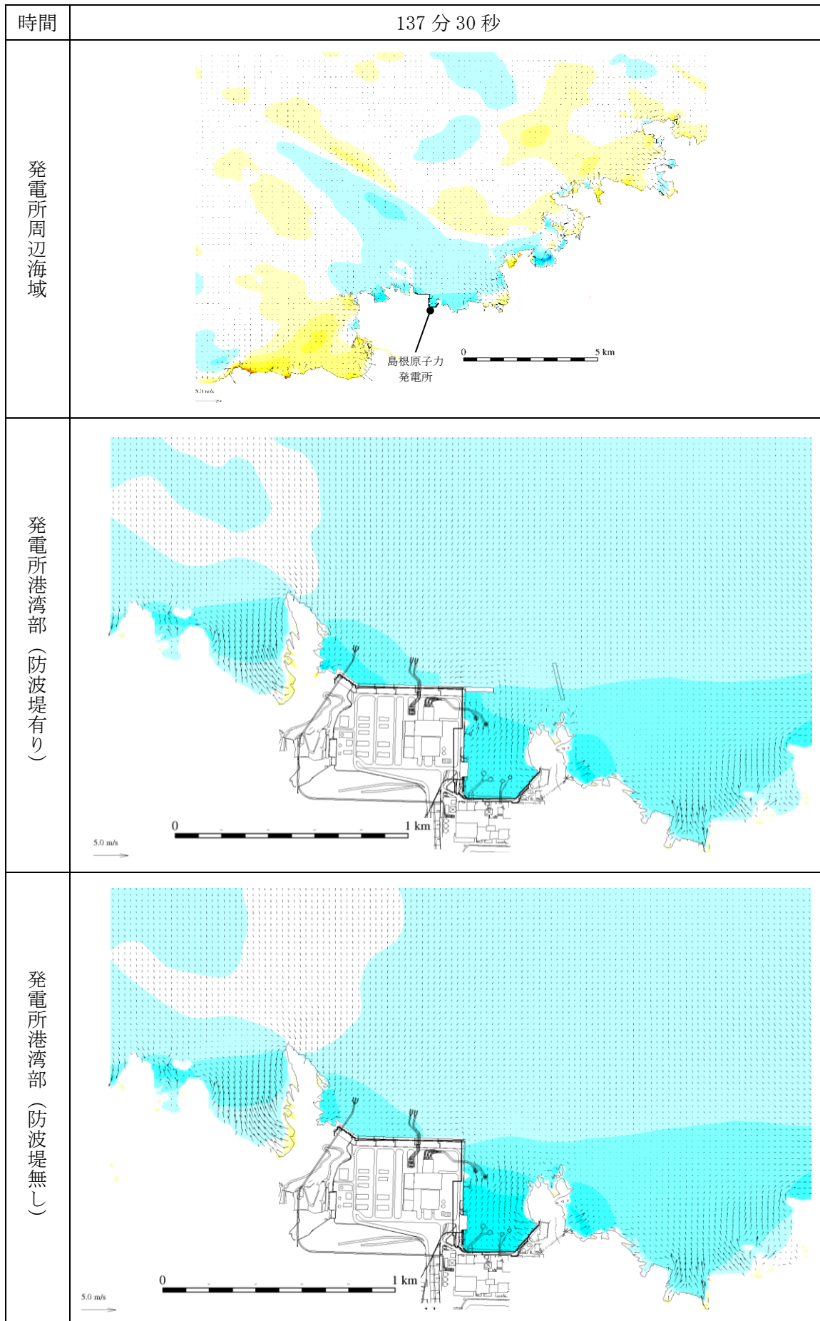
図 1-76 基準津波 1 の水位変動・流向ベクトル
