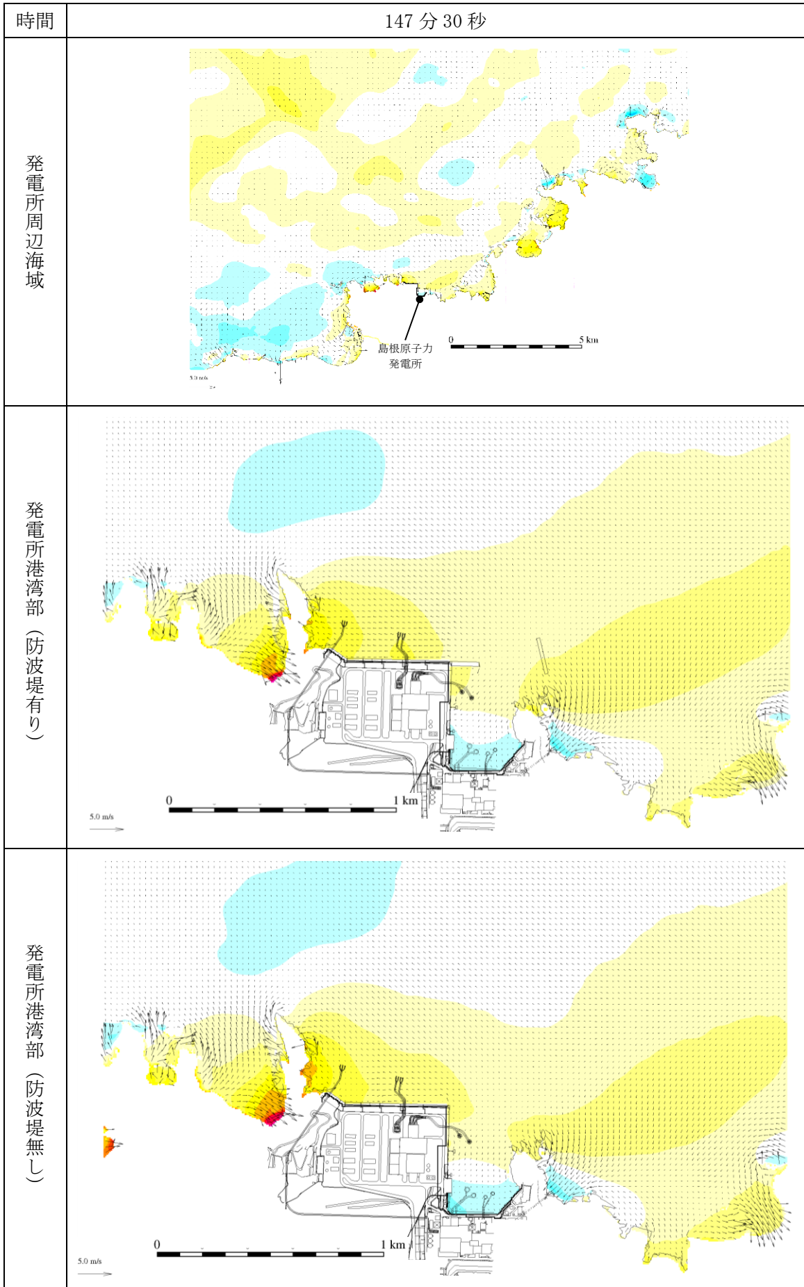
図 1-96 基準津波 1 の水位変動・流向ベクトル
