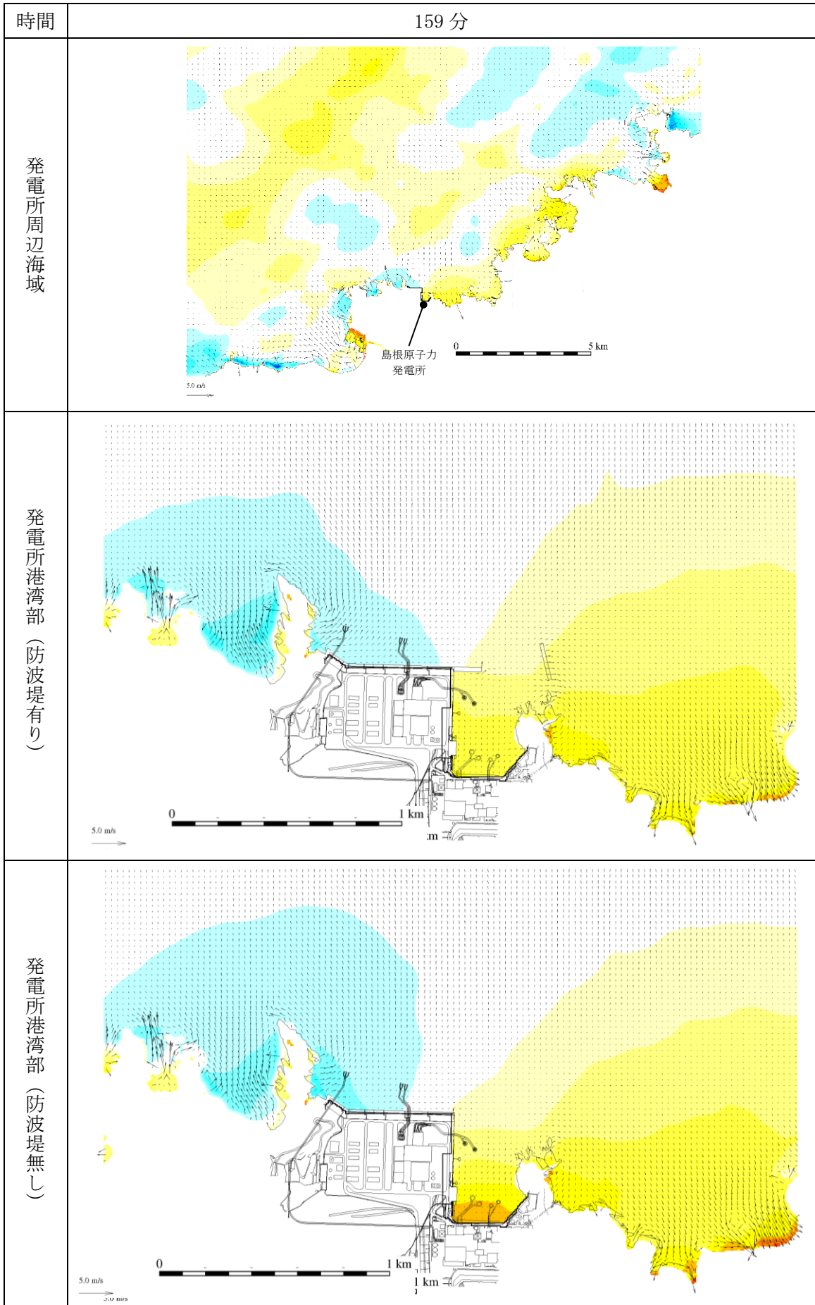
図 1-119 基準津波 1 の水位変動・流向ベクトル
