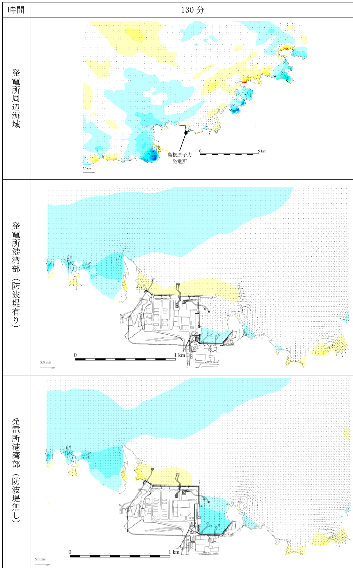
図 1-61 基準津波 1 の水位変動・流向ベクトル
