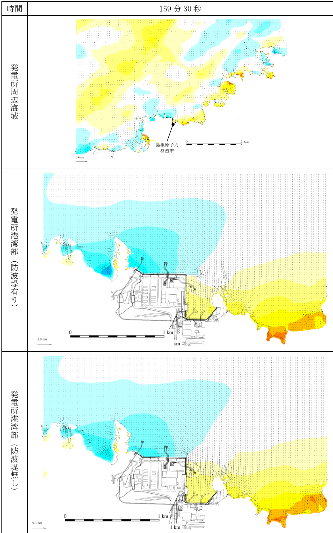
図 1-120 基準津波 1 の水位変動・流向ベクトル
