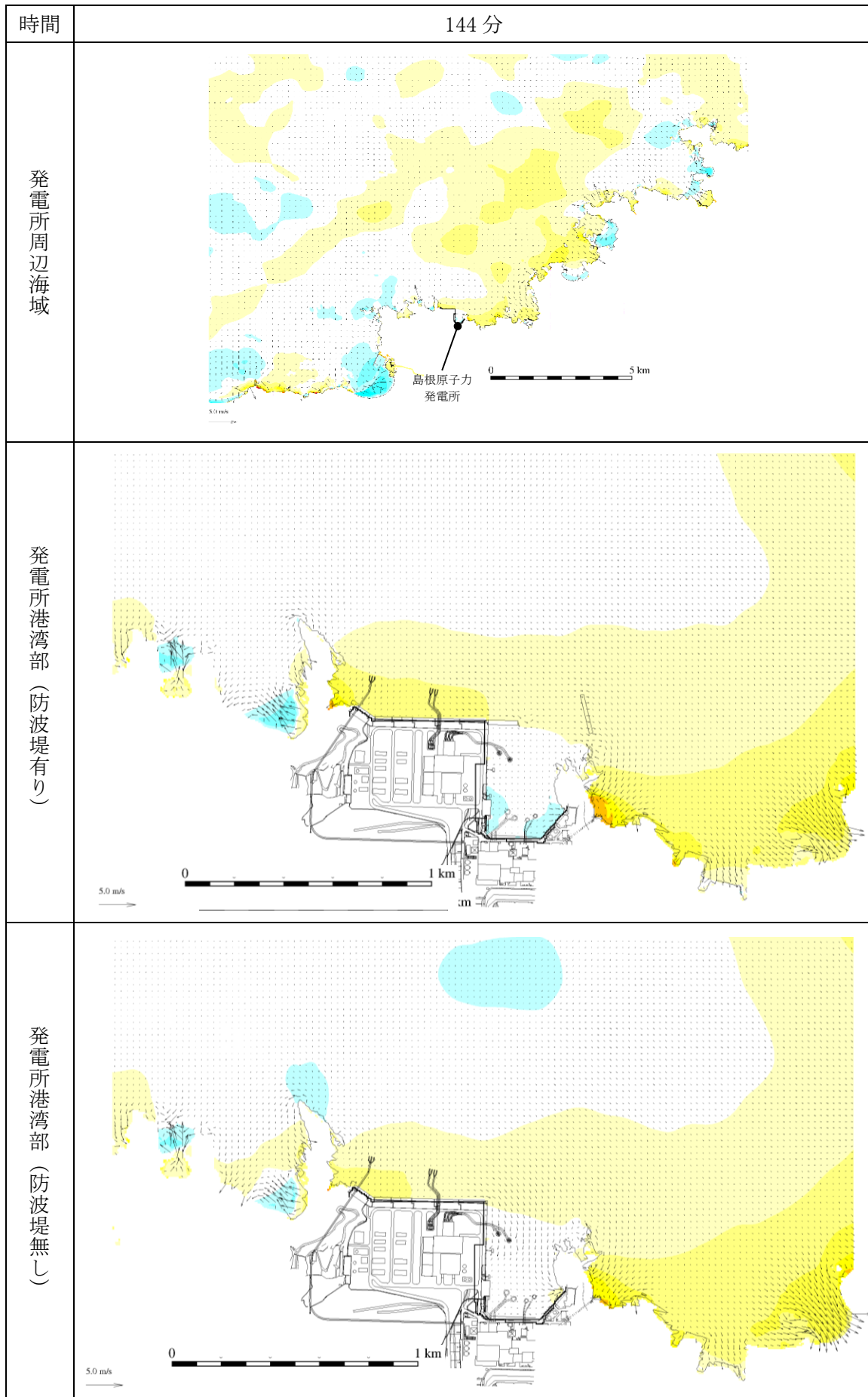
図 1-89 基準津波 1 の水位変動・流向ベクトル
