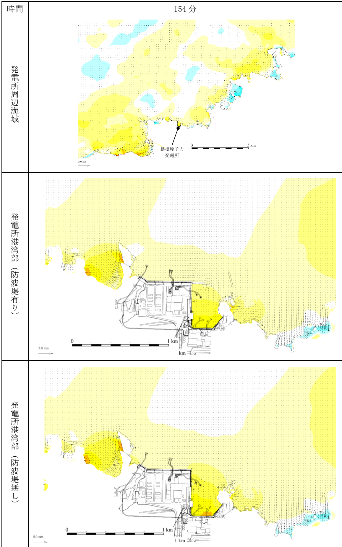
図 1-109 基準津波 1 の水位変動・流向ベクトル
