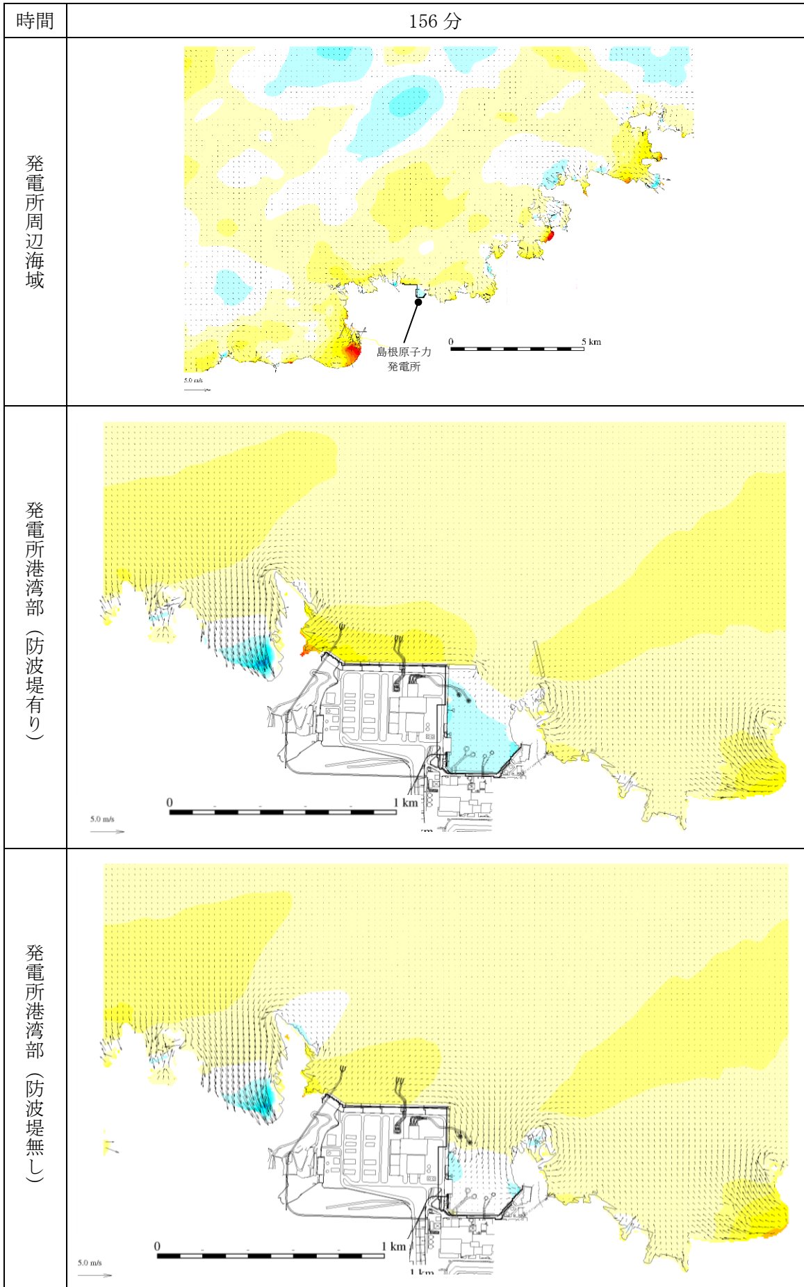
図 1-113 基準津波 1 の水位変動・流向ベクトル
