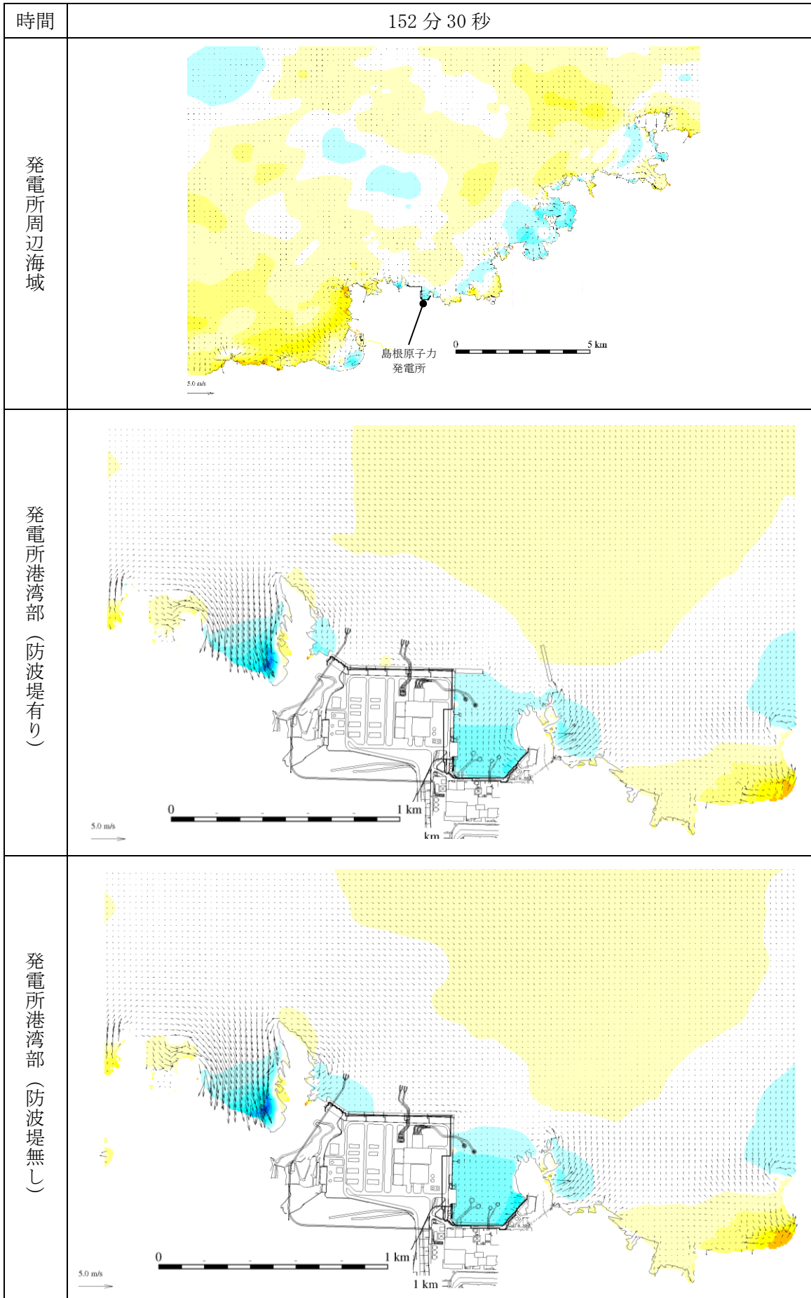
図 1-106 基準津波 1 の水位変動・流向ベクトル
