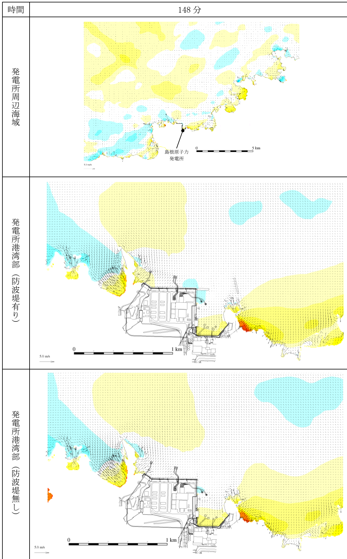
図 1-97 基準津波 1 の水位変動・流向ベクトル
