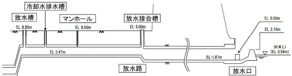
図 1.4-2-8 1号機放水施設断面図
