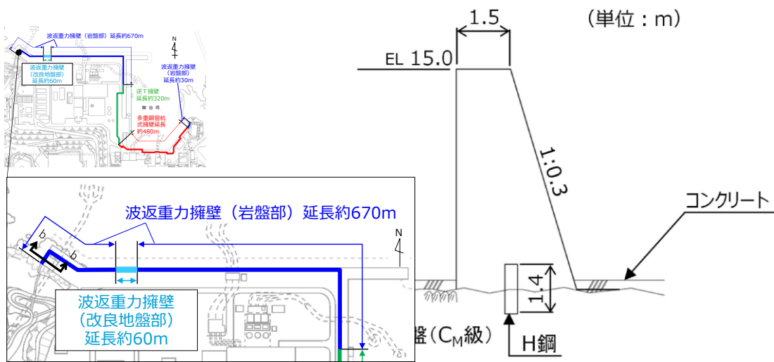
図 1.2-11 防波壁 (波返重力擁壁) 西端部 (b - b 断面) 断面図
