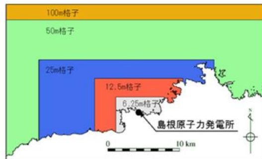
計算格子分割
