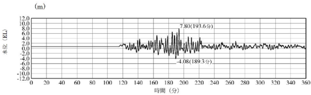
3号機取水槽最大ケース
