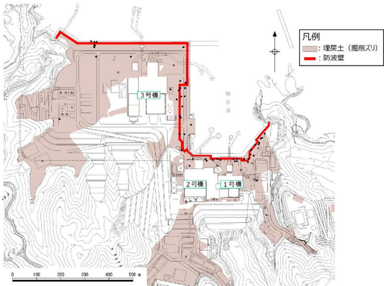
図 1.2-26(1) 埋戻土分布図
