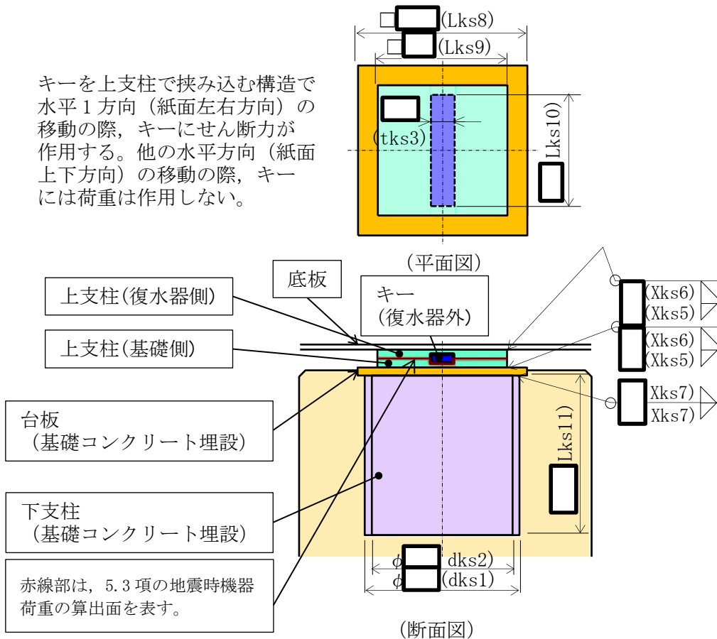
図 7.12-17 キーサポート⑩⑪平面図，断面図
