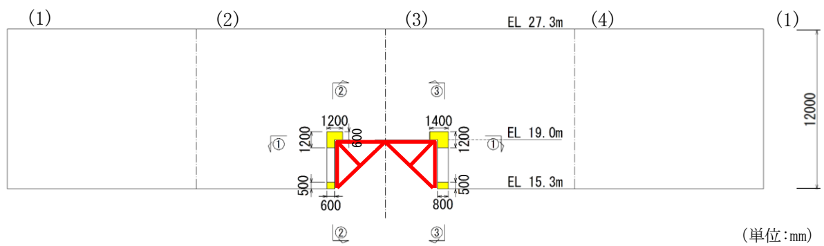
図 2.2-3 補助復水貯蔵タンク遮蔽壁の断面図 (A-A 断面, 東西)
