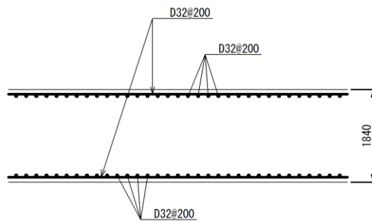
図 2.2-6(1) 補助復水貯蔵タンク遮蔽壁の概略配筋図
