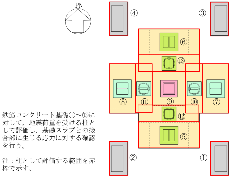
図 7.12-18 基礎コンクリートの評価
