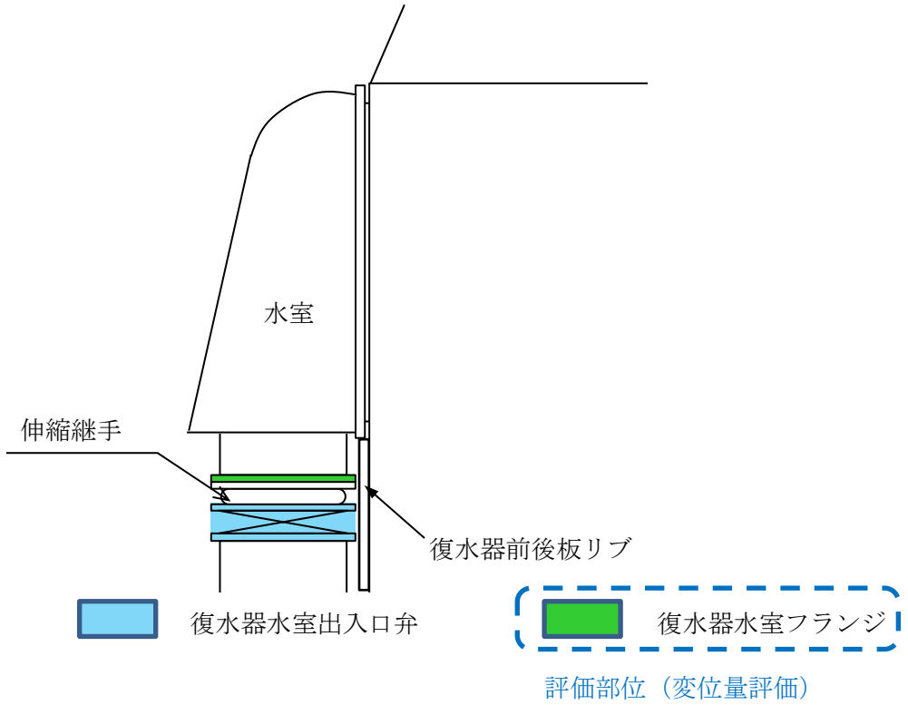
図 7.12-19 復水器水室出入口弁，復水器水室フランジ
