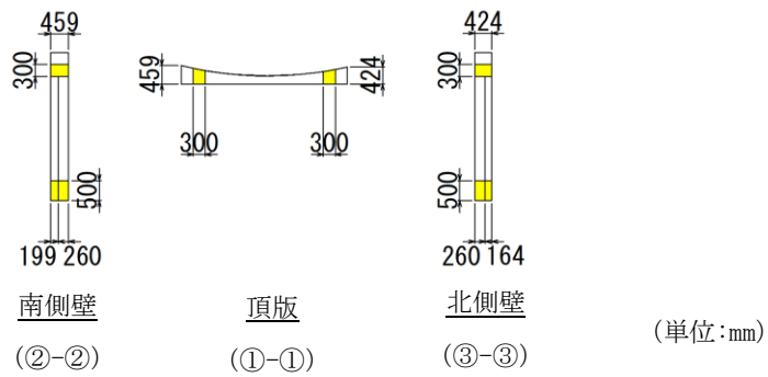
図 1-4 トーラス水受入タンク遮蔽壁の PHb による耐震補強の概要
