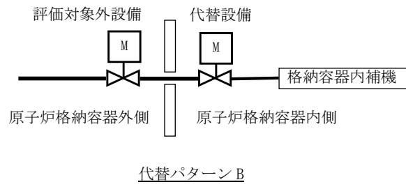
図 1.2-2 系統概略図
