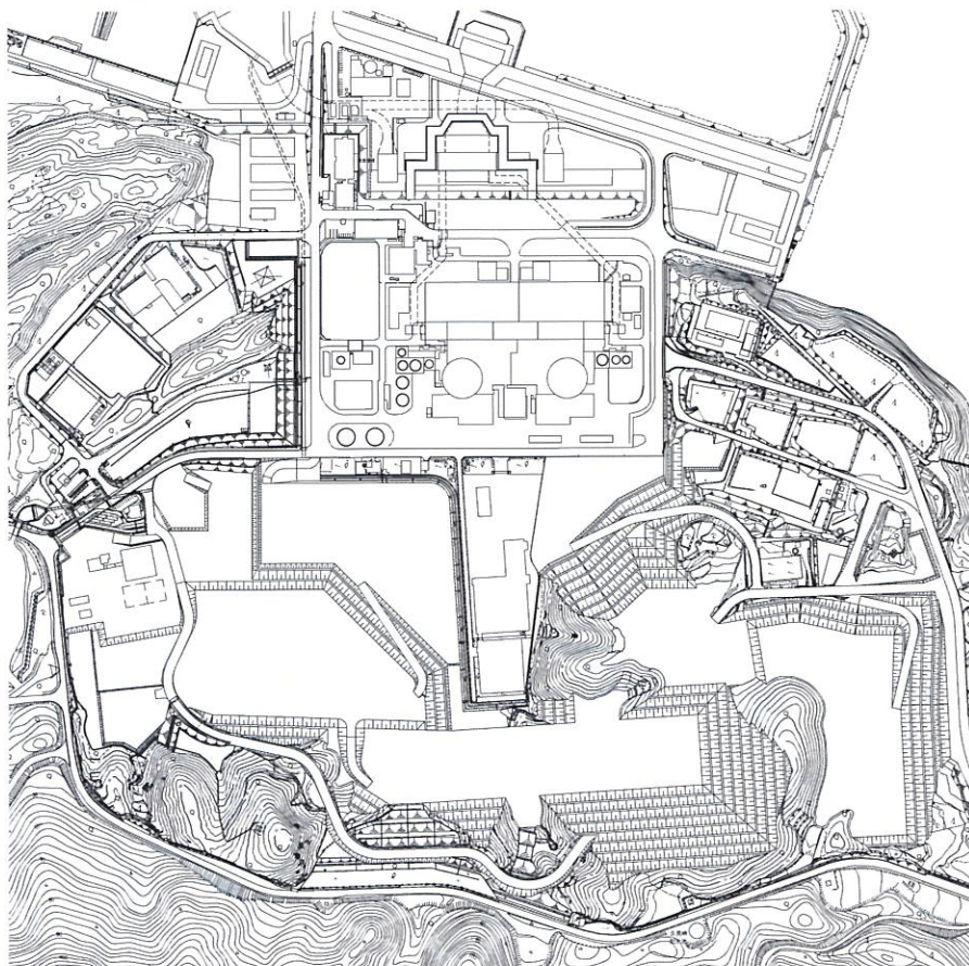
既許可時点の敷地平面図(2017年2月8日)
