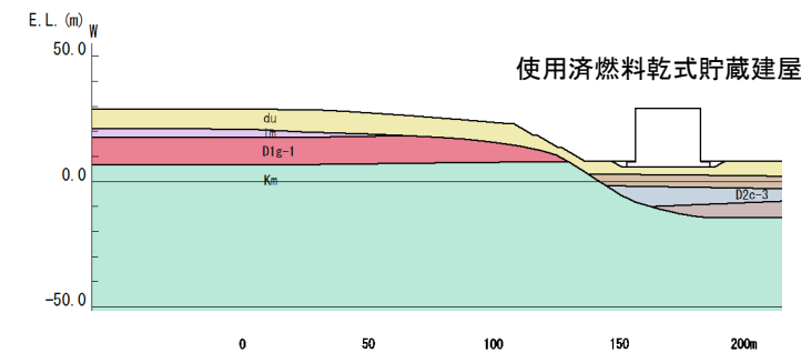
地質断面図
