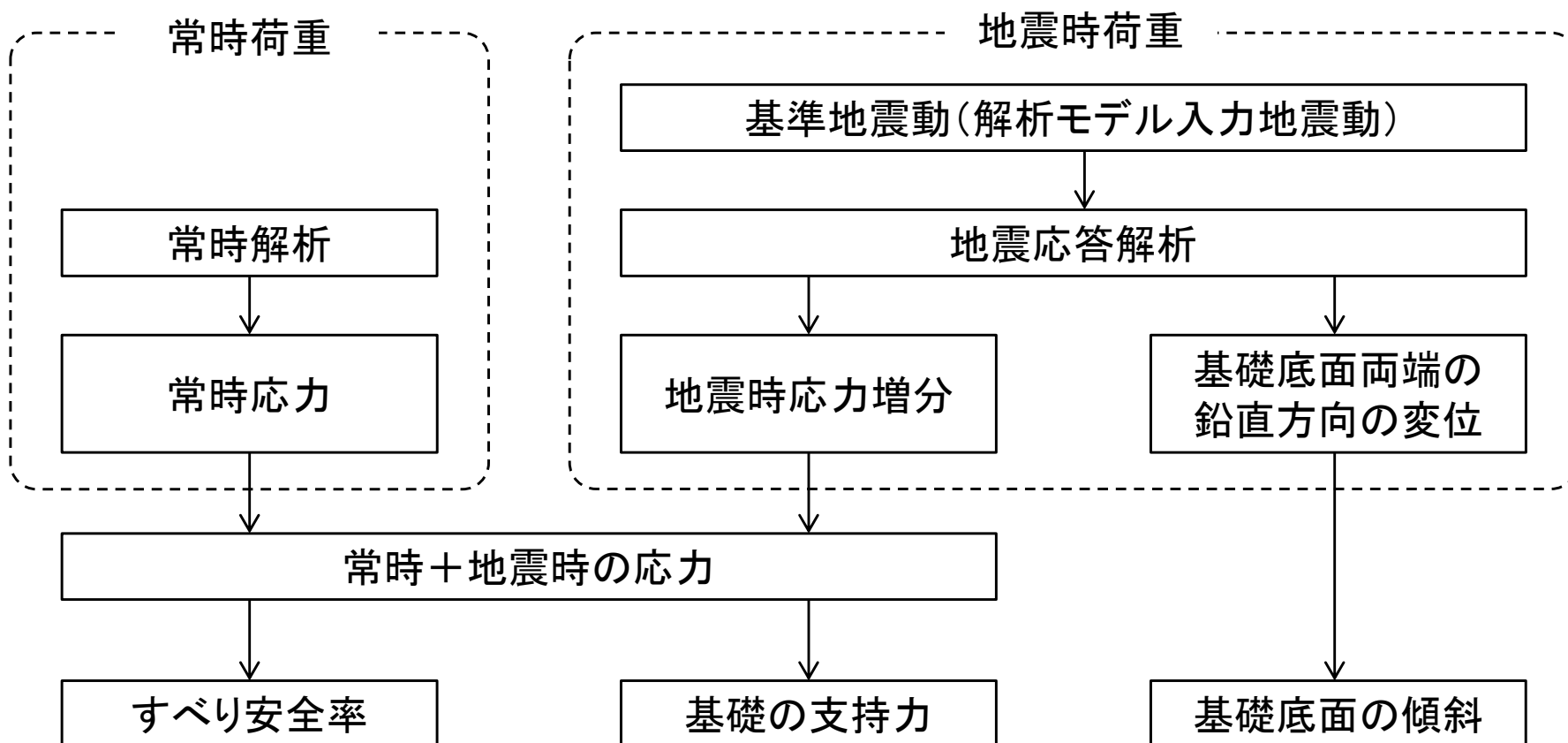
安定性評価フロー
