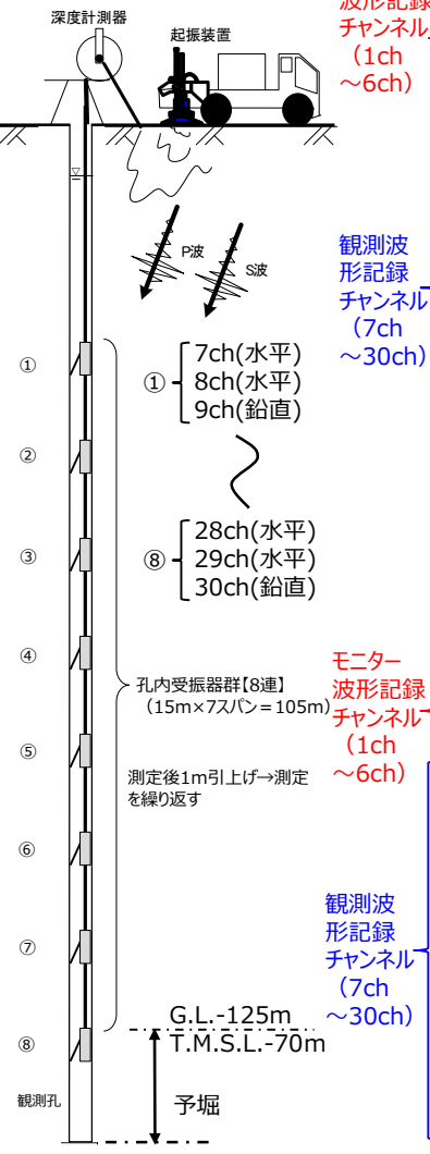
図3 Q値測定概要図
