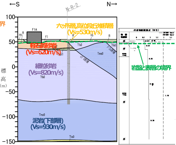
図5 中央地盤の地震観測位置の地質断面図及びPS検層結果
