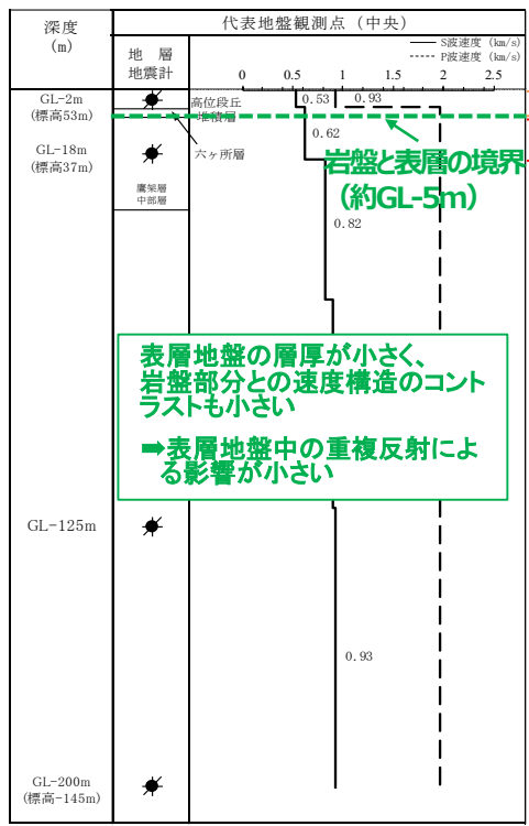
図13 地震観測位置の速度構造（中央地盤）
