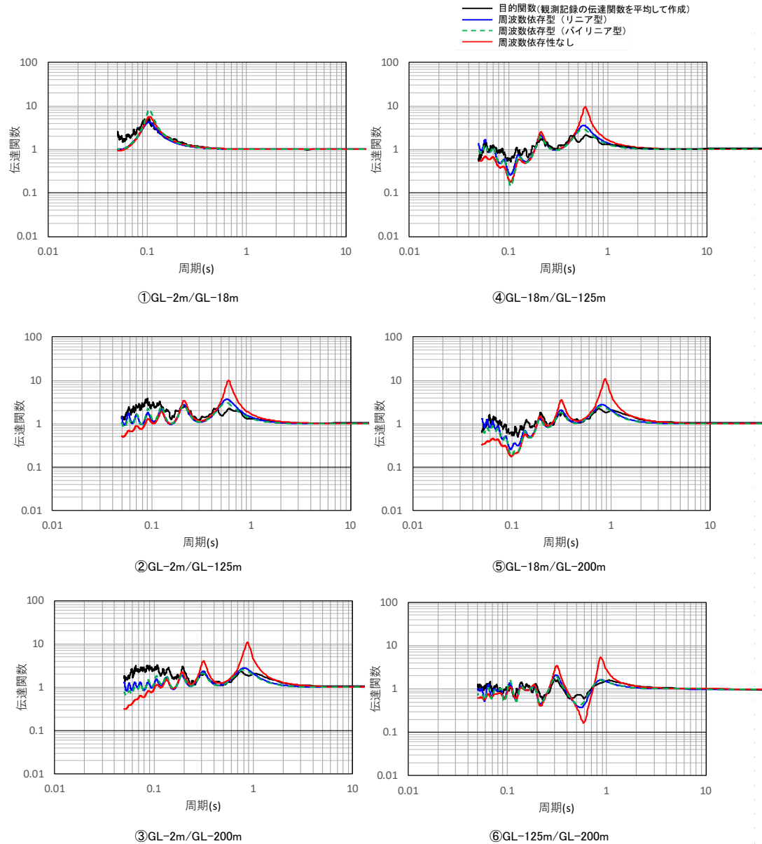
図 伝達関数の検討結果（中央地盤、水平）
