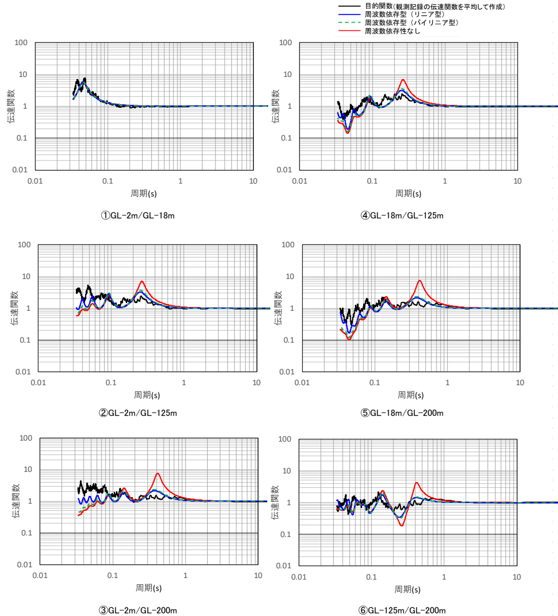
図 伝達関数の検討結果（中央地盤、鉛直）
