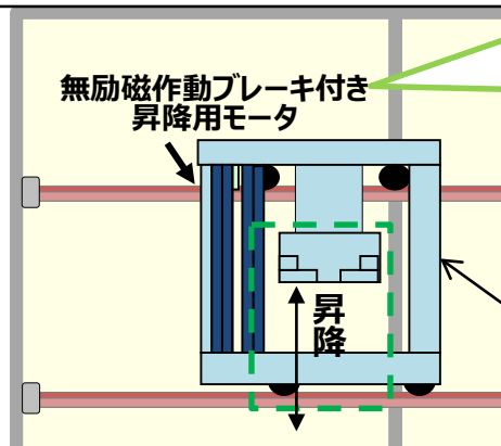
スタック編成設備グローブボックス
