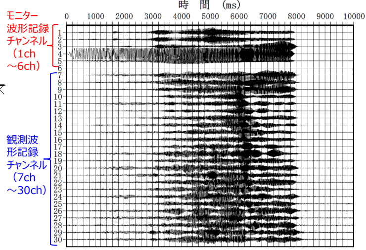
図4 起振波形及び孔内受振器による観測波形例 (コリレーション処理前: R5-Q6孔)
