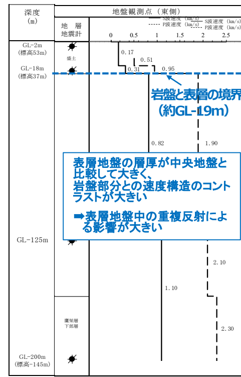
図14 地震観測位置の速度構造（東側地盤）
