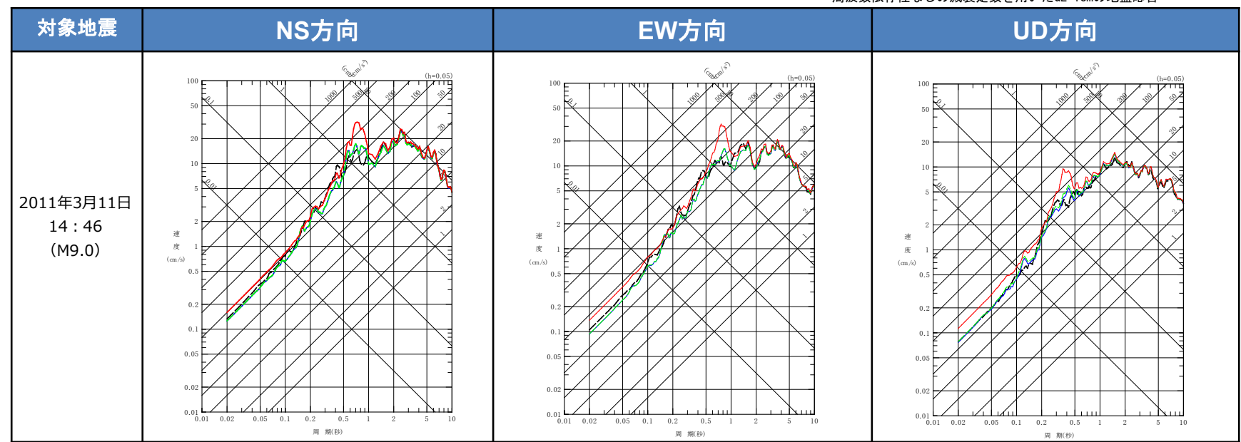
図11 地震観測記録に対するシミュレーション解析結果（東側地盤）
