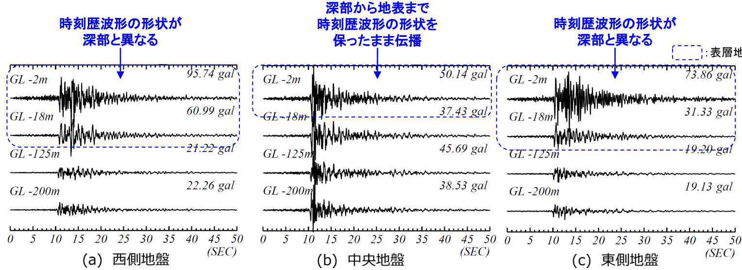
図3 観測記録の時刻歴波形（2012年5月24日 0時2分の地震）
