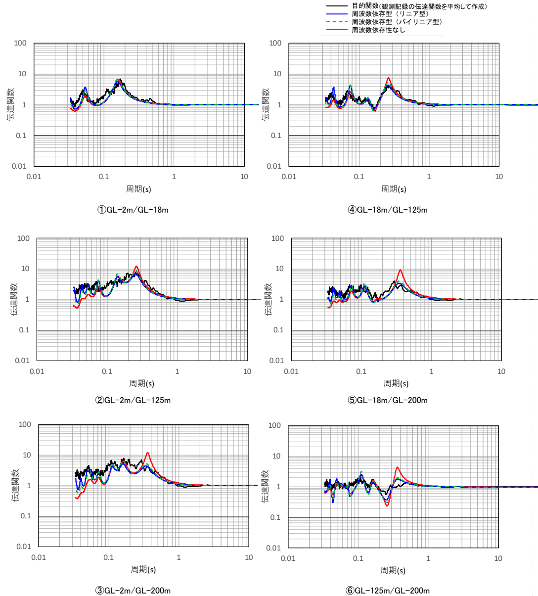
図 伝達関数の検討結果（東側地盤、鉛直）
