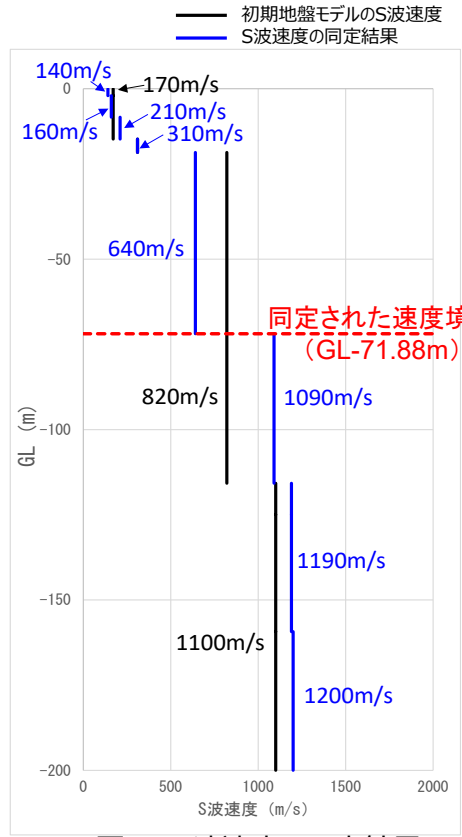
図9 S波速度の同定結果
