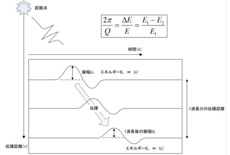
図6 振幅減衰の概念(Q値解析)
