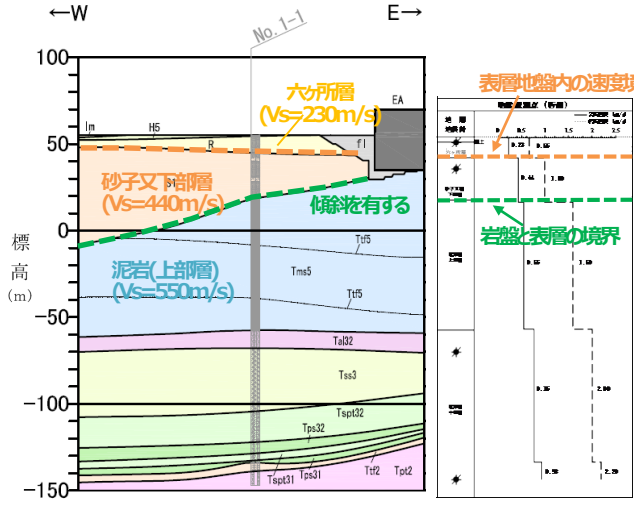
図4 西側地盤の地震観測位置の地質断面図及びPS検層結果
