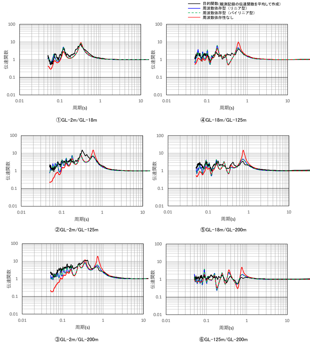
図 伝達関数の検討結果（東側地盤、水平）
