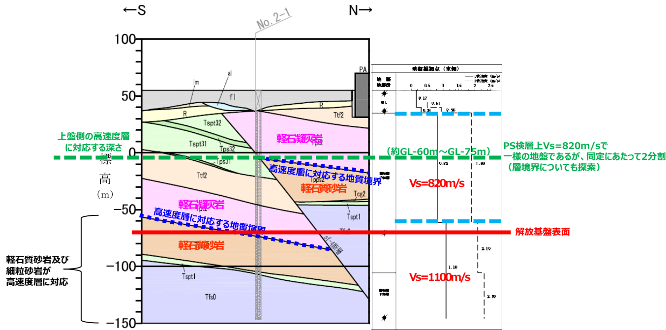
図7 東側地盤の地震観測位置の地質断面図及びPS検層結果側地盤
