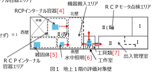
図1 地上1階の評価対象壁
