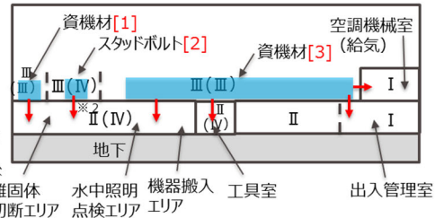
図 2 立面図 (B-B'断面)
