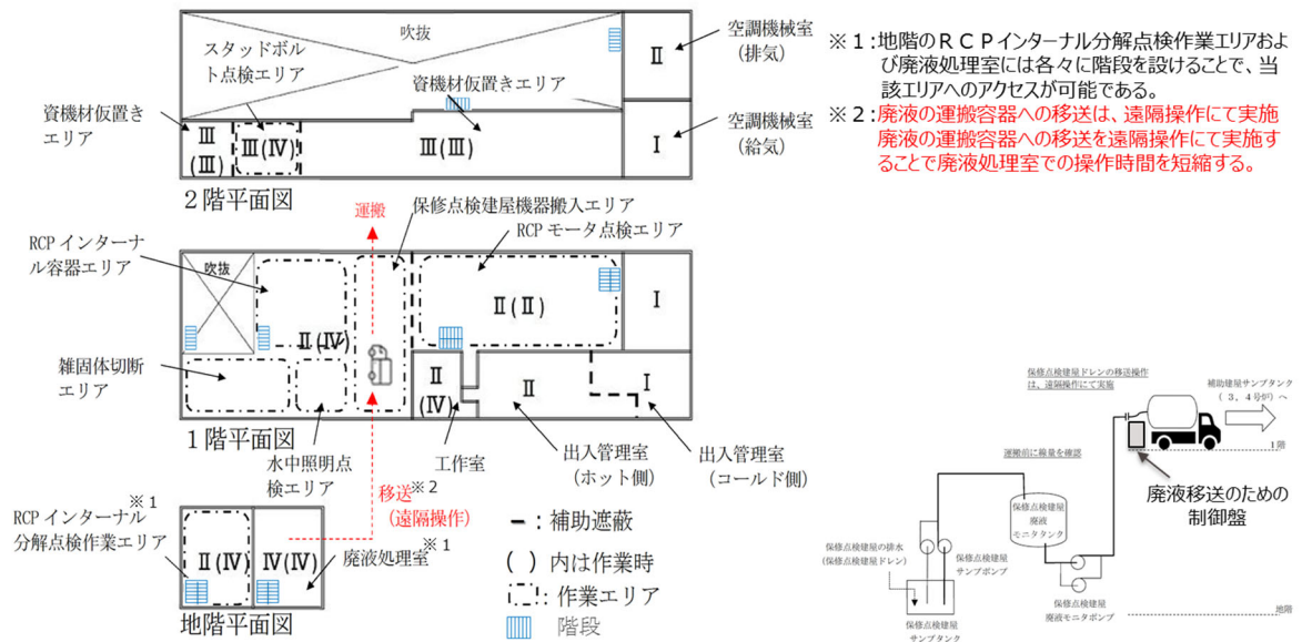
図1 保守点検建屋内の作業等エリアと遮蔽設計区分
