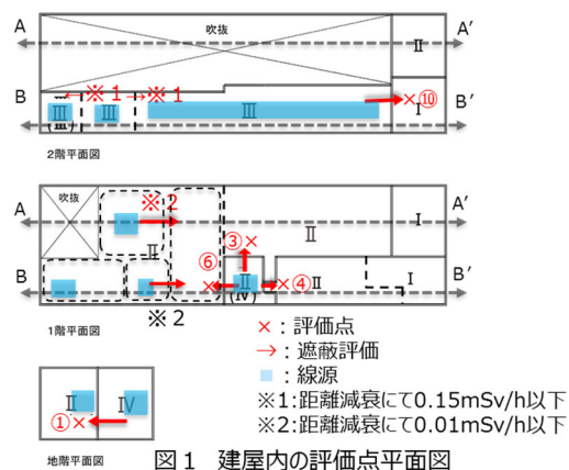
図1 建屋内の評価点平面図
