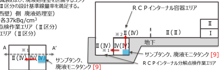
図2 立面図（A-A'断面）
