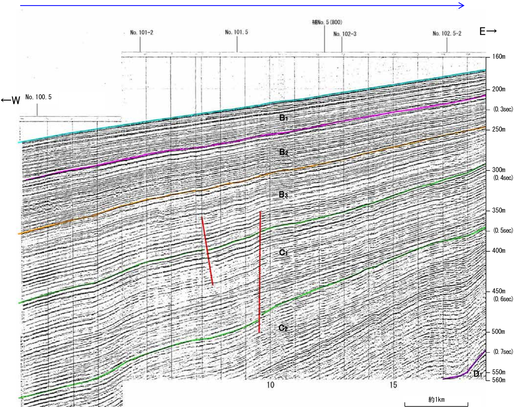
小断層群密集域
