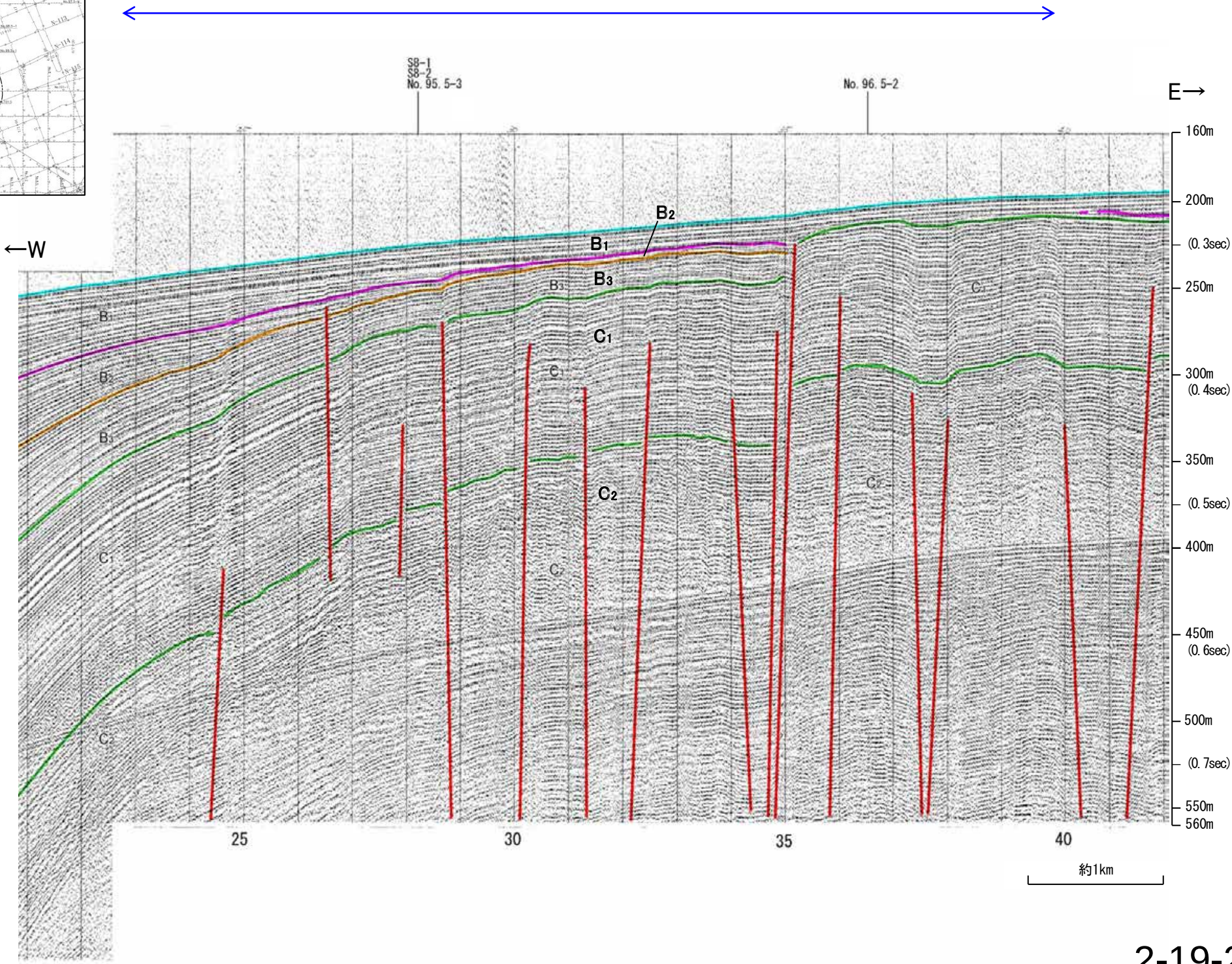
小断層群密集域
