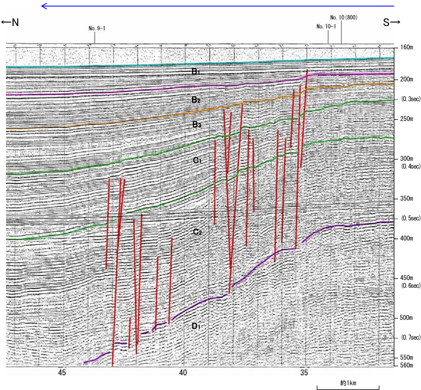
小断層群密集域
