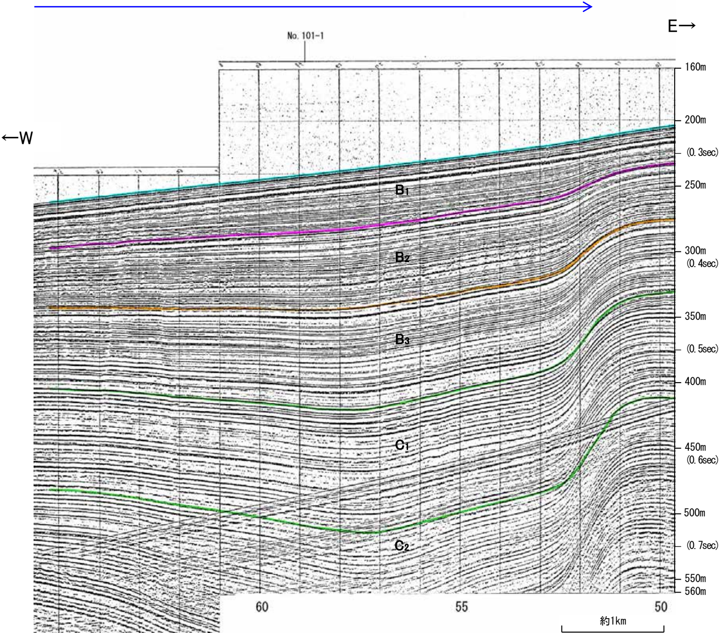
小断層群密集域
