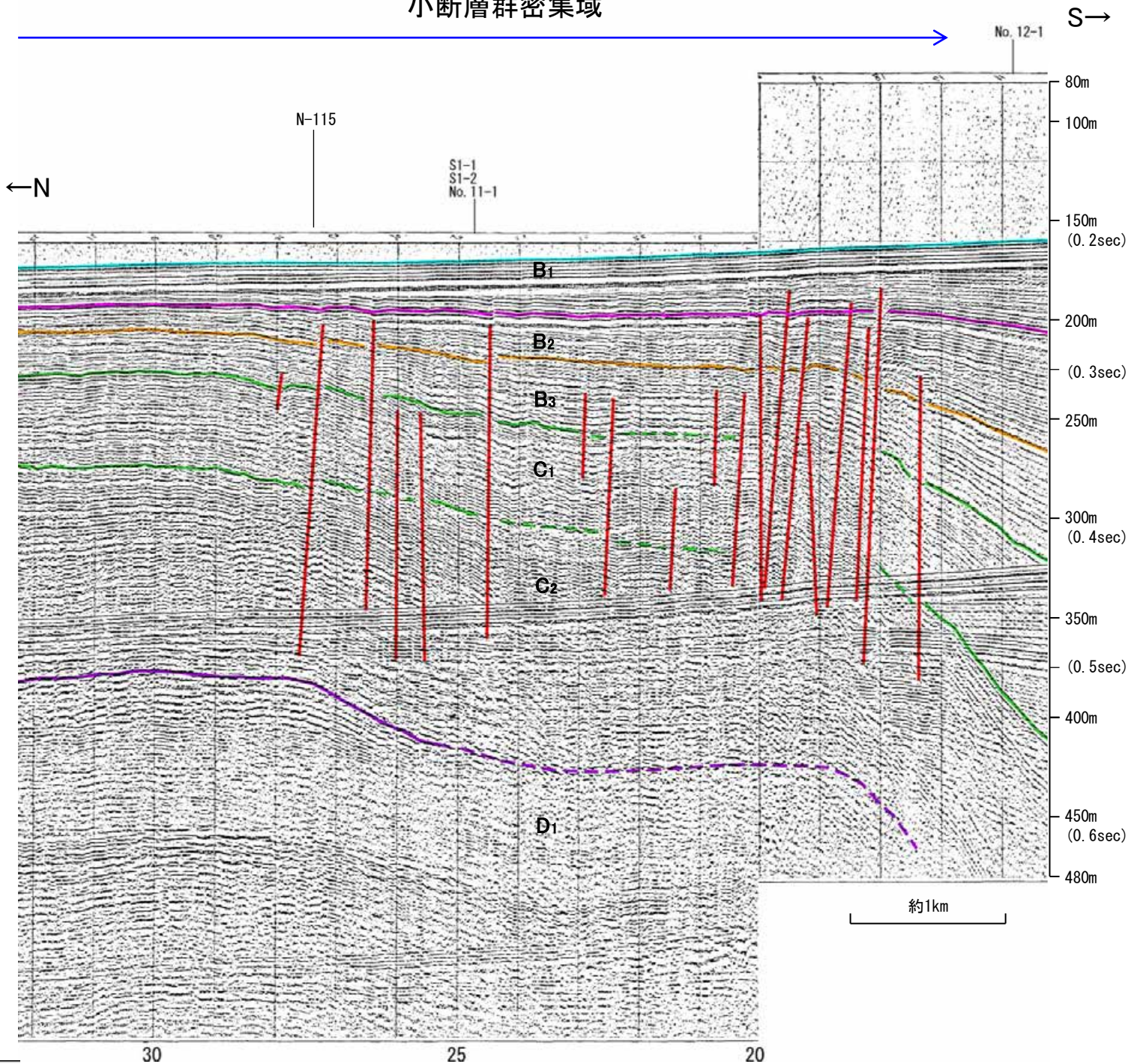
小断層群密集域
