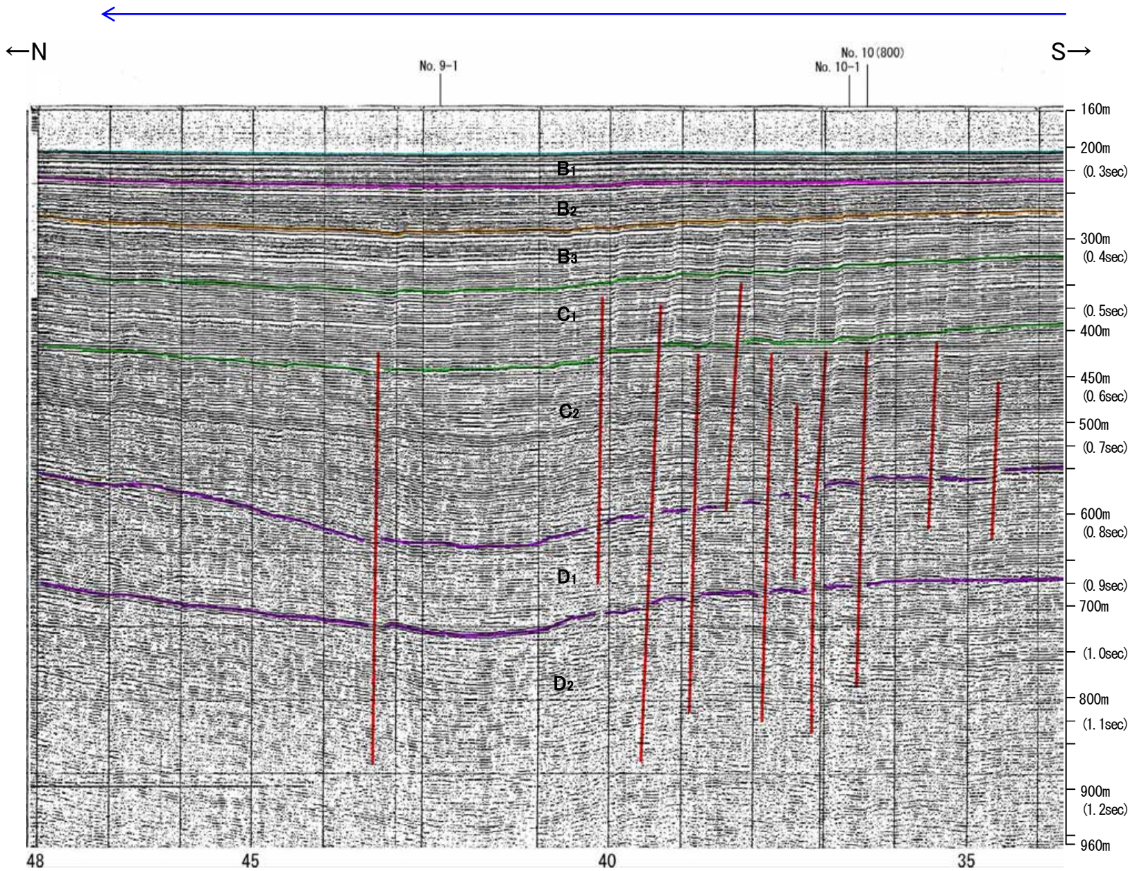
小断層群密集域
