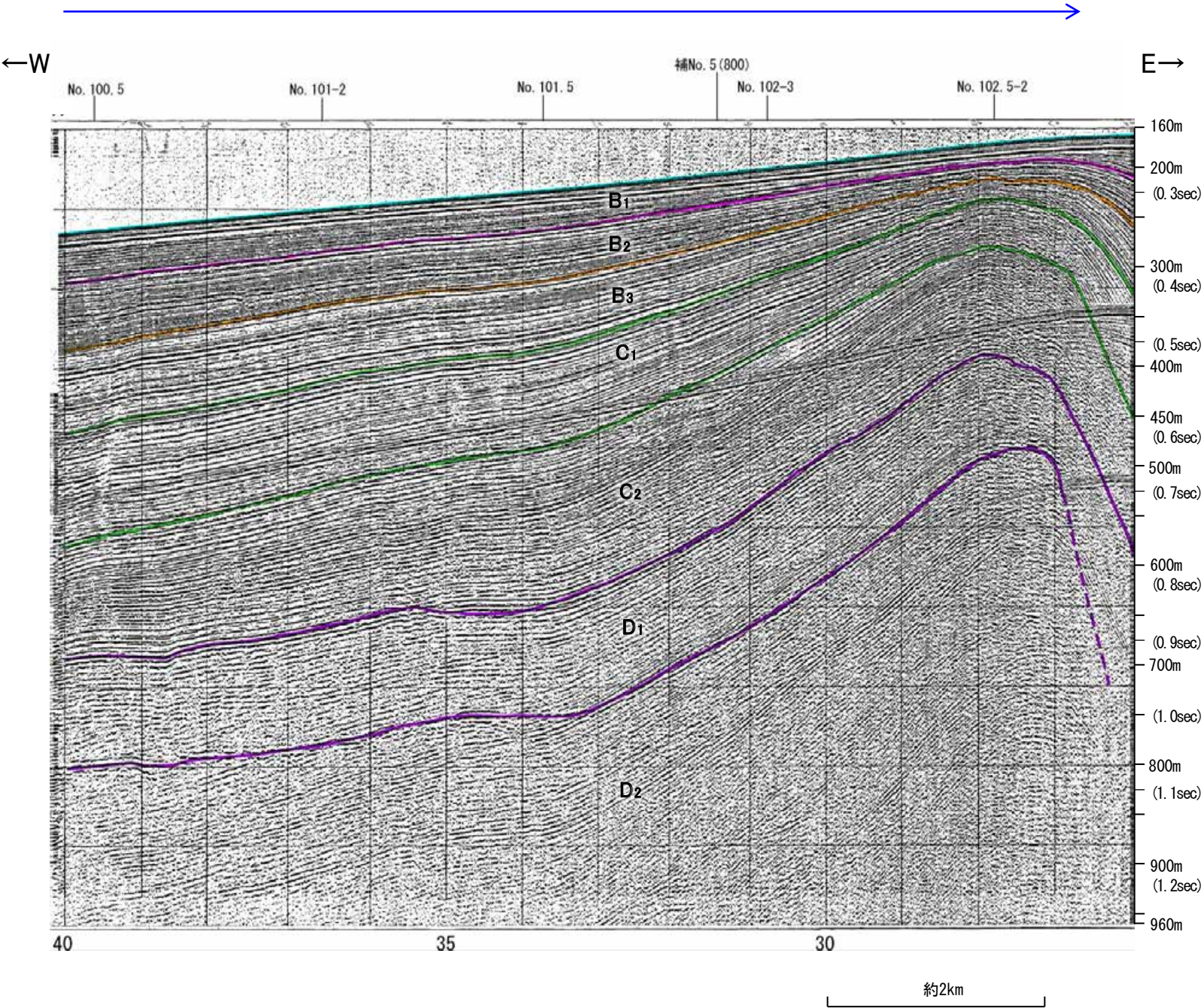
小断層群密集域
