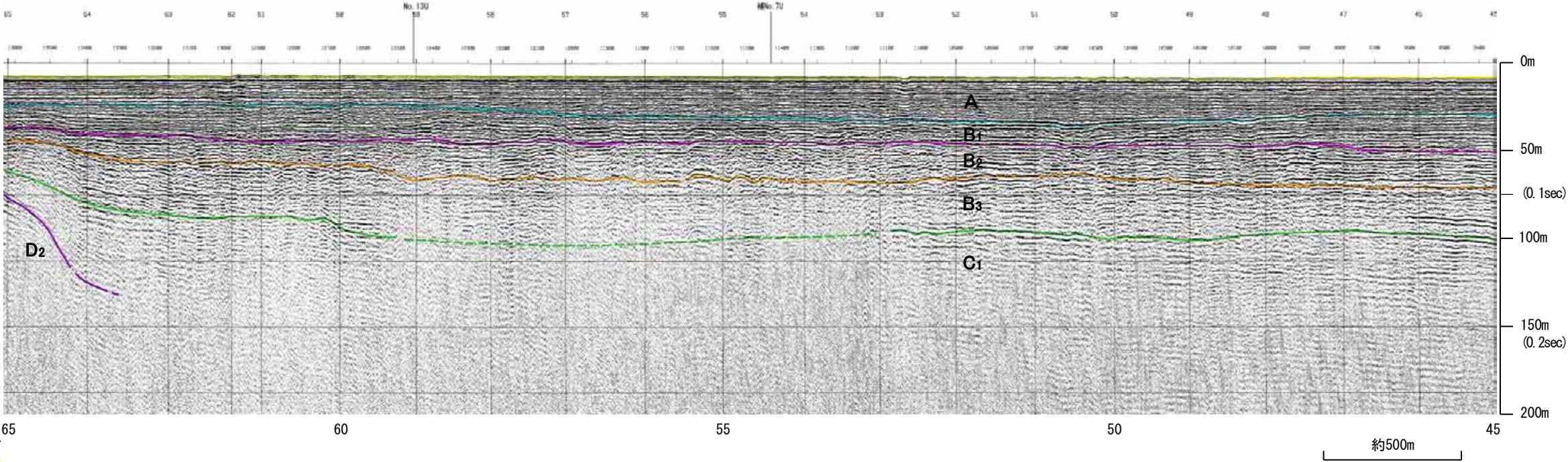
眉丈山第2断層 延長部
