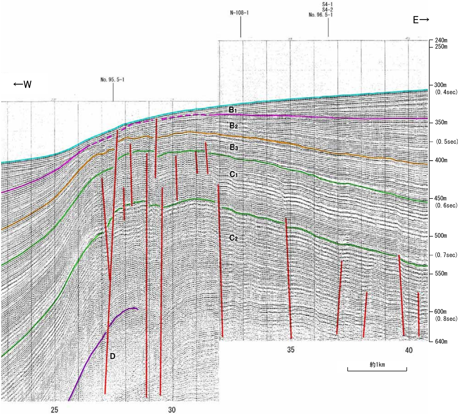
小断層群密集域
