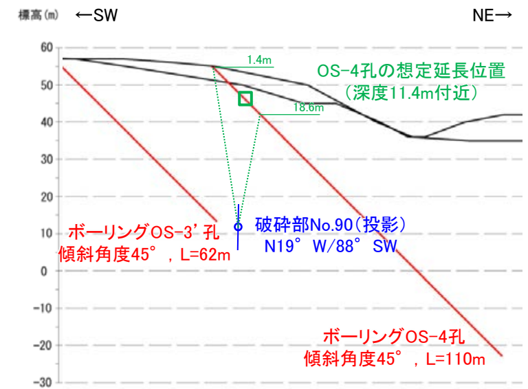
断面図
