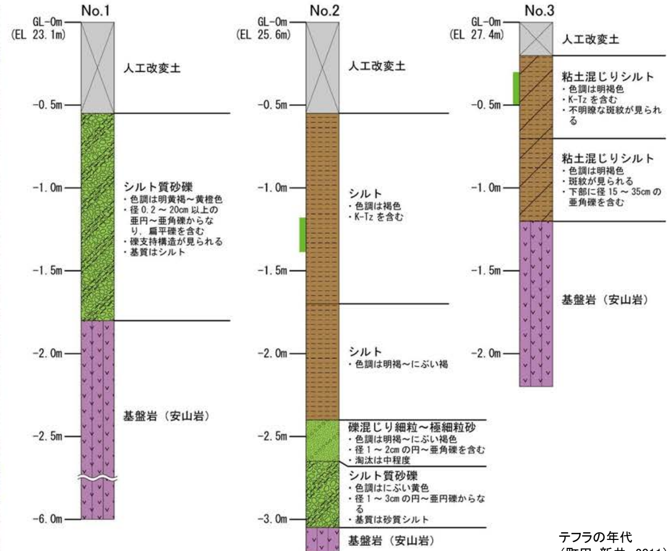
柱状図 凡例
