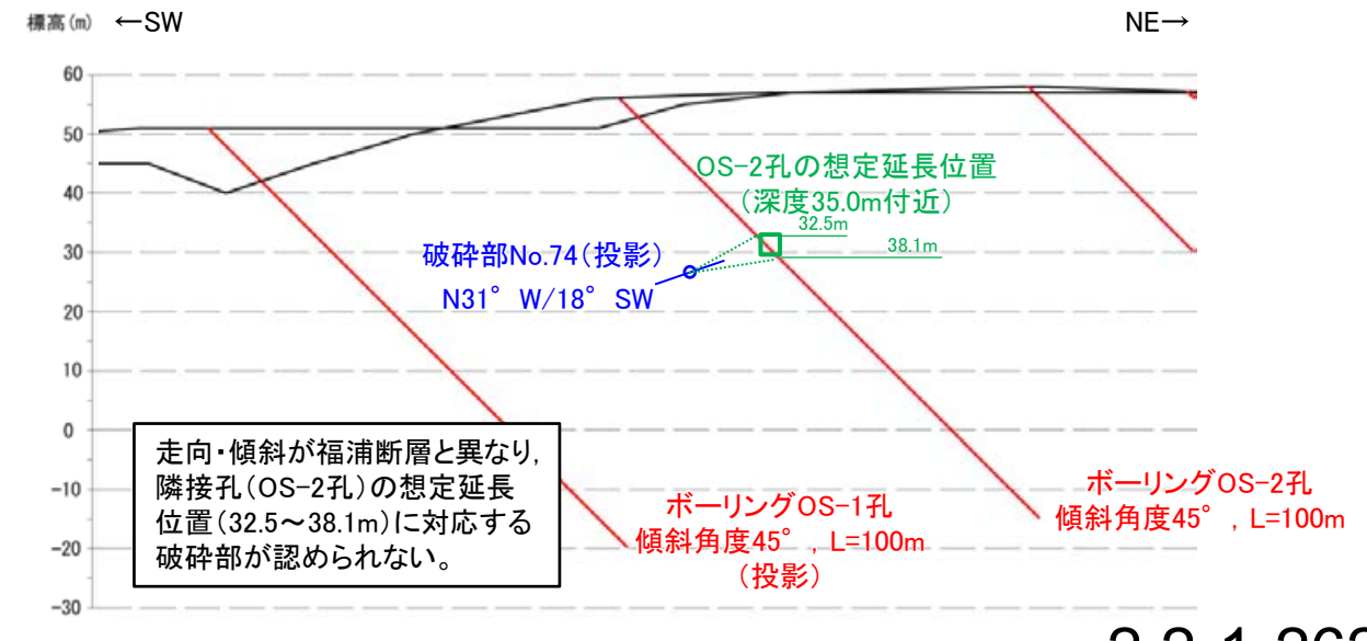
断面図
