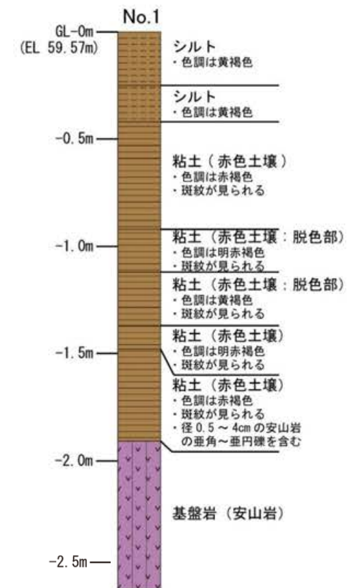
柱状図
