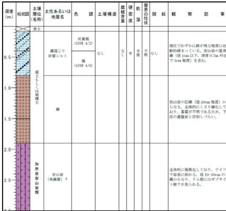
柱状図i
