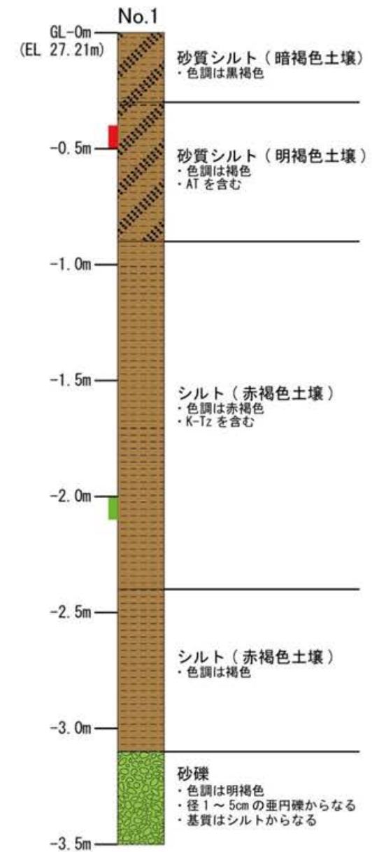
柱状図
