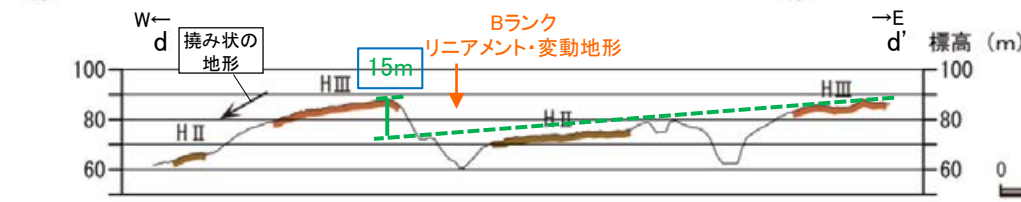
地形断面図(H:V=1:4)(断面は航空レーザ計測データにより作成)
