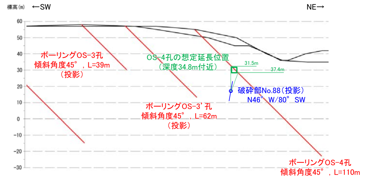
断面図
