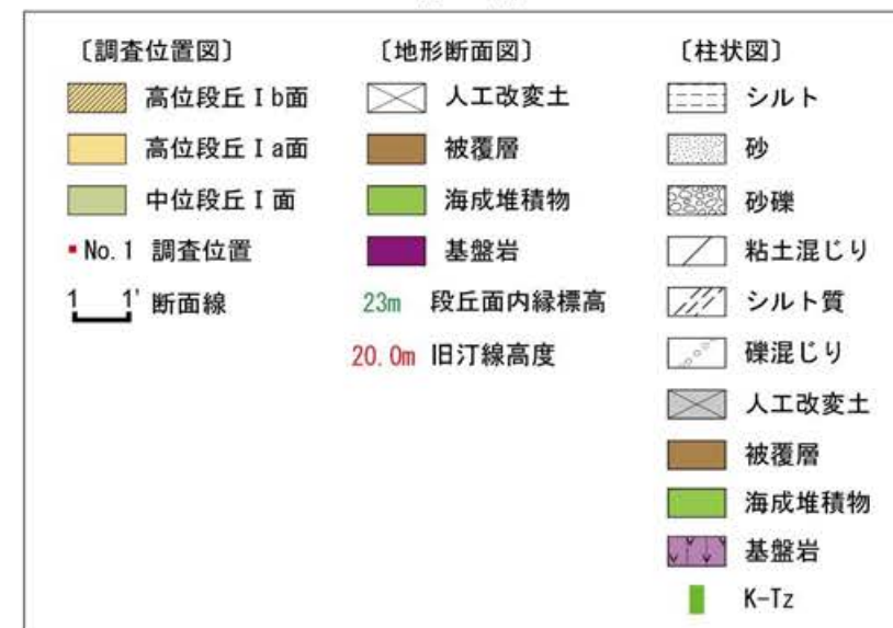
柱状図 凡例
