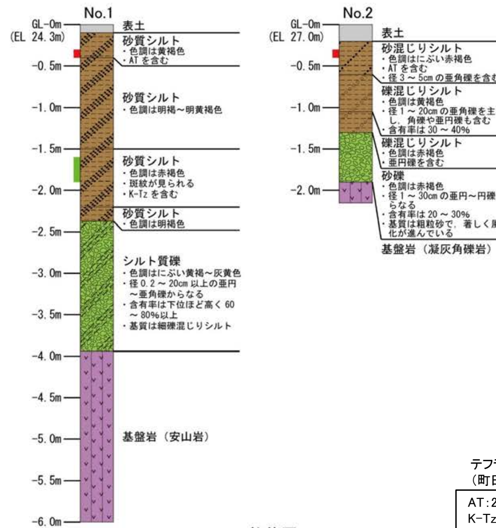
柱状図
