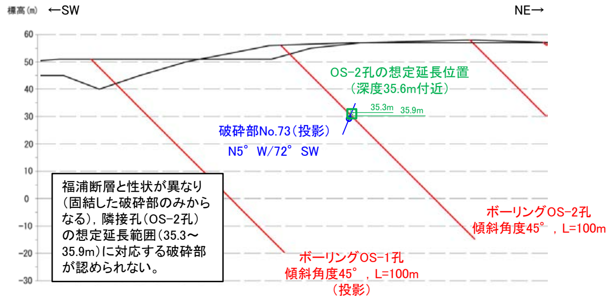
断面図
