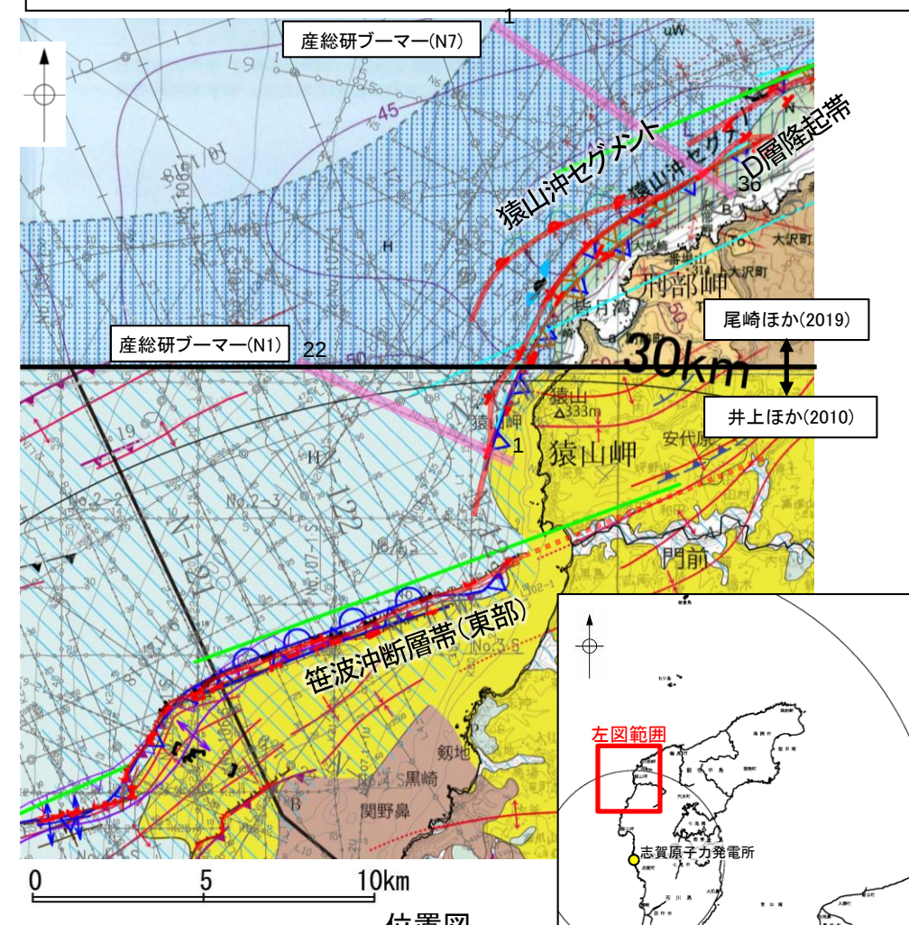
位置図 (井上ほか(2010), 尾崎ほか(2019)に加筆)
