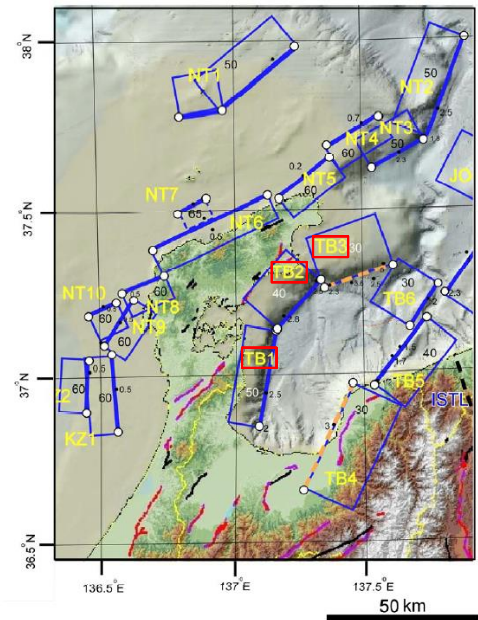
富山湾西側海域断層に対応するTB1, TB2, TB3の位置図 (文科省ほか(2015)を一部加筆) 矩形内の白数字は断層の傾斜(単位は度)
