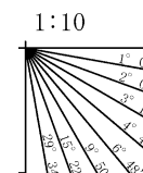
断層位置 (細線は分岐断層と評価したもの)
