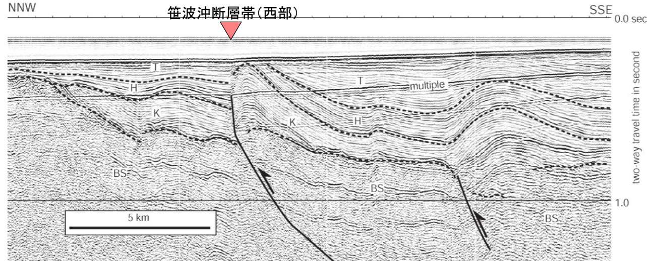
Fig.17解釈断面図(岡村, 2007a)に加筆
