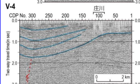
砺波平野における地下構造探査記録にみる活構造 (後藤ほか(2015)が石油公団(1982, 1983)の反射法地震探査記録に加筆して作成)(一部加筆)
