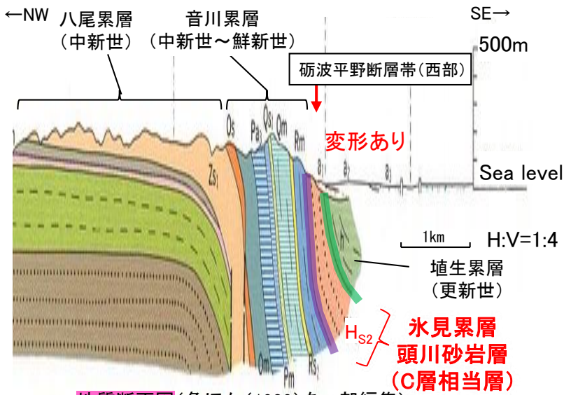
地質断面図(角ほか(1989)を一部編集)
