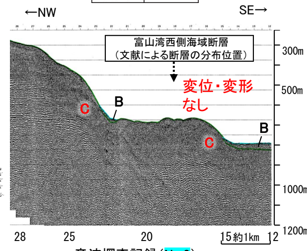
音波探査記録(No.8)
