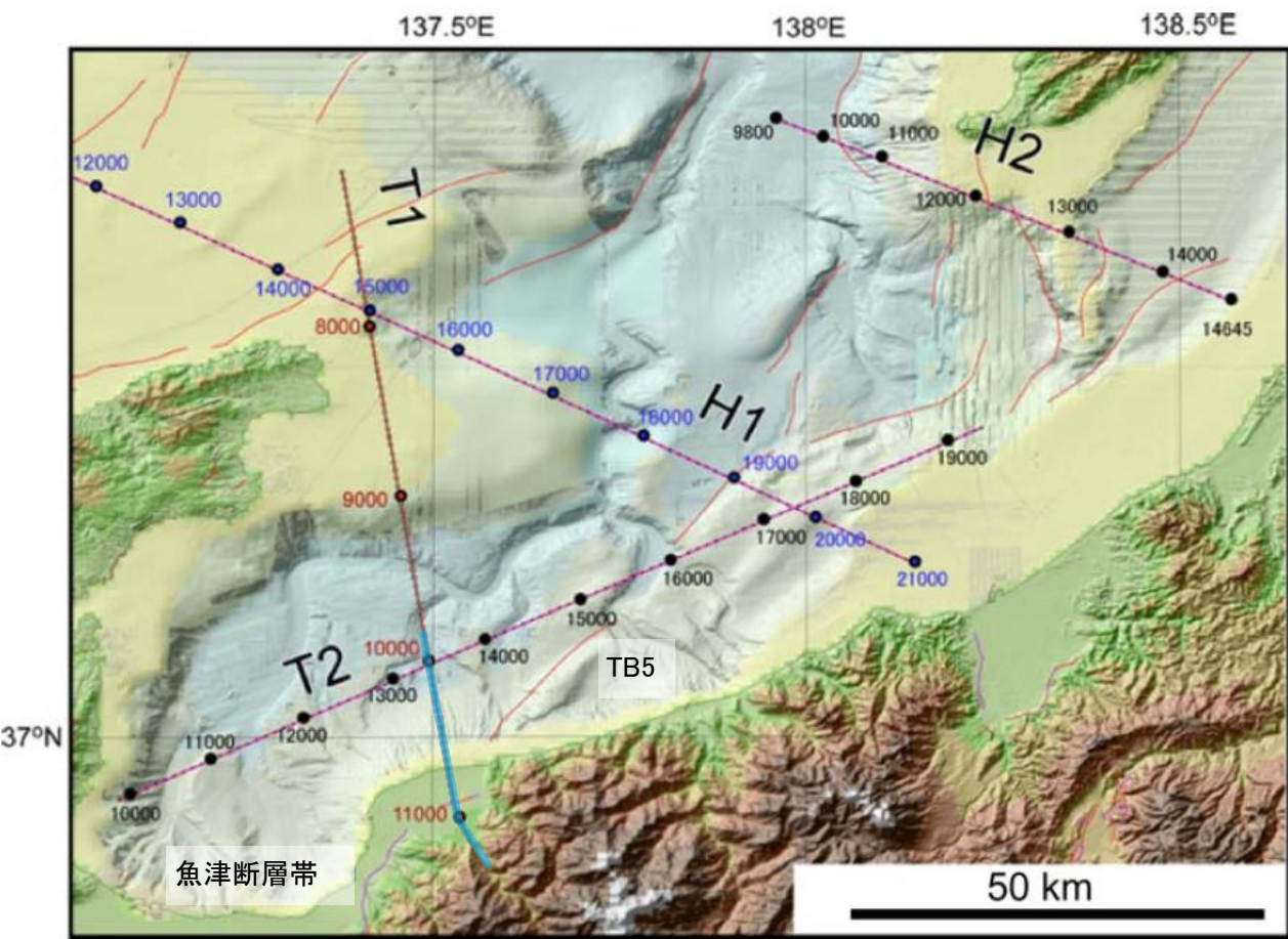
赤線:岡村(2002), 中田・今泉(2002)による活断層 上越沖海域周辺の測線図 文科省ほか(2015)に一部加筆
