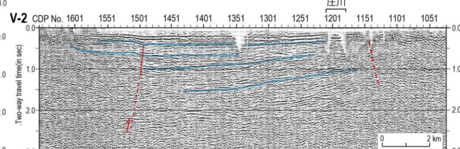
砺波平野における地下構造探査記録にみる活構造 (後藤ほか(2015)が石油公団(1982, 1983)の反射法地震探査記録に加筆して作成)(一部加筆)
