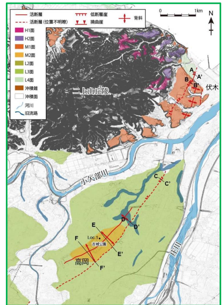
伏木～高岡の地形分類図(後藤ほか, 2015)
