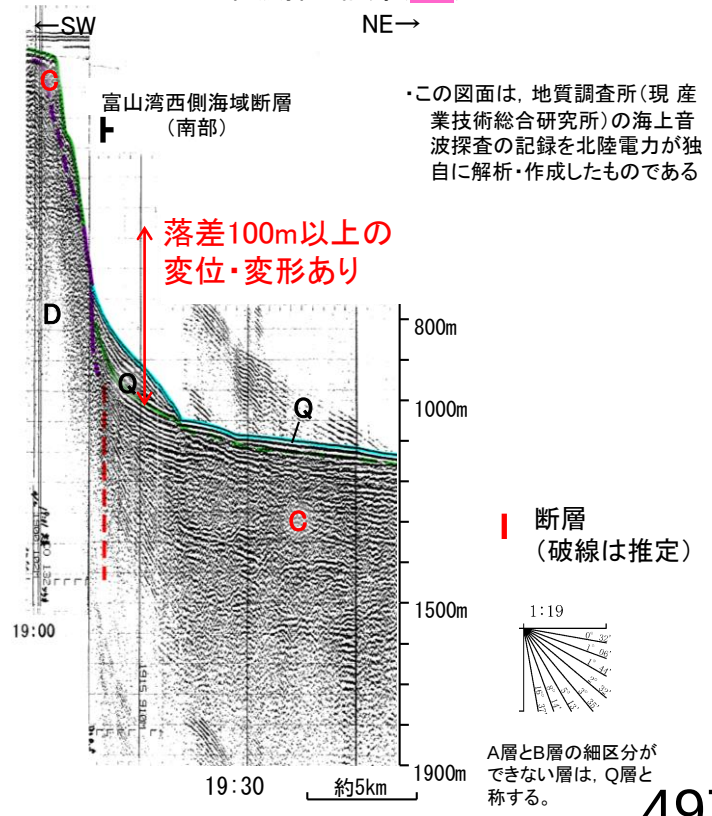
音波探査記録(N-4E)
