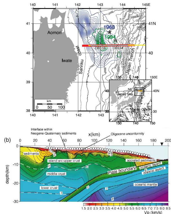
1968年の地震と1994年の地震の共通アスペリティ付近の地質構造 (Ito et al.(2004))
