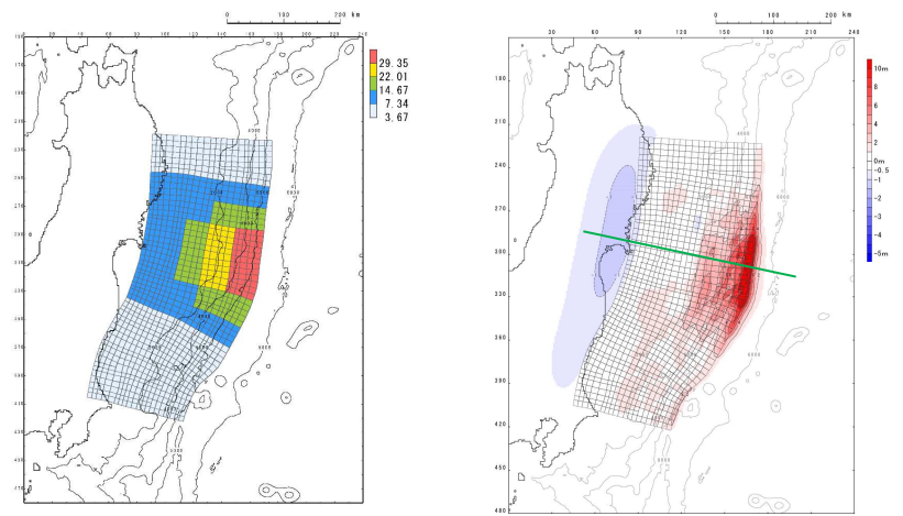
地殻変動量分布(平面図)
