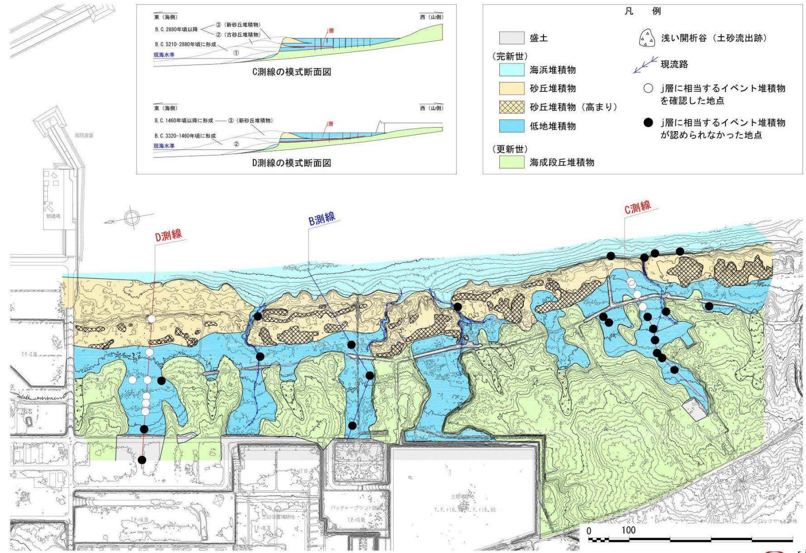
D4孔で認められた分布最高標高のイベント堆積物と同層準のイベント堆積物(j層)の分布
