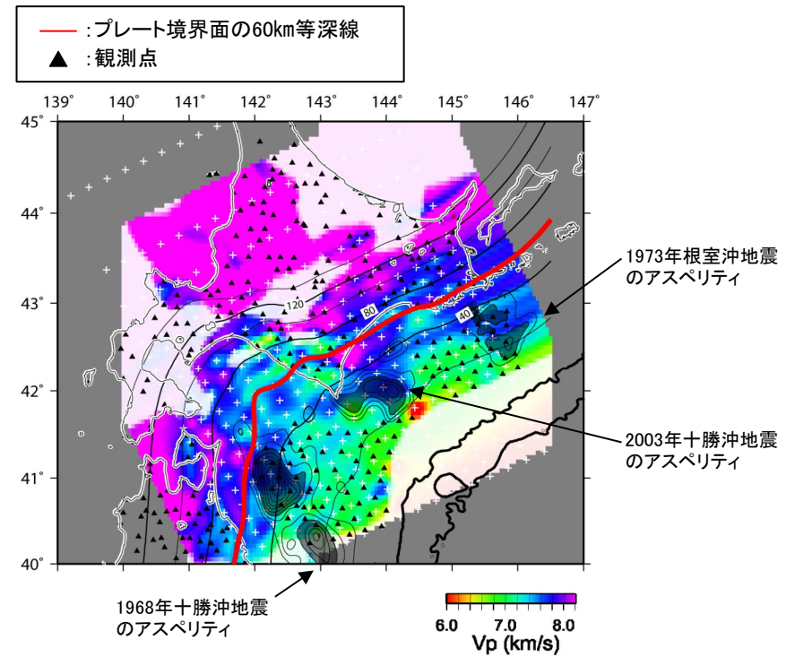
プレート境界面直下5kmにおけるVpの分布とプレート境界地震の破壊域、相似地震の震央の分布との比較 (文部科学省(2008a)一部加筆)
