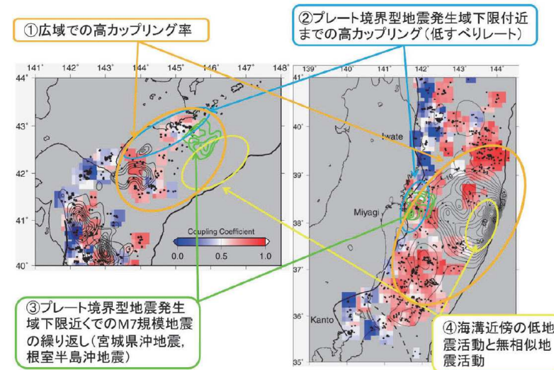
第2図. 北海道南東沖(左)および東北地方東方沖(右)の繰り返し地震分布(黒丸)およびそれにより推定したプレート間カップリング率(カラー)の比較. カップリング率は0.3°×0.3°のグリッドごとに、3つ以上の小繰り返し地震グループが存在する場所について推定した. 緑および黒のコンターはM7以上の地震のすべり量分布(Yamanaka and Kikuchi, 2004 6) ; Iinuma et al., 2012 7) ). 関東地方の沖の破線は、フィリピン海プレートの北東限(Uchida et al., 2009 8) ).
